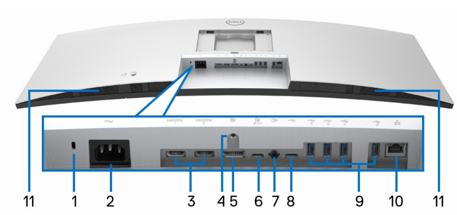
Ansicht von unten ohne Monitor-Standfuß
