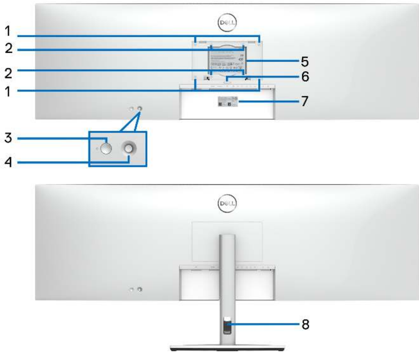
Rückansicht mit Monitorständer
