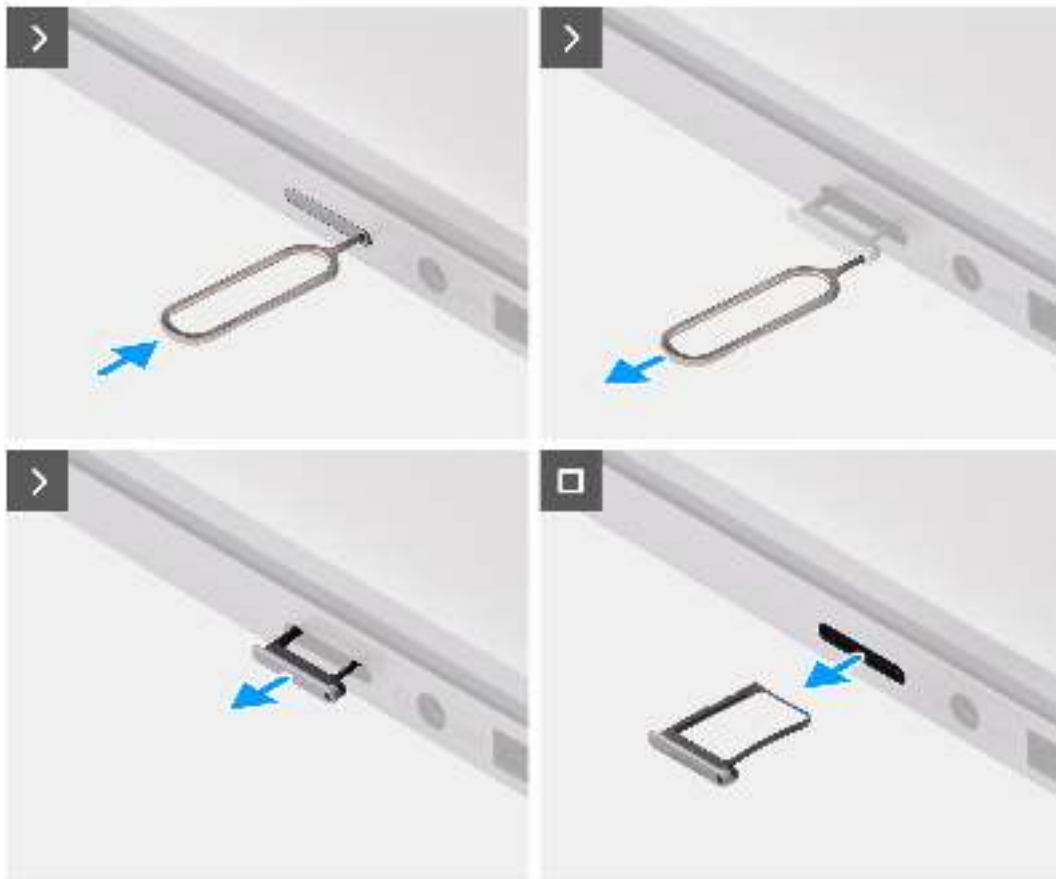
Abbildung 13. Entfernen des SIM-Kartenfachs
