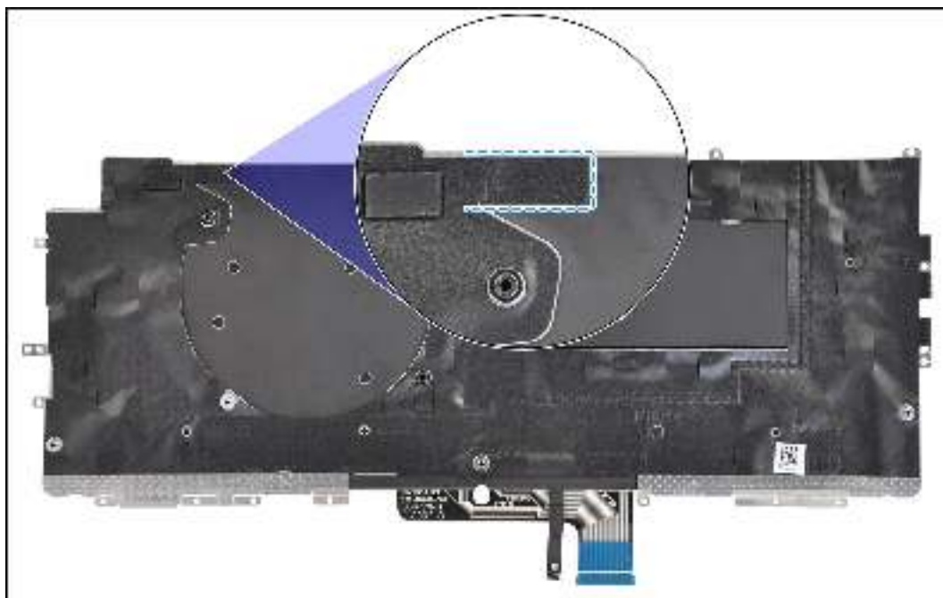
Abbildung 80. Entfernen der Tastaturfolie
