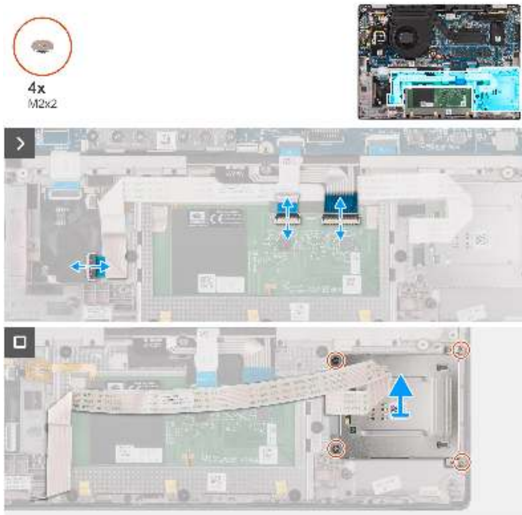
Abbildung 56. Entfernen des Smartcardlesegeräts
