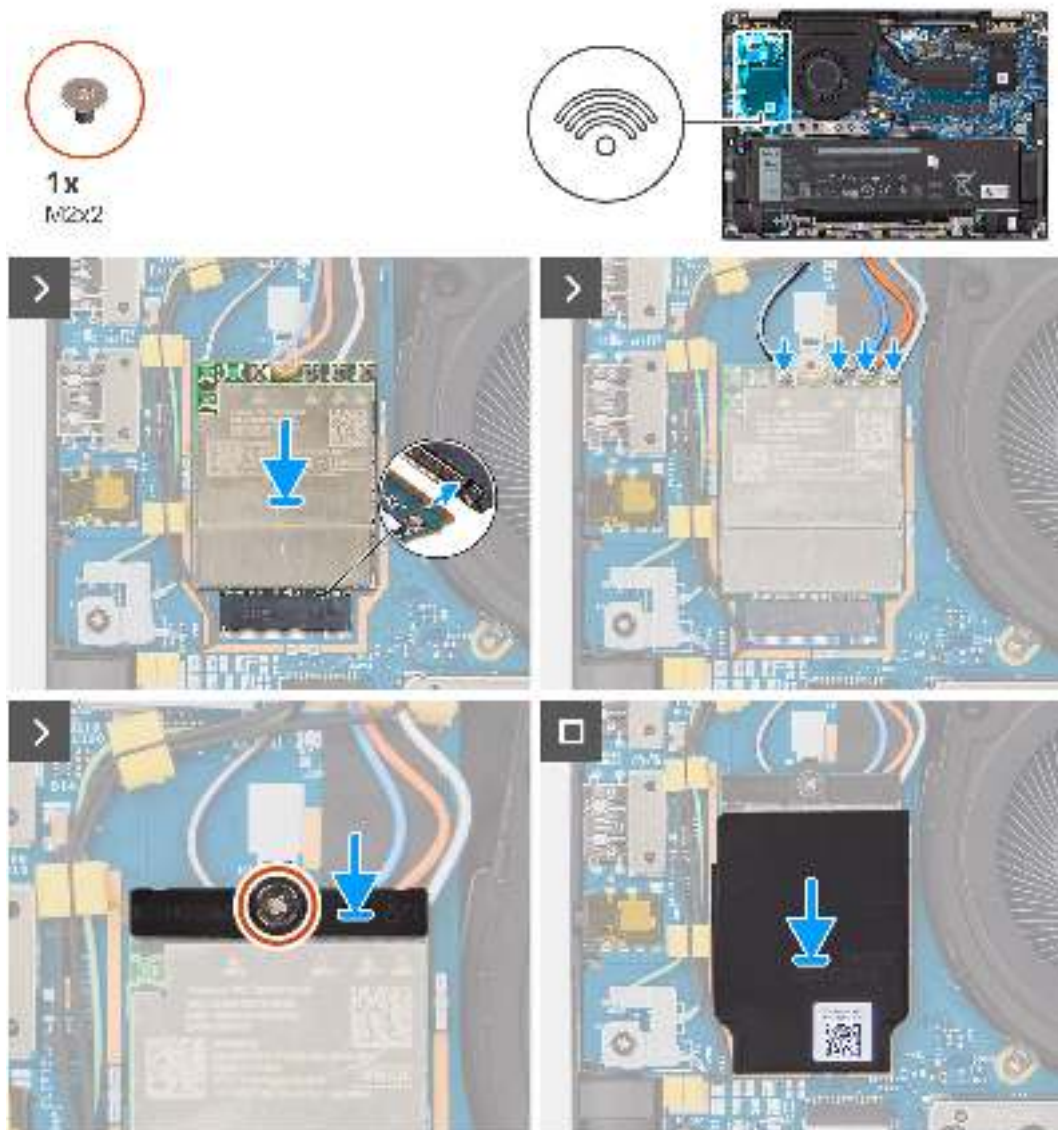
Abbildung 27. Installieren der 5G-WWAN-Karte
