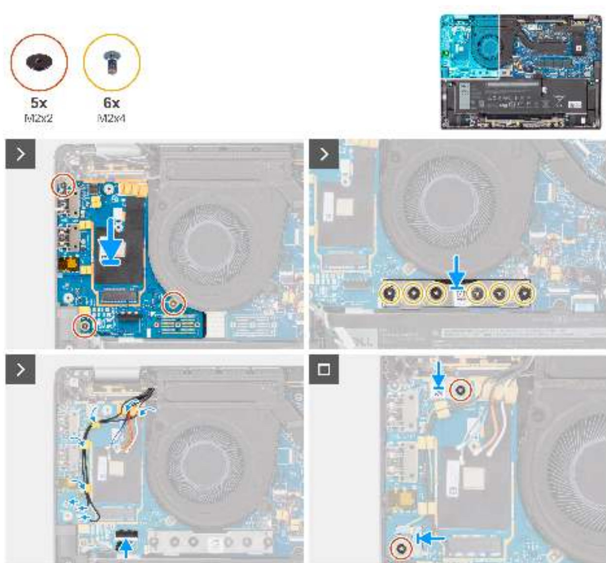
Abbildung 75. Installieren der I/O-Zusatzplatine
