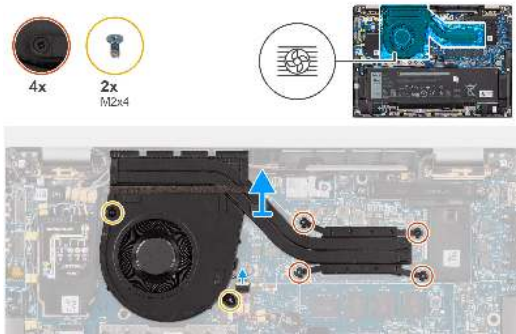
Abbildung 46. Entfernen der Kühlkörper/Lüfter-Baugruppe
