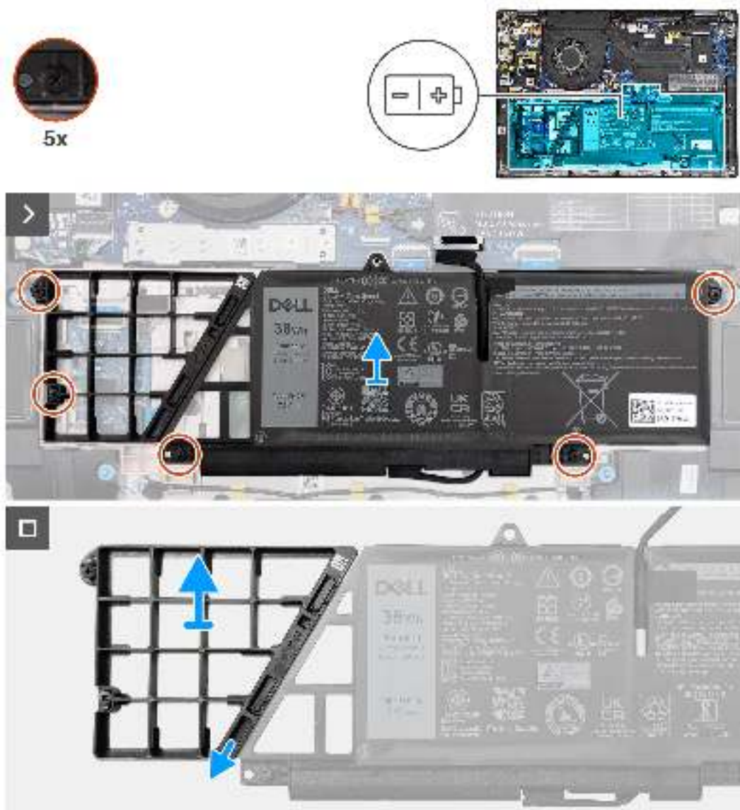
Abbildung 37. Entfernen des 2-Zellen-Akkus
