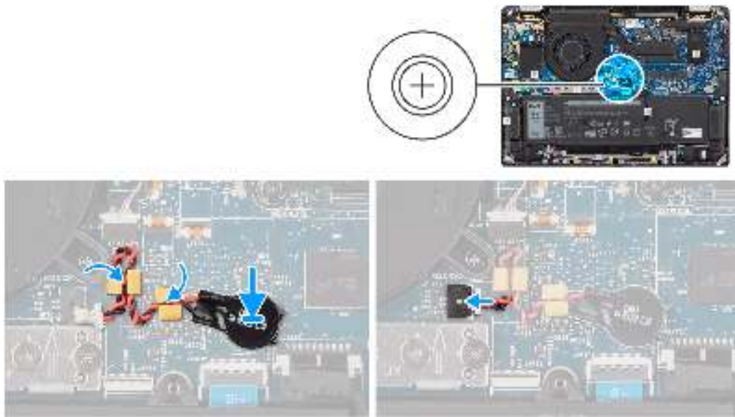
Abbildung 36. Installieren der Knopfzellenbatterie
