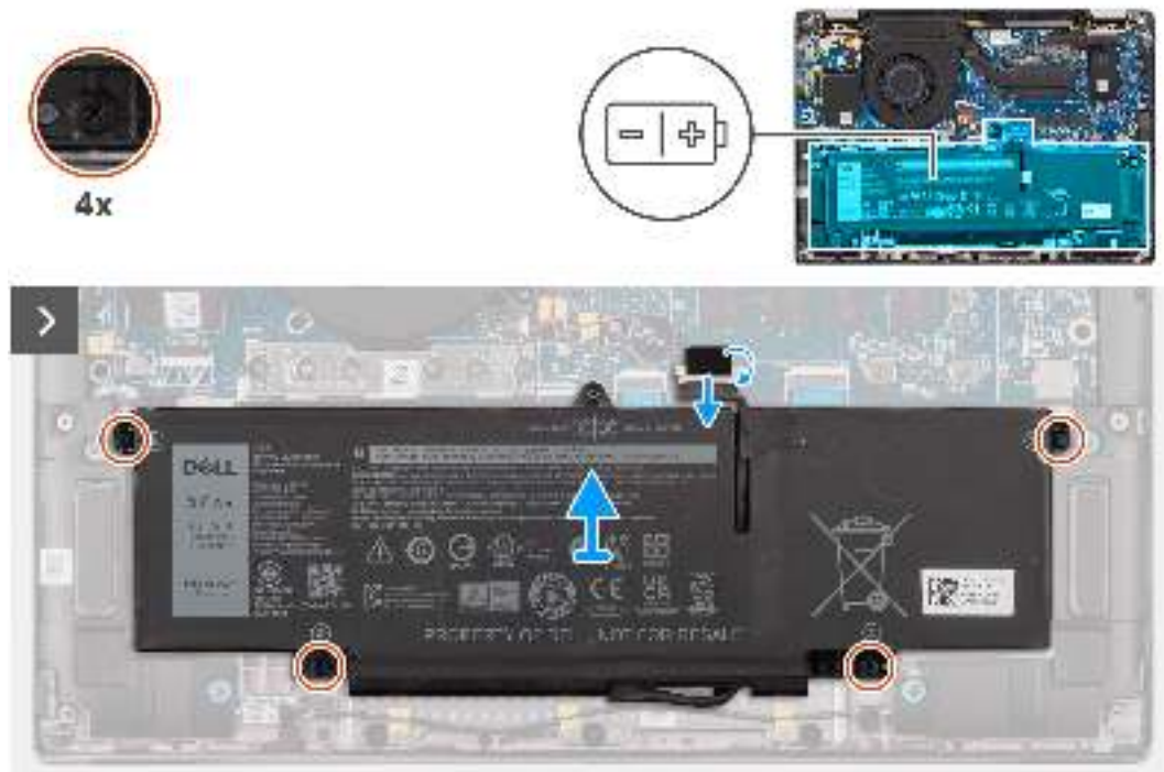
Abbildung 40. Entfernen des 3-Zellen-Akkus
