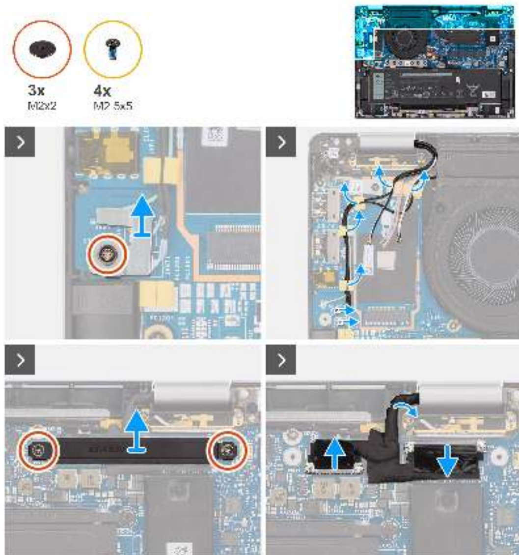
Abbildung 48. Entfernen der Displaybaugruppe
