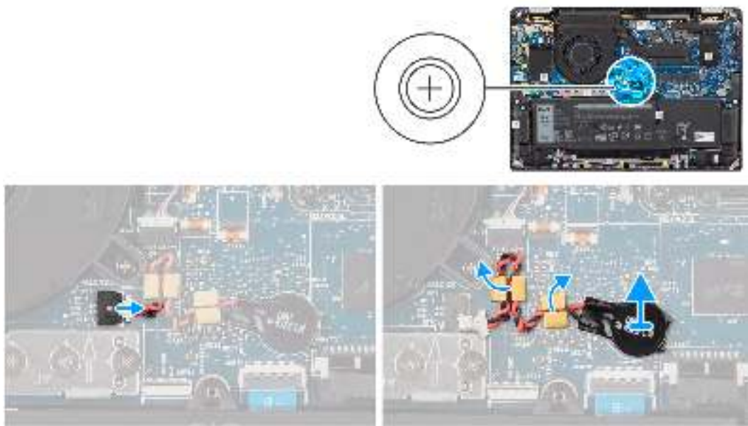
Abbildung 35. Entfernen der Knopfzellenbatterie
