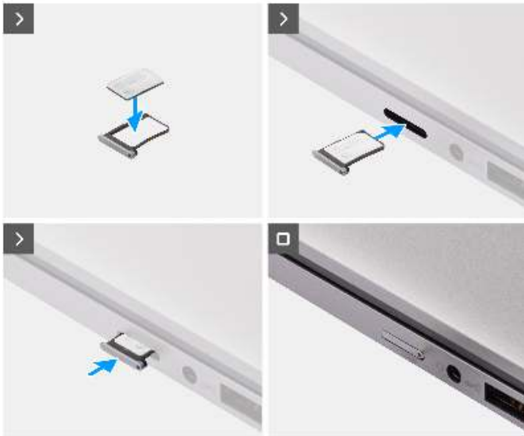
Abbildung 15. Installieren des SIM-Kartenfachs
