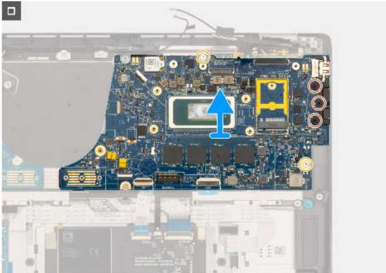
Abbildung 60. Entfernen der Hauptplatine
