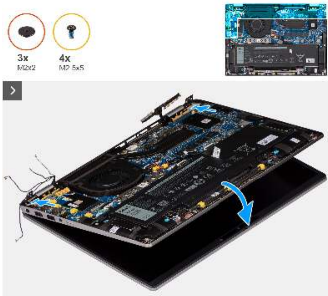
Abbildung 53. Installieren der Displaybaugruppe
