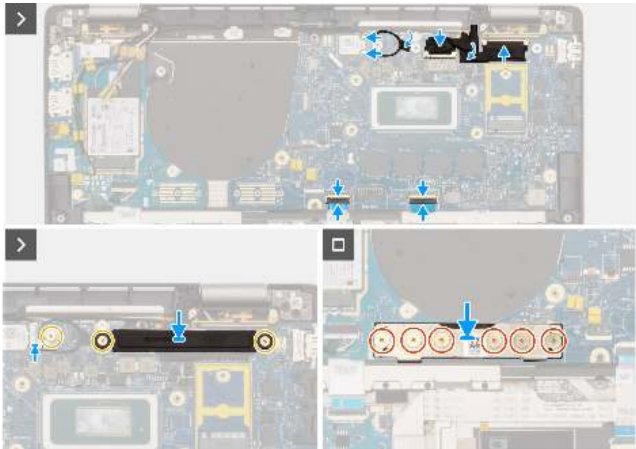
Abbildung 65. Installieren der Hauptplatine
