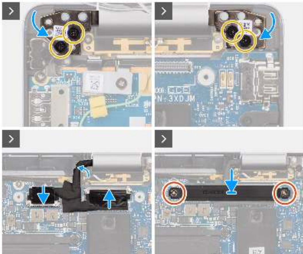
Abbildung 54. Installieren der Displaybaugruppe
