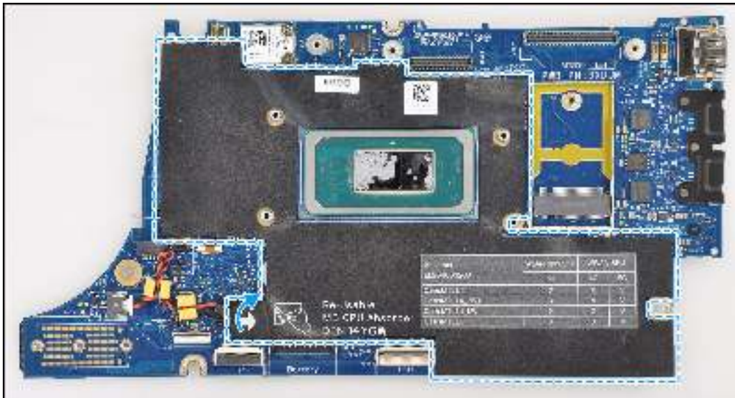
Abbildung 61. CPU-Absorber
