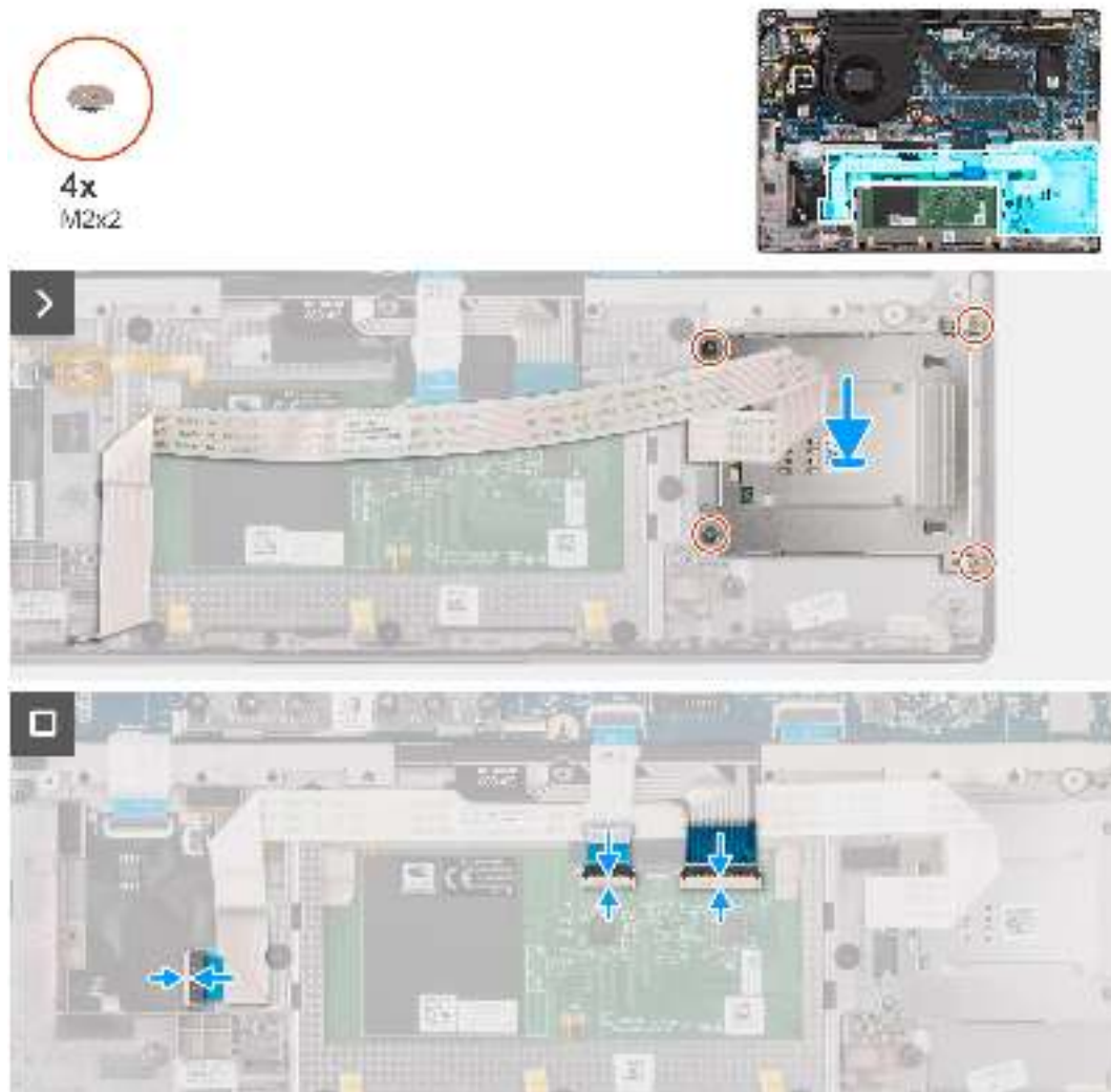
Abbildung 57. Installieren des Smartcardlesegeräts
