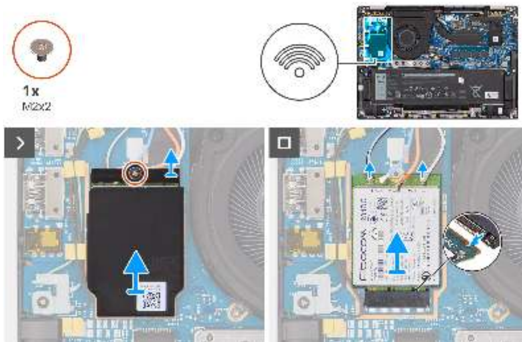
Abbildung 24. Entfernen der 4G-WWAN-Karte
