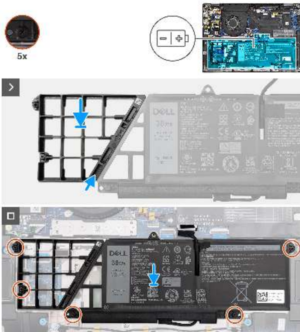
Abbildung 39. Installieren des 2-Zellen-Akkus
