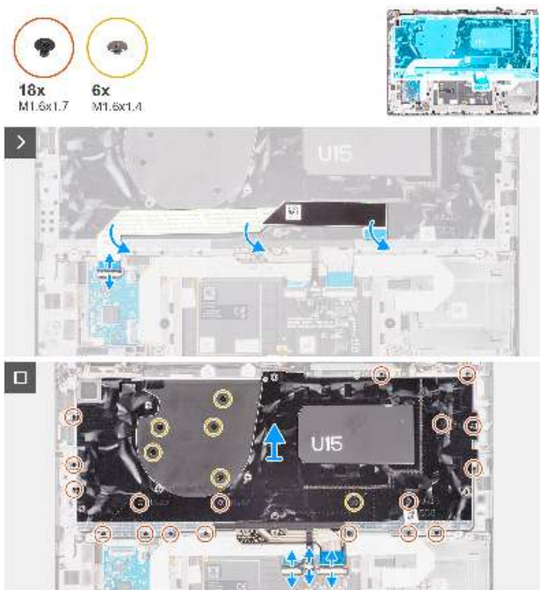
Abbildung 78. Entfernen der Tastatur
