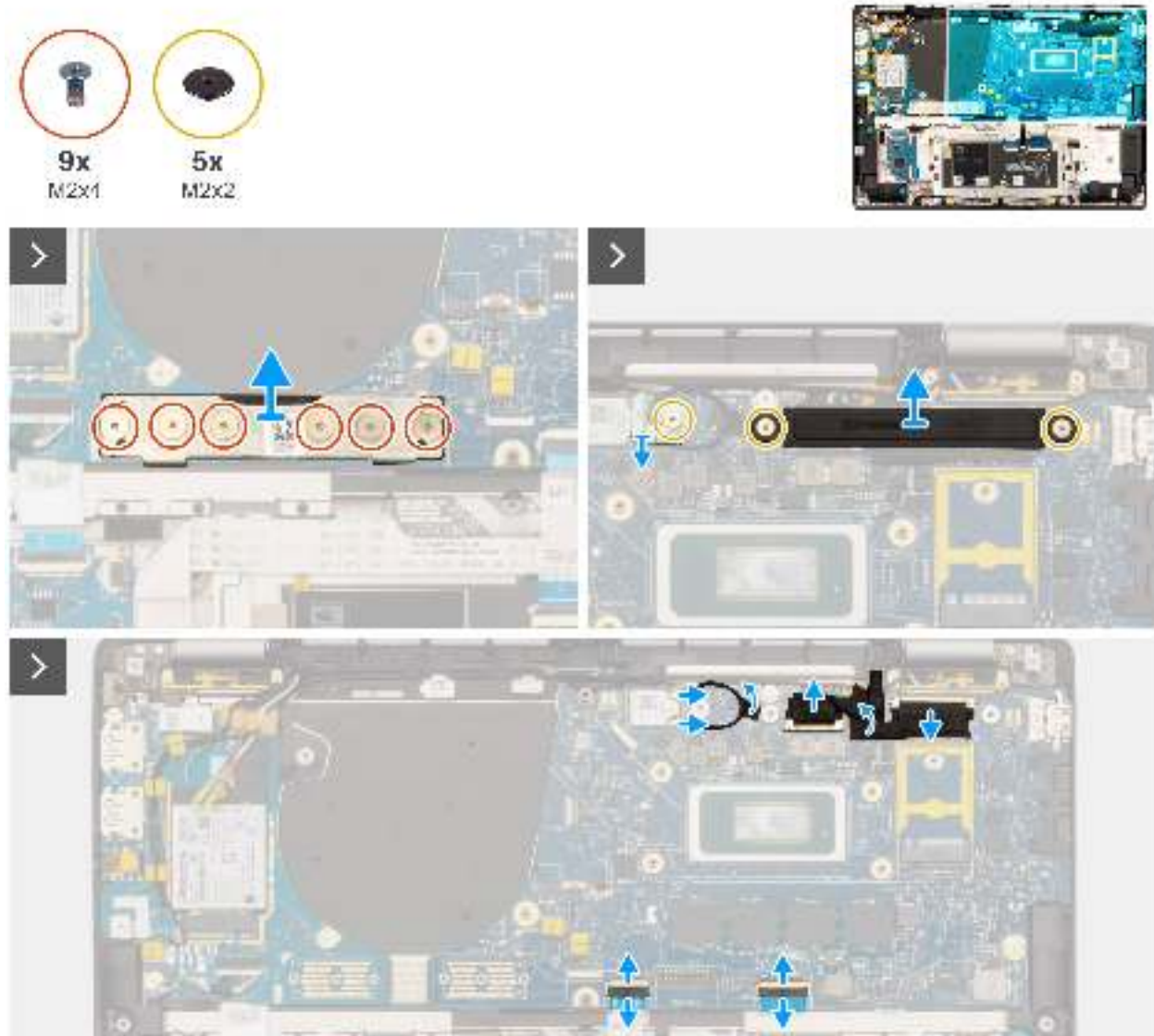
Abbildung 59. Entfernen der Hauptplatine
