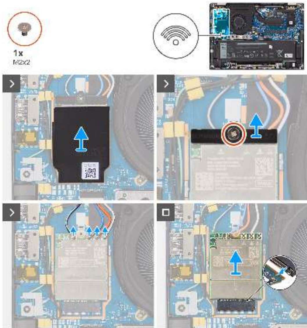
Abbildung 26. Entfernen der 5G-WWAN-Karte
