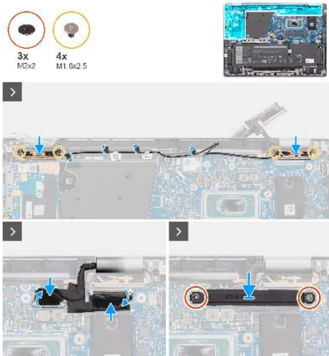
Abbildung 68. Installieren des WLAN-Antennenmoduls
