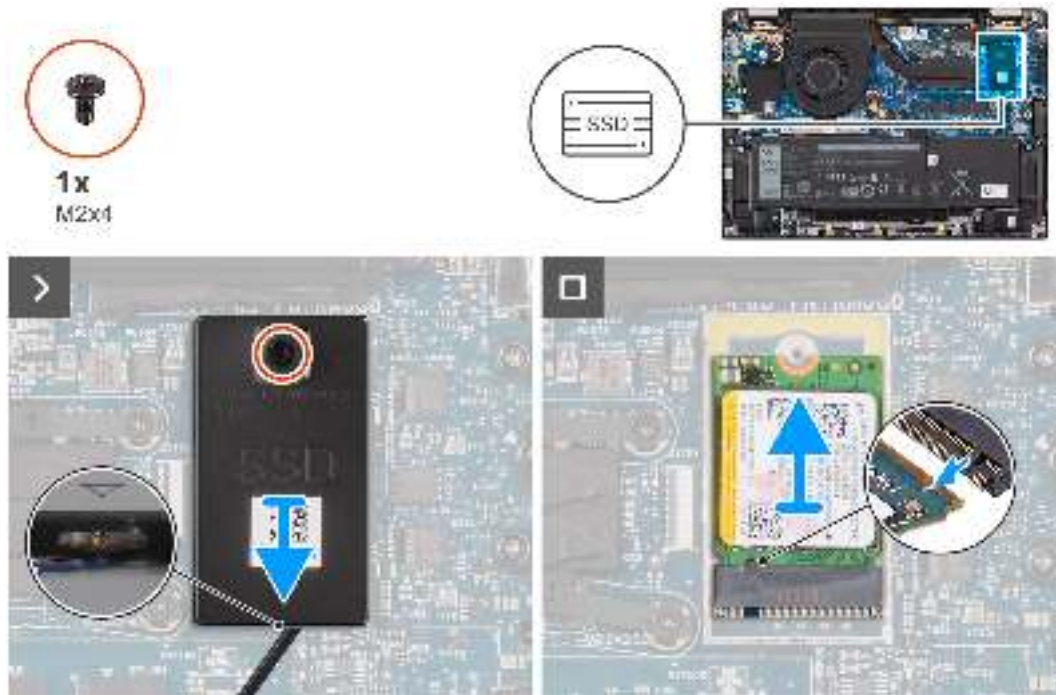
Abbildung 22. Entfernen des M.2-2230-Solid-State-Laufwerks
