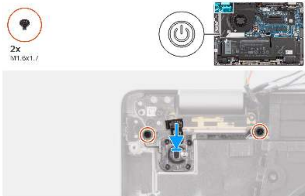
Abbildung 77. Installieren des Netzschalters mit optionalem Fingerabdruck-Lesegerät
