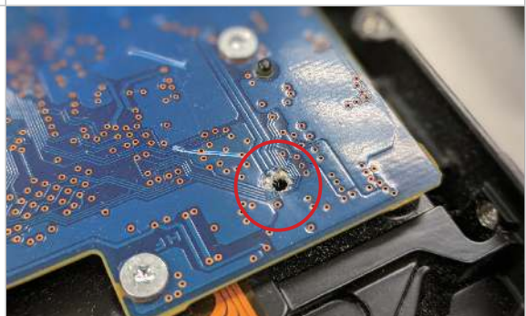
Beschädigte Leiterplatte
