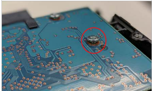
Gelockerte Schrauben
