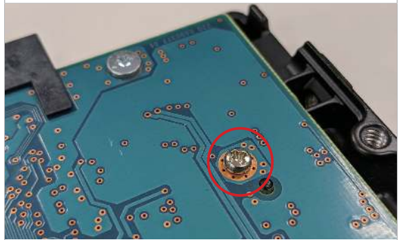
Falsche Schraube befestigt
