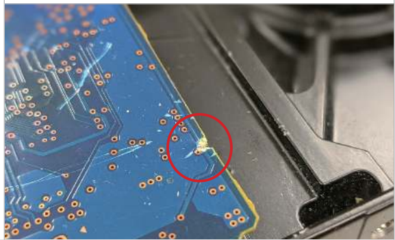
Starke Dellen auf Leiterplatte
