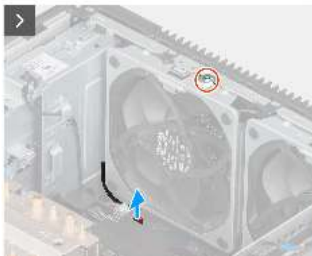
Abbildung 45. Vorderer Lüfter 1
