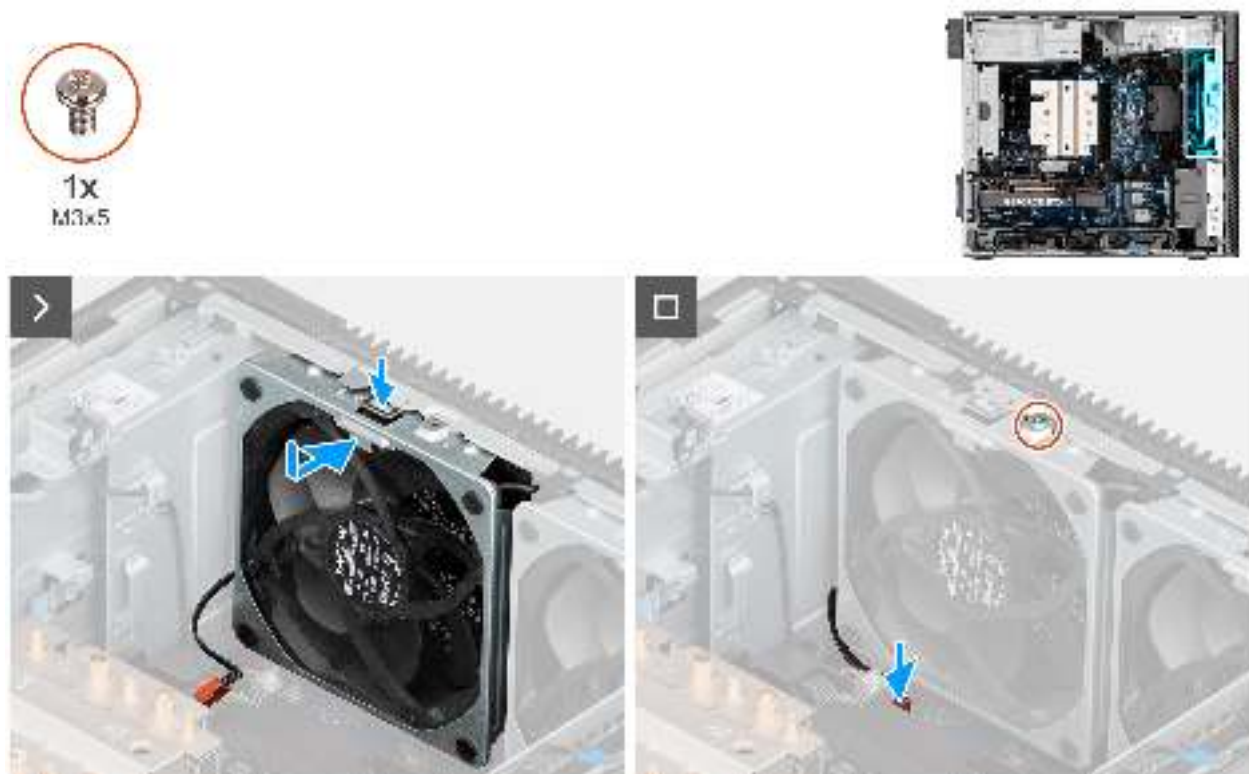
Abbildung 47. Vorderer Lüfter 1
