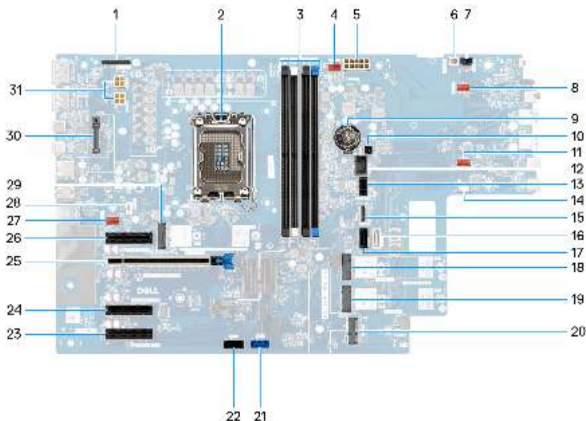
Abbildung 93. Systemplattenbeschriftung
