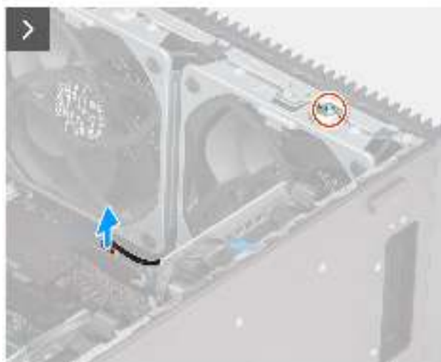
Abbildung 46. Vorderer Lüfter 2
