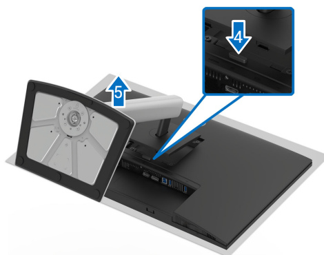
Abbildung 24. Monitorständer abnehmen
