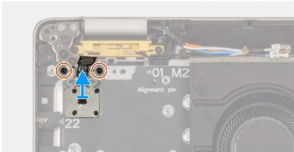
Abbildung 53. Installieren des Netzschalters mit optionalem Fingerabdruck-Lesegerät
