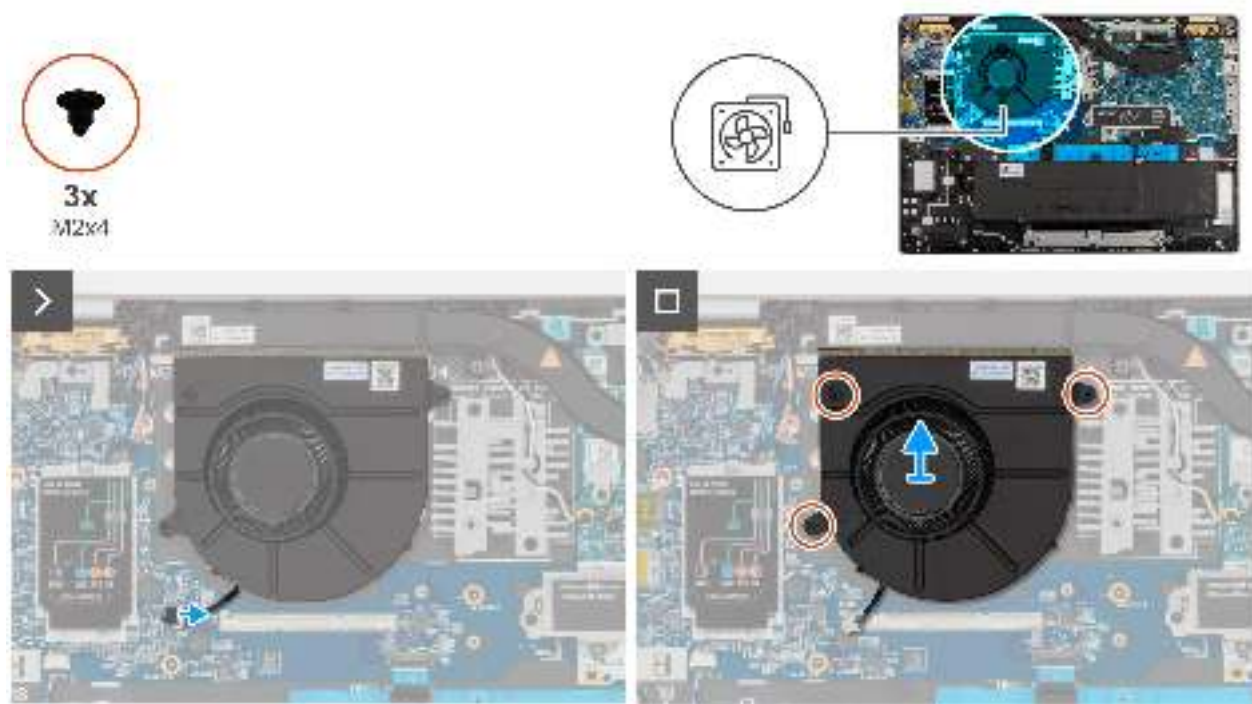
Abbildung 28. Entfernen des Lüfters
