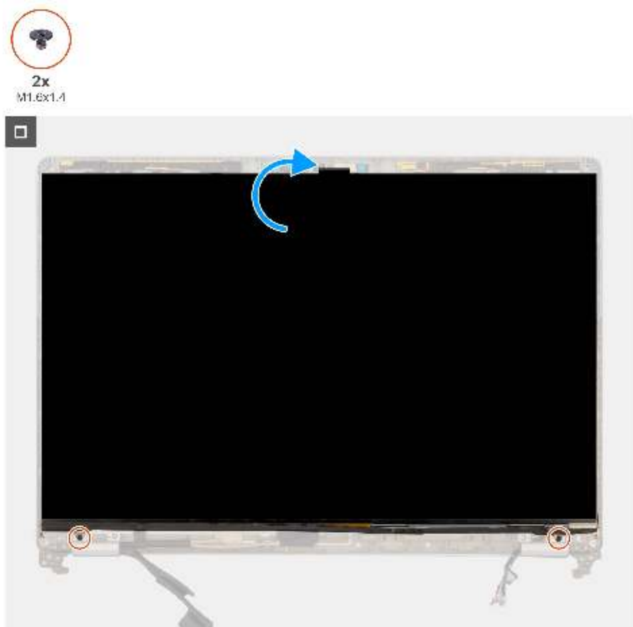
Abbildung 68. Einbauen des Bildschirms
