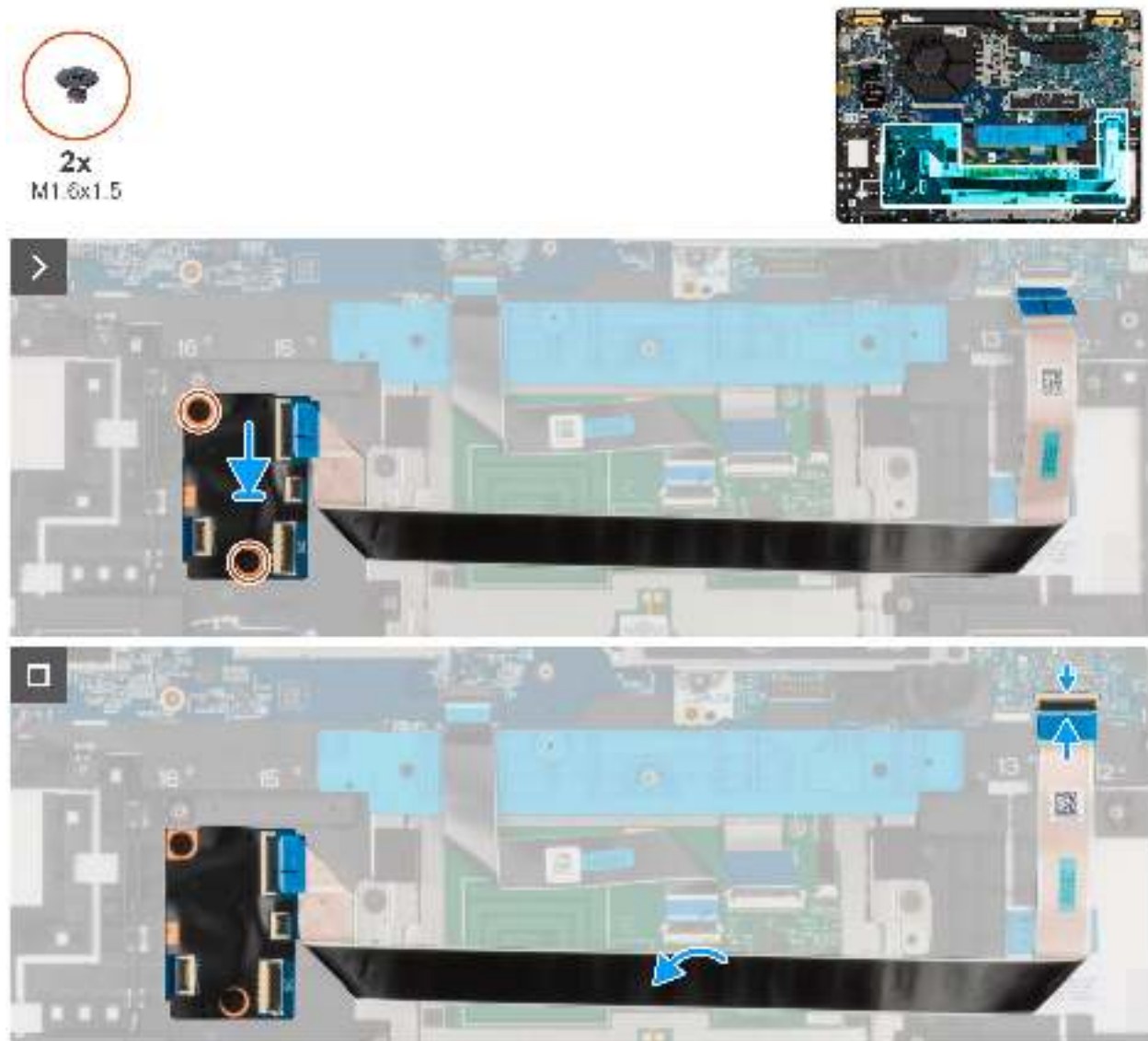
Abbildung 42. USH-Platine
