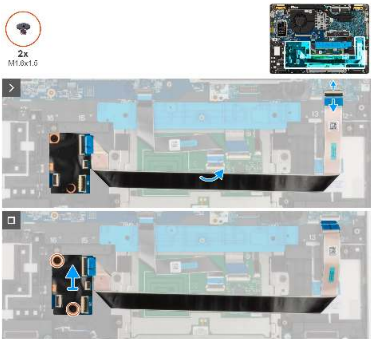
Abbildung 41. Entfernen der USH-Platine
