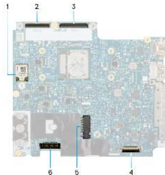
Abbildung 49. Anschlüsse auf der Hauptplatine
