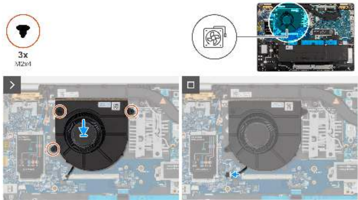
Abbildung 29. Einbauen des Lüfters
