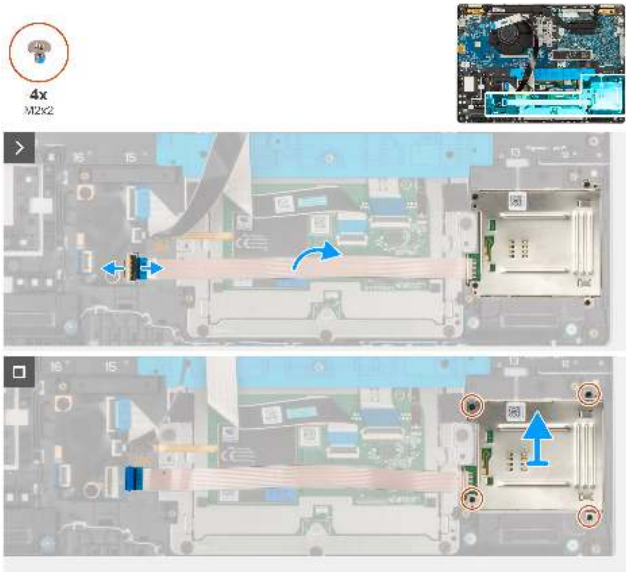
Abbildung 43. Entfernen des
