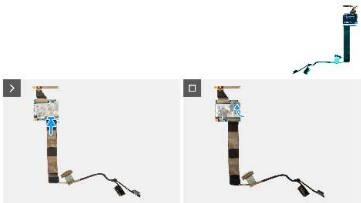
Abbildung 72. Einbauen des Bildschirmkabels
