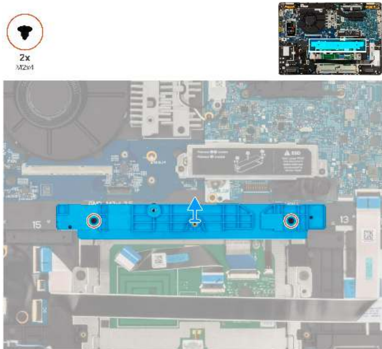
Abbildung 39. Akkuhalterung
