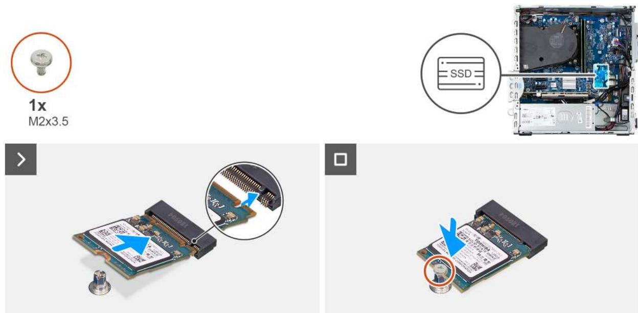
Abbildung 23. Installieren des M.2 2230-Solid-State-Laufwerks
