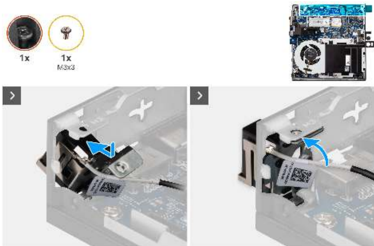
Abbildung 68. Einbauen des Antennenmoduls (weißes Kabel)
