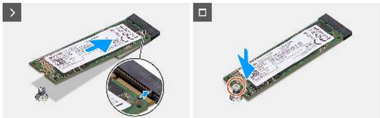
Abbildung 21. Einbauen des M.2-2280-Solid-State-Laufwerks
