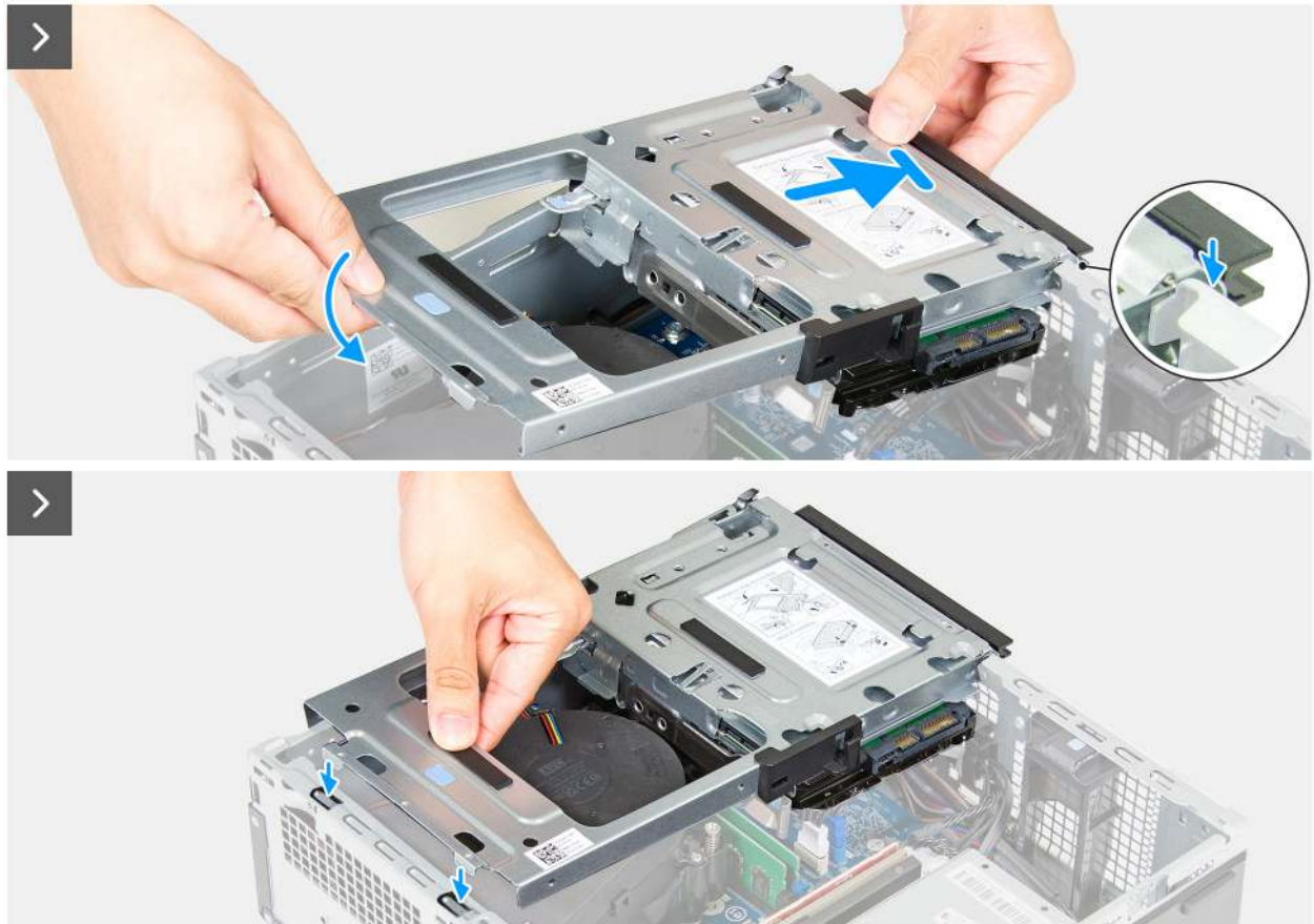
Abbildung 37. Installieren des Laufwerksschachts
