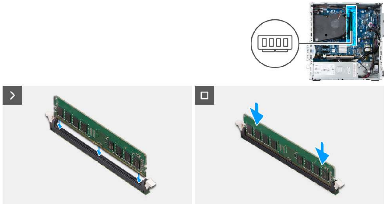
Abbildung 21. Einsetzen des Speichermoduls
