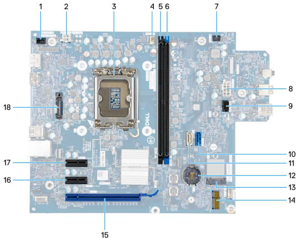
Abbildung 66. Übersicht über die Systemplatine
