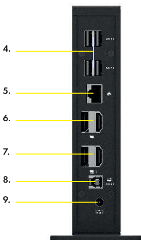
Rückansicht
