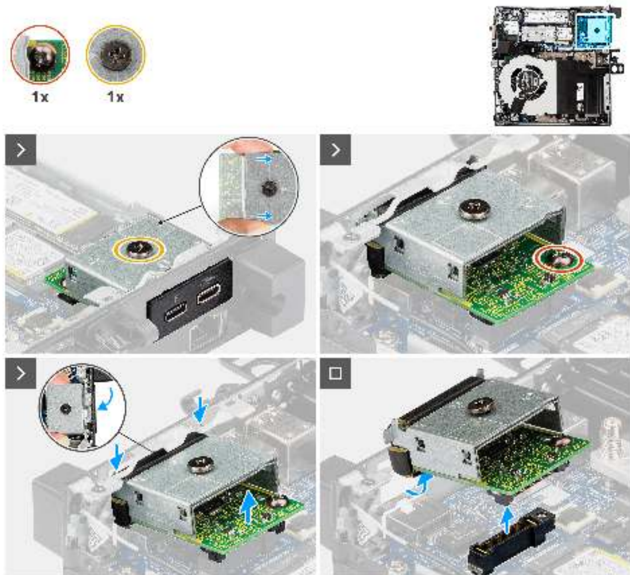
Abbildung 44. Entfernen des Thunderbolt-Ports und USB-Typ-C-Anschlussmoduls
