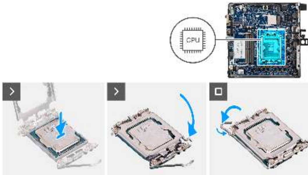
Abbildung 77. Einbauen des Prozessors
