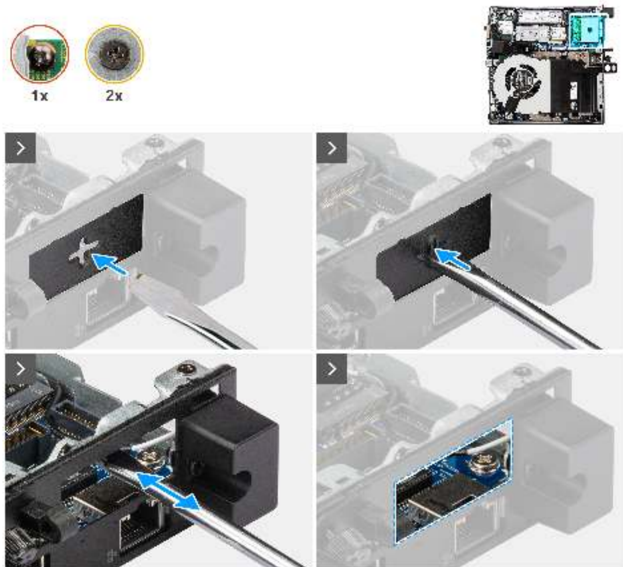
Abbildung 63. Installieren des Glasfasermoduls
