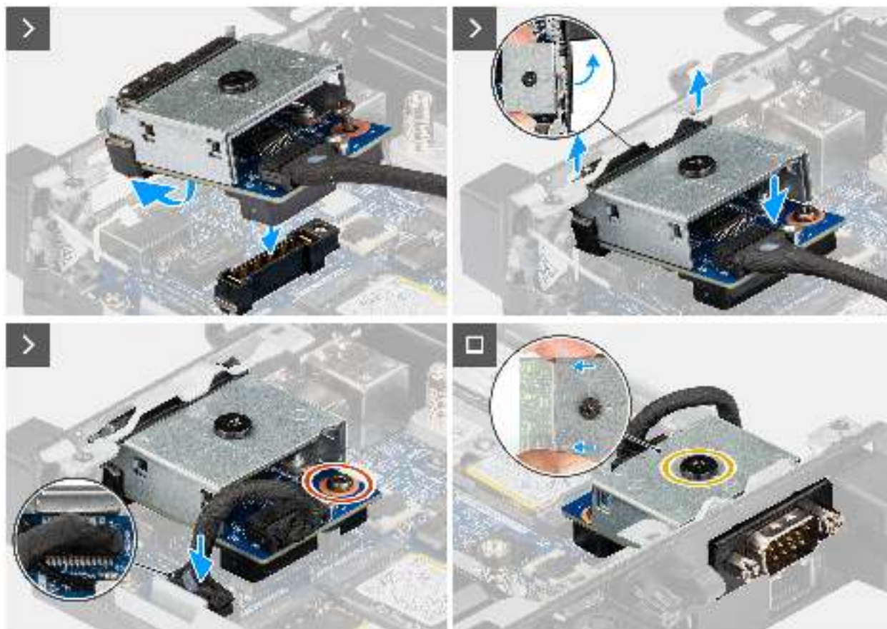
Abbildung 61. Installieren des seriellen Anschlussmoduls
