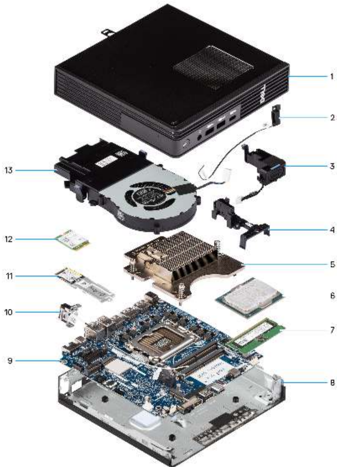
Abbildung 9. Hauptkomponenten des Dell Pro Micro Plus, QBM1250
