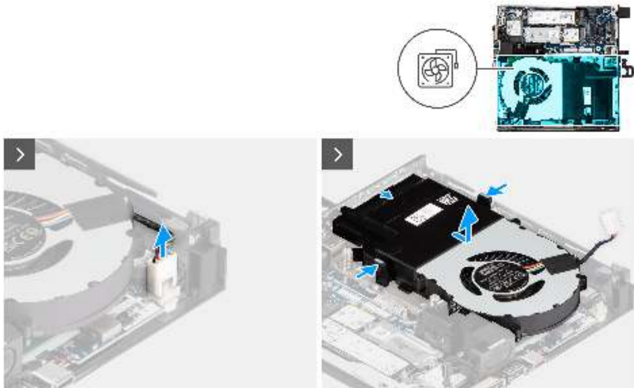
Abbildung 28. Entfernen des Lüfters
