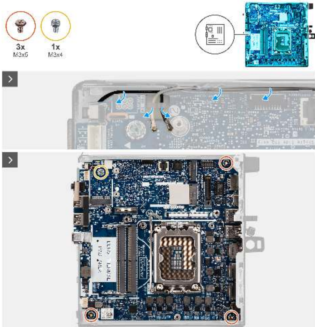
Abbildung 81. Entfernen der Systemplatine
