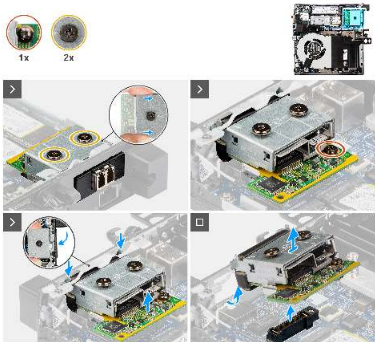
Abbildung 62. Entfernen des Glasfasermoduls
