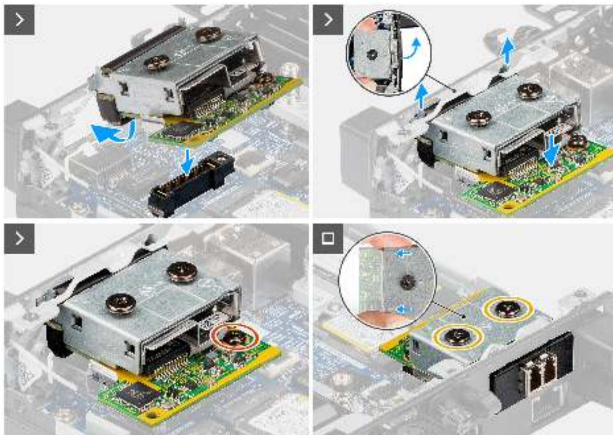
Abbildung 64. Installieren des Glasfasermoduls
