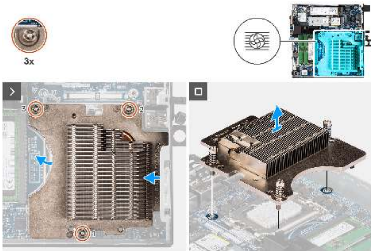
Abbildung 68. Kühlkörper entfernen
