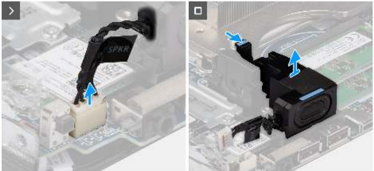
Abbildung 14. Entfernen des Lautsprechers
