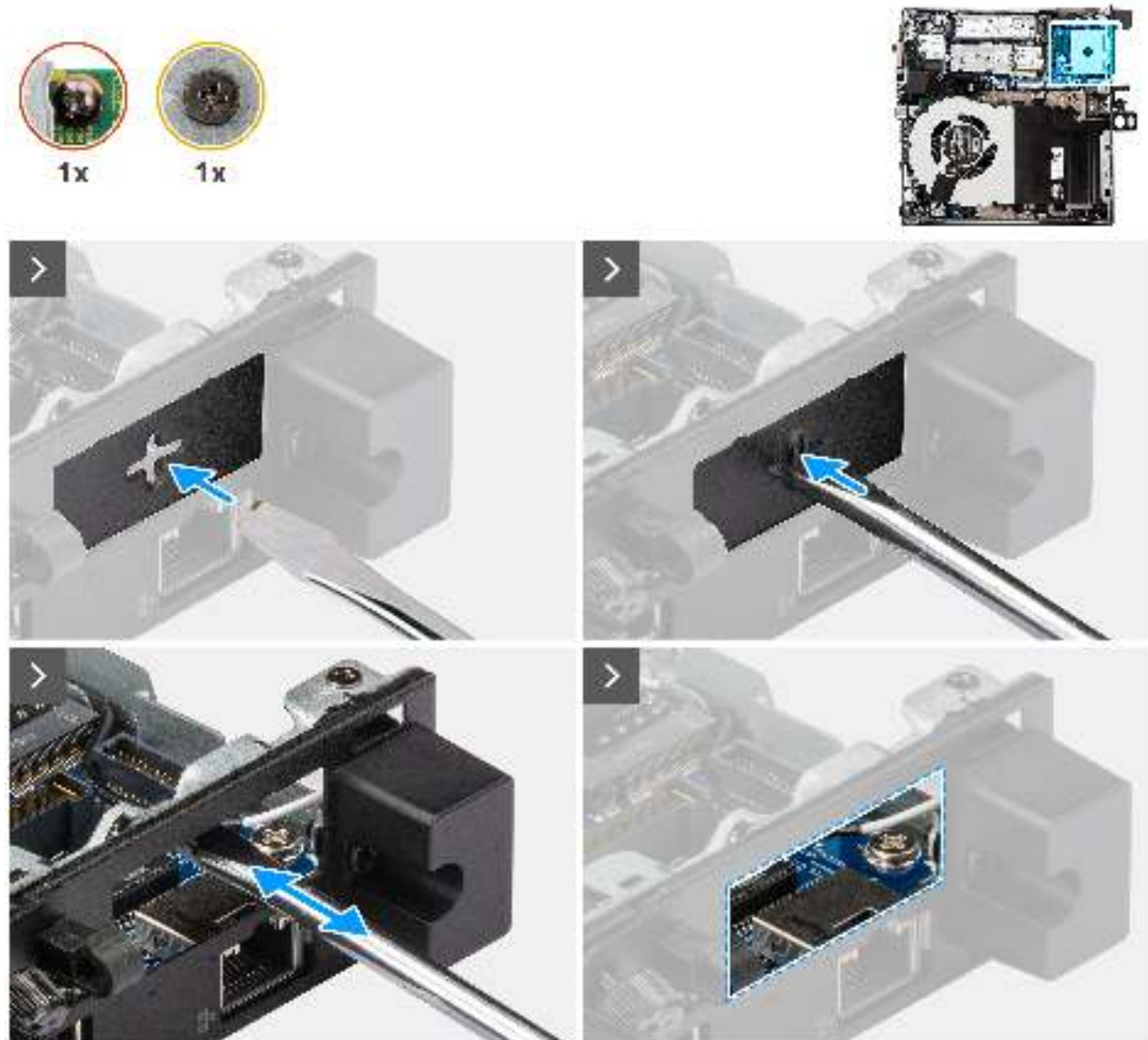
Abbildung 45. Installieren des Thunderbolt Port und USB-Typ-C-Anschlussmoduls
