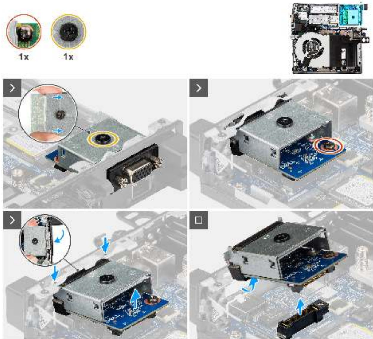
Abbildung 53. Entfernen des VGA-Anschlussmoduls
