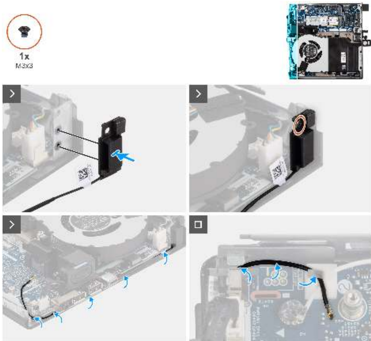
Abbildung 71. Einbauen des Antennenmoduls (schwarzes Kabel)
