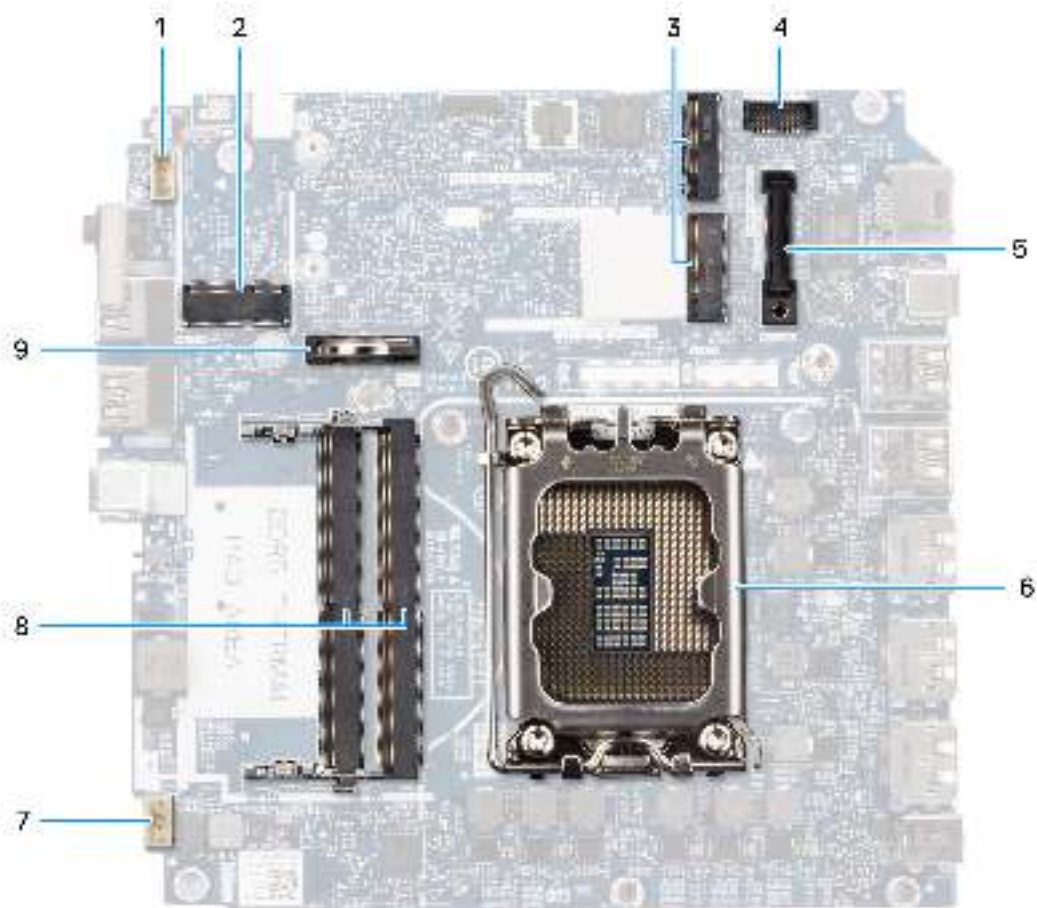
Abbildung 80. Anschlüsse auf der Hauptplatine
