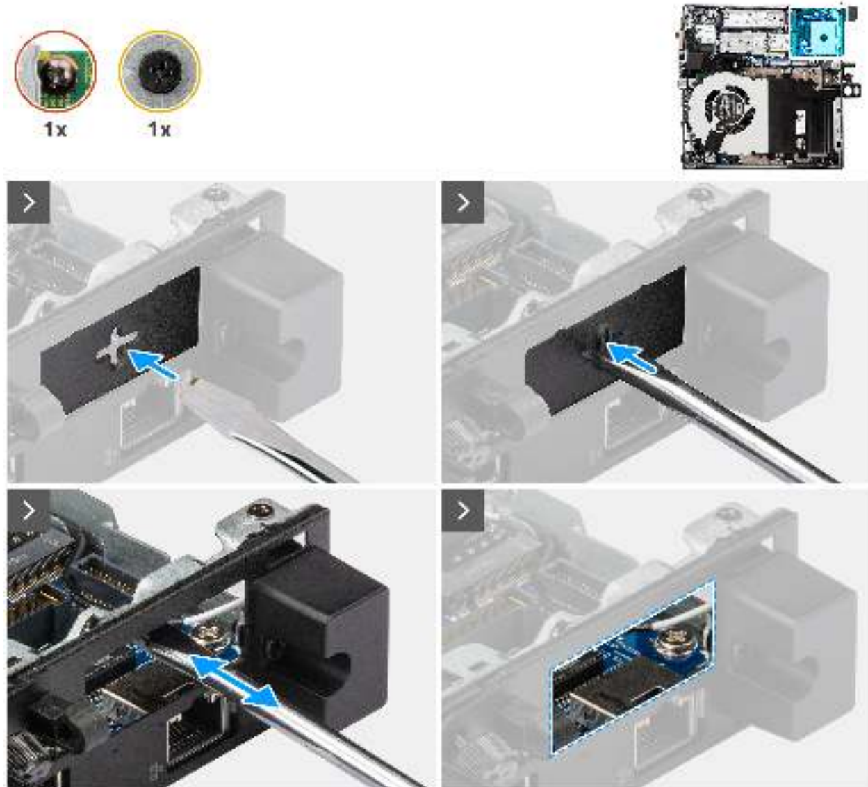
Abbildung 60. Installieren des seriellen Anschlussmoduls
