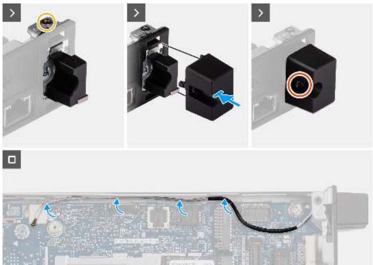
Abbildung 75. Einbauen des Antennenmoduls (weißes Kabel)
