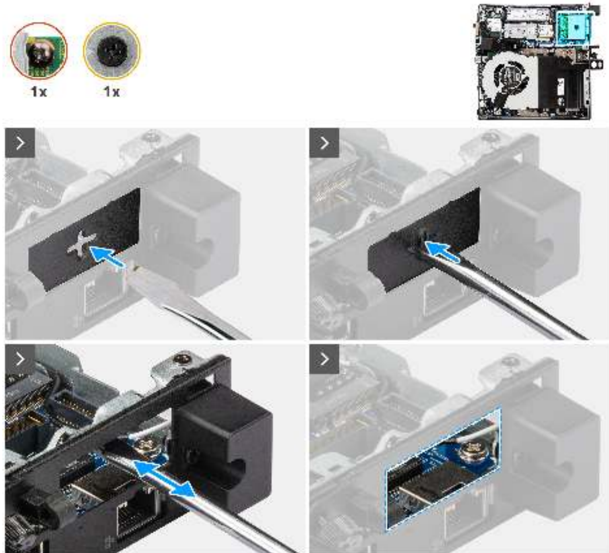
Abbildung 51. Einbauen des HDMI-Anschlussmoduls
