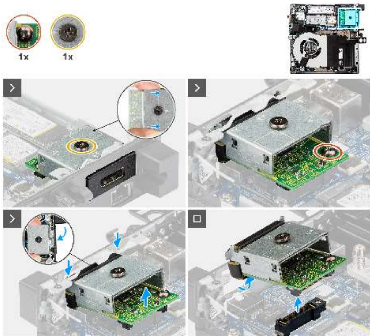
Abbildung 47. Entfernen des DisplayPort-Moduls
