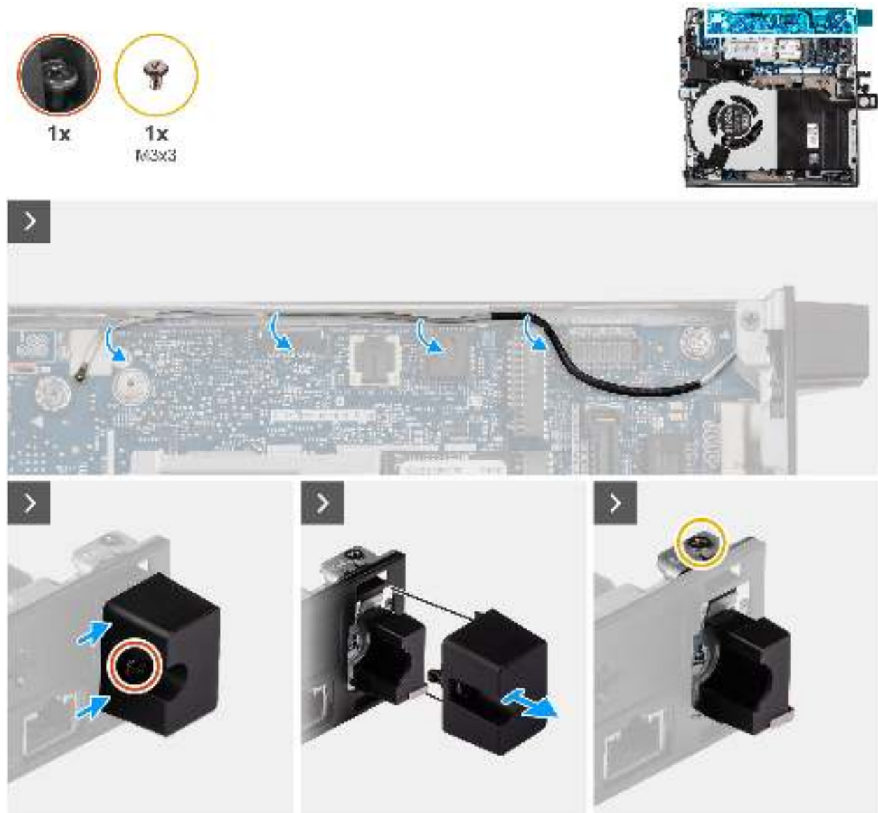
Abbildung 72. Entfernen des Antennenmoduls (weißes Kabel)
