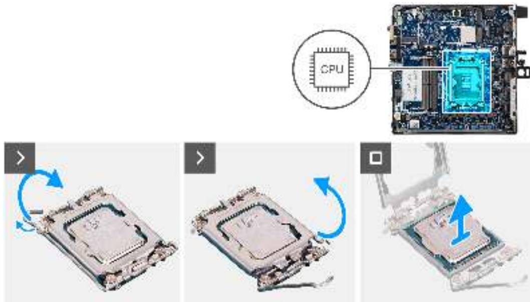
Abbildung 76. Entfernen des Prozessors
