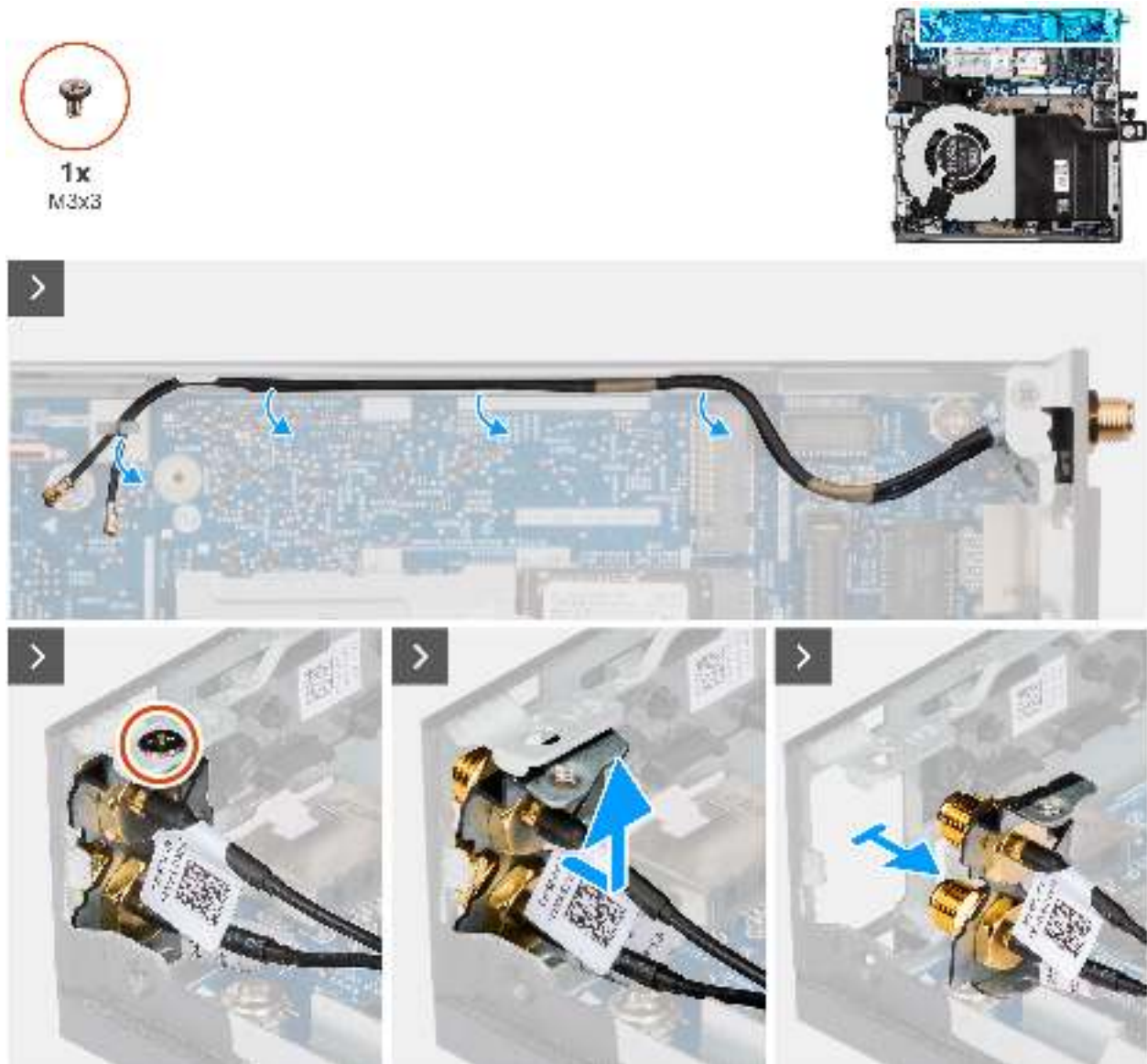
Abbildung 36. Entfernen der SMA-Antenne
