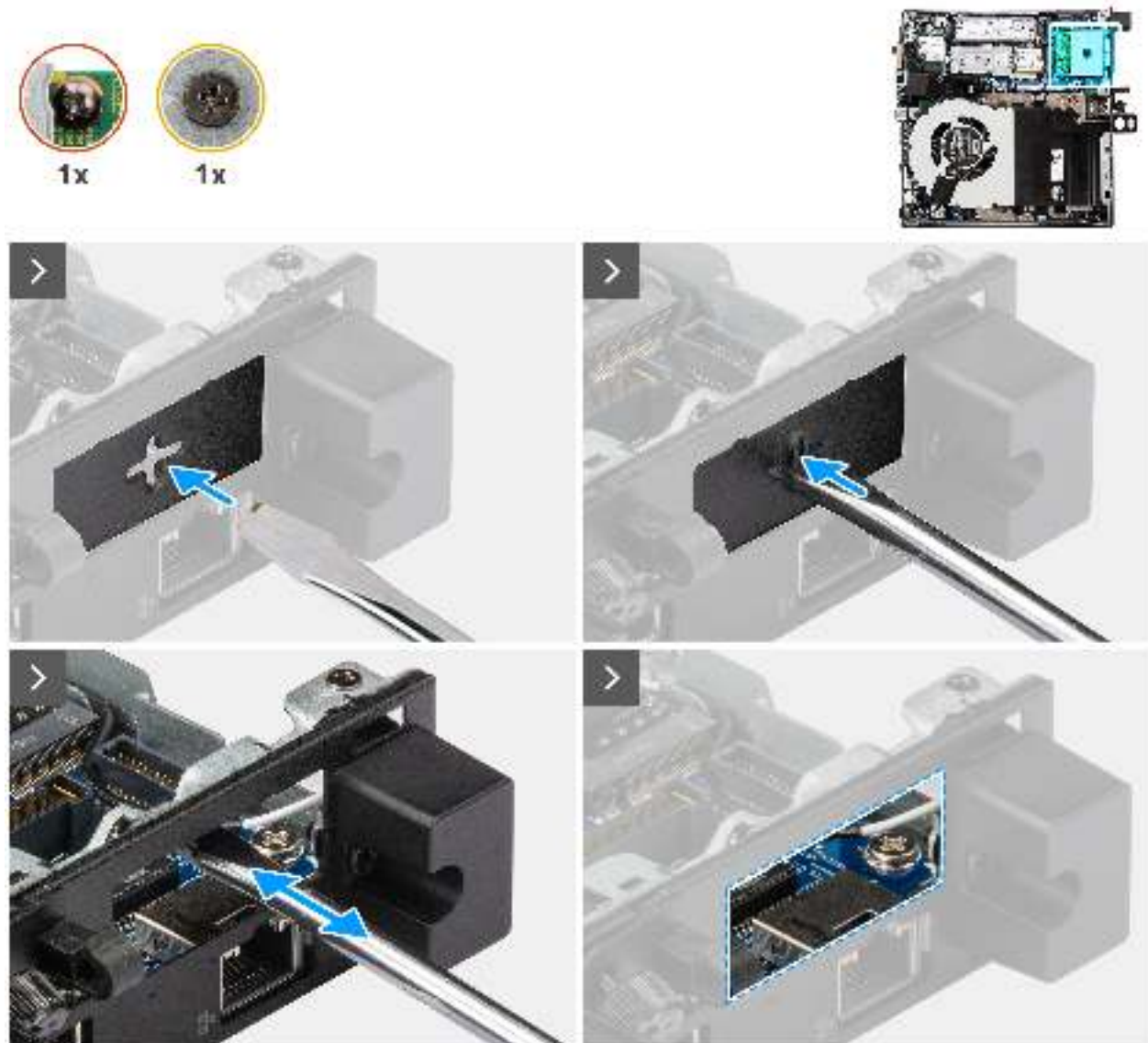
Abbildung 48. Einbauen des DisplayPort-Moduls
