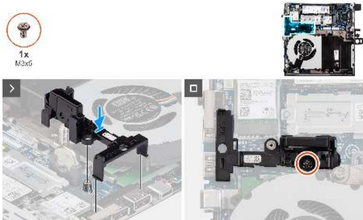
Abbildung 79. Installieren der Lautsprecherhalterung
