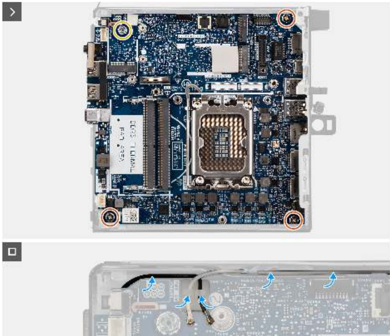
Abbildung 85. Einbauen der Systemplatine
