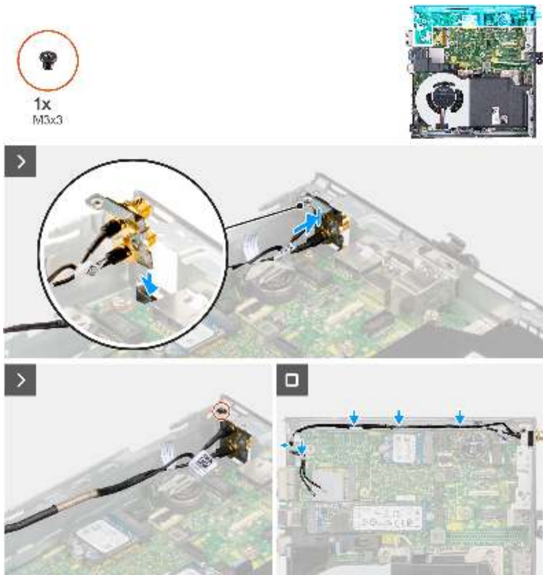
Abbildung 37. Installieren des SMA-Antennenmoduls
