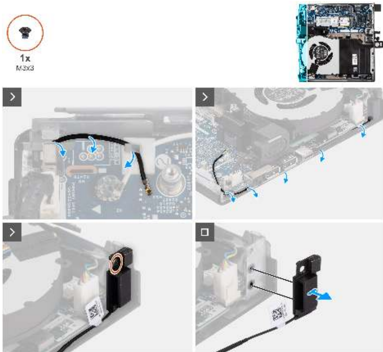
Abbildung 70. Entfernen des Antennenmoduls (schwarzes Kabel)
