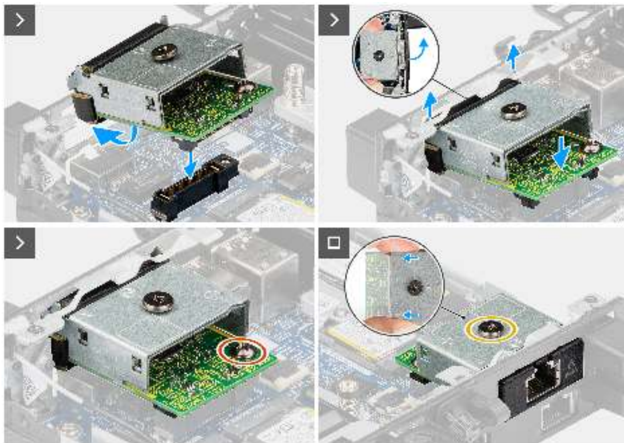
Abbildung 67. Installieren des RJ45-Ethernet-Anschlussmoduls
