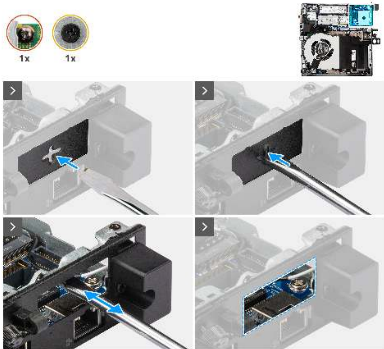
Abbildung 57. Einbauen des PS2-Anschlussmoduls
