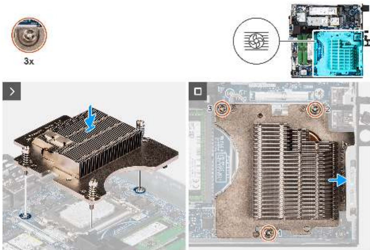
Abbildung 69. Einsetzen des Kühlkörpers
