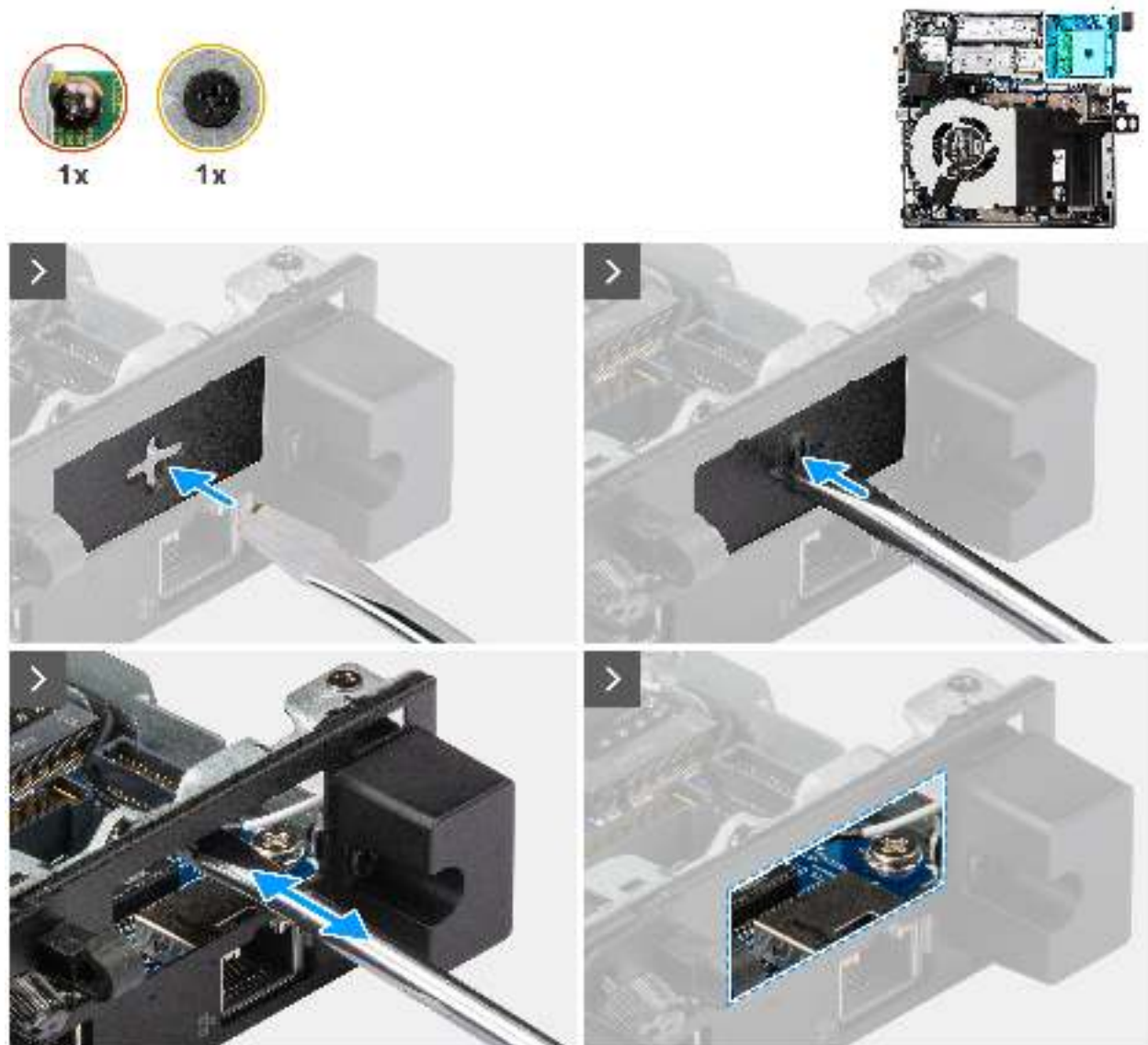
Abbildung 54. Installieren des VGA-Anschlussmoduls
