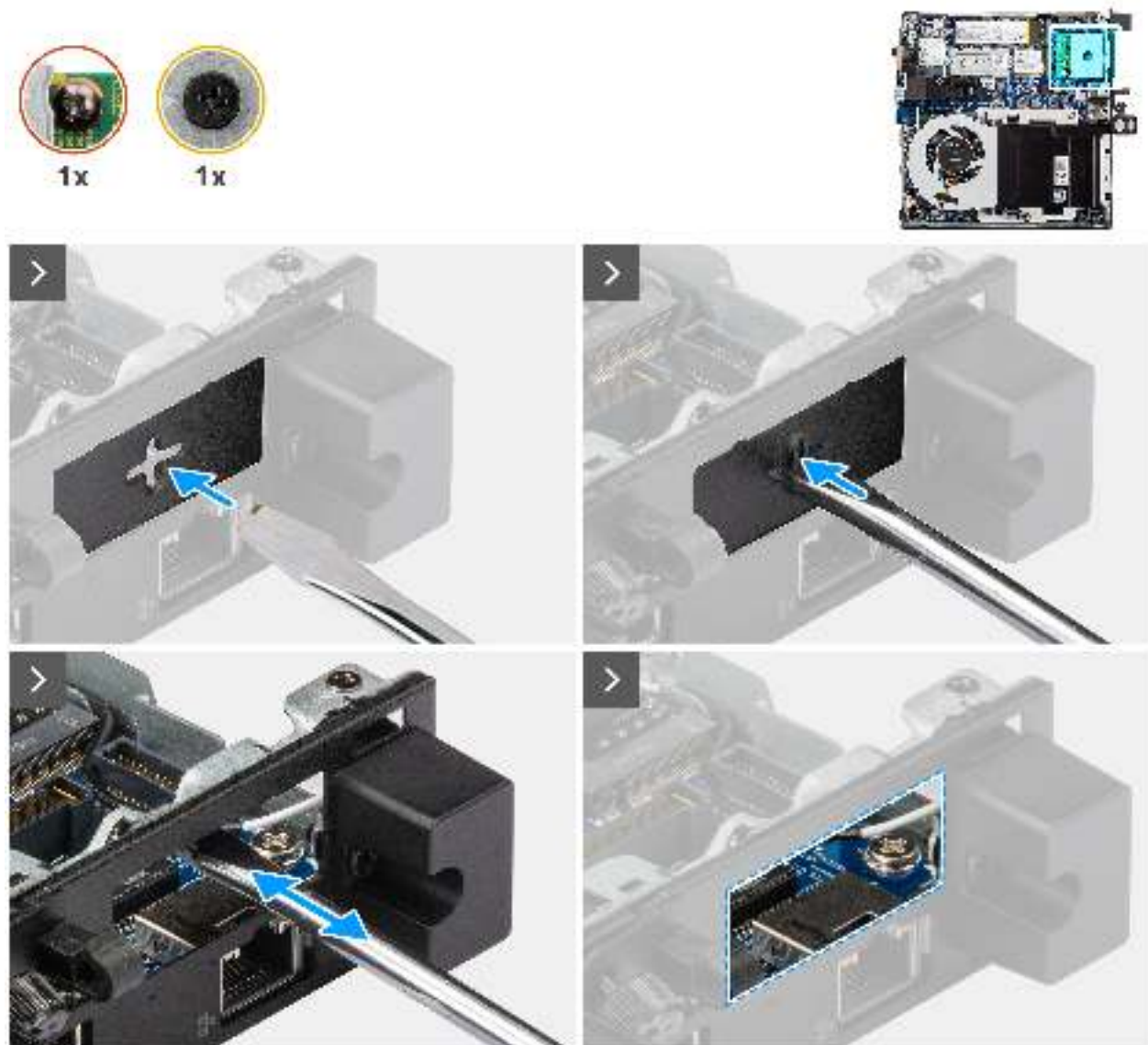
Abbildung 66. Installieren des RJ45-Ethernet-Anschlussmoduls
