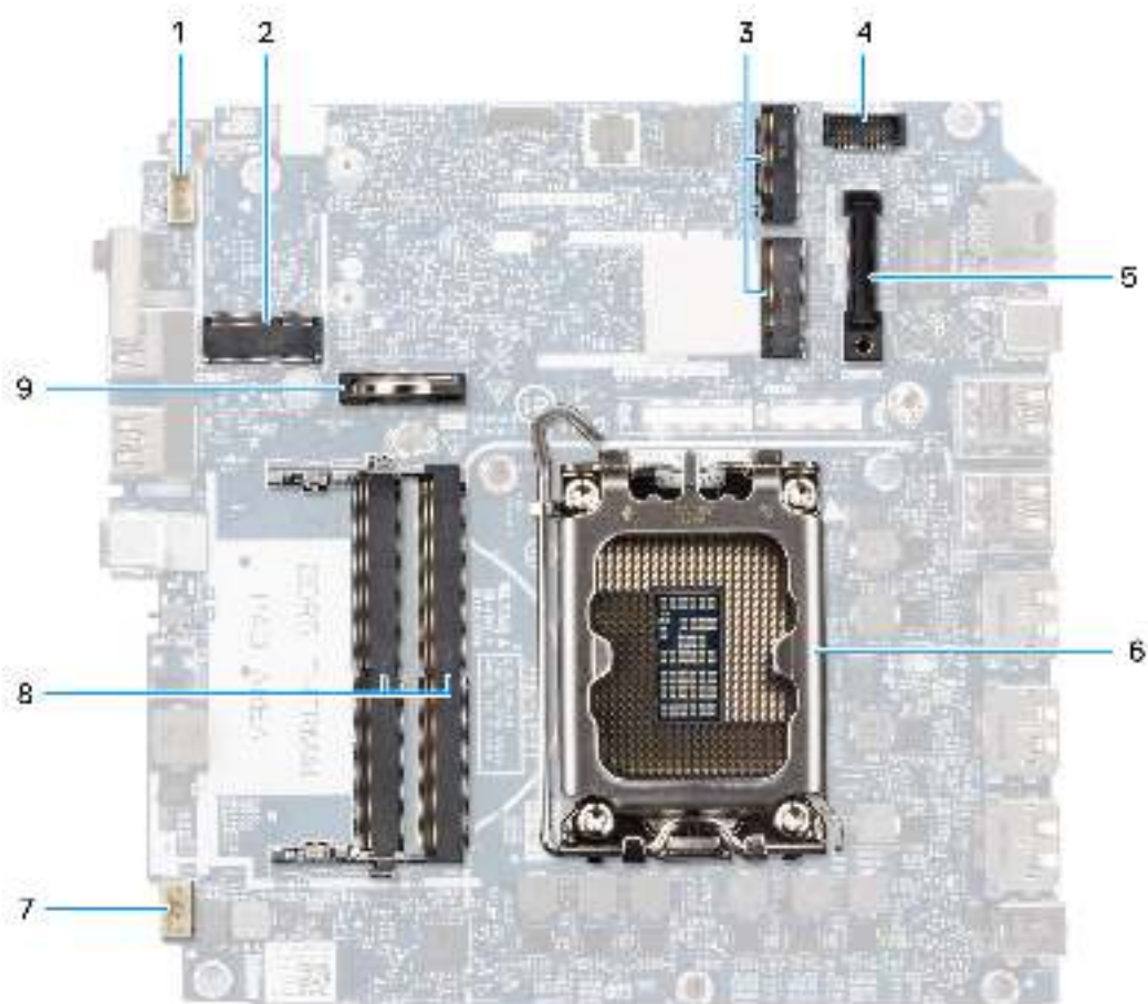
Abbildung 83. Anschlüsse auf der Hauptplatine
