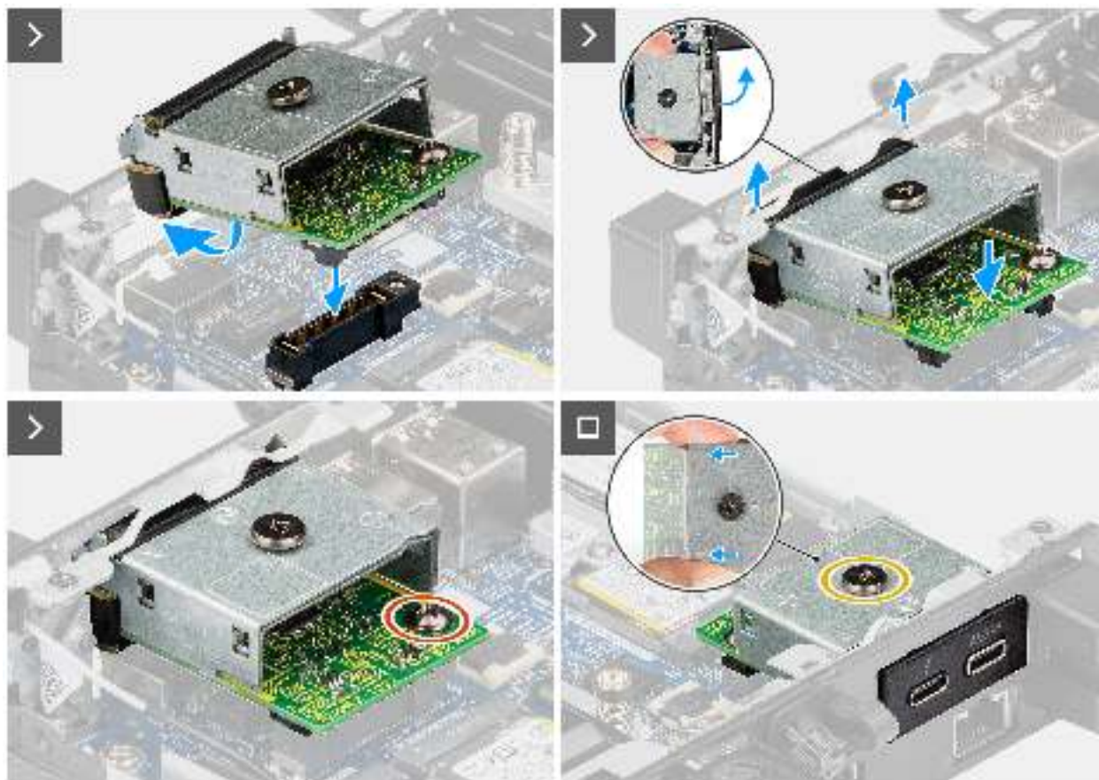
Abbildung 46. Installieren des Thunderbolt Port und USB-Typ-C-Anschlussmoduls
