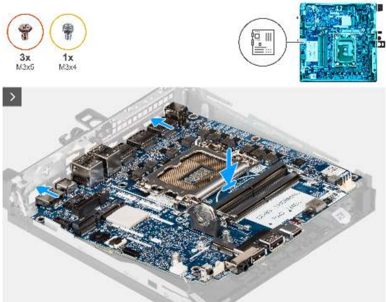
Abbildung 84. Einbauen der Systemplatine
