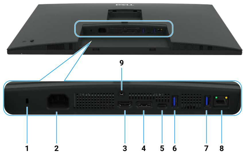
Abbildung 4. Unteransicht des Monitors
