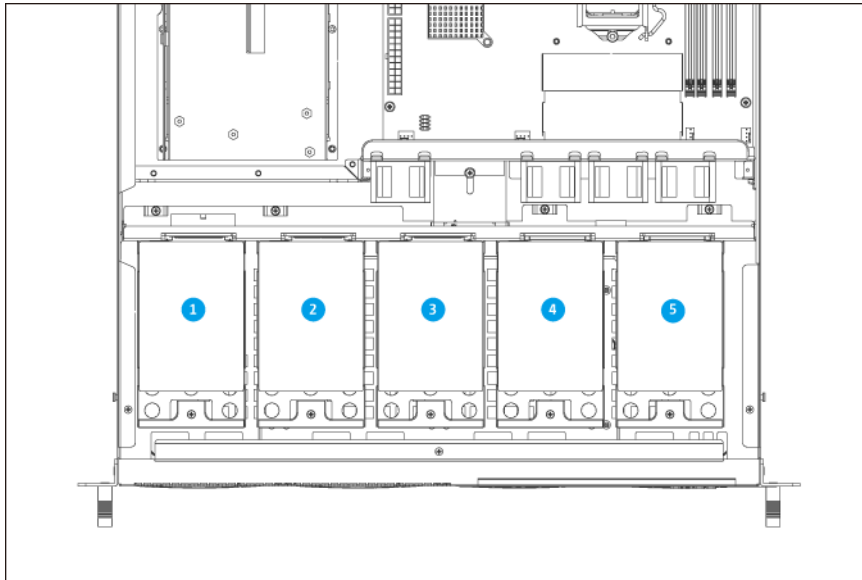
2,5-Zoll Laufwerksschächte
