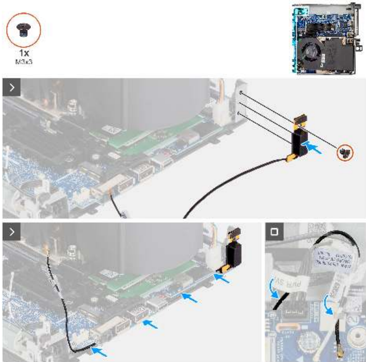
Abbildung 61. Einbauen der internen Antenne – Position 2
