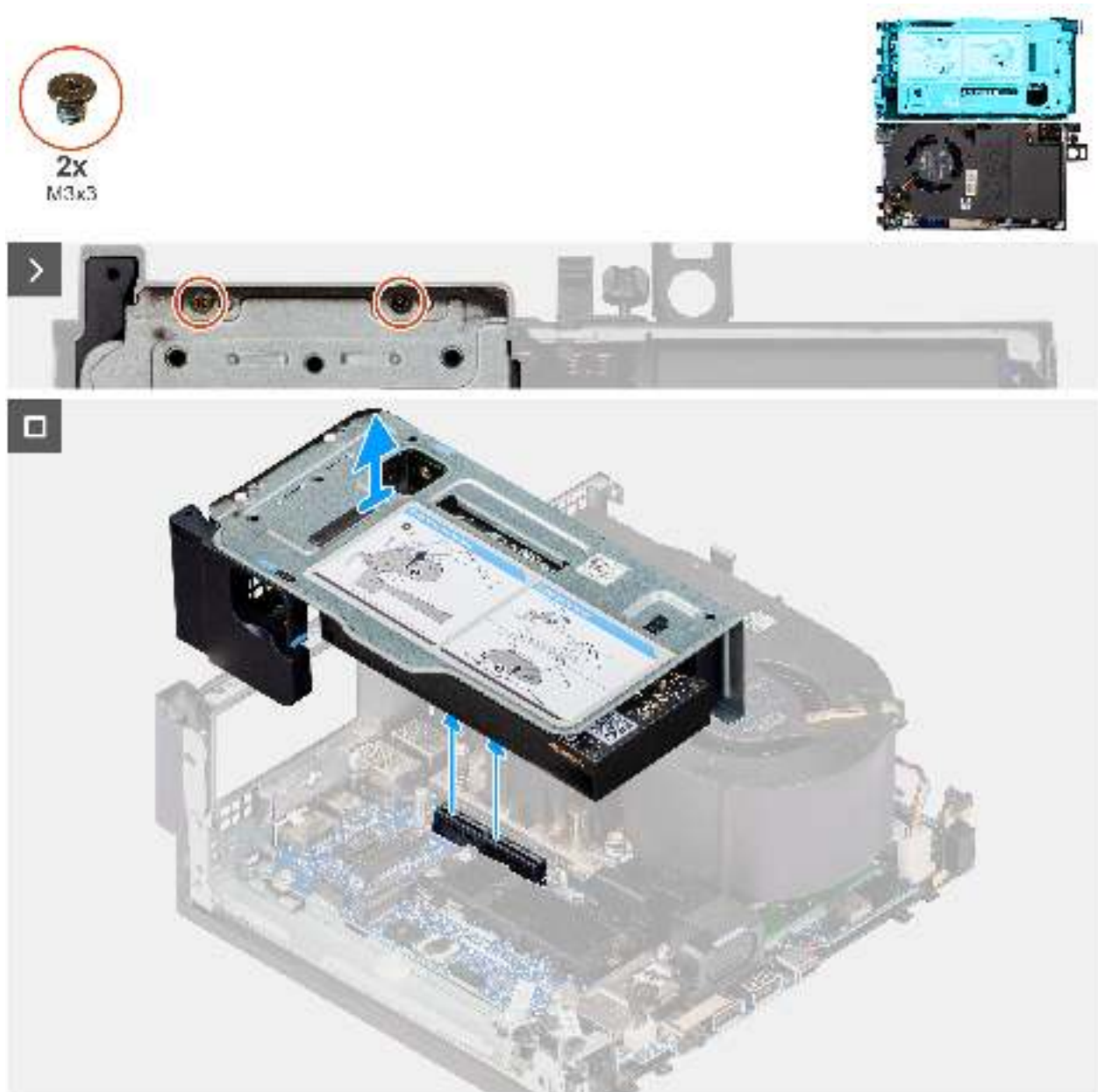
Abbildung 9. Entfernen des Riser-Kartenmoduls
