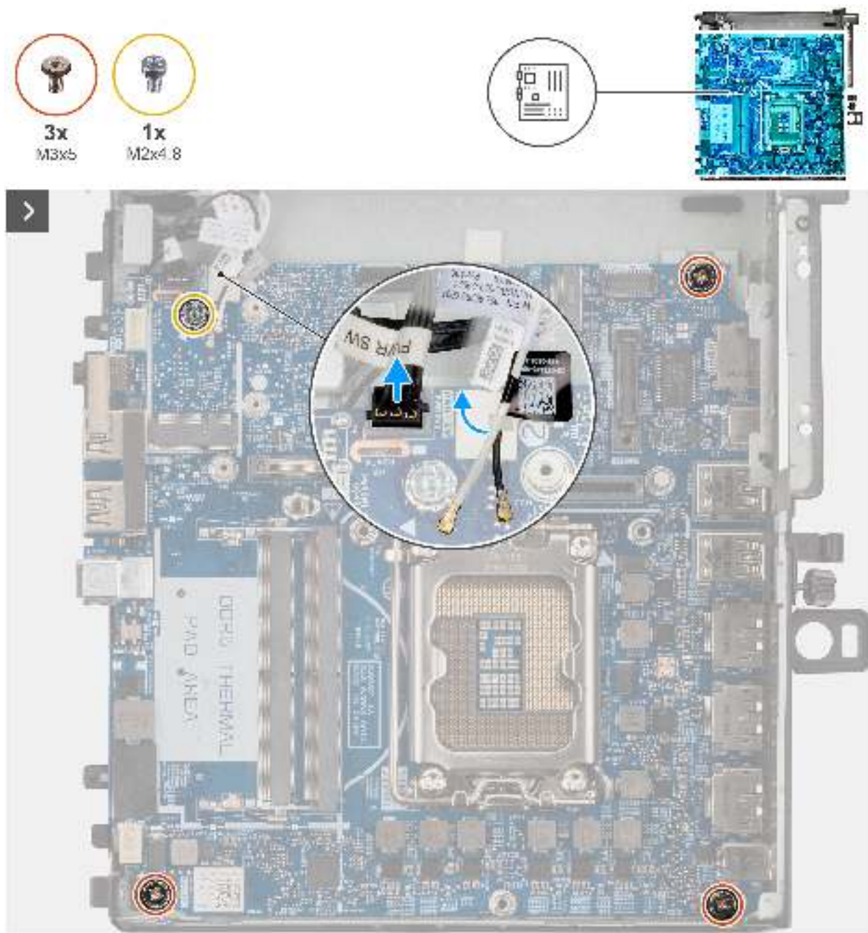
Abbildung 51. Entfernen der Systemplatine
