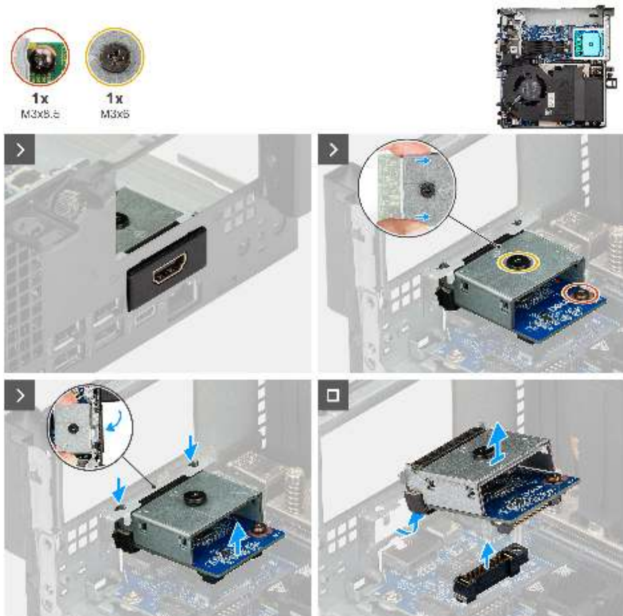
Abbildung 45. Entfernen des HDMI-Anschlusses
