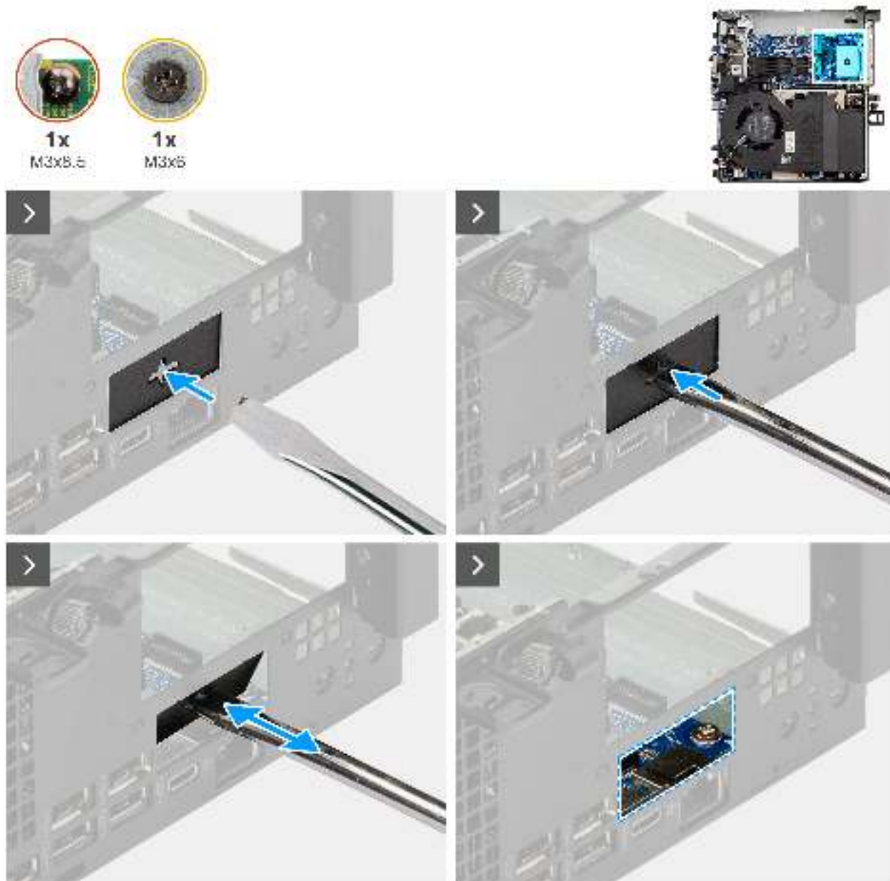
Abbildung 34. Einbauen des PS2-Anschlusses
