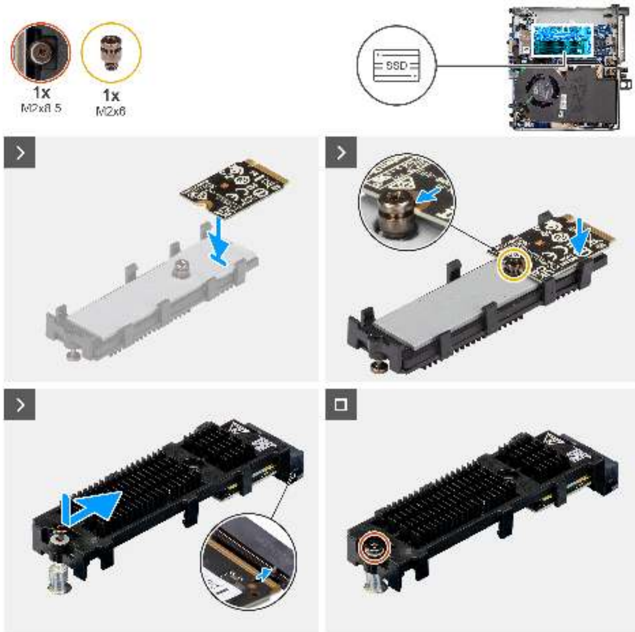
Abbildung 20. Einbauen des M.2-2230-PCle-Solid-State-Laufwerks (Steckplatz 1)
