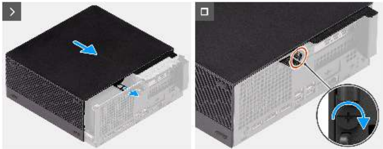
Abbildung 6. Anbringen der Seitenabdeckung
