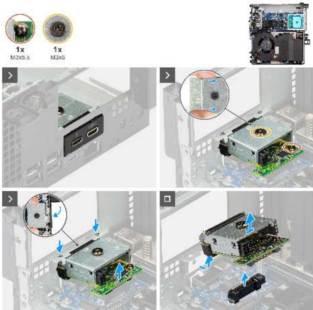
Abbildung 42. Entfernen des Thunderbolt-Anschlusses
