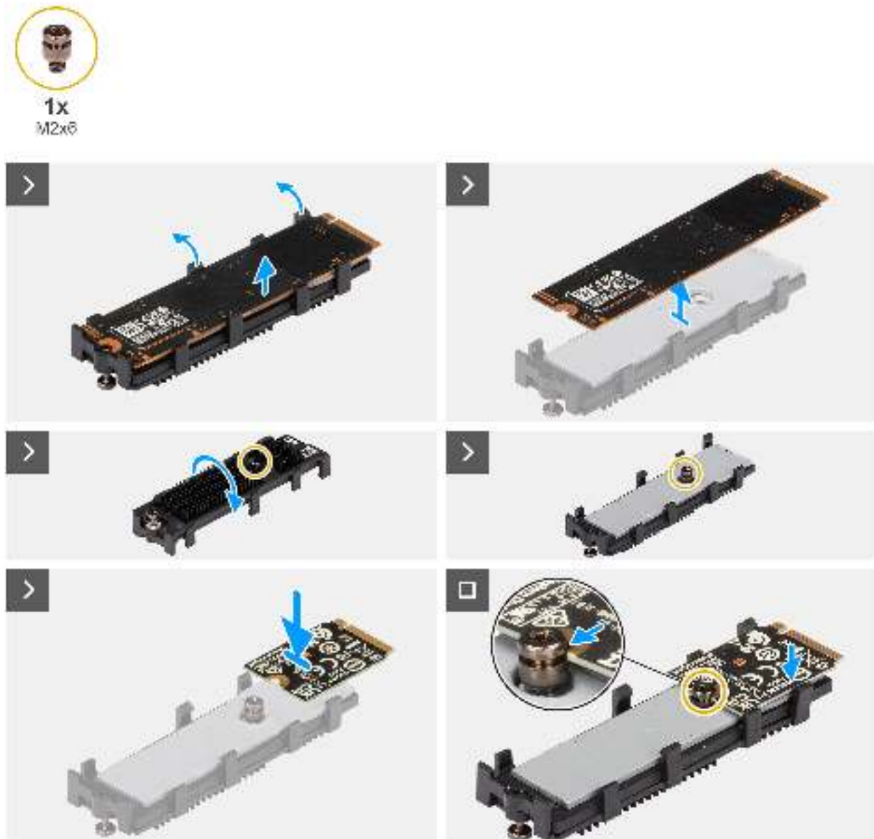
Abbildung 24. Ersetzen der M.2-2280-SSD durch eine M.2-2230-SSD
