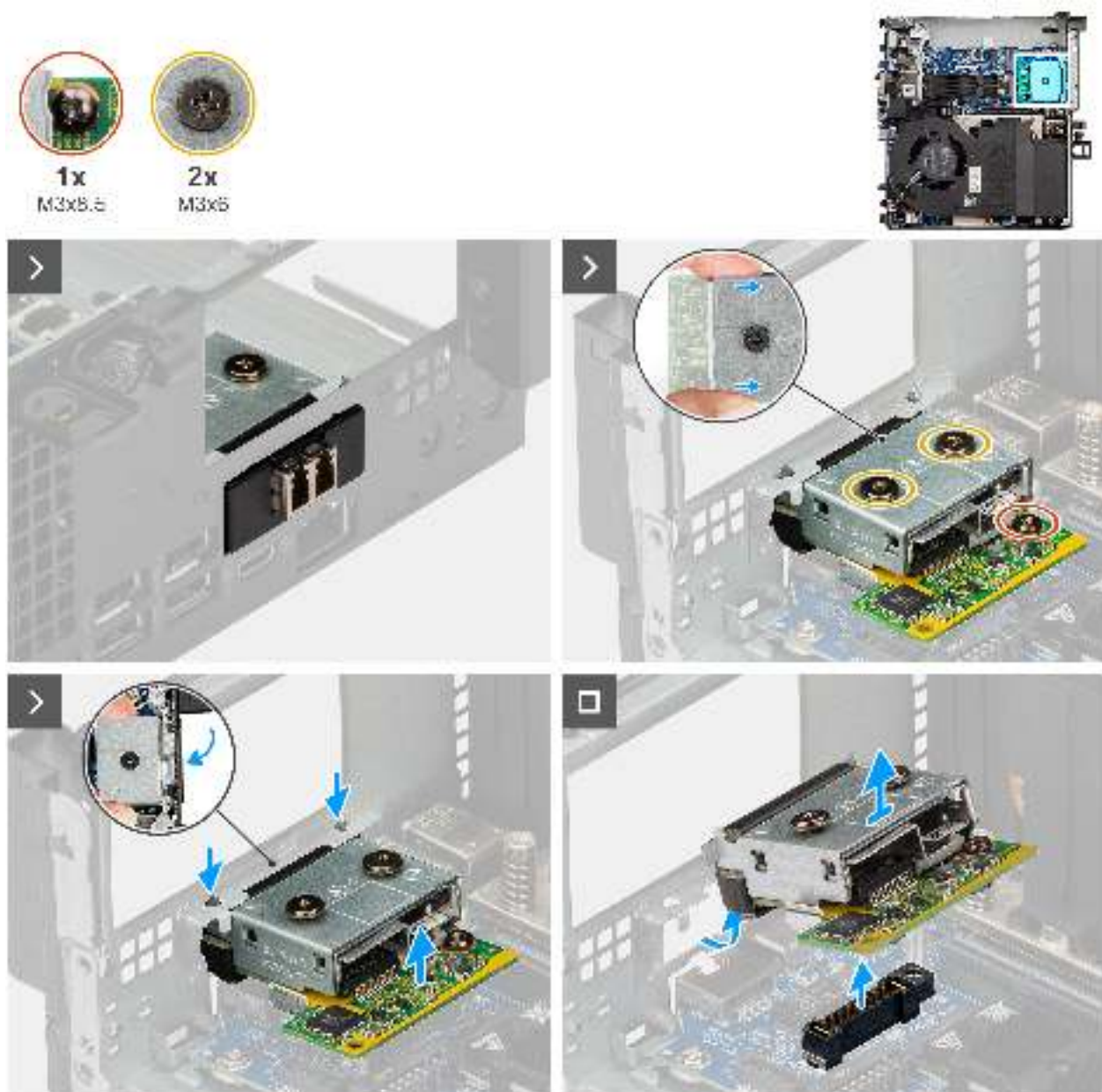
Abbildung 33. Entfernen des optischen 5G-Glasfaseranschlusses
