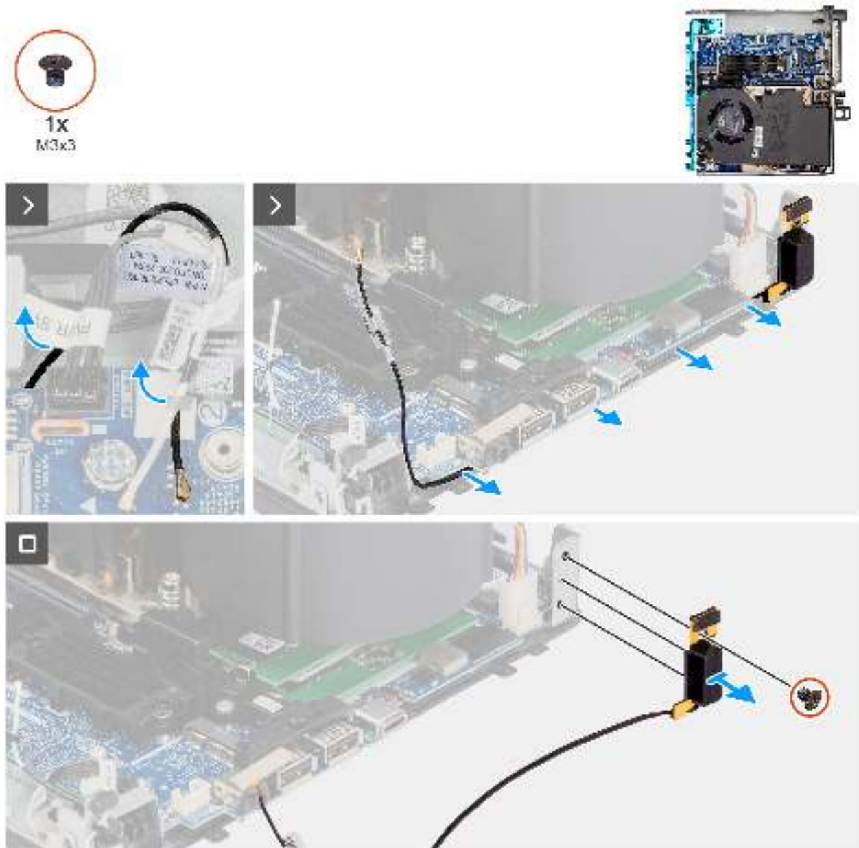
Abbildung 60. Entfernen der internen Antenne – Position 2
