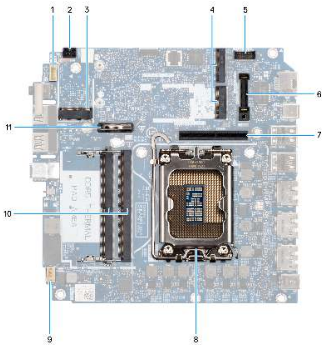
Abbildung 53. Anschlüsse auf der Hauptplatine
