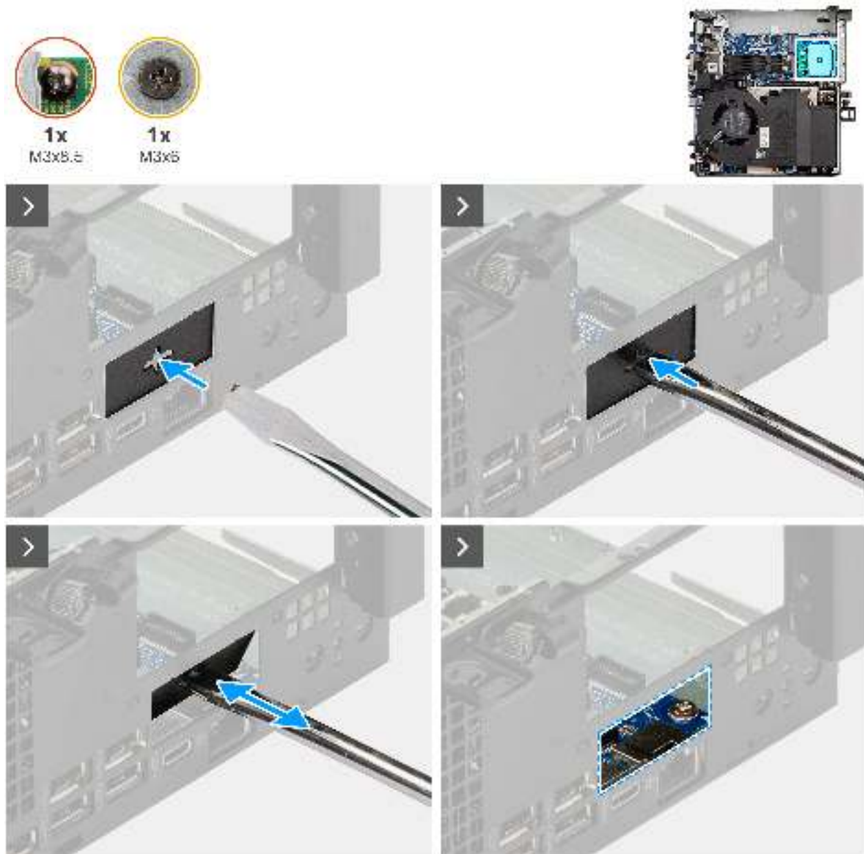
Abbildung 40. Einbauen des Thunderbolt-Anschlusses
