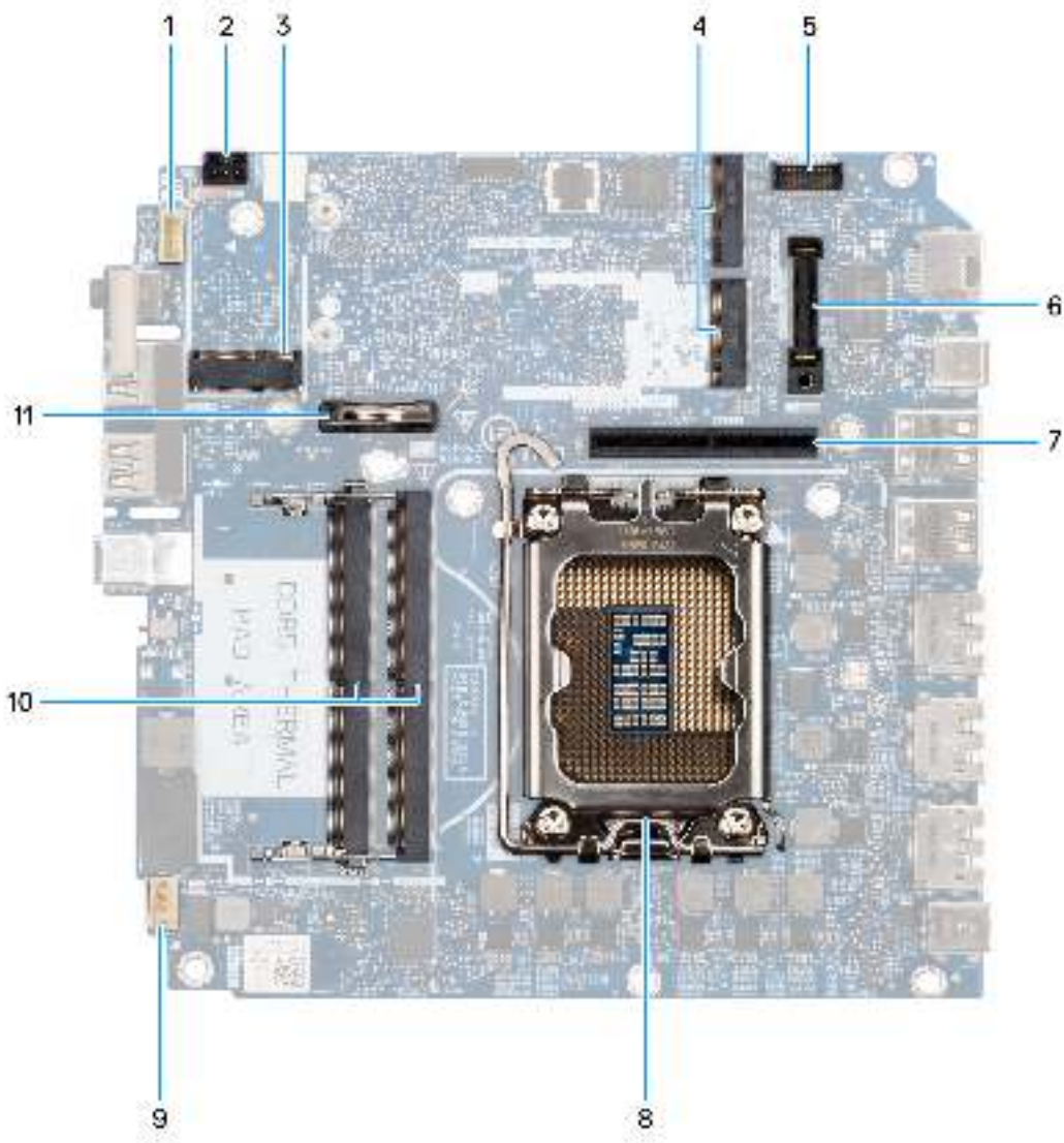
Abbildung 50. Anschlüsse auf der Hauptplatine
