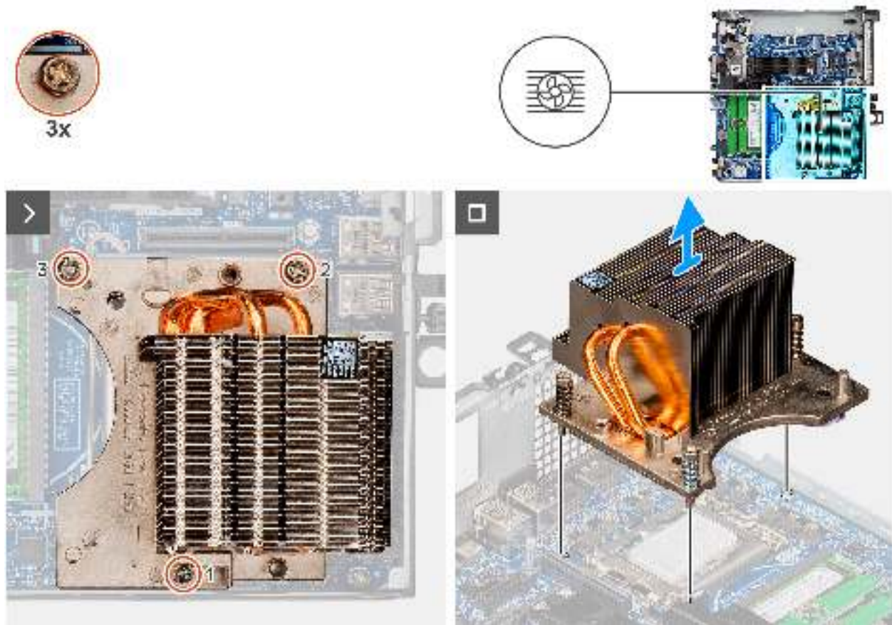
Abbildung 46. Kühlkörper entfernen
