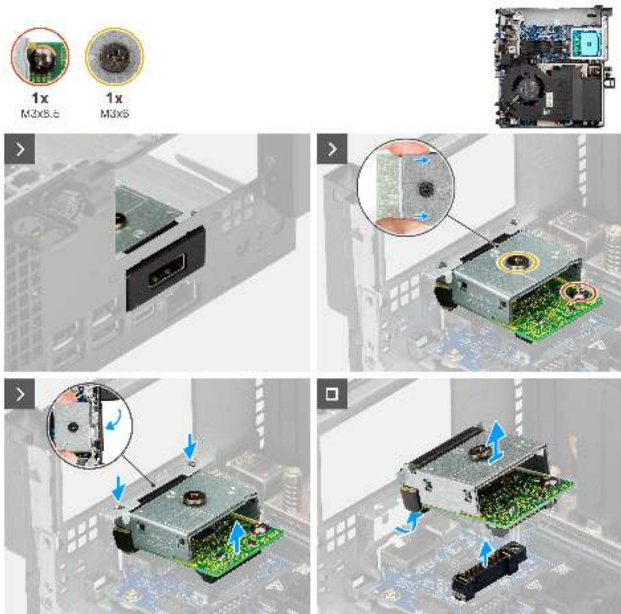
Abbildung 39. Entfernen des DisplayPorts
