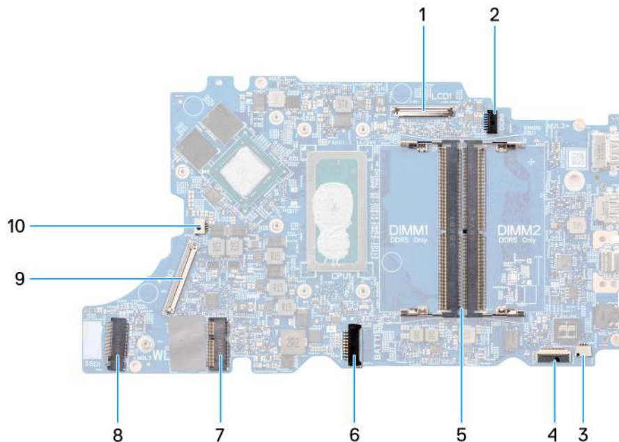
Abbildung 41. Hauptplattenanschlüsse
