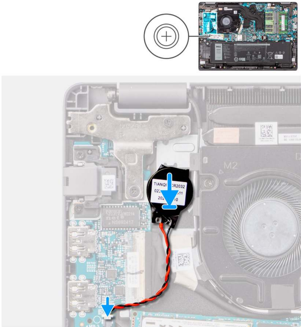
Abbildung 20. Einsetzen der Knopfzellenbatterie
