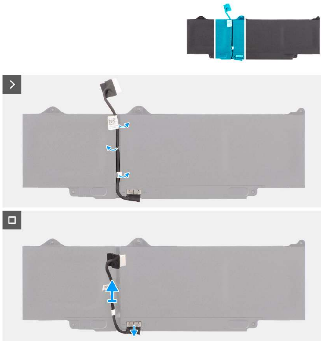
Abbildung 27. Entfernen des Akkukabels
