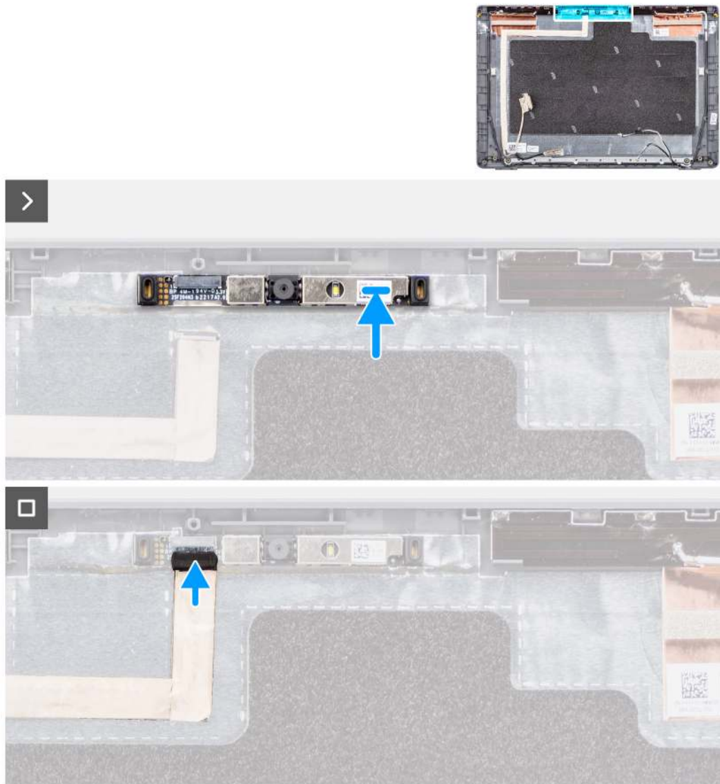
Abbildung 65. Installieren der Kamera
