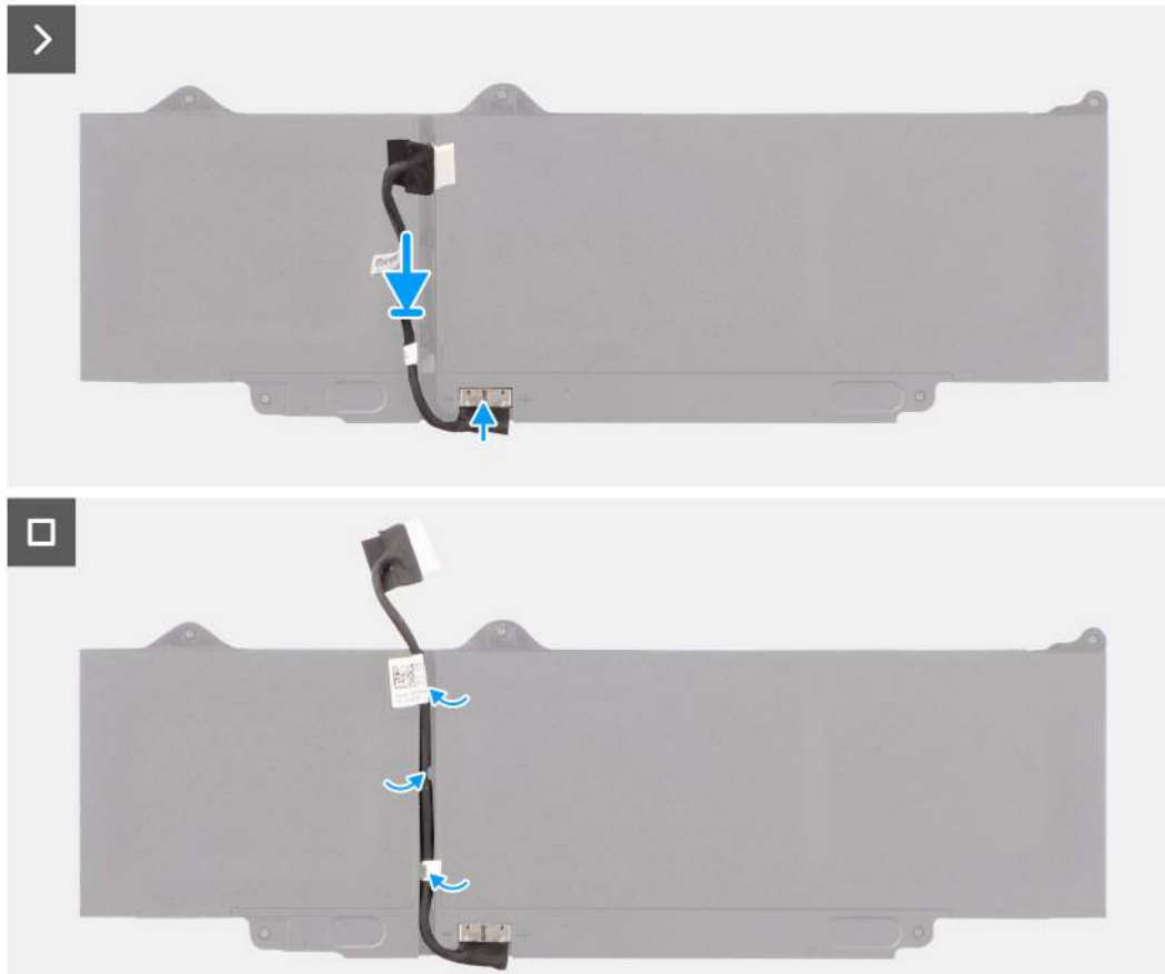
Abbildung 28. Einsetzen des Akkukabels
