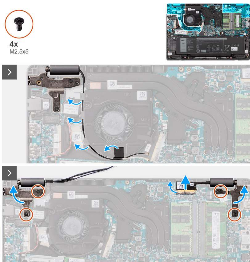
Abbildung 47. Entfernen der Bildschirmbaugruppe
