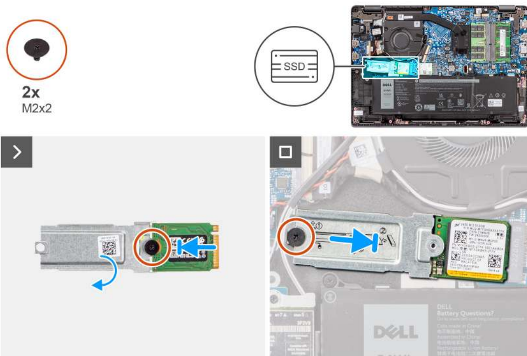
Abbildung 22. Installieren des M.2-2230-Solid-State-Laufwerks
