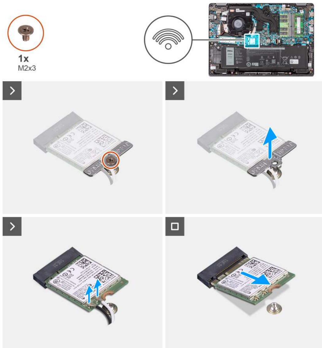
Abbildung 15. Entfernen der Wireless-Karte
