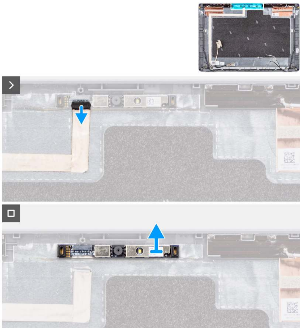
Abbildung 64. Entfernen der Kamera
