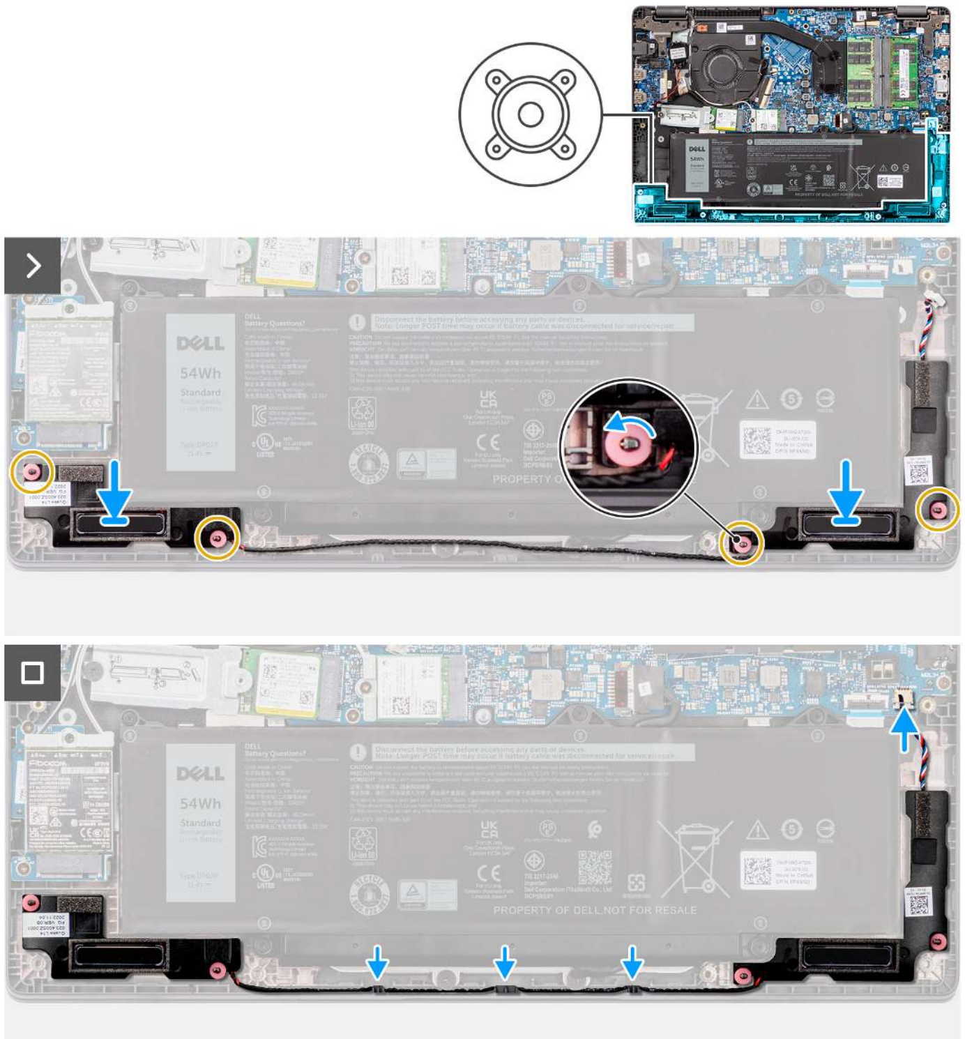
Abbildung 24. Einbauen der Lautsprecher
