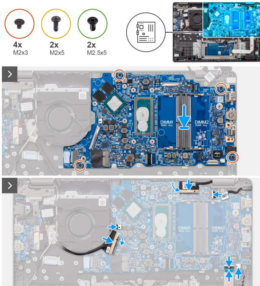
Abbildung 43. Einbauen der Hauptplatine
