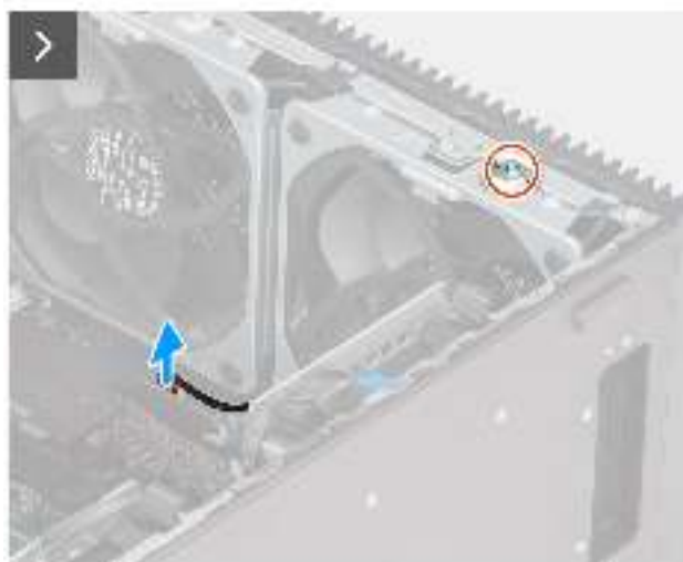
Abbildung 46. Vorderer Lüfter 2
