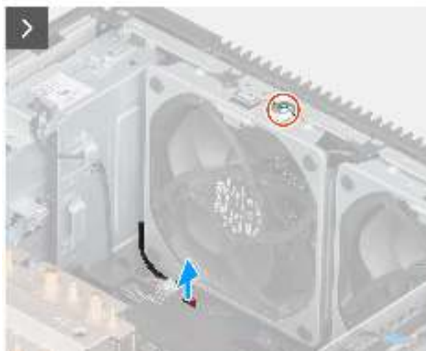
Abbildung 45. Vorderer Lüfter 1
