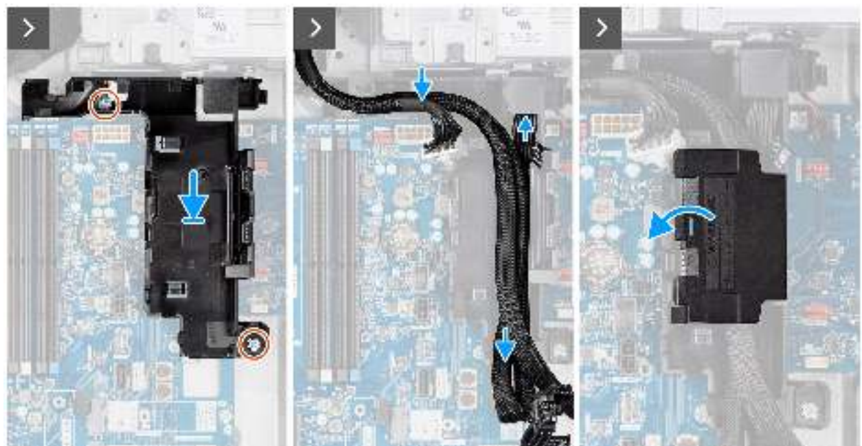
Abbildung 96. Einbauen der Systemplatine
