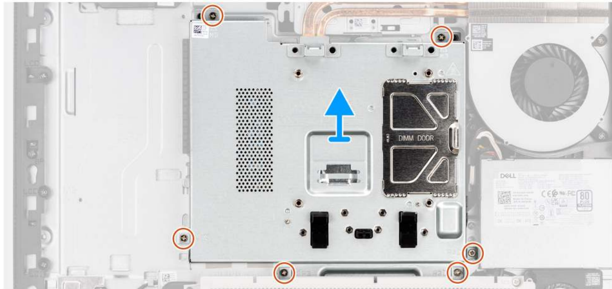
Abbildung 27. Entfernen der Abdeckung der Systemplatine
