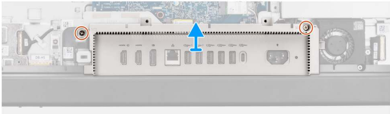
Abbildung 43. Entfernen der I/O-Abdeckung
