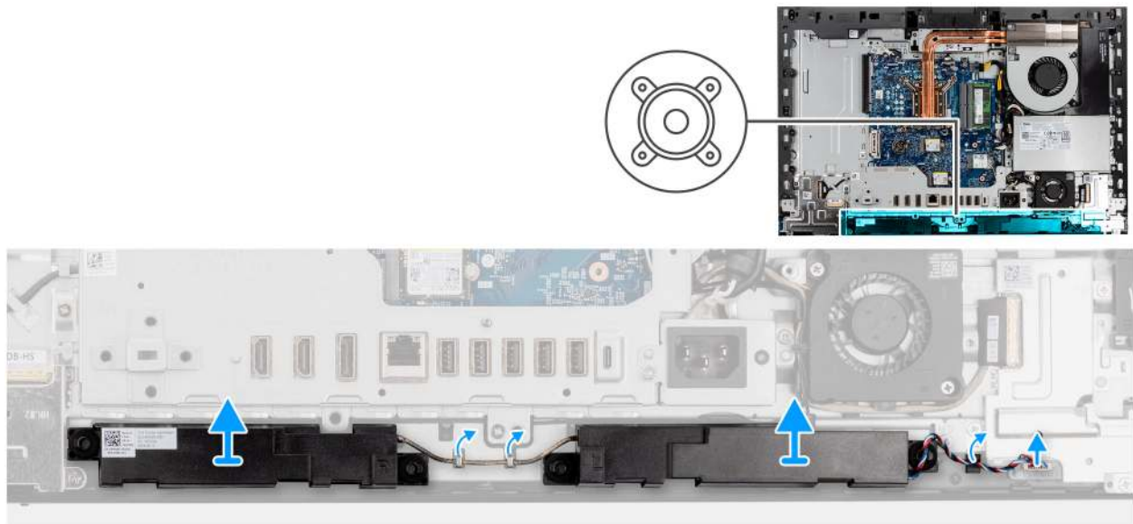
Abbildung 57. Entfernen der Lautsprecher
