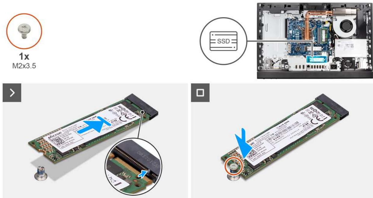
Abbildung 39. Installieren des M.2 2280-SSD-Laufwerks in M.2-Steckplatz 1
