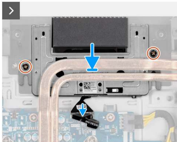
Abbildung 48. Installieren der einziehbaren Kamerabaugruppe
