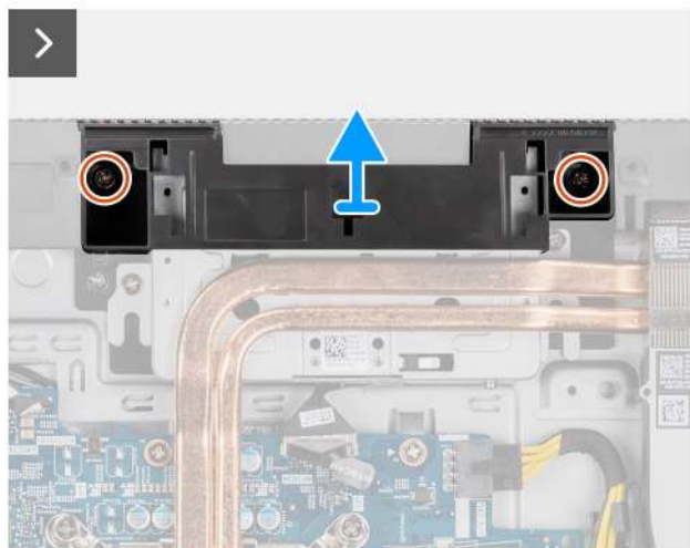
Abbildung 47. Entfernen der einziehbaren Kamerabaugruppe
