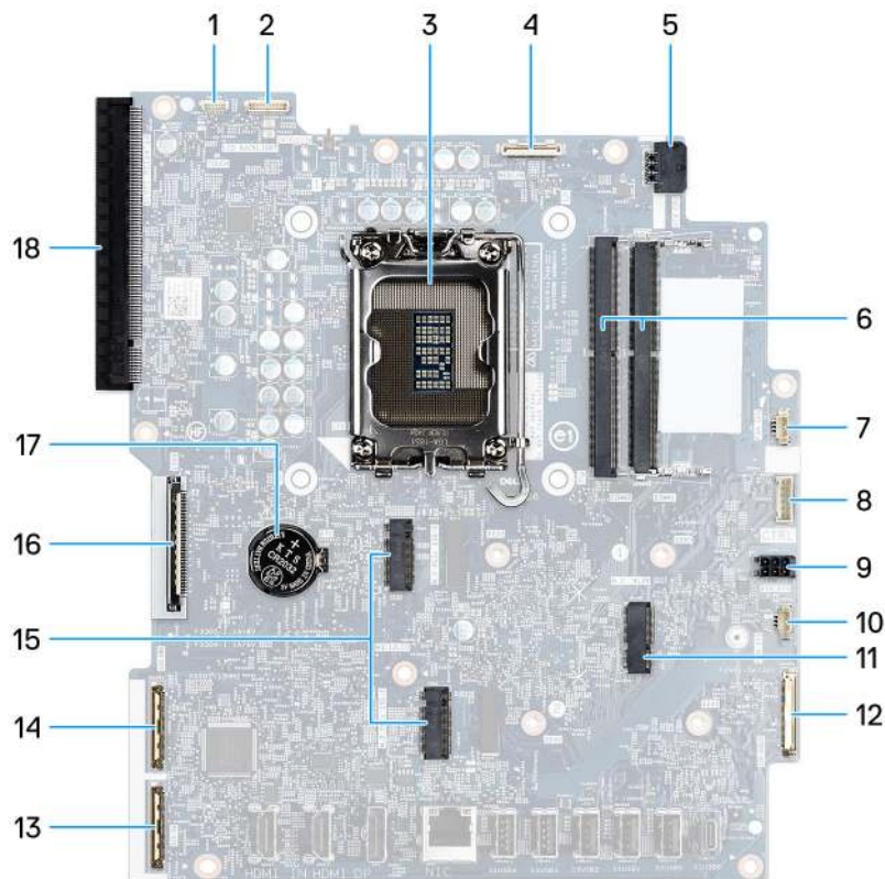
Abbildung 63. Systemplatinenbeschriftung
