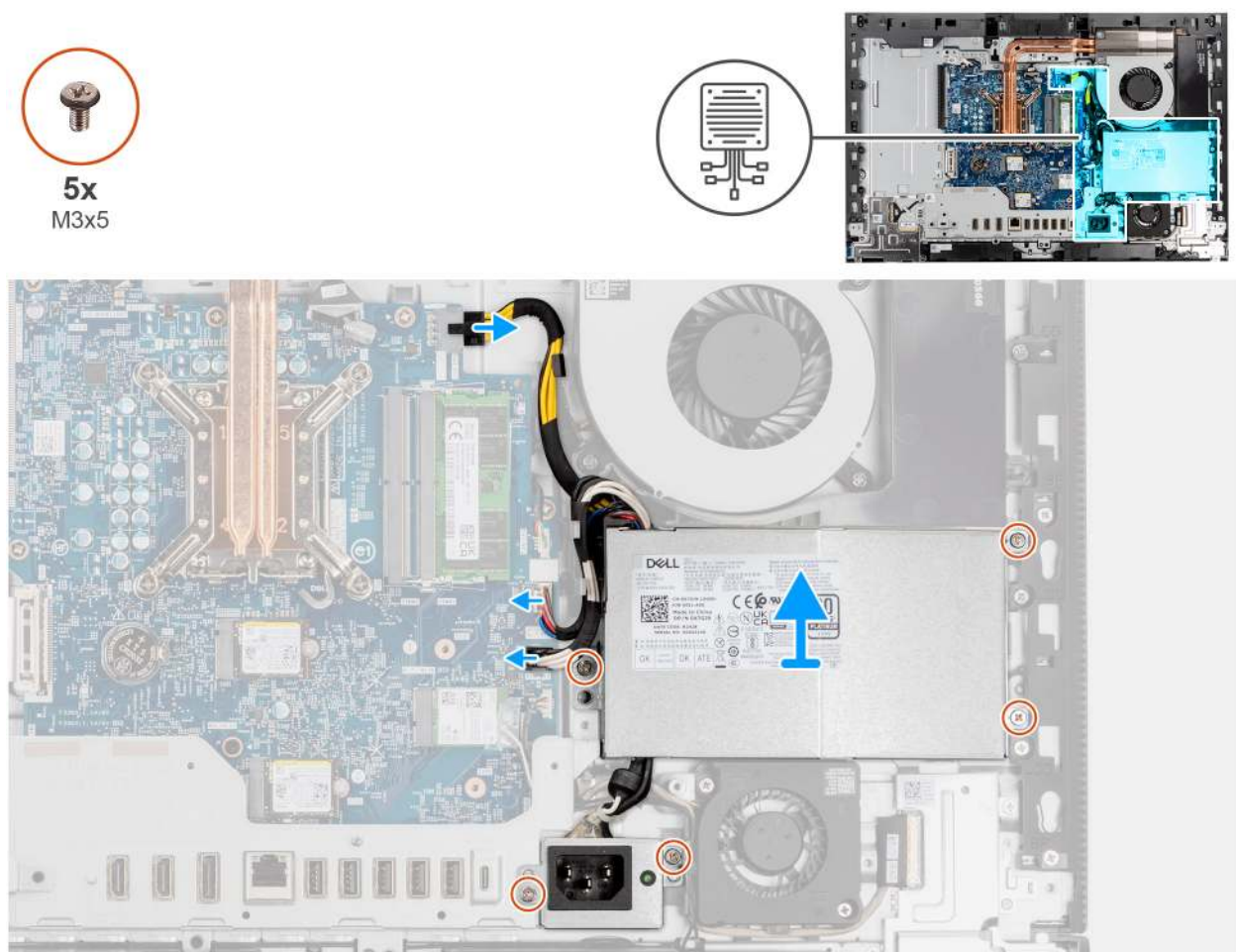
Abbildung 51. Entfernen der Stromversorgungseinheit
