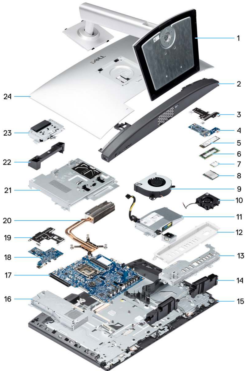
Abbildung 14. Hauptkomponenten Ihres Dell Pro 24-All-in-one Plus, QB24250
