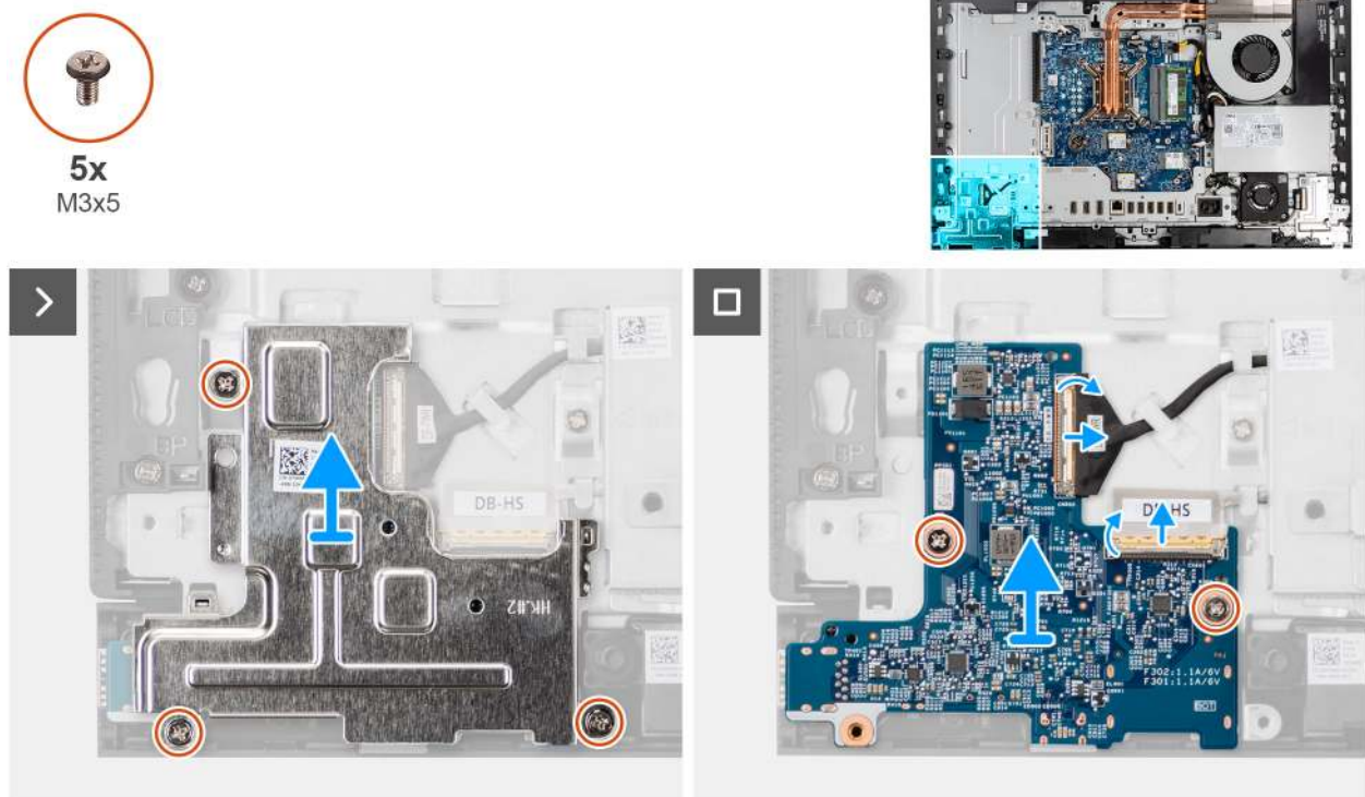
Abbildung 69. Entfernen des Netzschalters und der E/A-Platine
