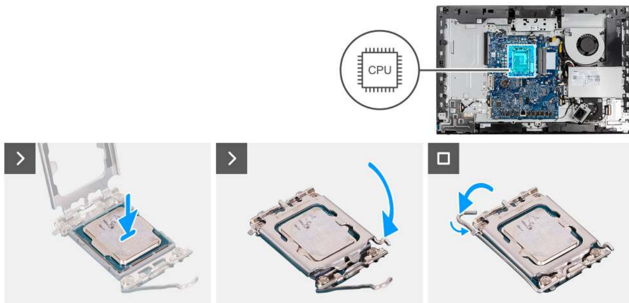
Abbildung 62. Einbauen des Prozessors
