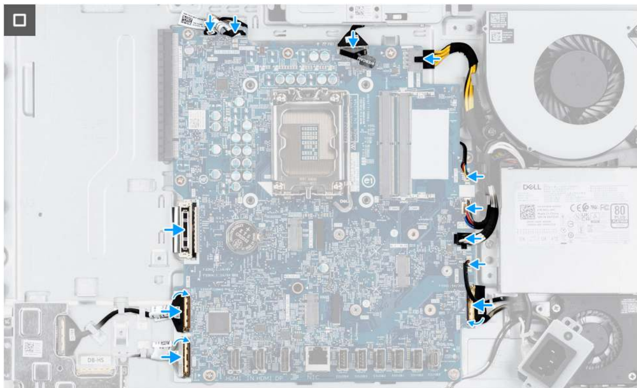
Abbildung 68. Einbauen der Systemplatine
