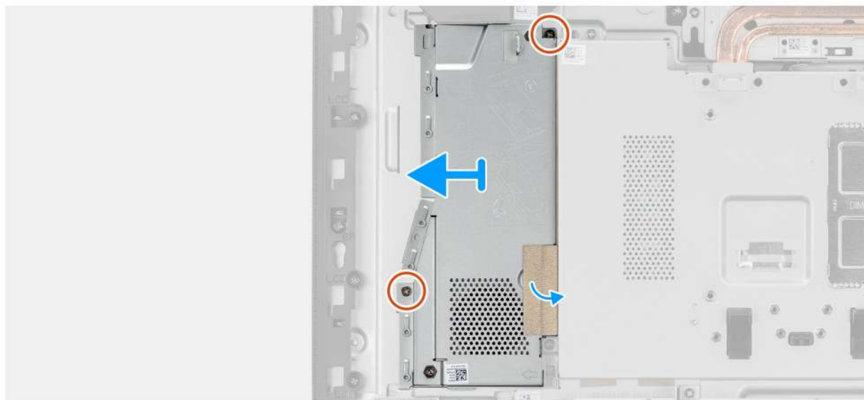
Abbildung 23. Entfernen der Grafikkartenbaugruppe (Modell mit Touch-Funktion)
