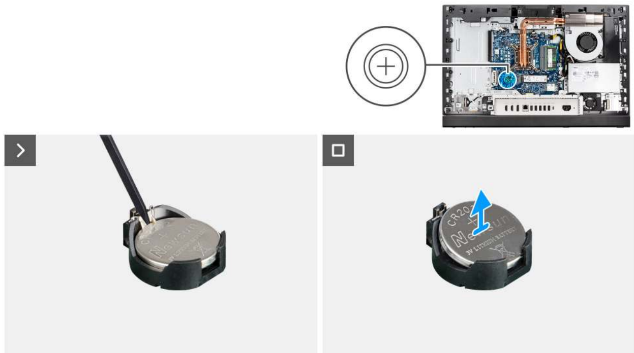
Abbildung 41. Entfernen der Knopfzellenbatterie
