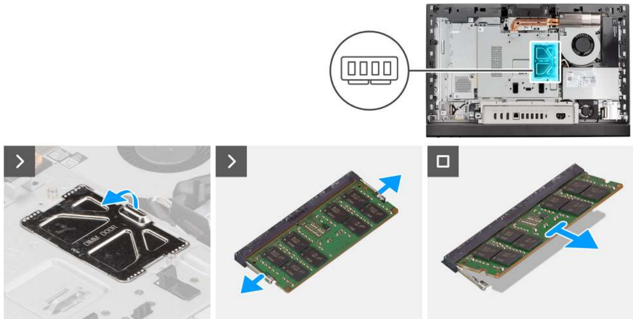
Abbildung 21. Entfernen des Speichers
