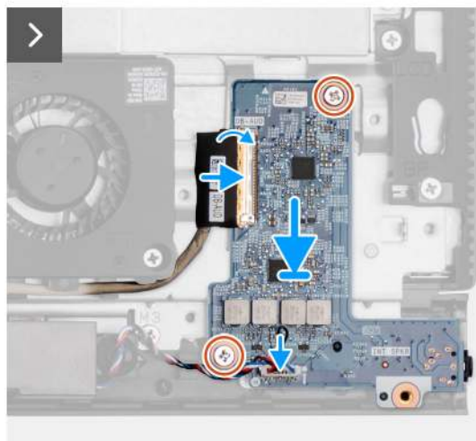
Abbildung 72. Einbauen der Audioplattine
