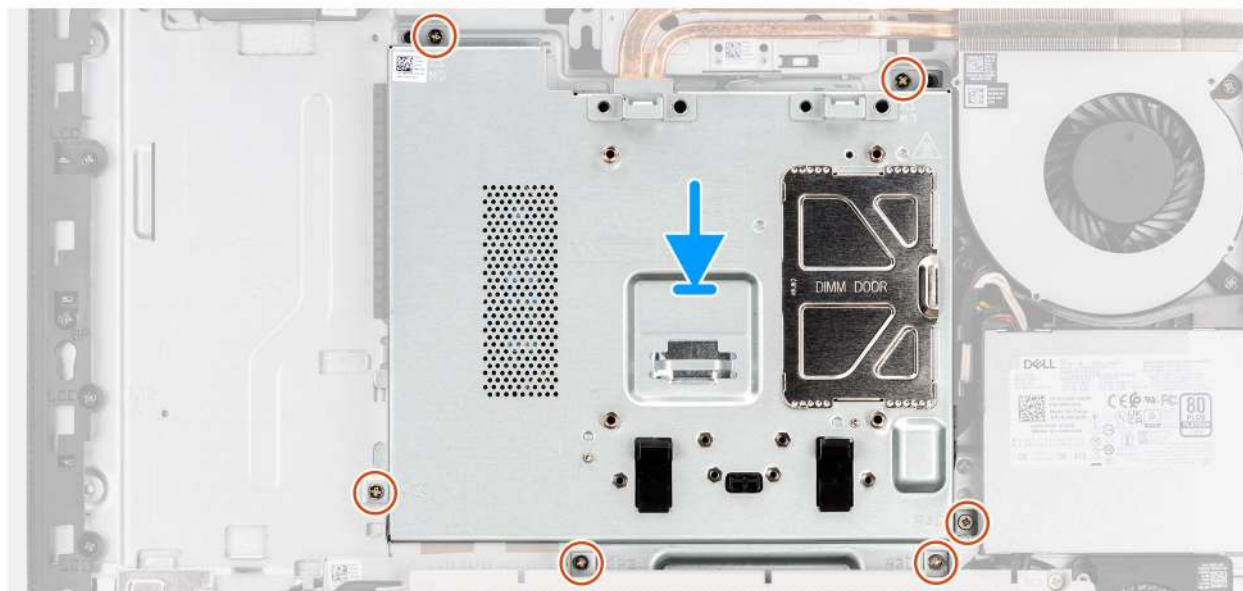
Abbildung 28. Einbauen der Abdeckung der Systemplatine
