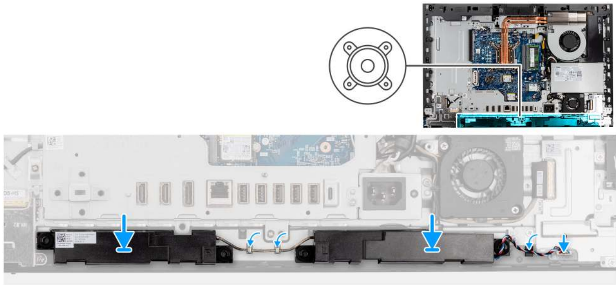
Abbildung 58. Installieren der Lautsprecher
