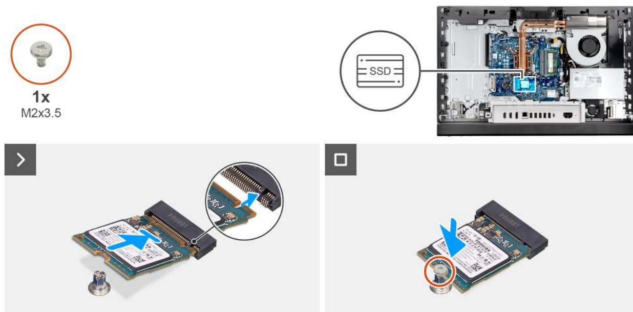
Abbildung 32. Installieren des M.2-2230-SSD-Laufwerks in M.2-Steckplatz 0
