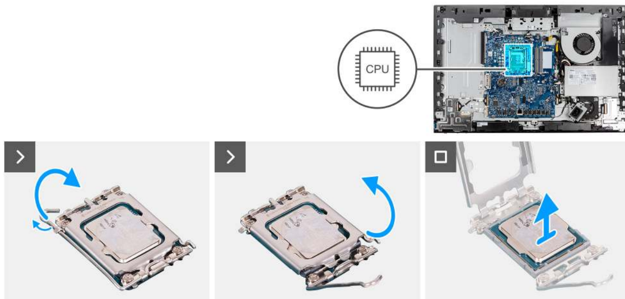
Abbildung 61. Entfernen des Prozessors
