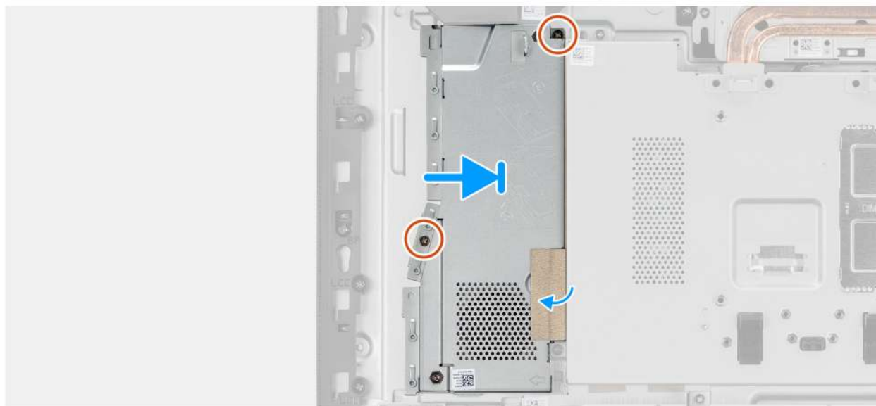
Abbildung 26. Installieren der Grafikkartenbaugruppe (Modell ohne Touch-Funktion)
