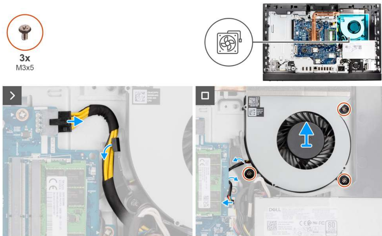
Abbildung 49. Entfernen des Lüfters
