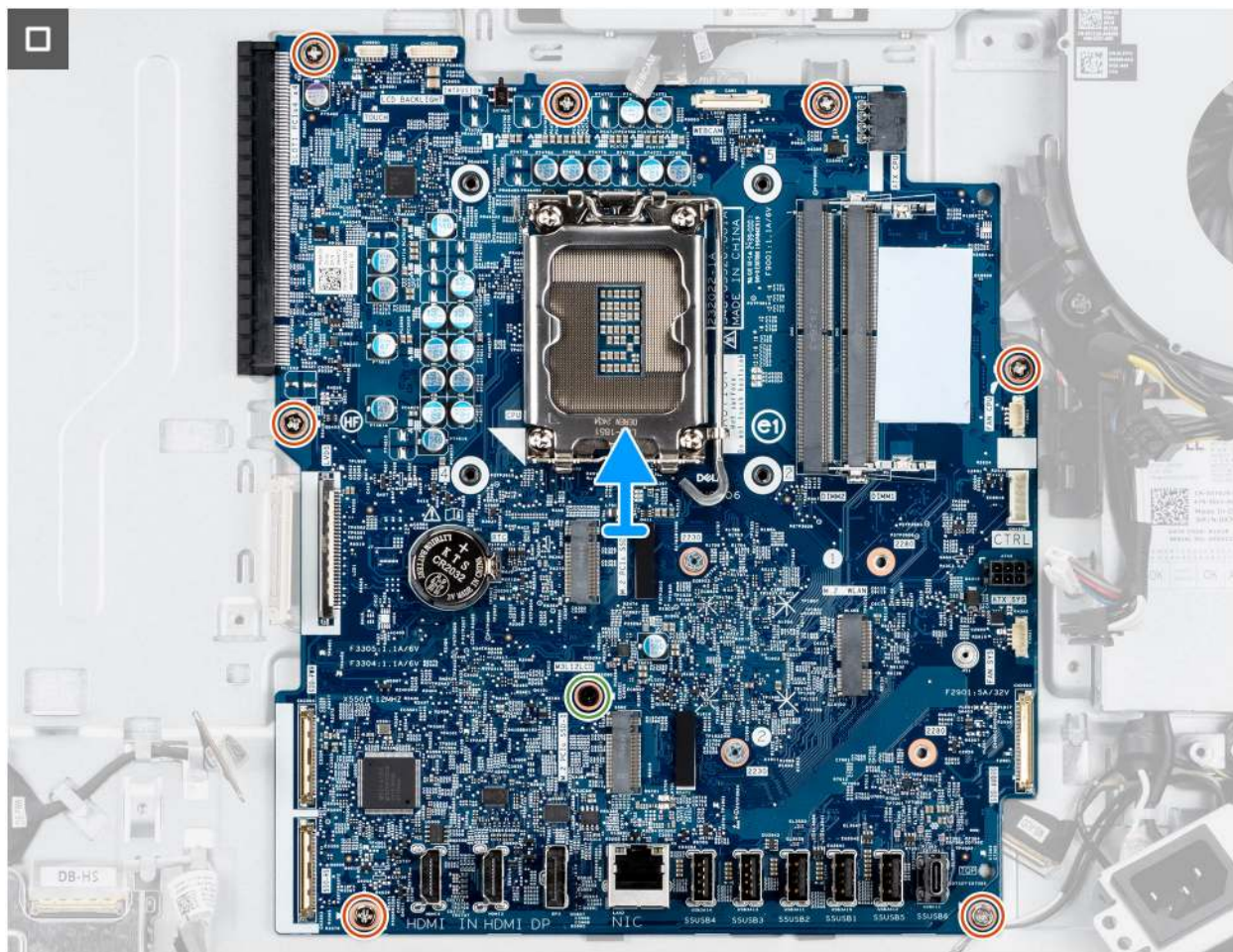
Abbildung 65. Entfernen der Systemplatine
