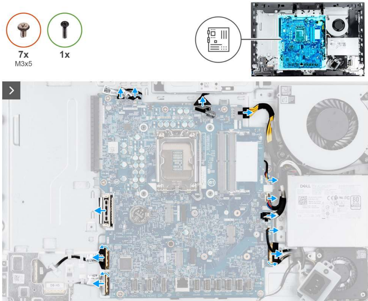
Abbildung 64. Entfernen der Systemplatine
