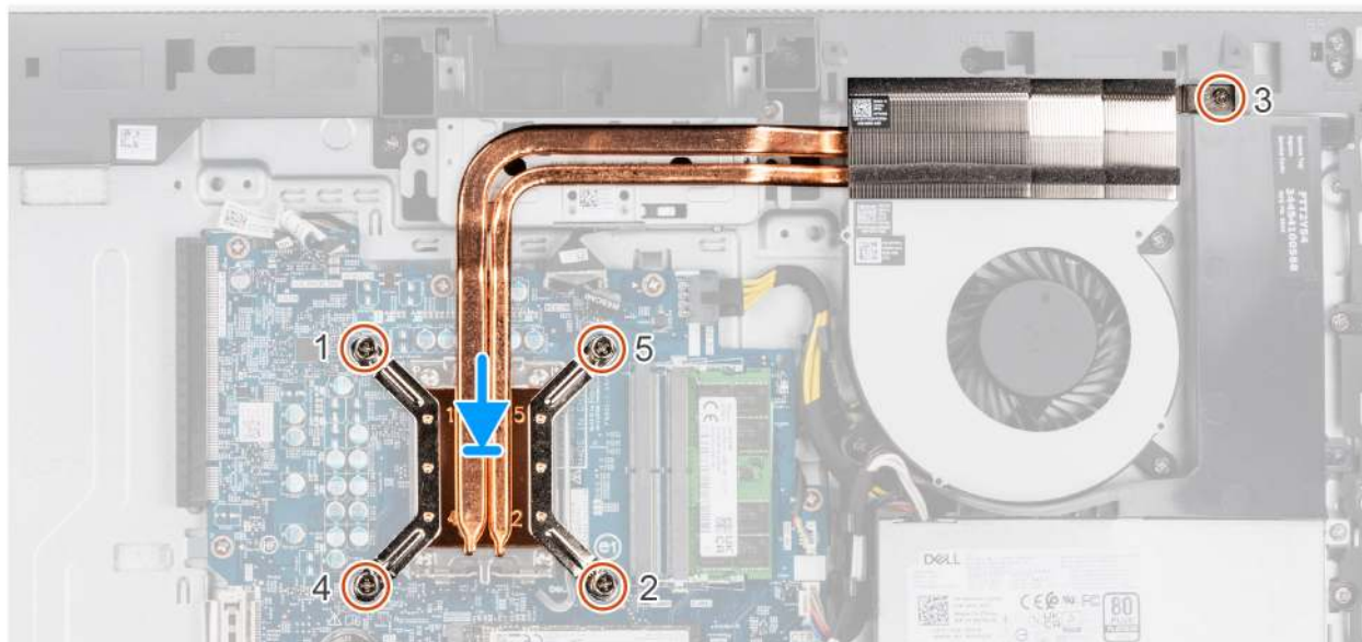
Abbildung 60. Einsetzen des Kühlkörpers
