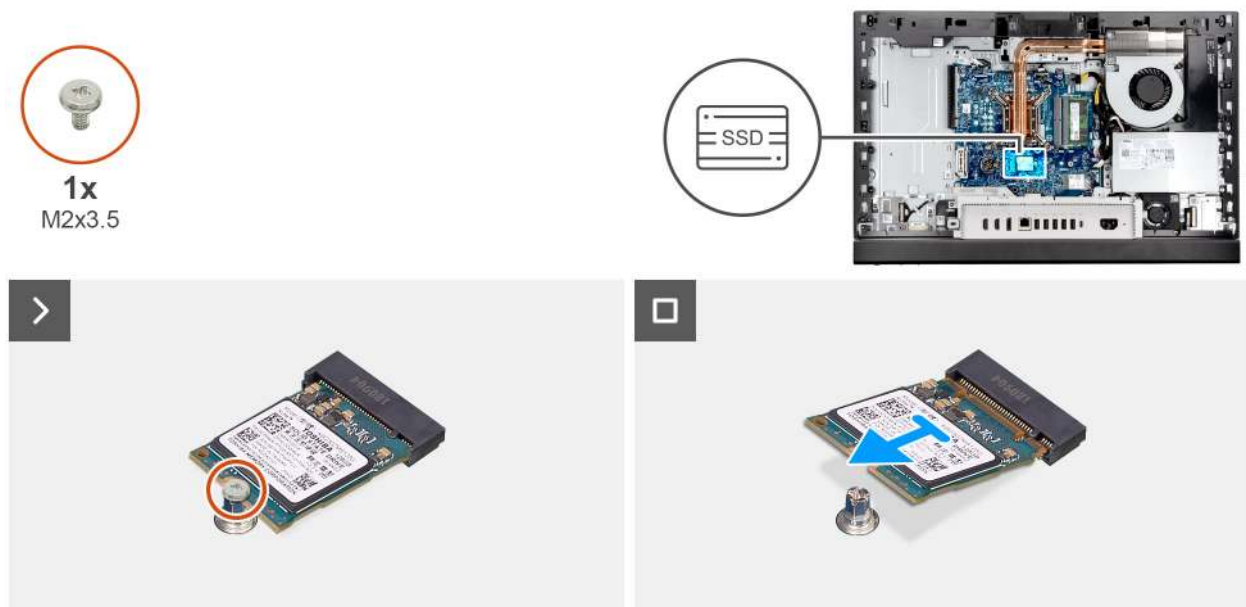
Abbildung 31. Entfernen des M.2 2230-SSD-Laufwerks aus M.2-Steckplatz 0
