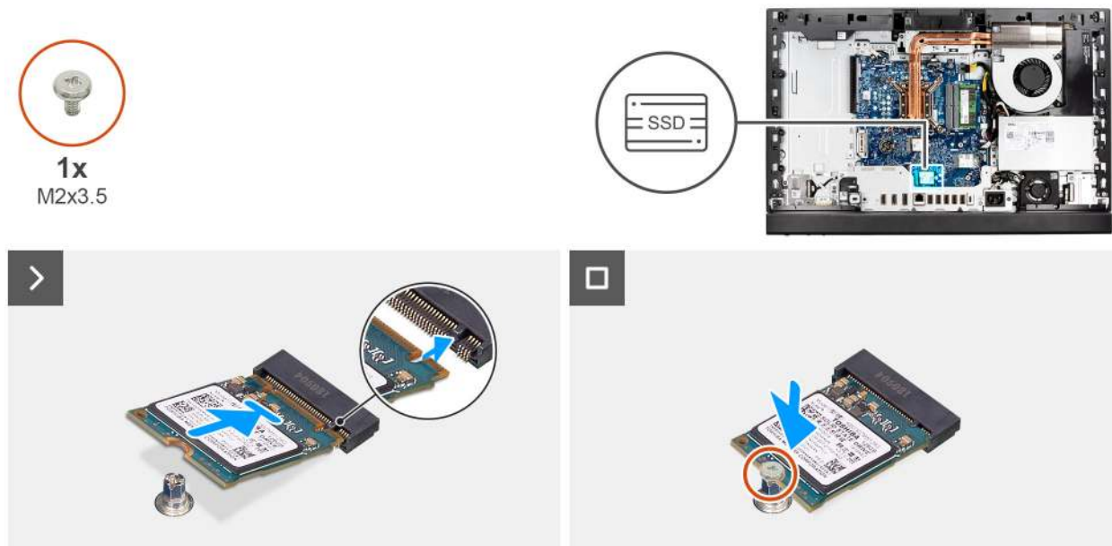
Abbildung 37. Installieren des M.2-2230-SSD-Laufwerks in M.2-Steckplatz 1
