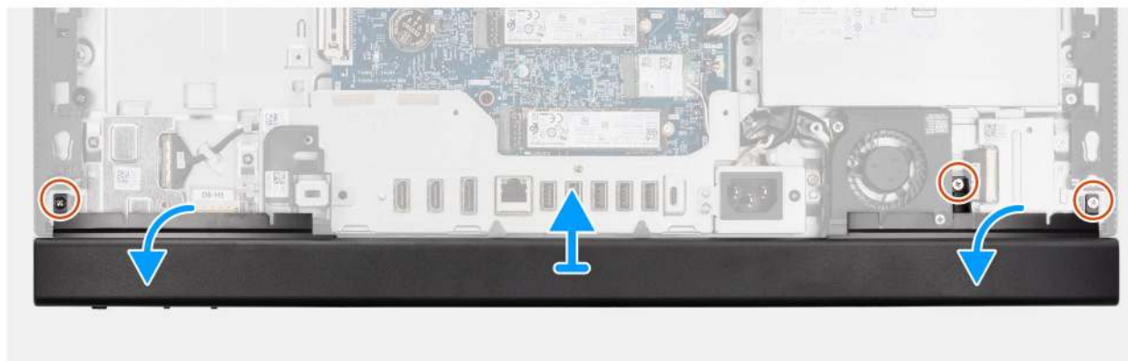
Abbildung 45. Entfernen der unteren Abdeckung
