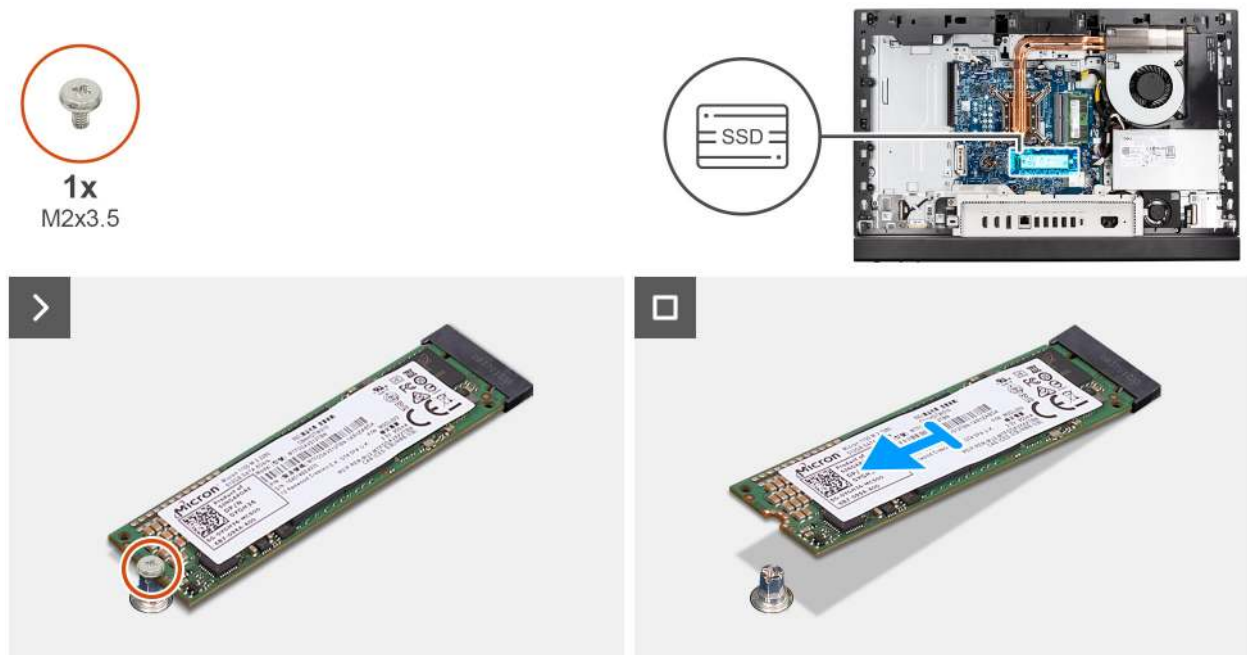
Abbildung 33. Entfernen des M.2 2280-SSD-Laufwerks aus M.2-Steckplatz 0
