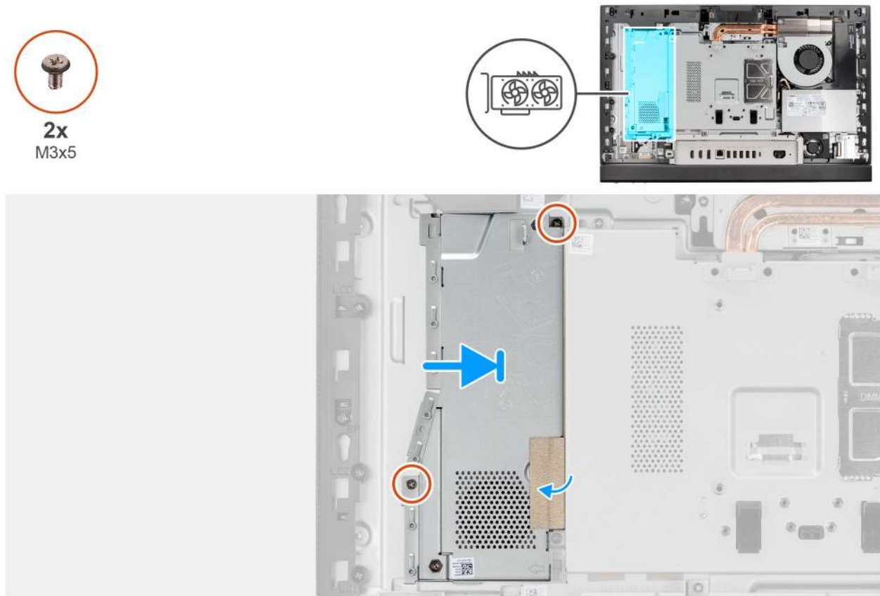
Abbildung 25. Installieren der Grafikkartenbaugruppe (Modell mit Touch-Funktion)
