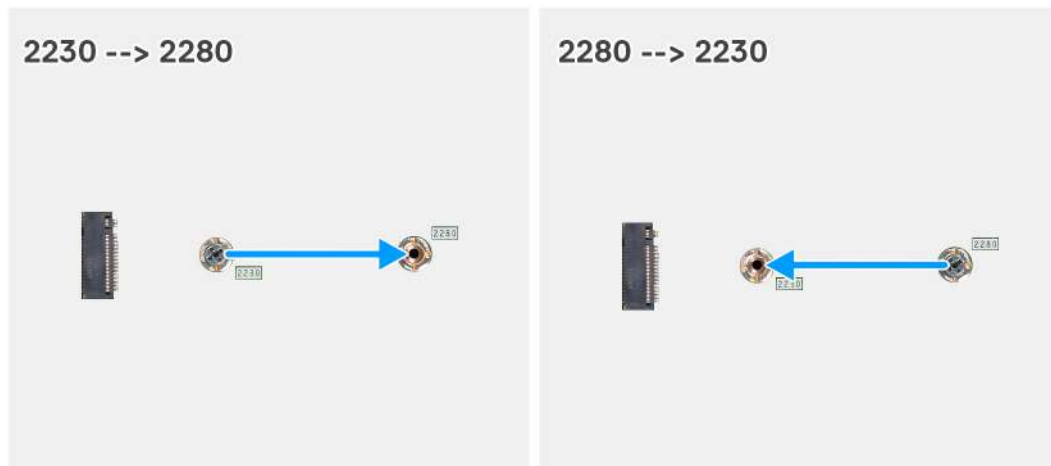
Abbildung 40. Verschieben der Solid-State-Schraubenhalterung auf M.2-Steckplatz 1
