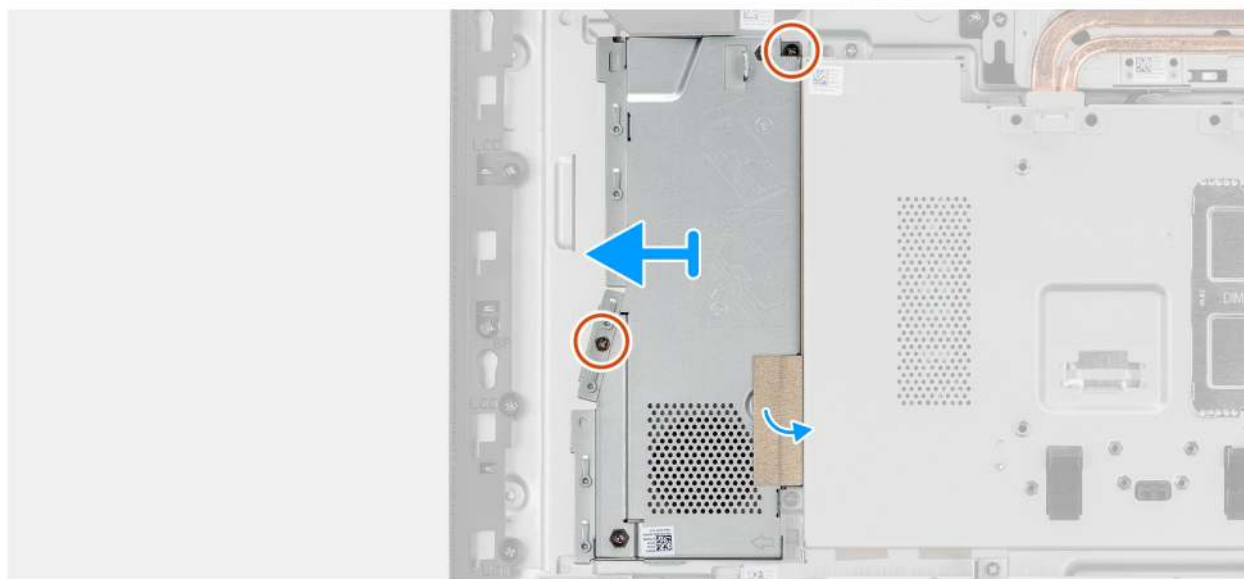
Abbildung 24. Entfernen der Grafikkartenbaugruppe (Modell ohne Touch-Funktion)
