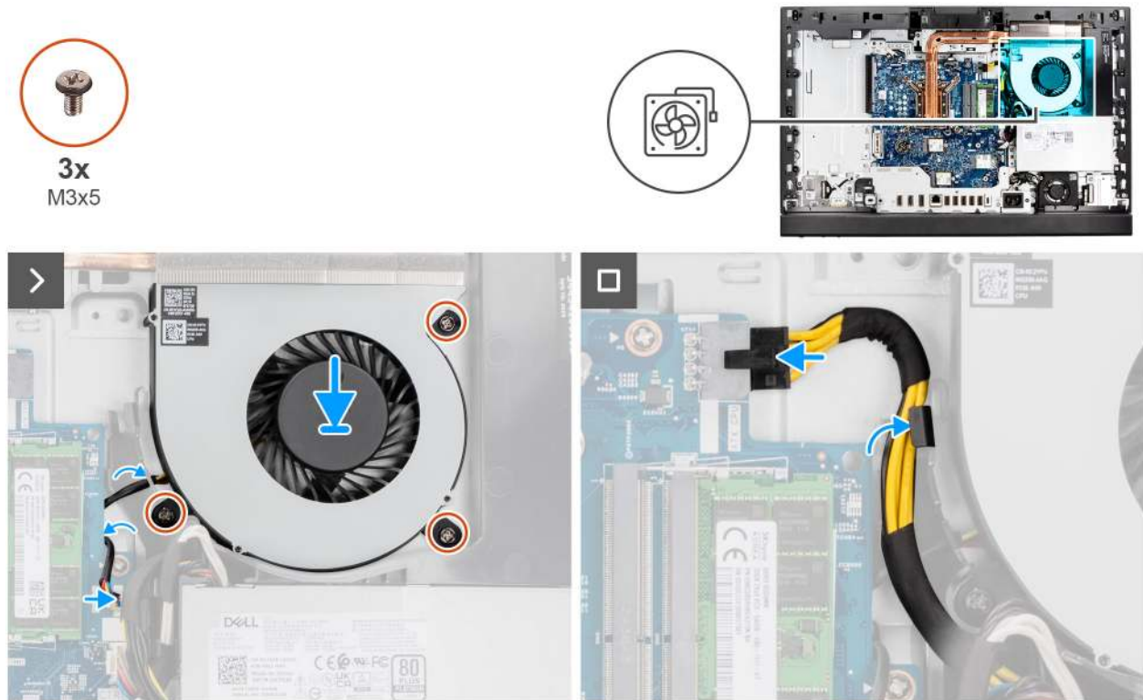
Abbildung 50. Einbauen des Lüfters
