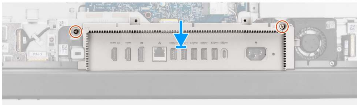
Abbildung 44. Einbauen der E/A-Abdeckung
