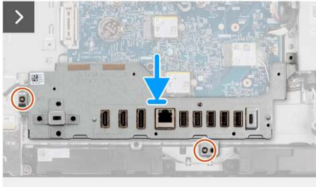
Abbildung 56. Einbauen der E/A-Halterung
