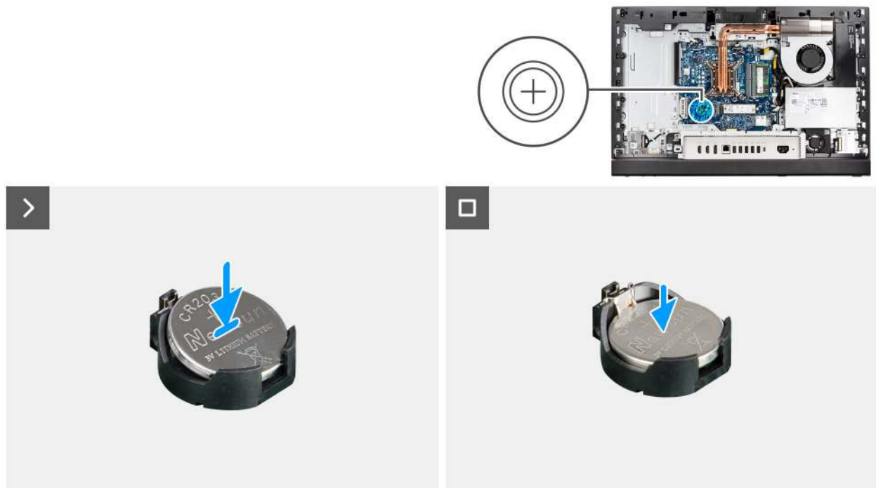
Abbildung 42. Einsetzen der Knopfzellenbatterie
