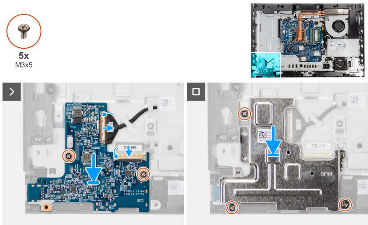
Abbildung 70. Einbauen der Netzschalter- und E/A-Platine
