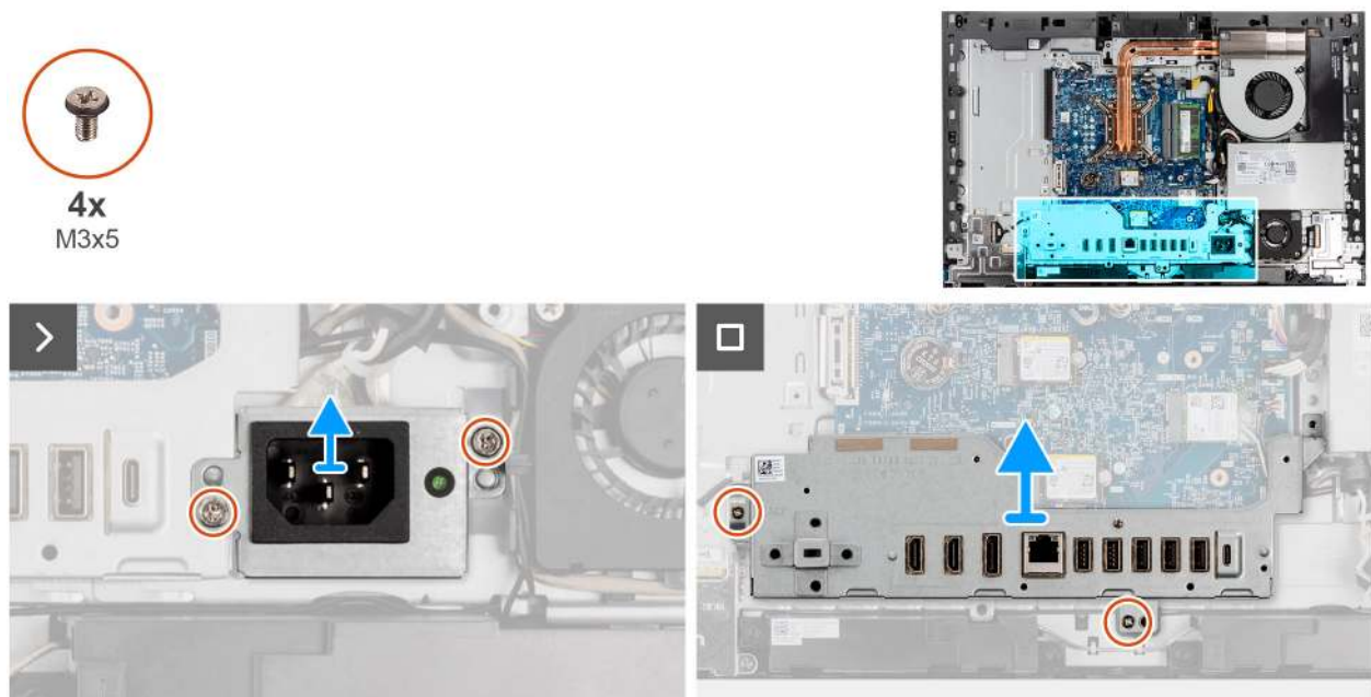
Abbildung 55. Entfernen der E/A-Halterung
