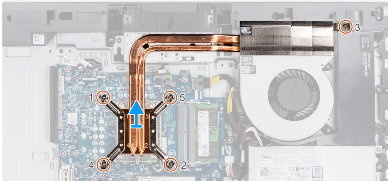
Abbildung 59. Kühlkörper entfernen
