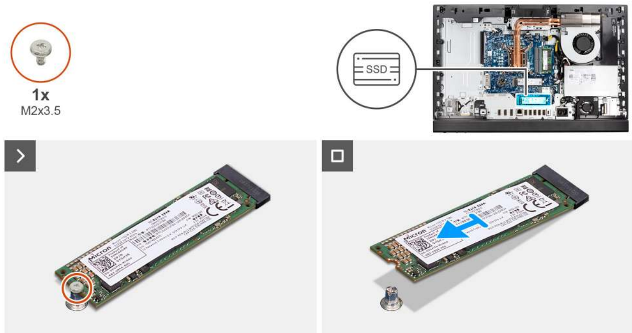
Abbildung 38. Entfernen des M.2 2280-SSD-Laufwerks aus M.2-Steckplatz 1
