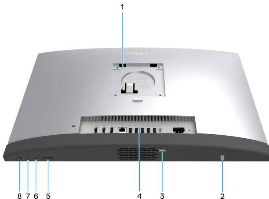
Abbildung 7. Untere Ansicht
