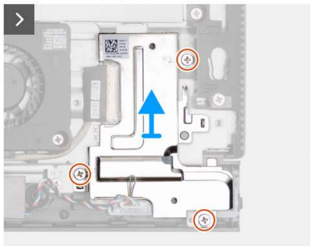
Abbildung 71. Entfernen der Audioplatine
