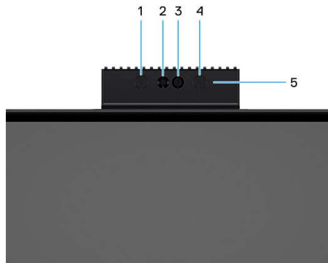
Abbildung 5. Einziehbare Kamera mit 5-MP-RGB- und -Infrarotkamera
