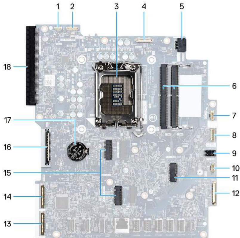
Abbildung 66. Systemplatinenbeschriftung
