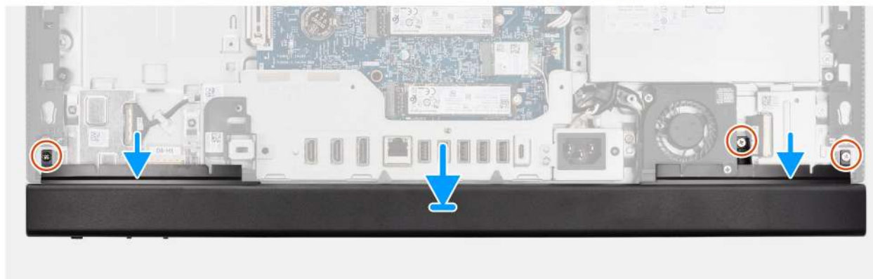
Abbildung 46. Anbringen der unteren Abdeckung
