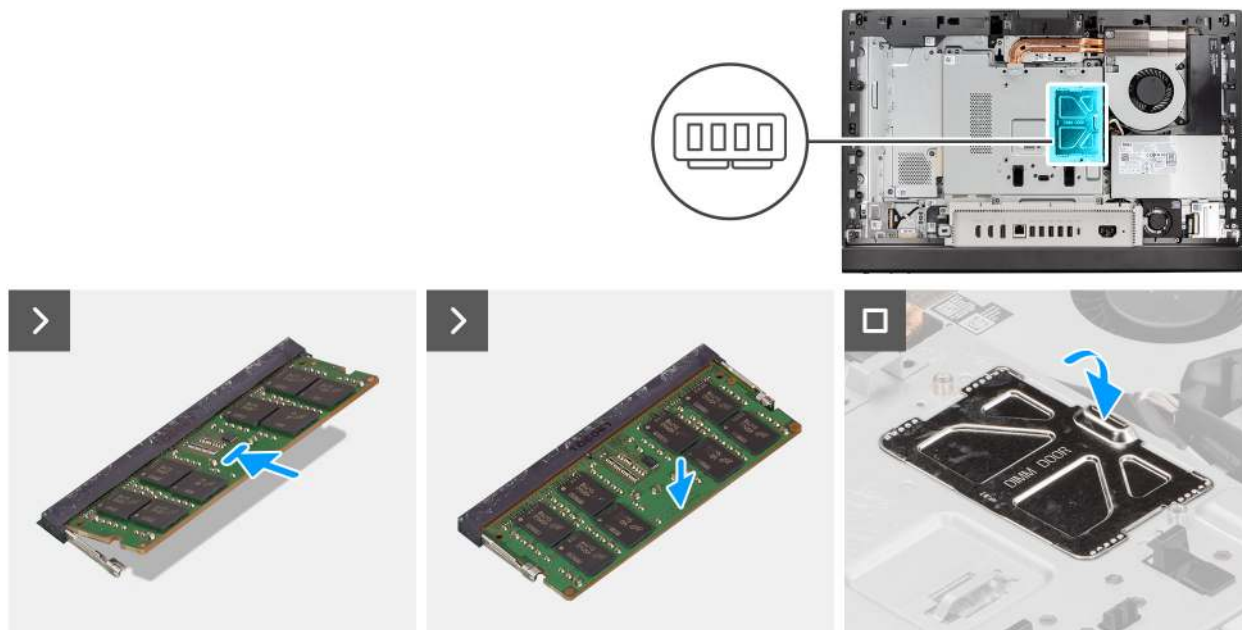
Abbildung 22. Einbauen des Speichers
