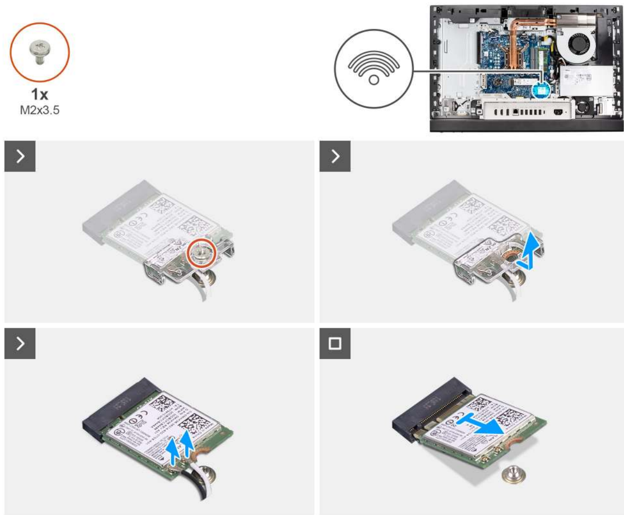
Abbildung 29. Entfernen der Wireless-Karte
