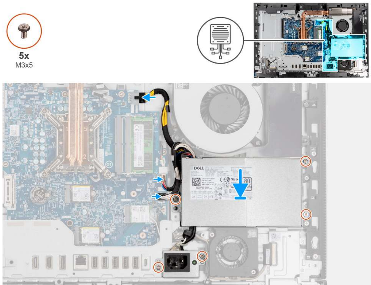
Abbildung 52. Installieren der Stromversorgungseinheit
