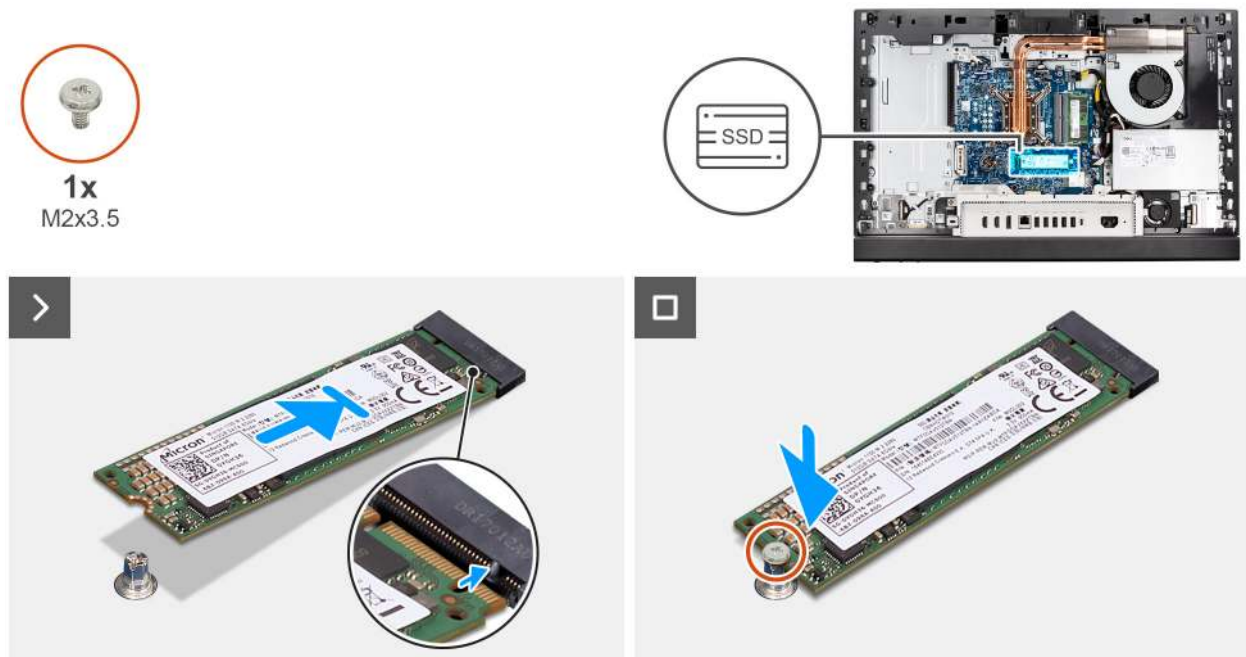
Abbildung 34. Installieren des M.2 2280-SSD-Laufwerks in M.2-Steckplatz 0
