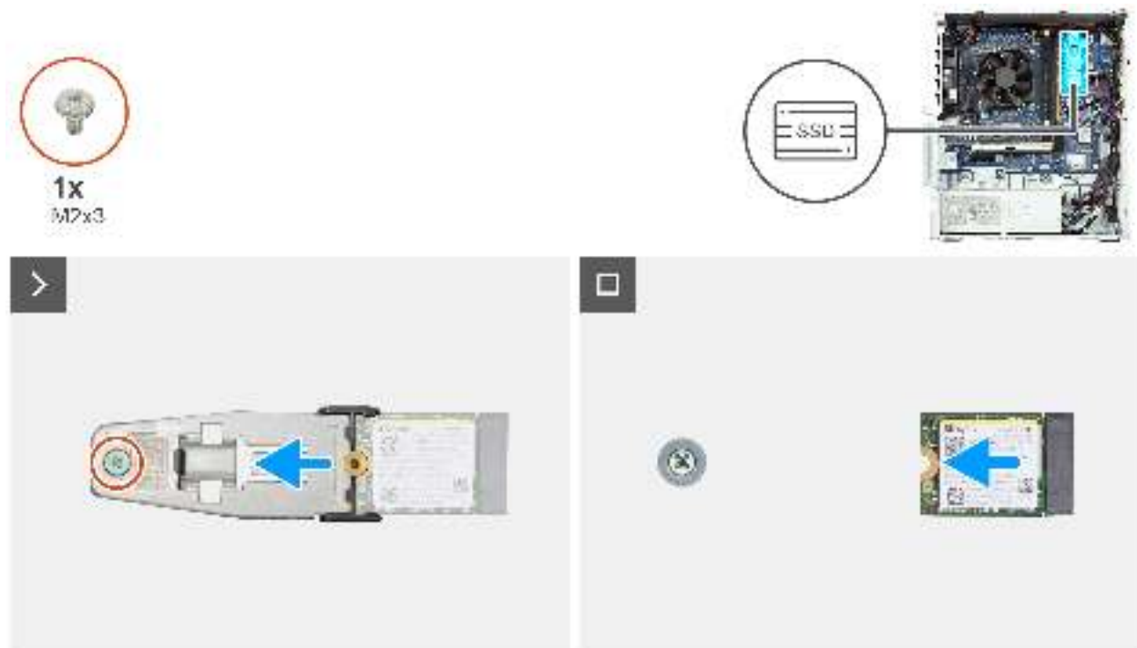
Abbildung 35. Entfernen des M.2-2230-SSD-Laufwerks aus Steckplatz 2
