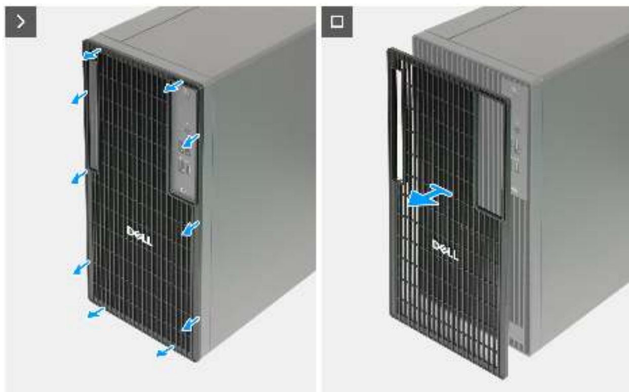
Abbildung 20. Entfernen des Staubfilters
