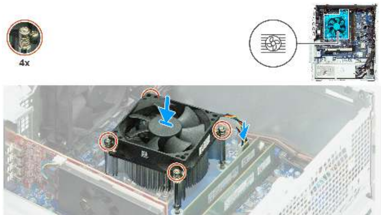
Abbildung 91. Installieren des Prozessorlüfters und der Kühlkörperbaugruppe
