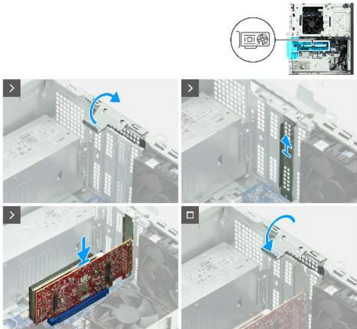
Abbildung 40. Installieren der Grafikkarte
