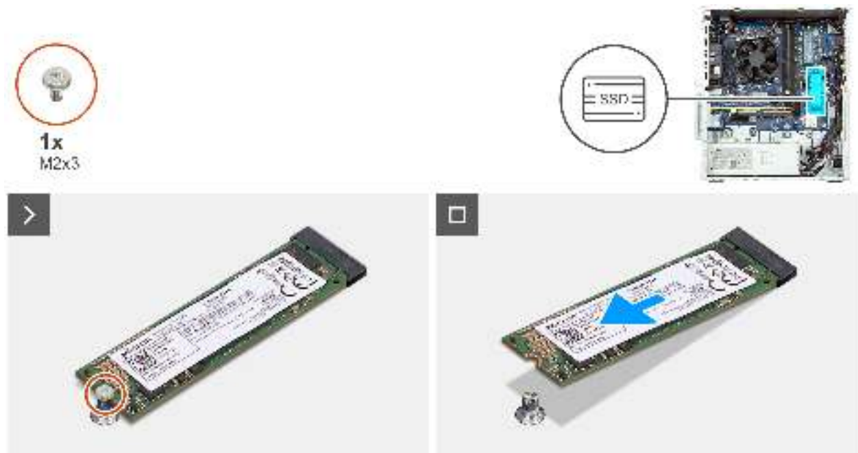
Abbildung 30. Entfernen des M.2-2280-SSD-Laufwerks aus Steckplatz 0
