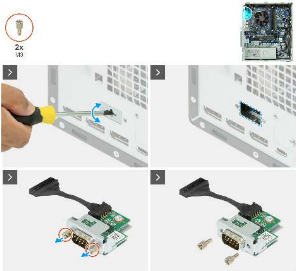
Abbildung 80. Installieren des seriellen Anschlussmoduls
