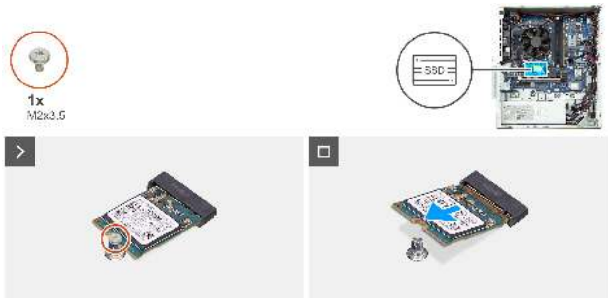
Abbildung 33. Entfernen des M.2-2230-SSD-Laufwerks aus Steckplatz 1
