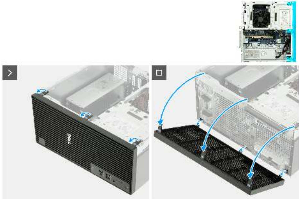
Abbildung 22. Entfernen der vorderen Abdeckung
