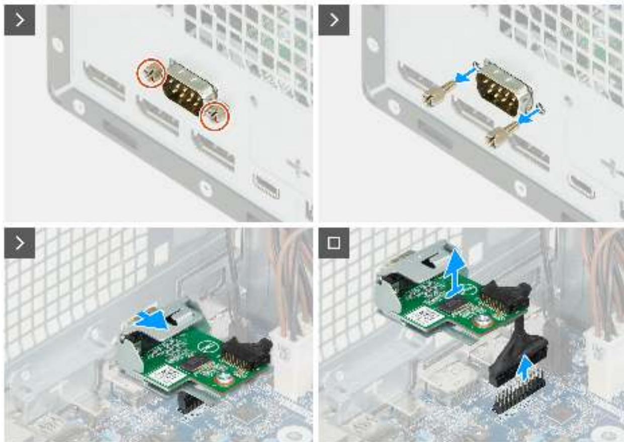
Abbildung 79. Entfernen des Moduls für den seriellen Anschluss
