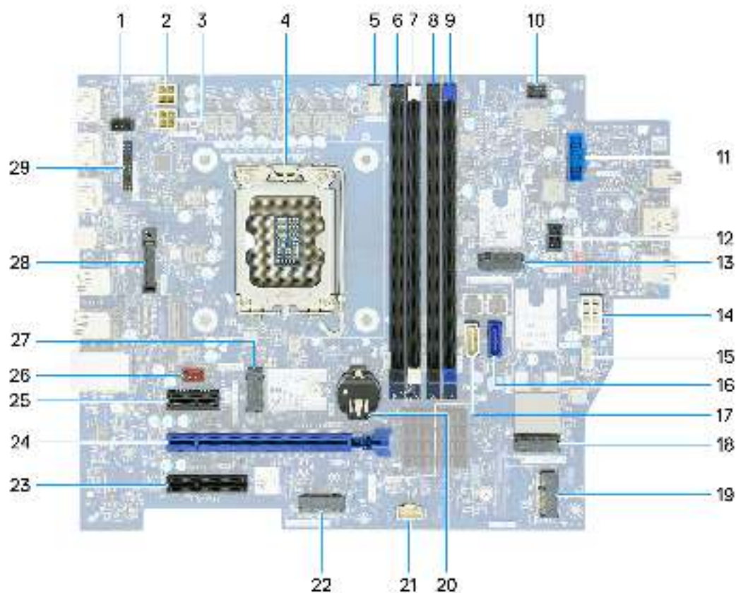
Abbildung 94. Systemplatinenbeschriftung
