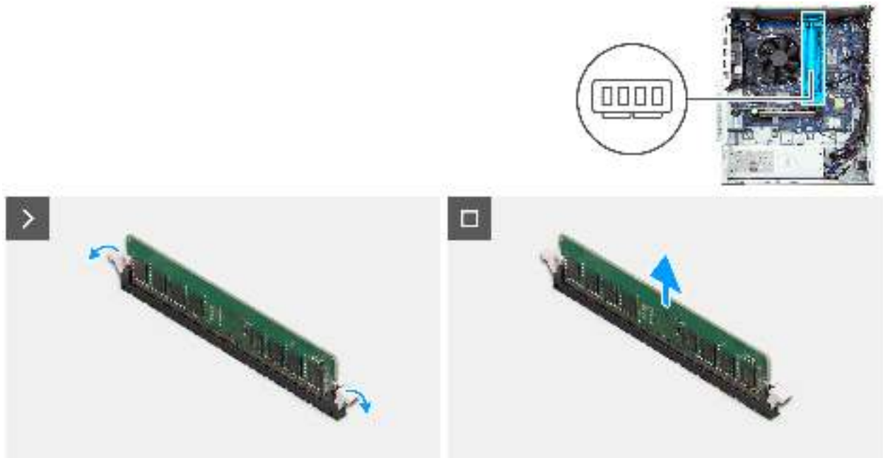
Abbildung 26. Entfernen des Speichers
