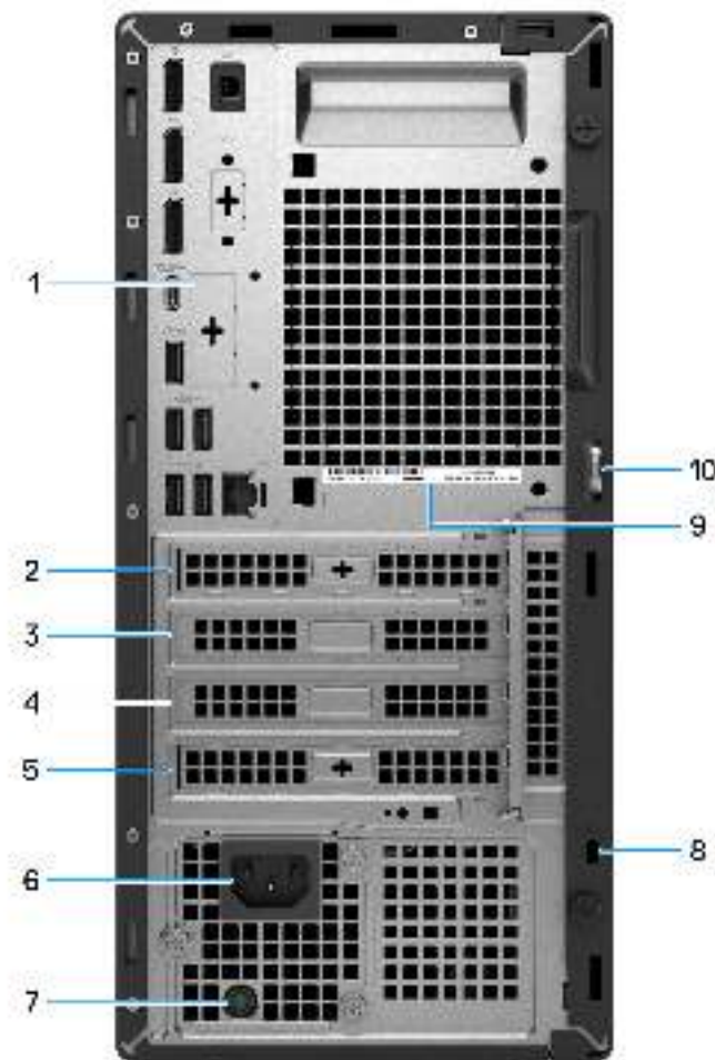
Abbildung 2. Rückseite des Dell Pro Tower Plus, QBT1250
