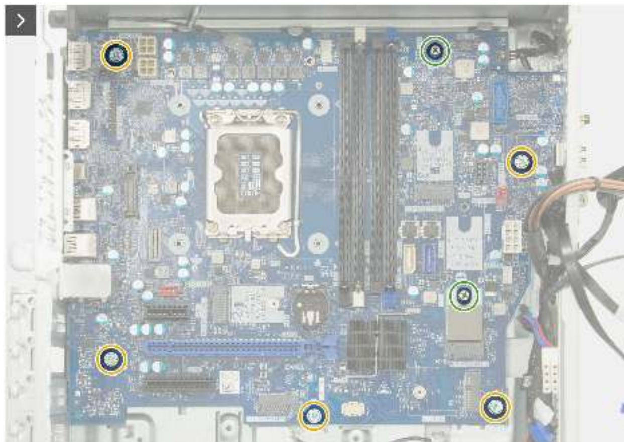
Abbildung 101. Einbauen der Systemplatine
