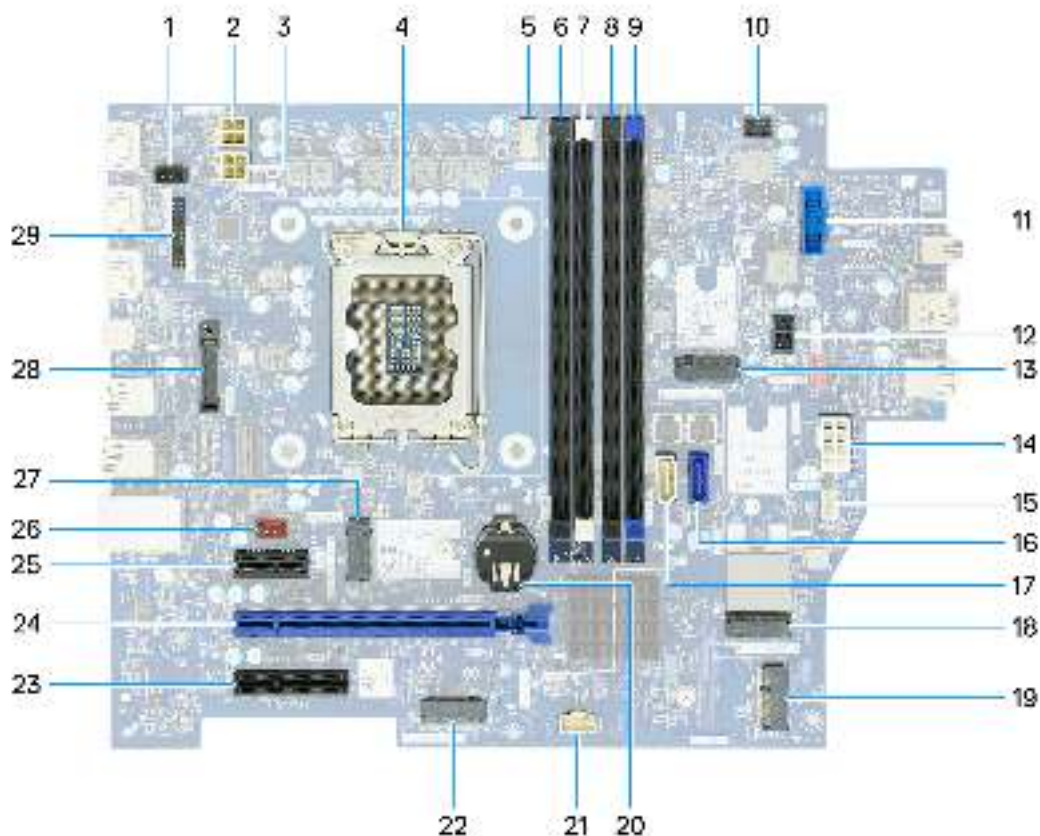
Abbildung 99. Systemplatinenbeschriftung
