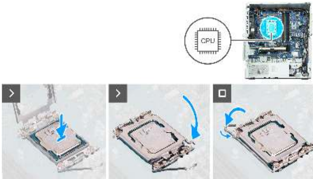
Abbildung 93. Einbauen des Prozessors
