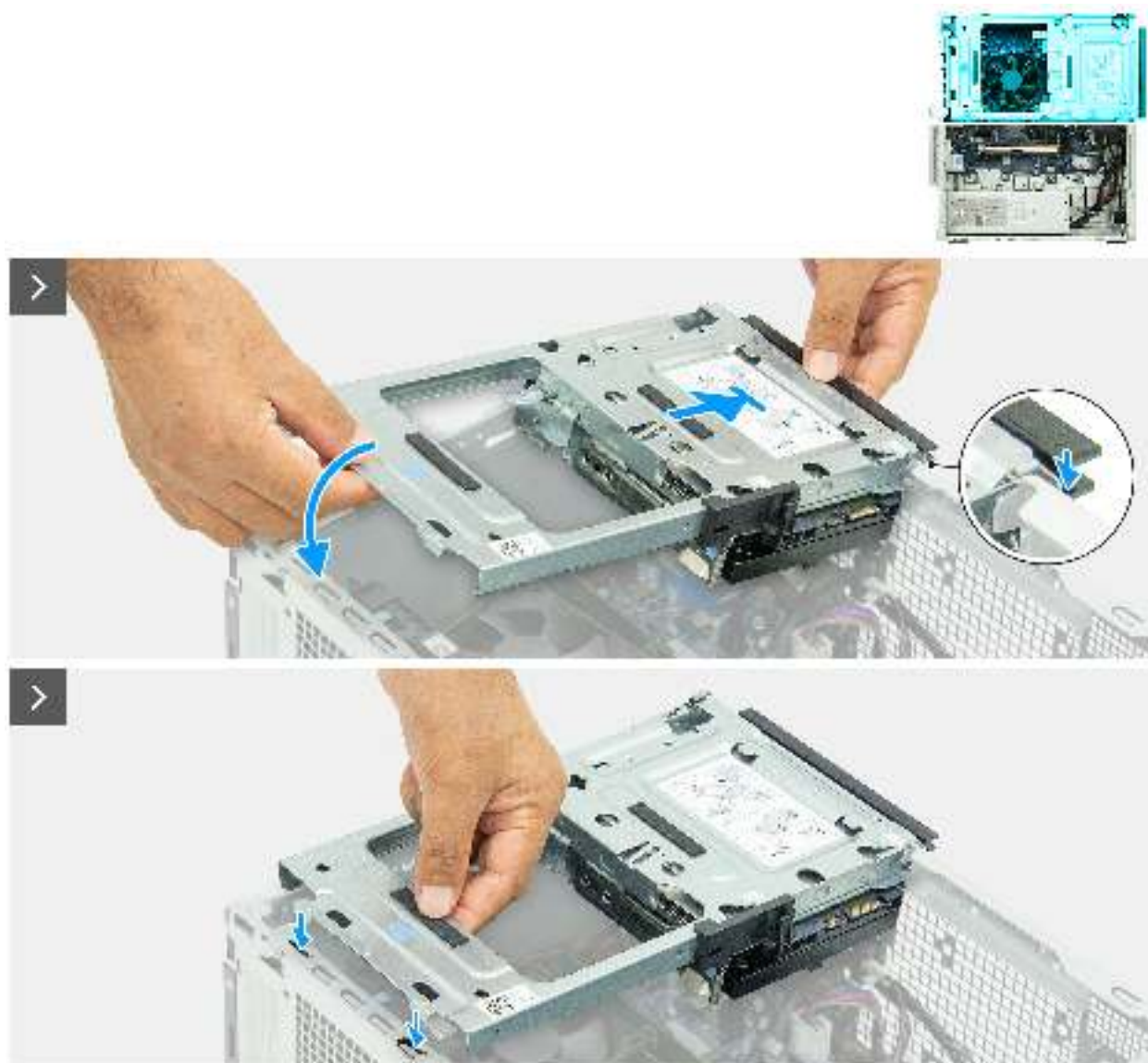
Abbildung 59. Installieren des Laufwerksschachts
