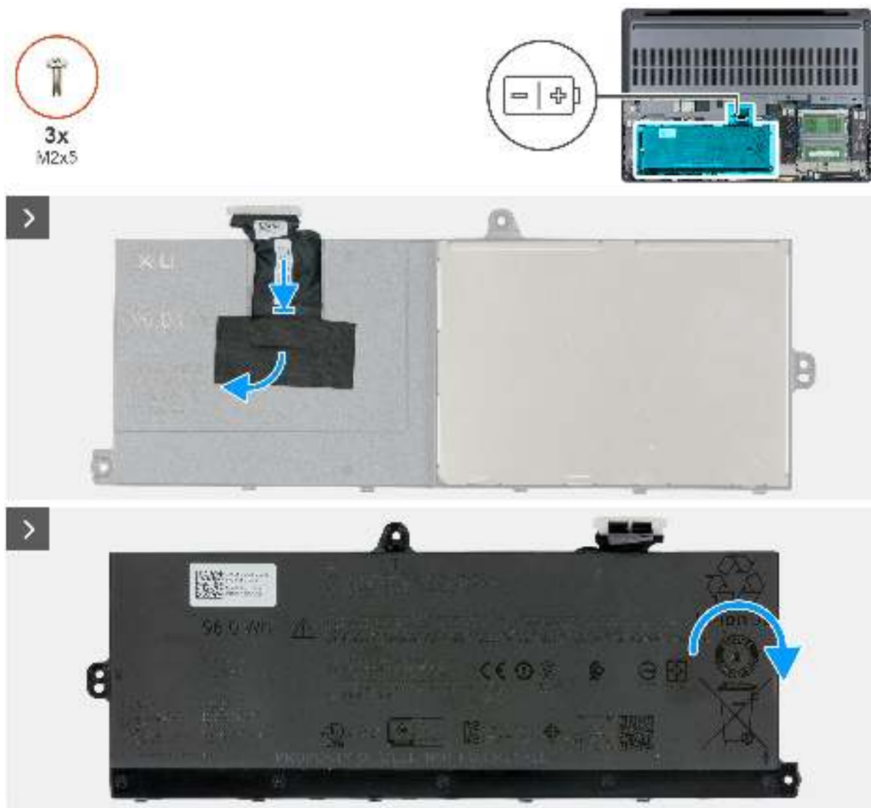
Abbildung 46. Austauschen des Akkukabels
