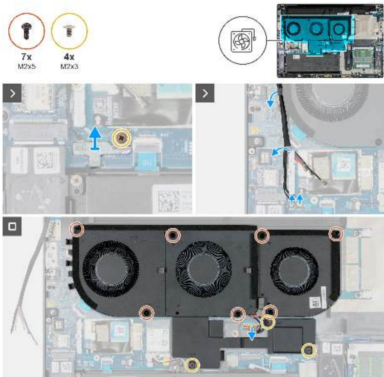
Abbildung 61. Entfernen der Lüfterbaugruppe
