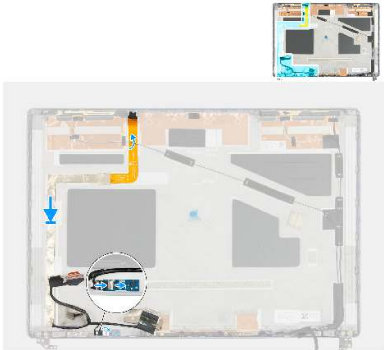
Abbildung 105. Einbauen des Bildschirmkabels
