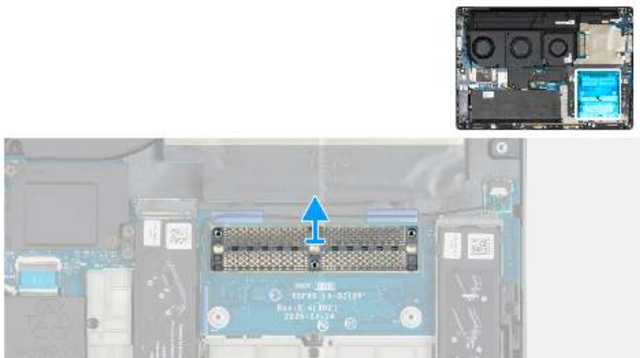
Abbildung 69. Entfernen des Speicheranschlusses
