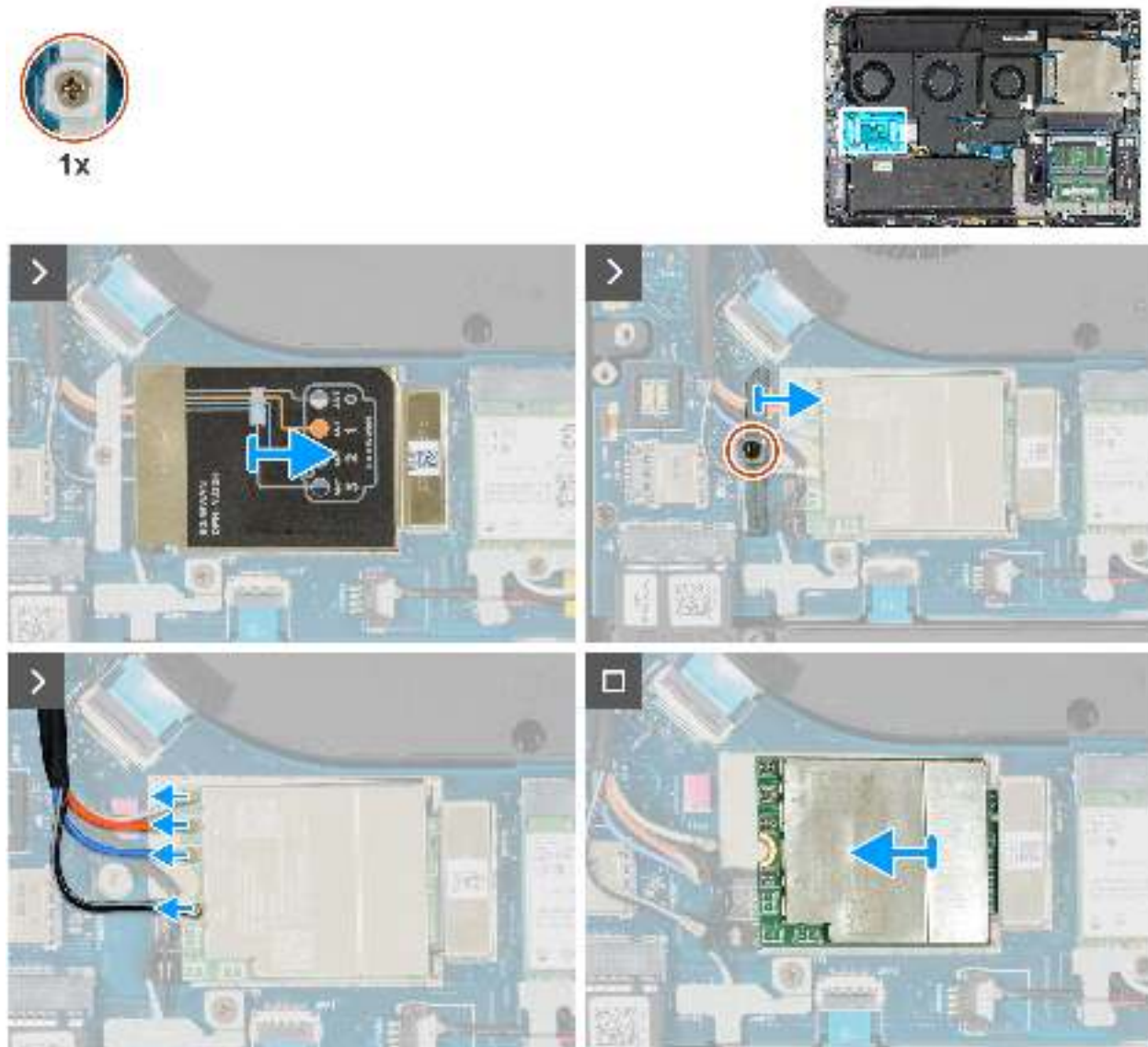
Abbildung 52. Entfernen der WWAN-Karte
