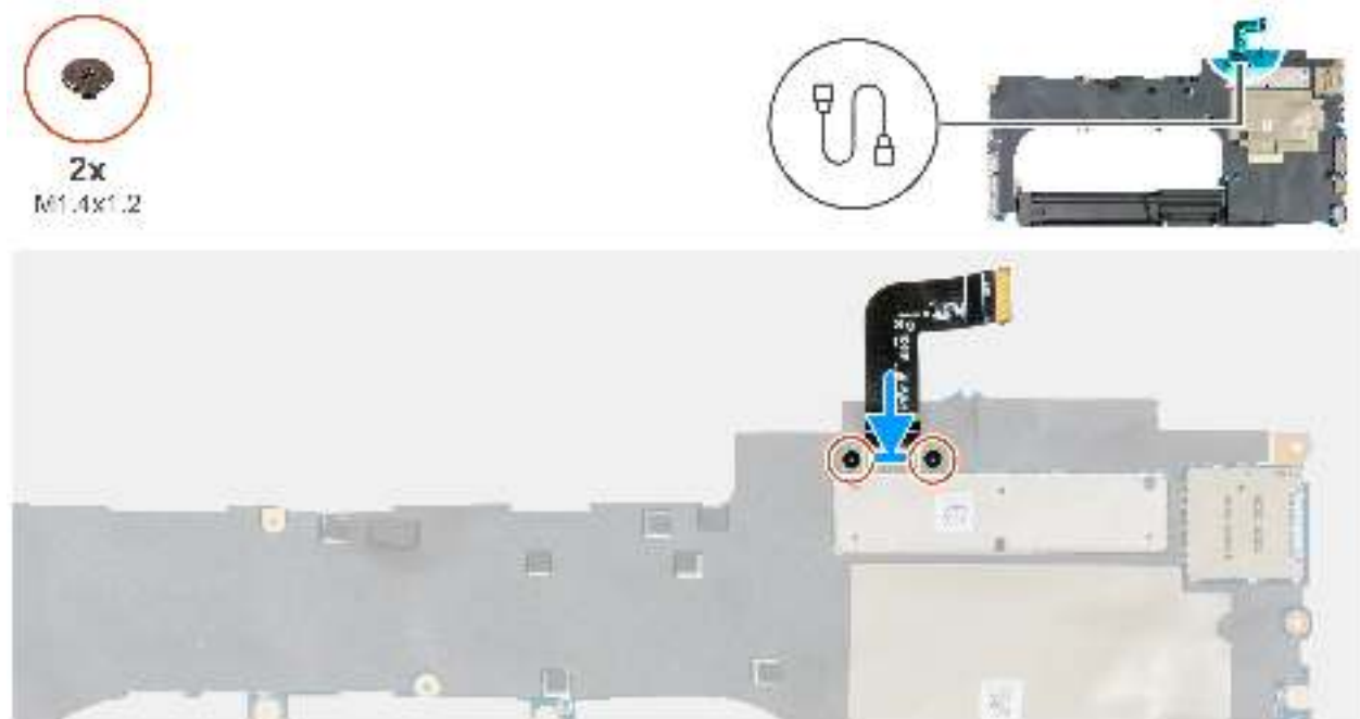
Abbildung 118. Einbauen des USh-Platinenkabels
