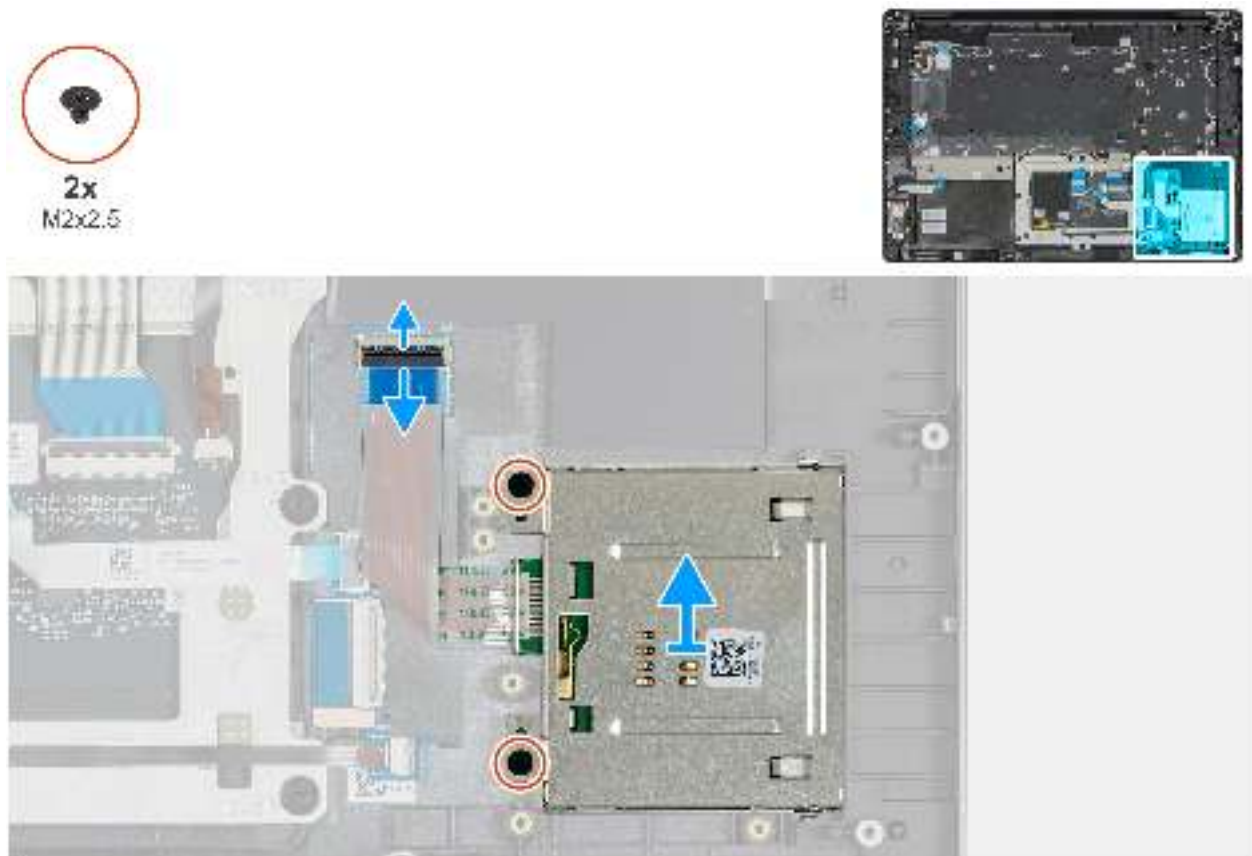
Abbildung 123. Entfernen des Smartcardlesegeräts
