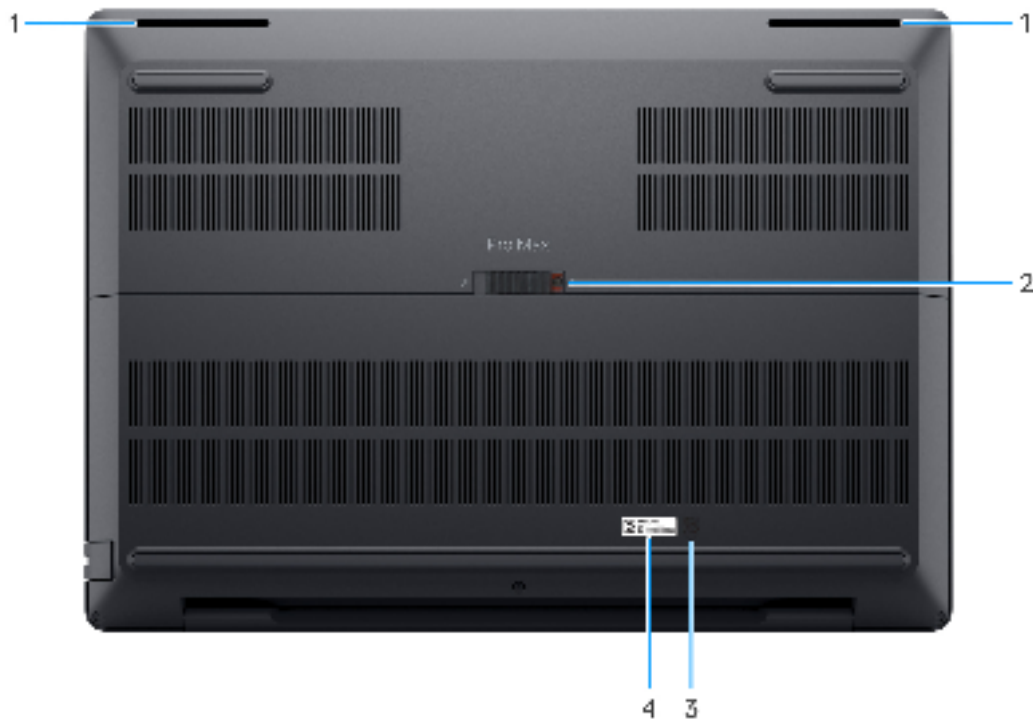
Abbildung 5. Untere Ansicht
