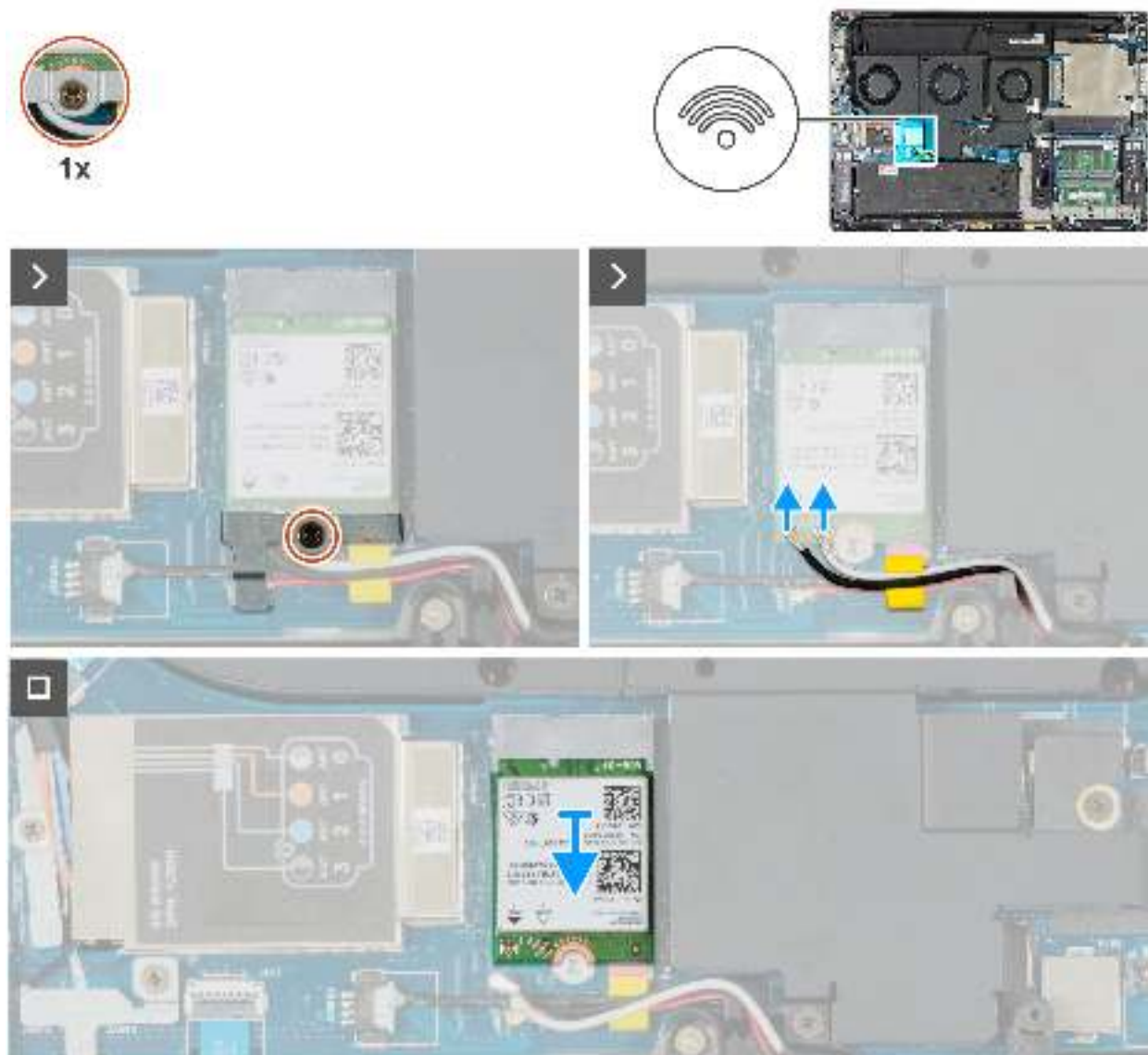
Abbildung 48. Entfernen der WLAN-Karte
