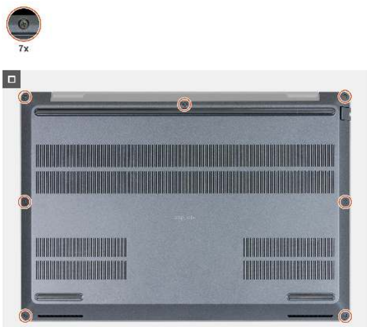
Abbildung 29. Festziehen der unverlierbaren Schrauben
