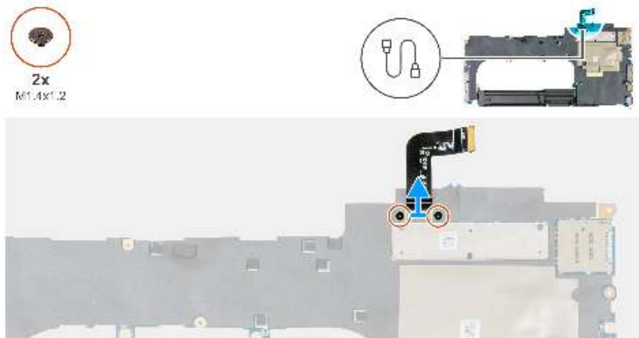
Abbildung 117. Entfernen des USH-Platinkabels
