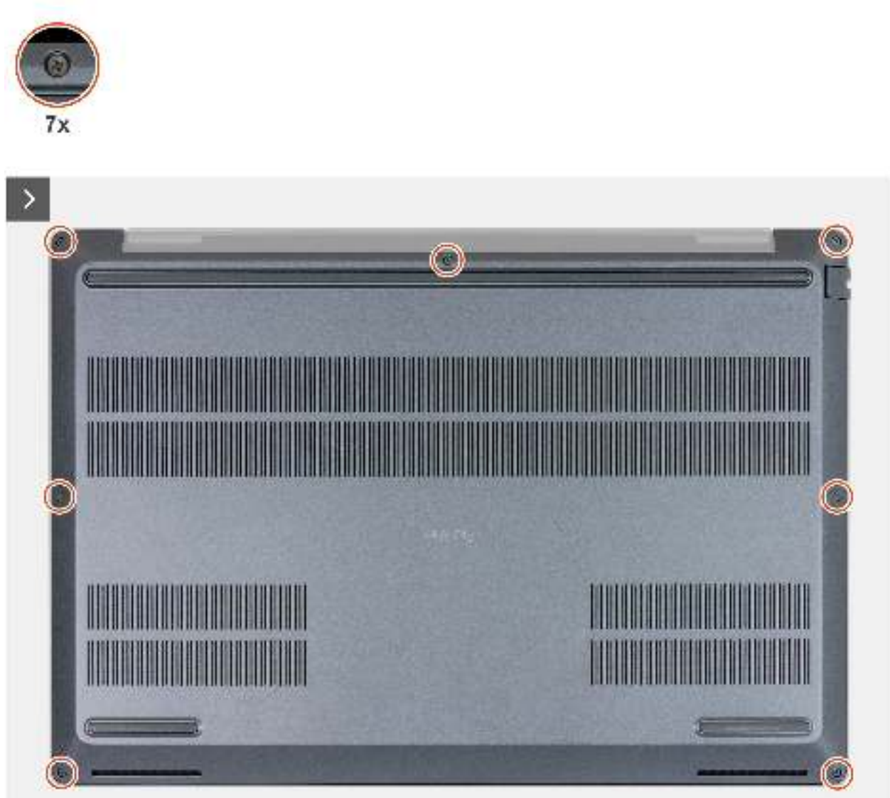
Abbildung 24. Lösen der unverlierbaren Schrauben
