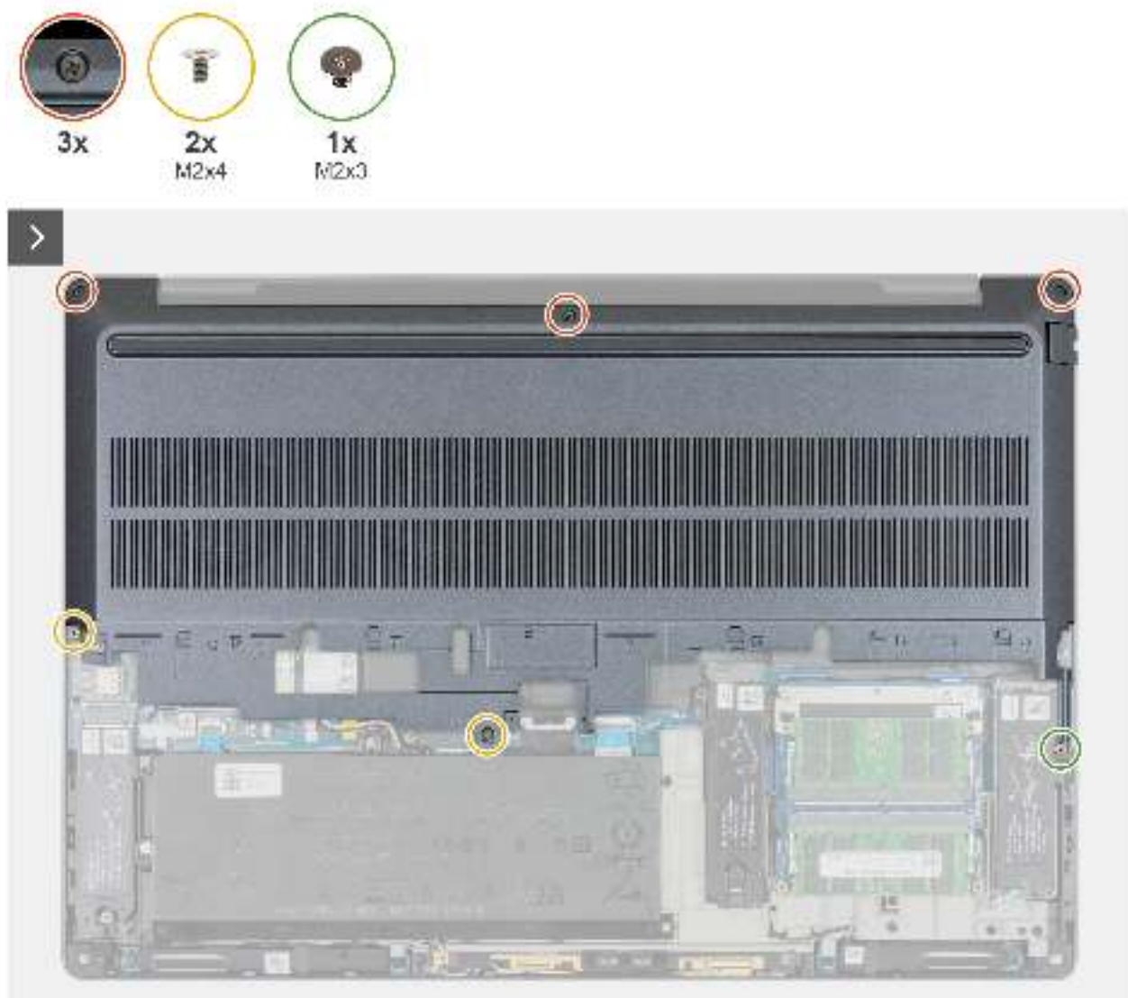
Abbildung 18. Lösen der drei unverlierbaren Schrauben und Entfernen der drei Schrauben
