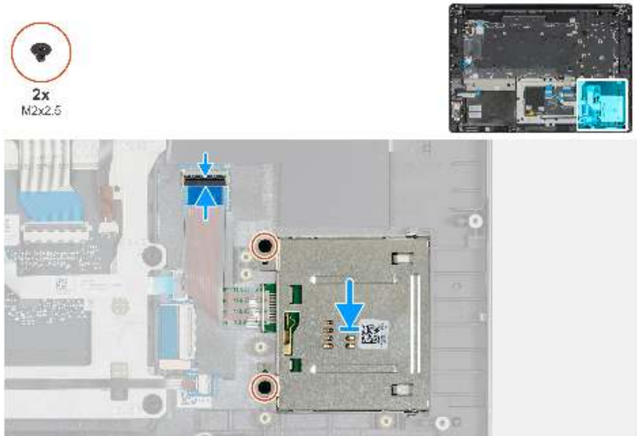
Abbildung 124. Installieren des Smartcardlesegeräts
