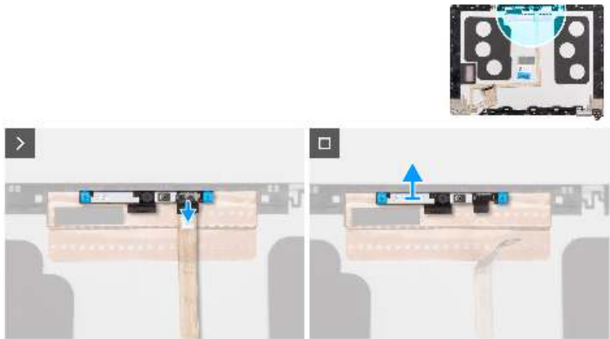
Abbildung 78. Entfernen des Kameramoduls
