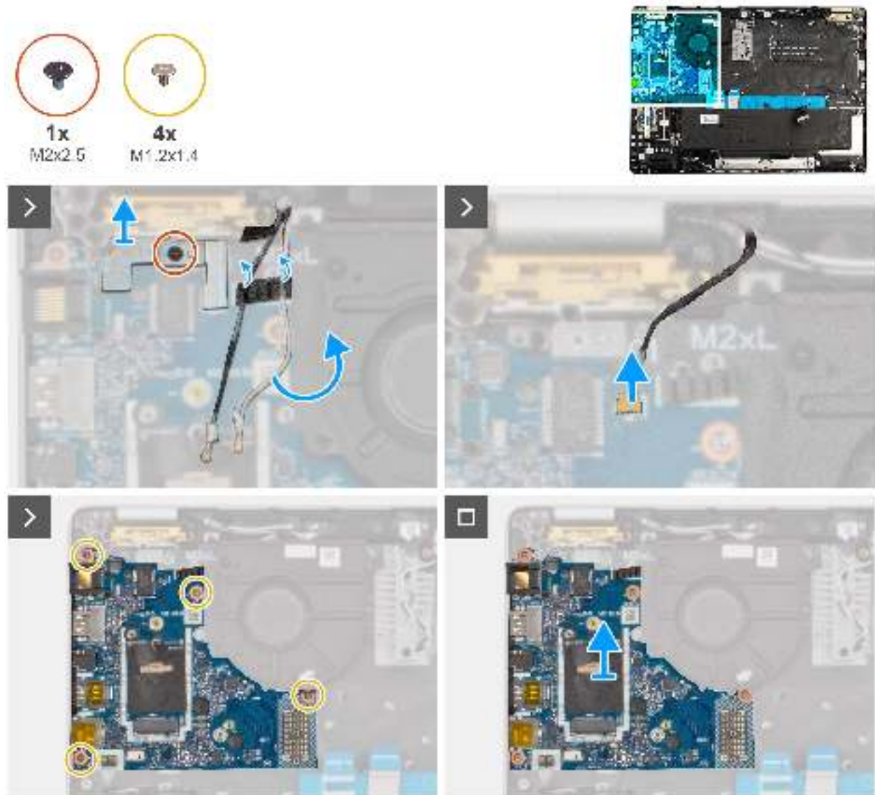
Abbildung 57. Entfernen der I/O-Platine
