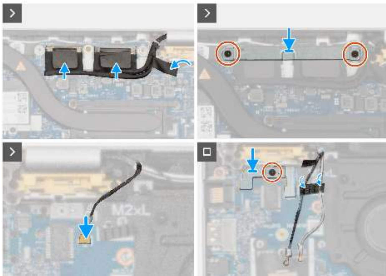
Abbildung 46. Installieren der WLAN-Antenne
