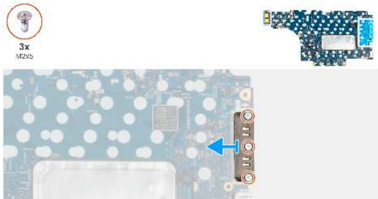
Abbildung 82. Entfernen des USB Type-C-Anschlussmoduls
