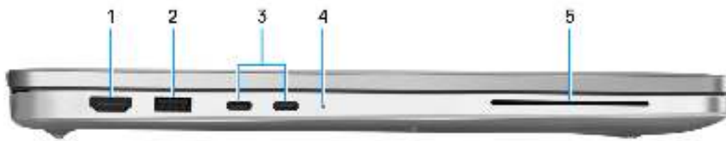
Abbildung 2. Linke Seitenansicht
