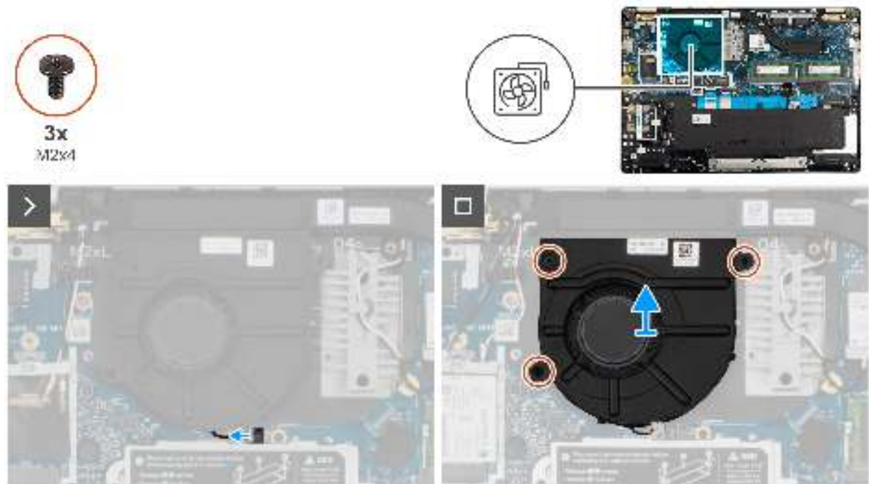
Abbildung 37. Entfernen des Lüfters
