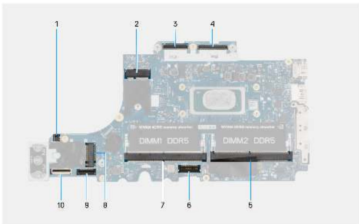
Abbildung 54. Hauptplattenanschluss
