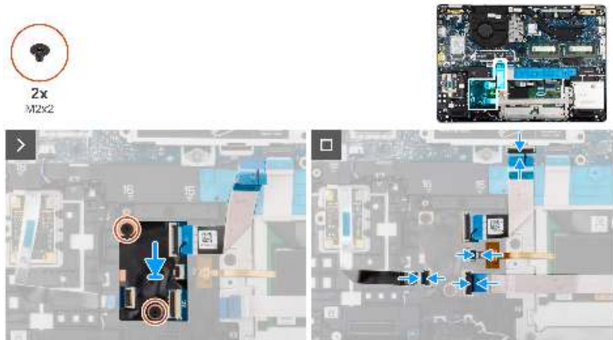
Abbildung 49. USH-Platine
