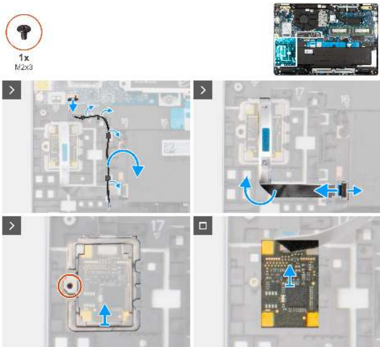
Abbildung 41. Entfernen des optionalen Fingerabdruck-Lesegeräts
