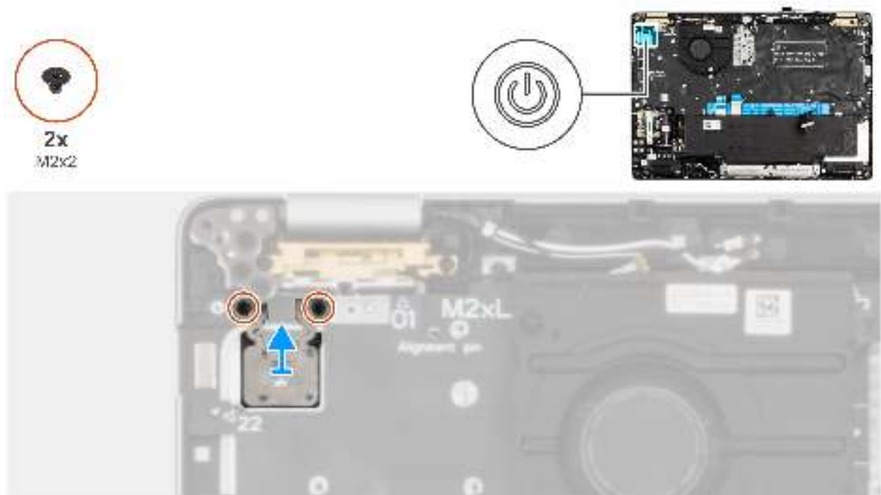
Abbildung 59. Installieren des Netzschalters mit optionalem Fingerabdruck-Lesegerät
