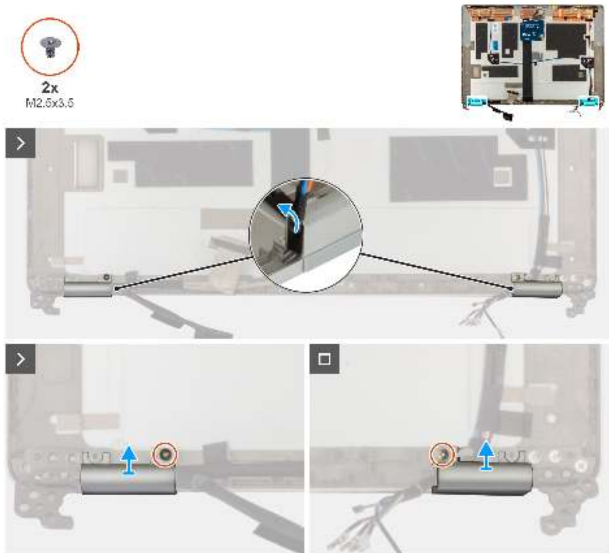
Abbildung 74. Entfernen der Bildschirmscharnierabdeckung
