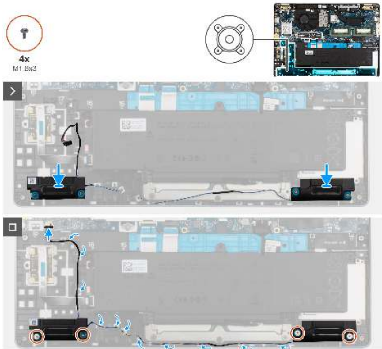
Abbildung 39. Installieren der Lautsprecher
