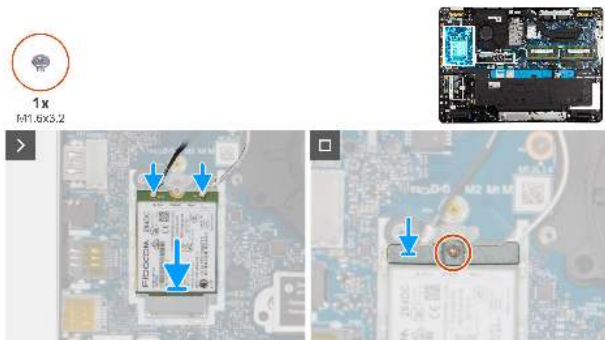
Abbildung 34. Installieren der 4G-WWAN-Karte
