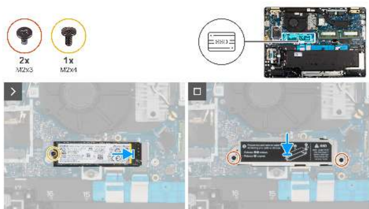
Abbildung 28. Einbauen der M.2230-SSD
