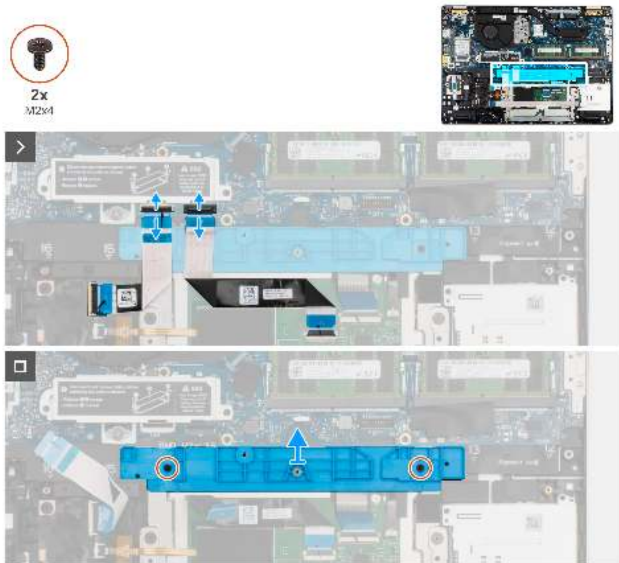
Abbildung 47. Entfernen der Akkuhalterung
