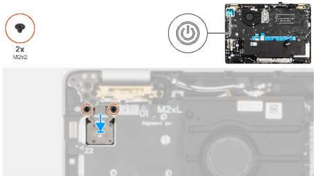
Abbildung 60. Installieren des Netzschalters mit optionalem Fingerabdruck-Lesegerät
