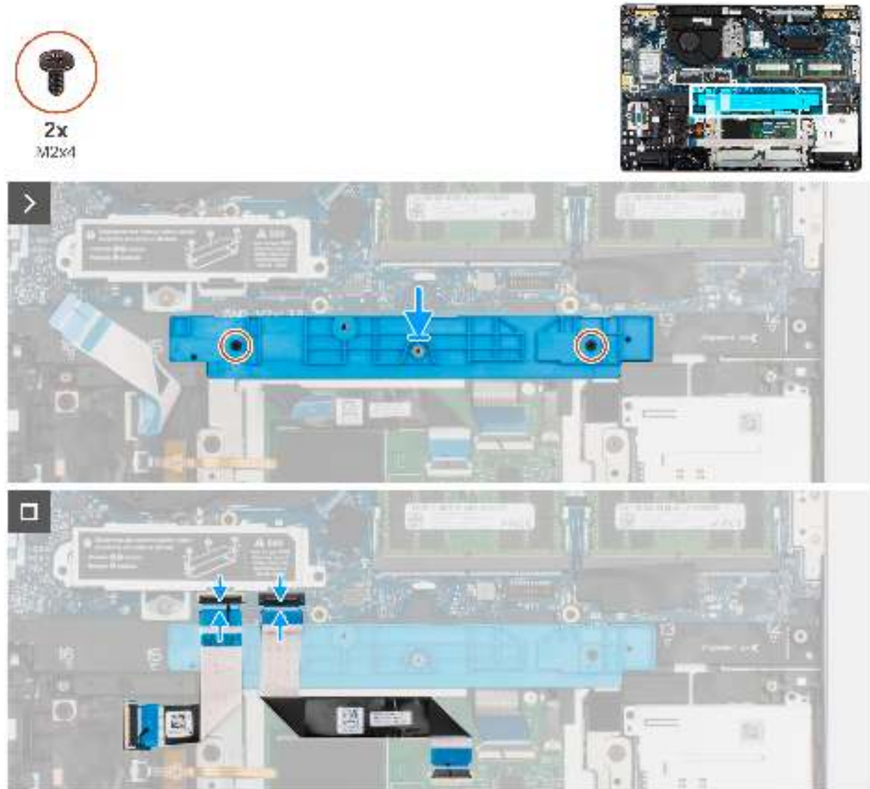
Abbildung 48. Installieren der Akkuhalterung
