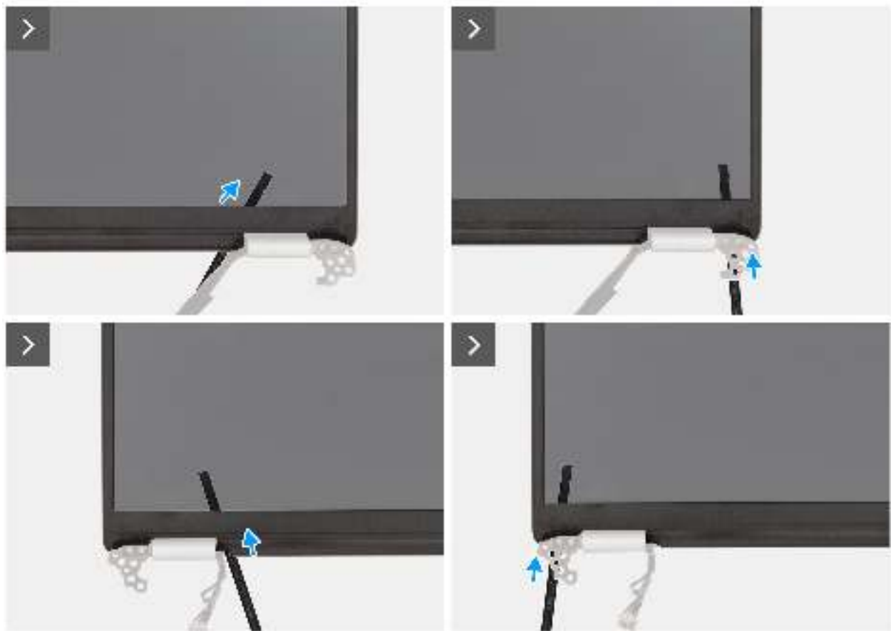
Abbildung 66. Entfernen der Bildschirmblende
