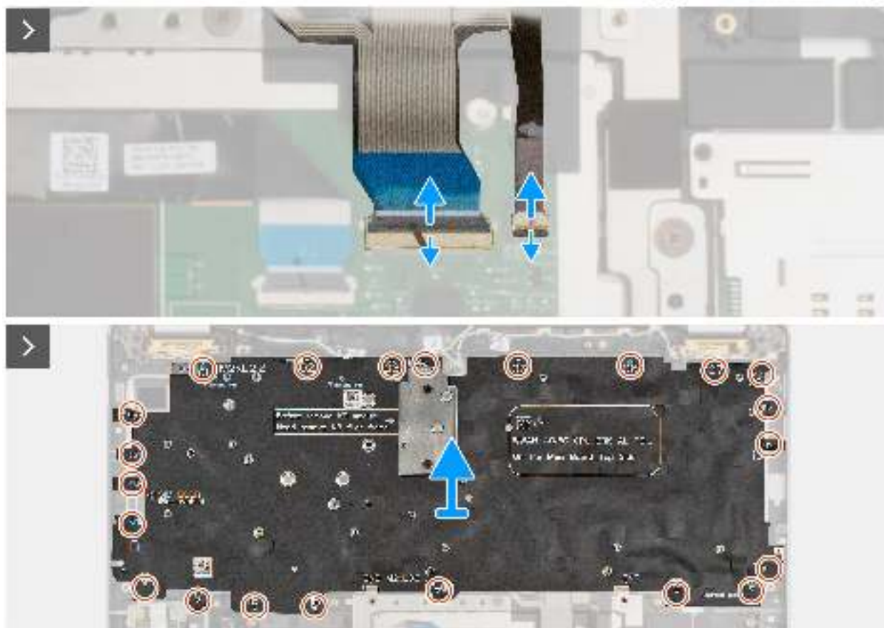
Abbildung 84. Entfernen der Tastatur
