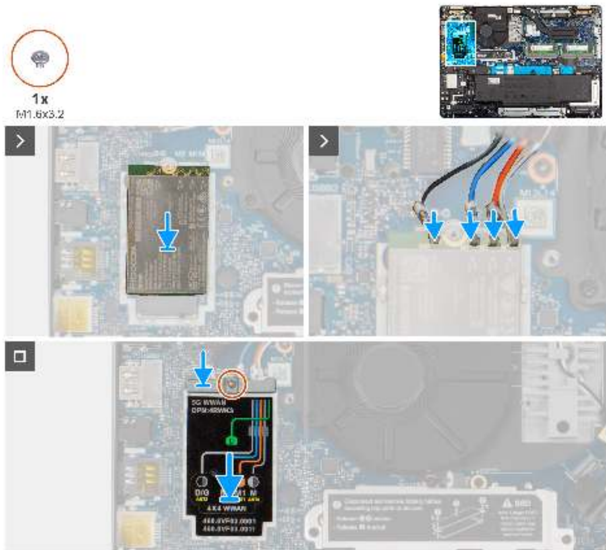
Abbildung 32. Installieren der 5G-WWAN-Karte
