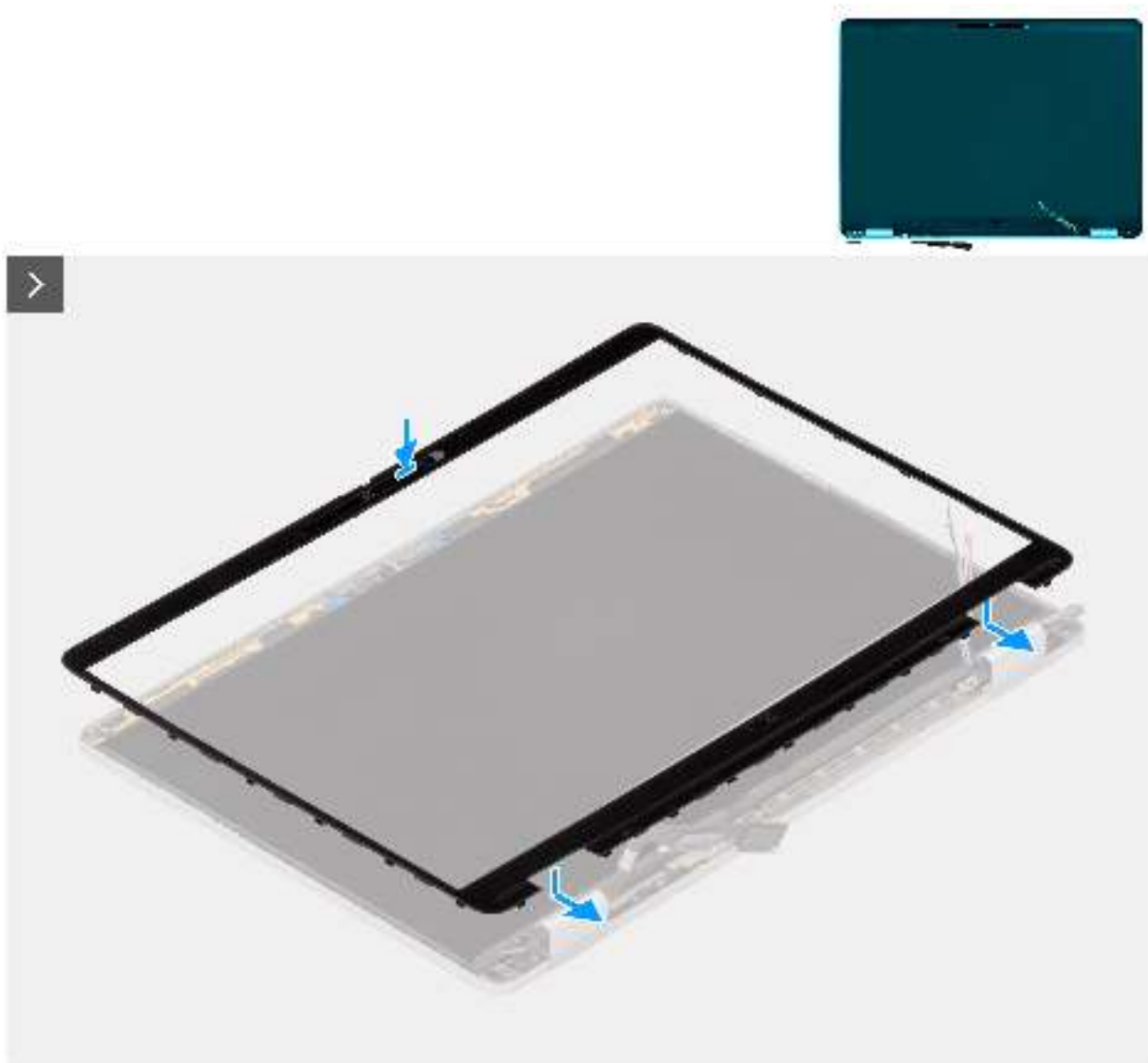
Abbildung 69. Einbauen der Bildschirmblende
