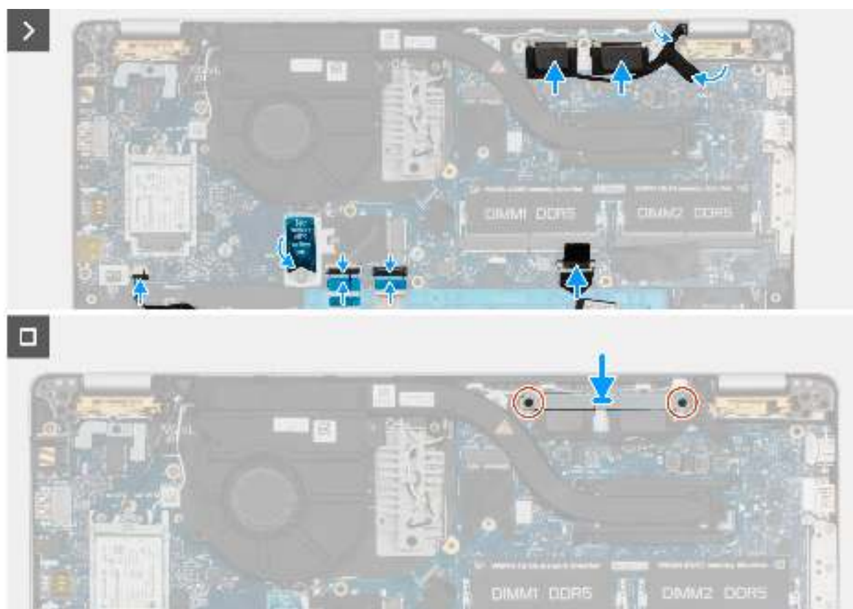
Abbildung 56. Einbauen der Systemplatine
