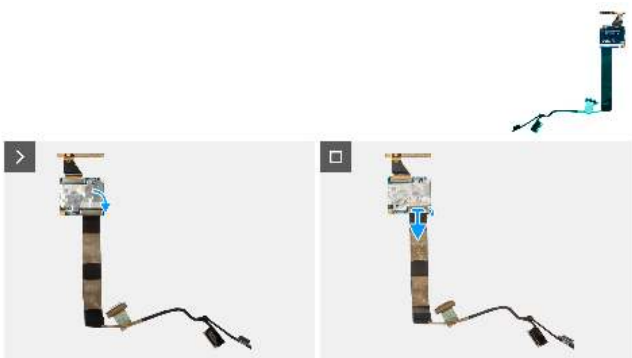
Abbildung 76. Entfernen des Bildschirmkabels
