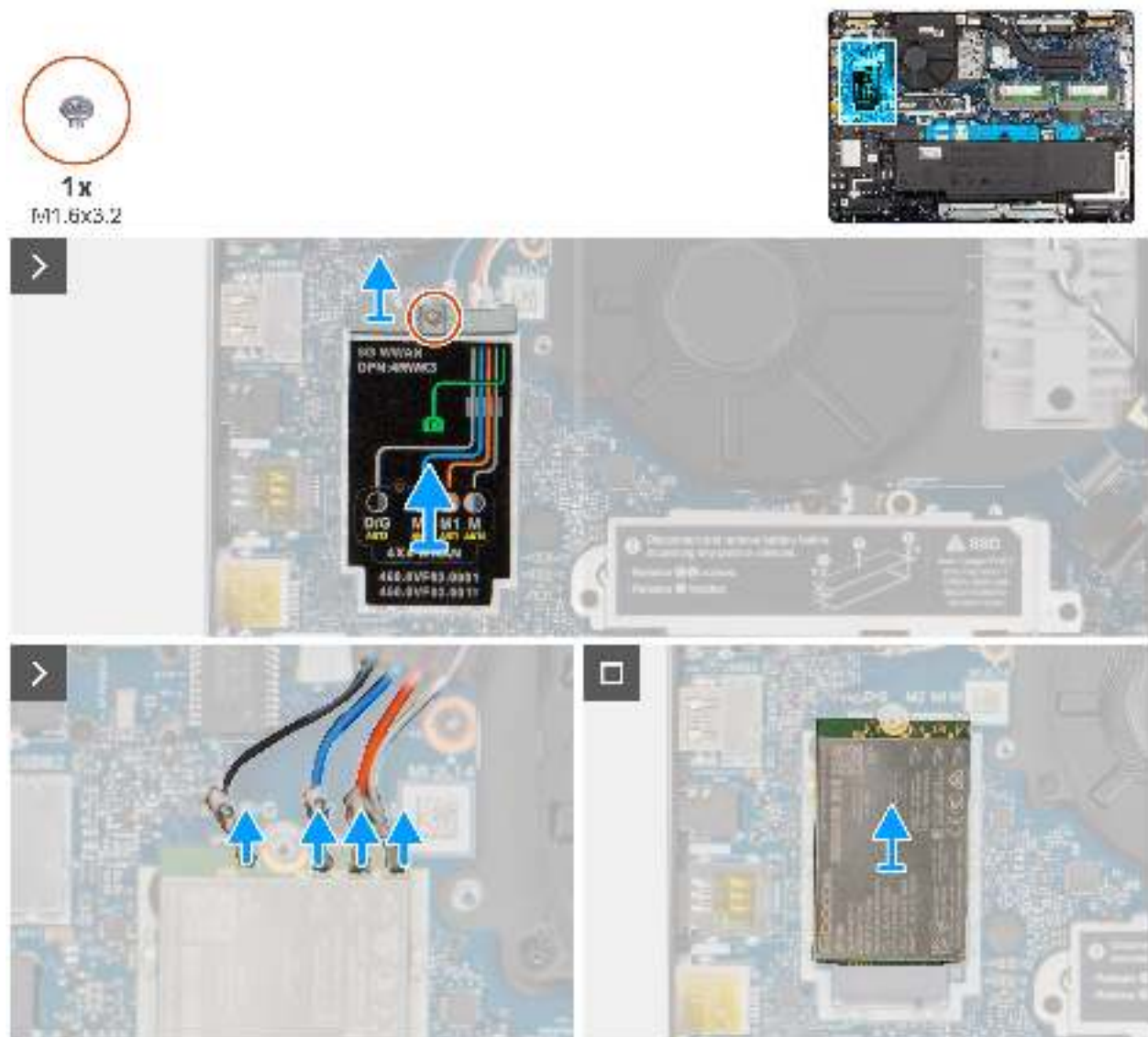
Abbildung 30. Entfernen der 5G-WWAN-Karte
