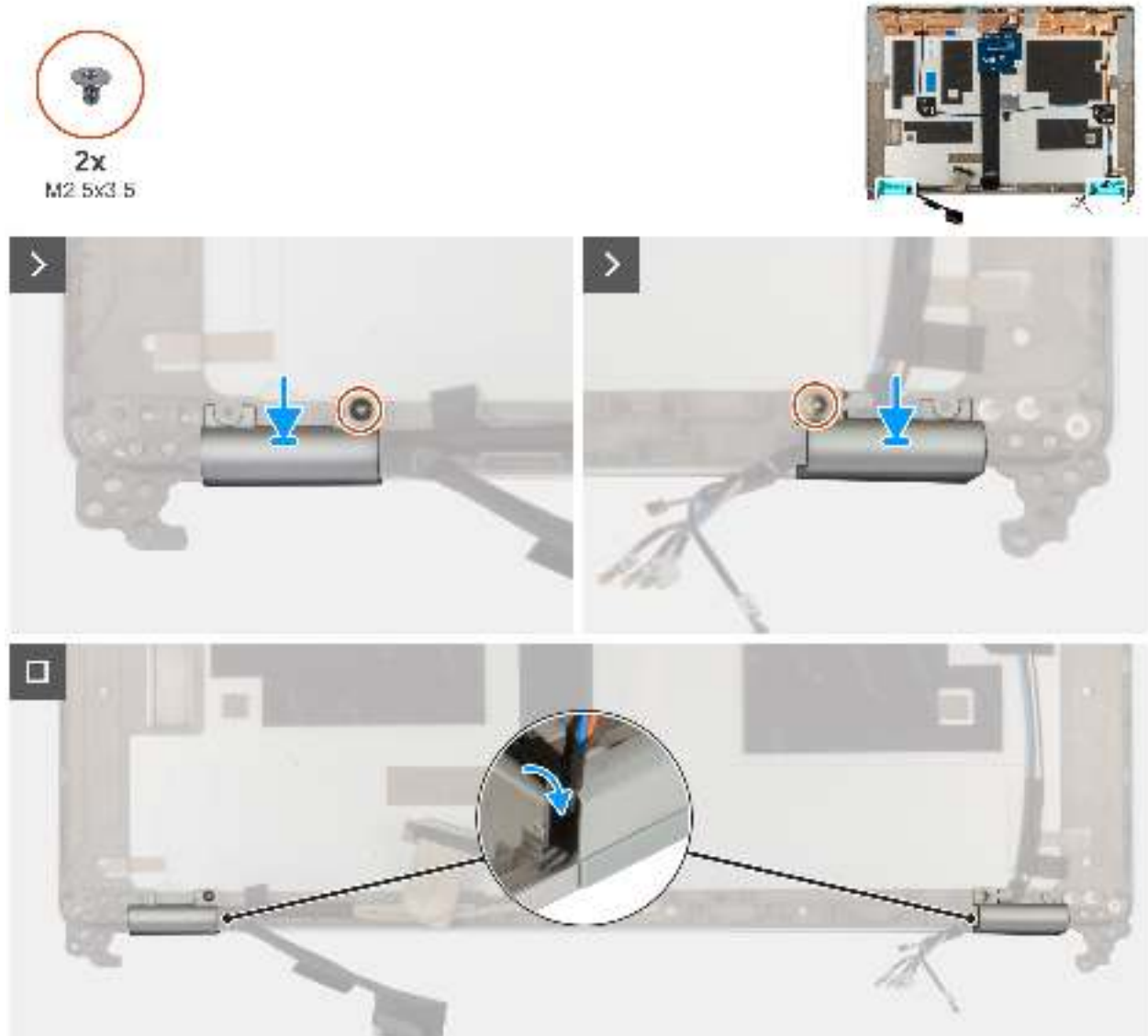
Abbildung 75. Einbauen der Bildschirmscharnierkappe
