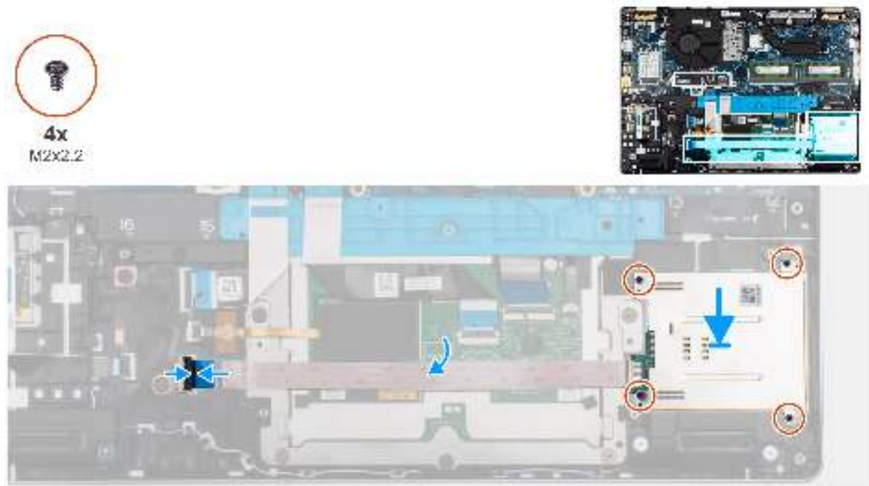
Abbildung 51. Einbauen des Smartcardlesegeräts
