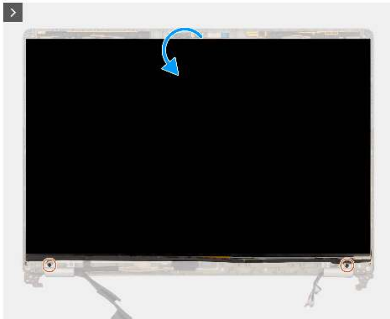
Abbildung 70. Entfernen des Bildschirms
