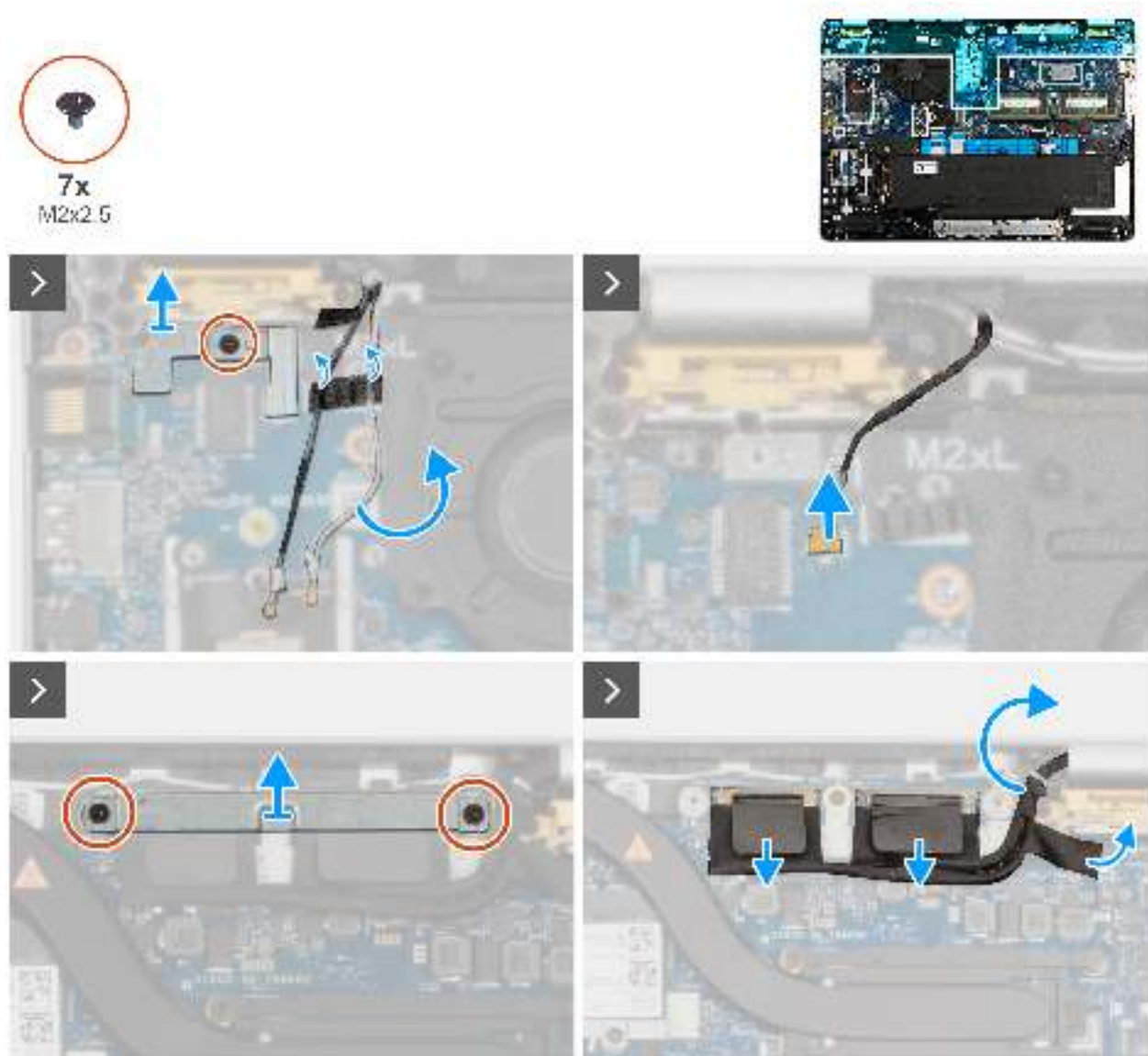
Abbildung 43. Entfernen der WLAN-Antenne
