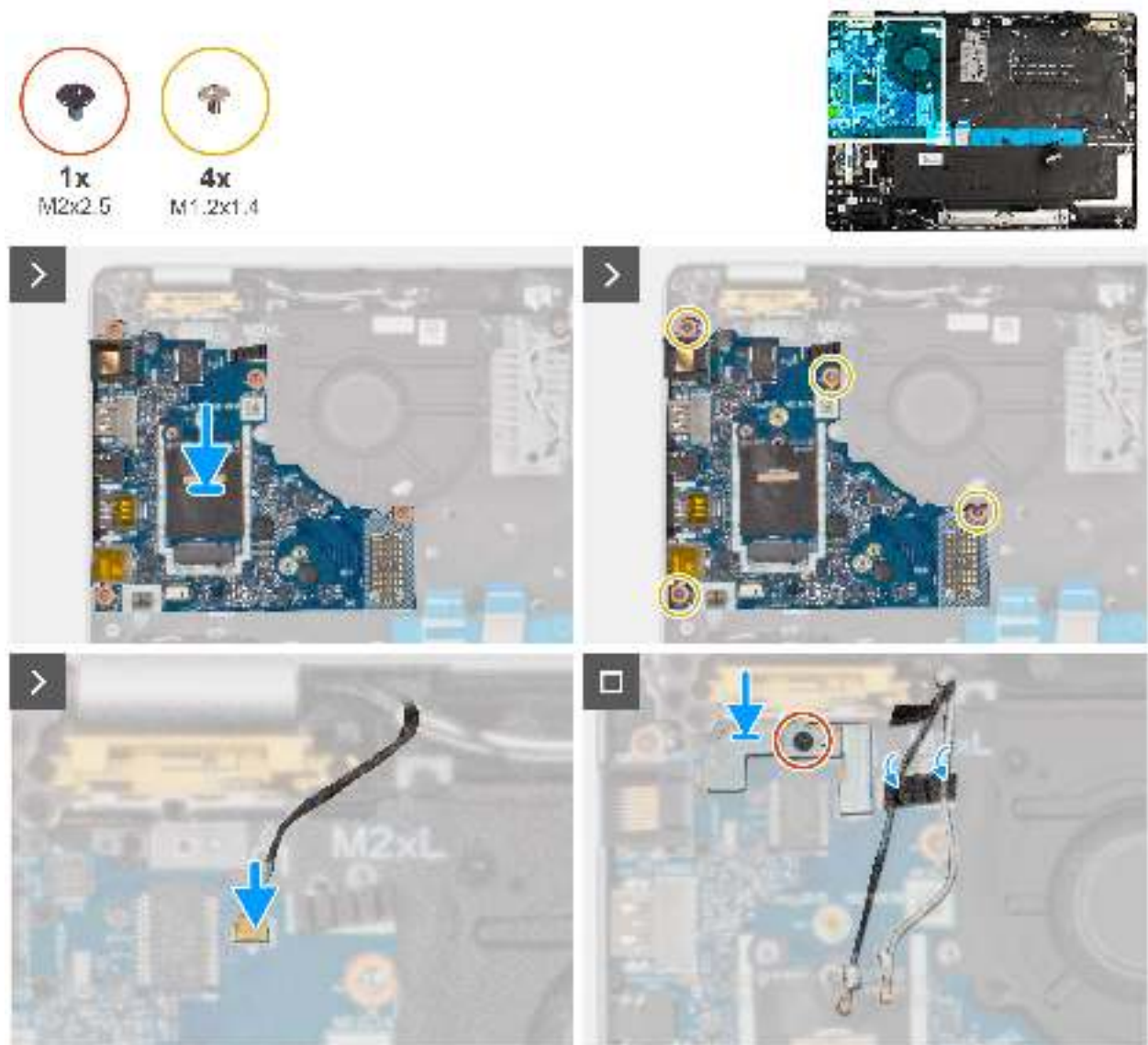
Abbildung 58. Entfernen der E/A-Platine
