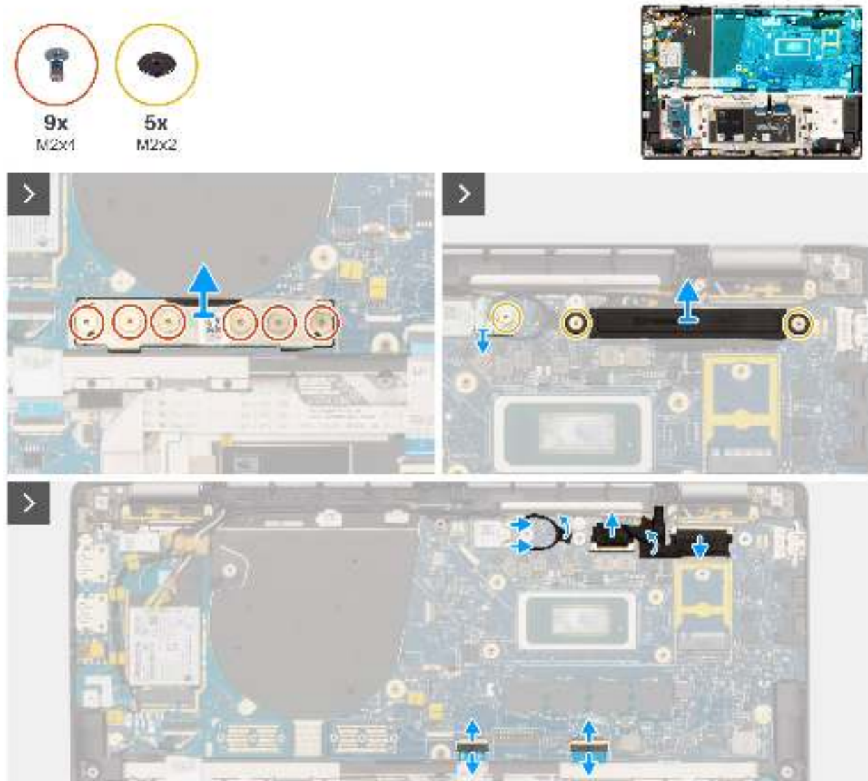
Abbildung 56. Entfernen der Systemplatine
