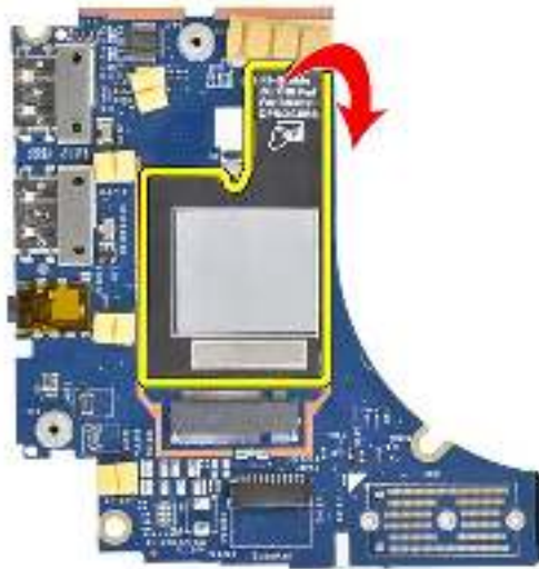
Abbildung 71. Latitude 7450 in der 5G-WWAN-Konfiguration (Wärmeleitpad-Aufkleber)
