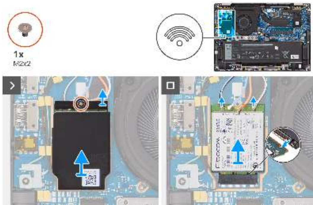
Abbildung 21. Entfernen der 4G-WWAN-Karte
