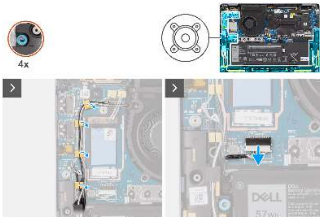
Abbildung 26. Entfernen der Lautsprecher (Ultralight)
