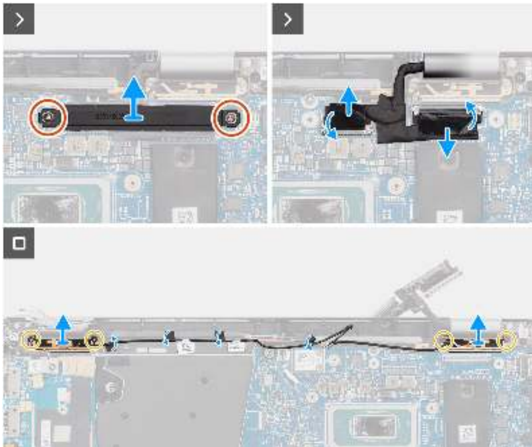
Abbildung 64. Entfernen des WLAN-Antennenmoduls
