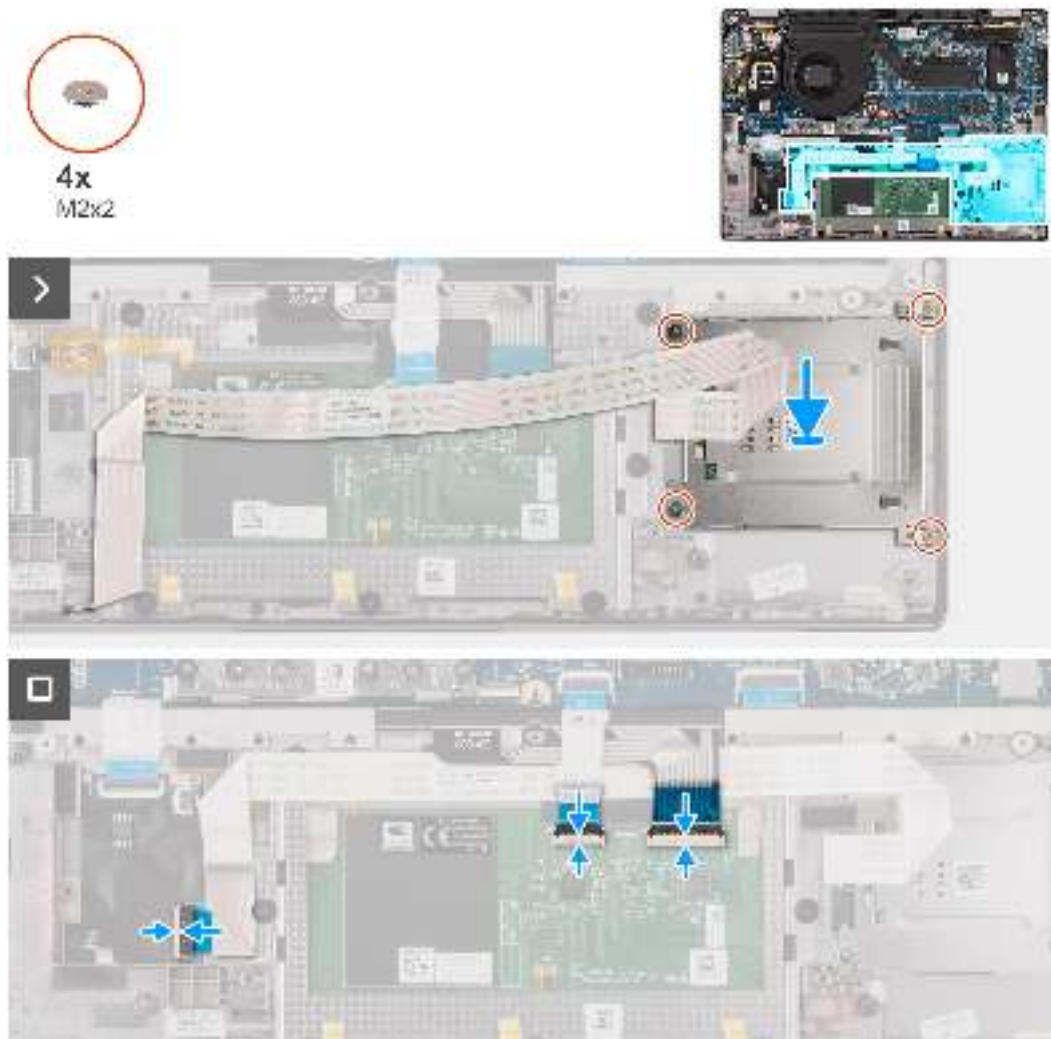
Abbildung 54. Installieren des Smartcardlesegeräts
