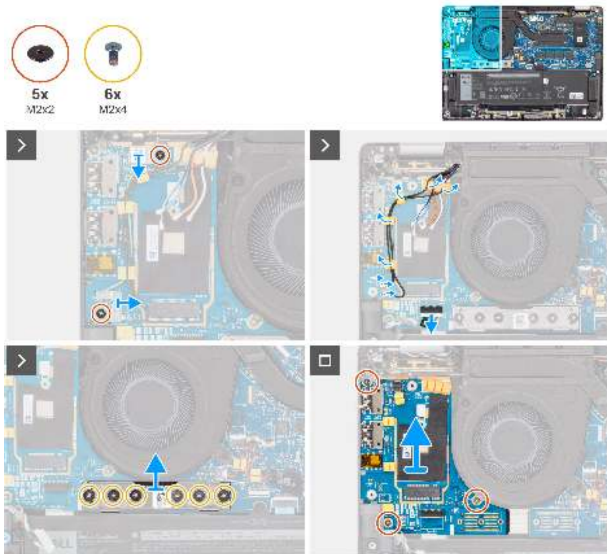
Abbildung 68. Entfernen der I/O-Zusatzplatine
