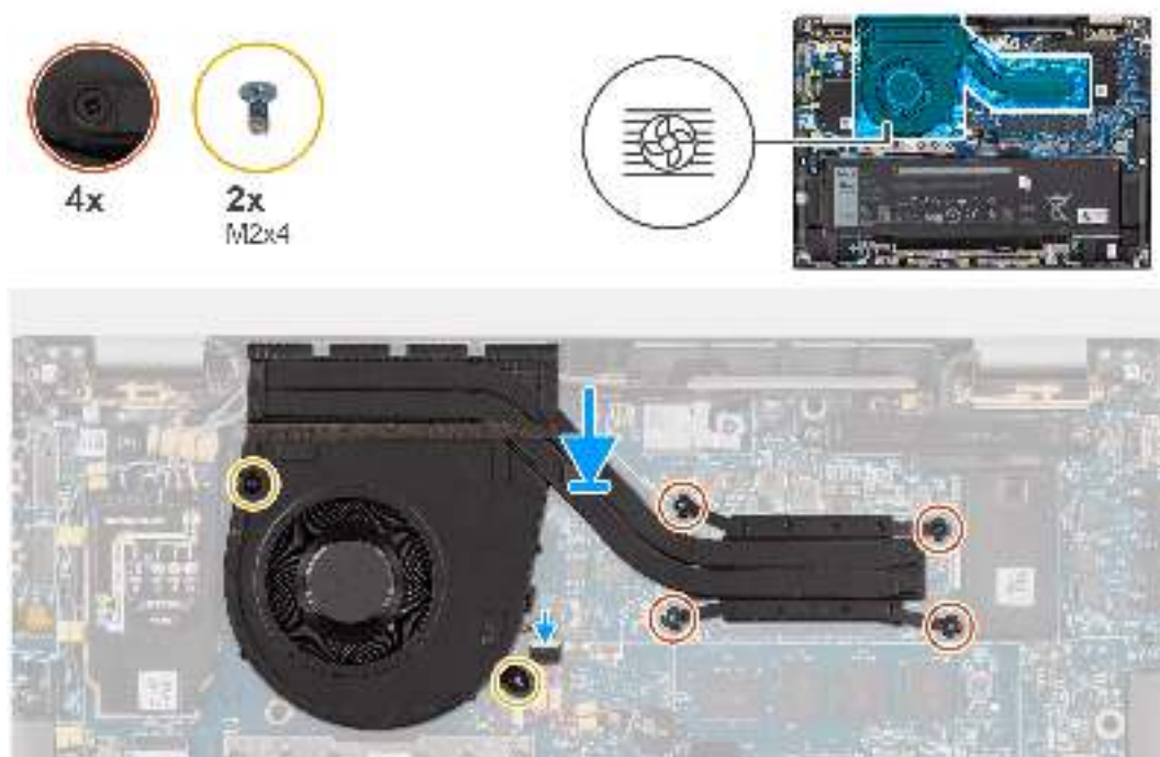
Abbildung 44. Installieren der Kühlkörper/Lüfter-Baugruppe
