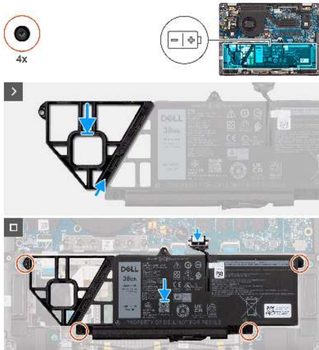
Abbildung 36. Installieren des 2-Zellen-Akkus
