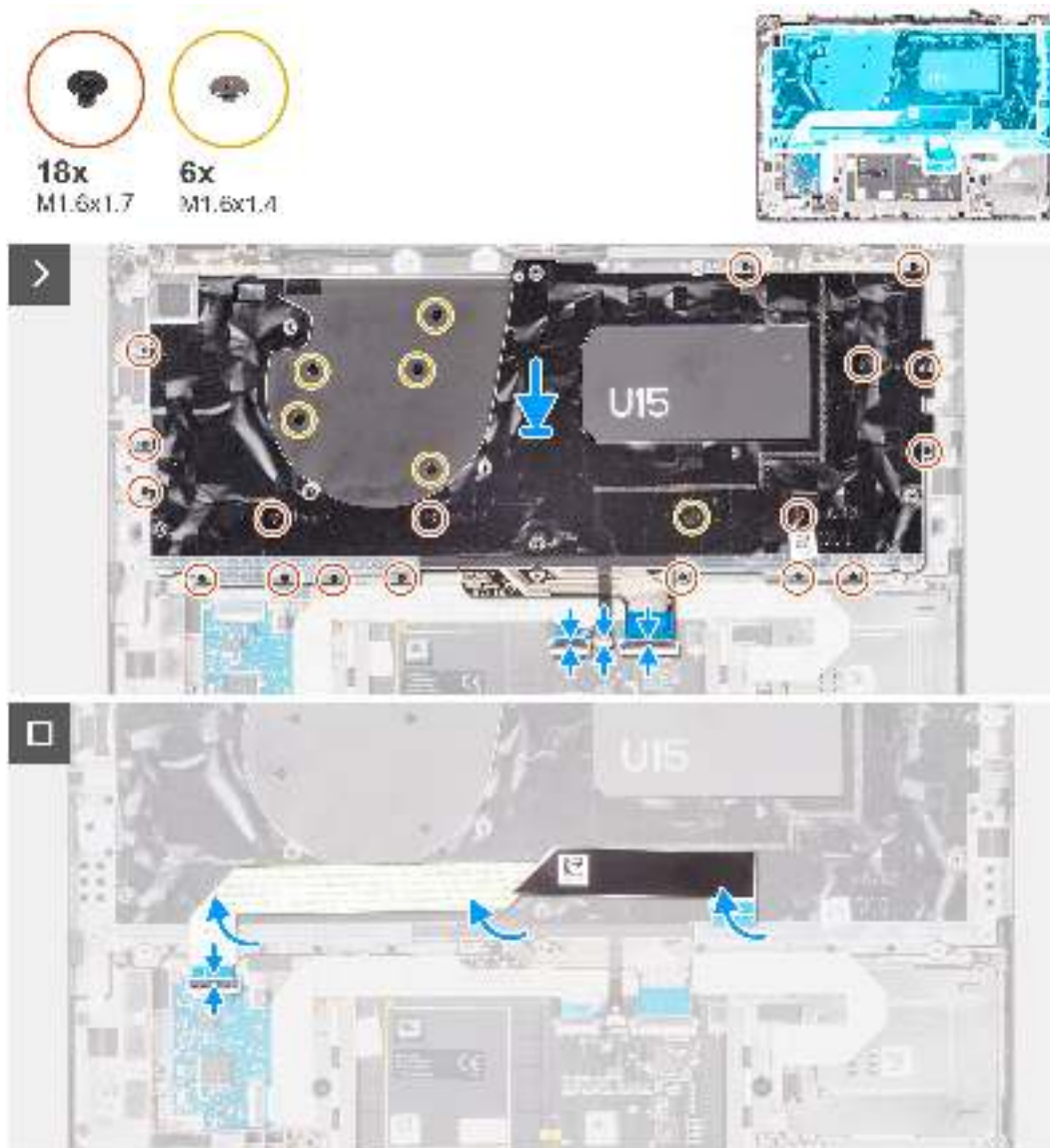
Abbildung 78. Installieren der Tastatur
