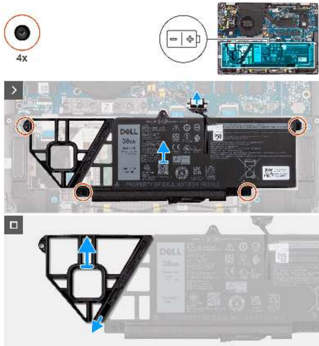
Abbildung 34. Entfernen des 2-Zellen-Akkus
