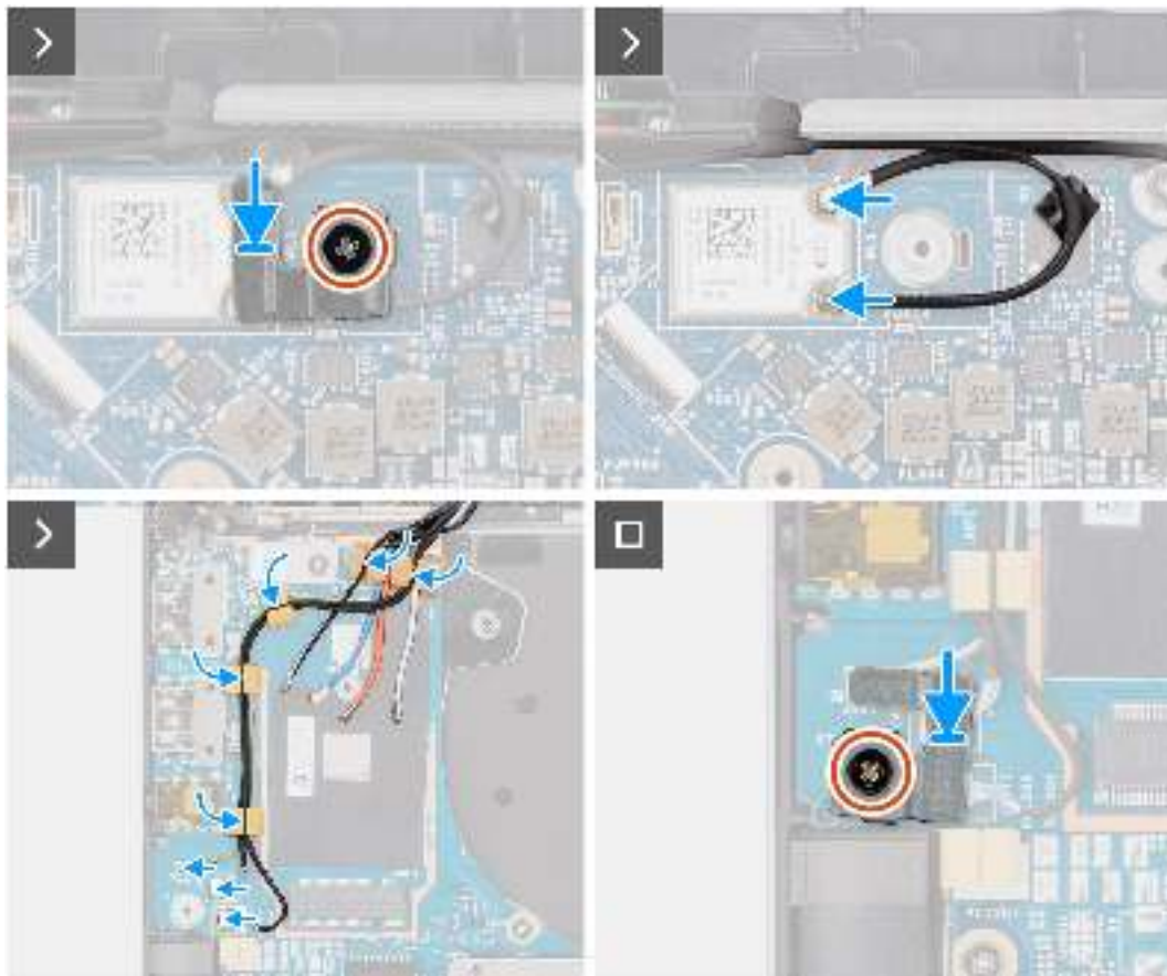
Abbildung 66. Installieren des WLAN-Antennenmoduls
