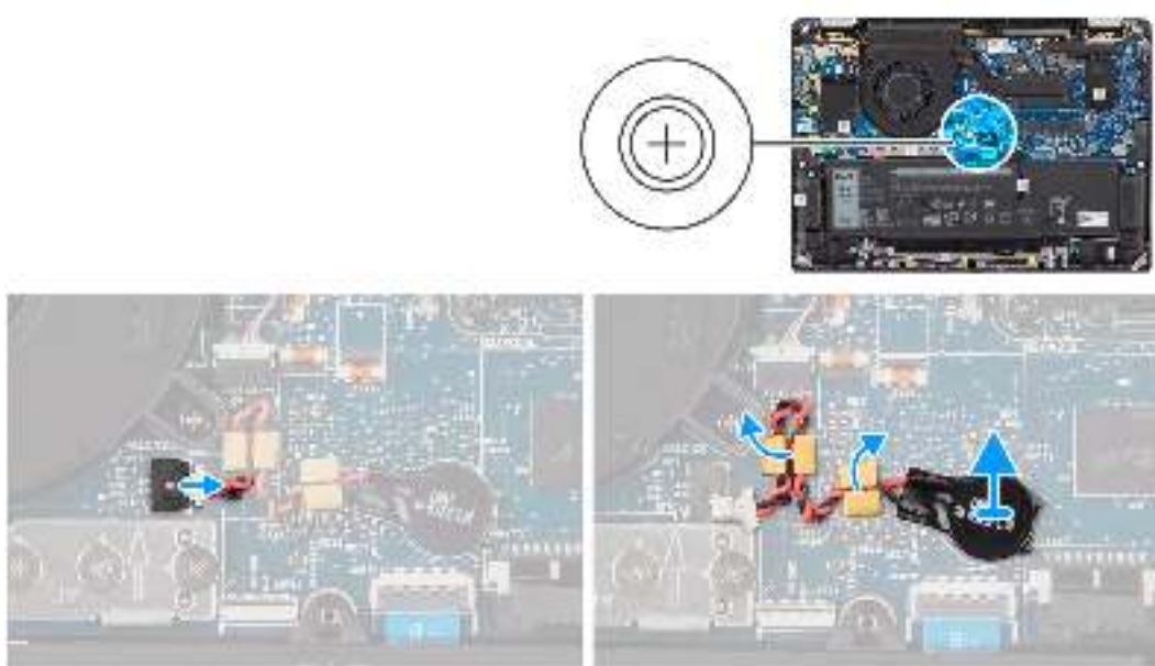
Abbildung 32. Entfernen der Knopfzellenbatterie
