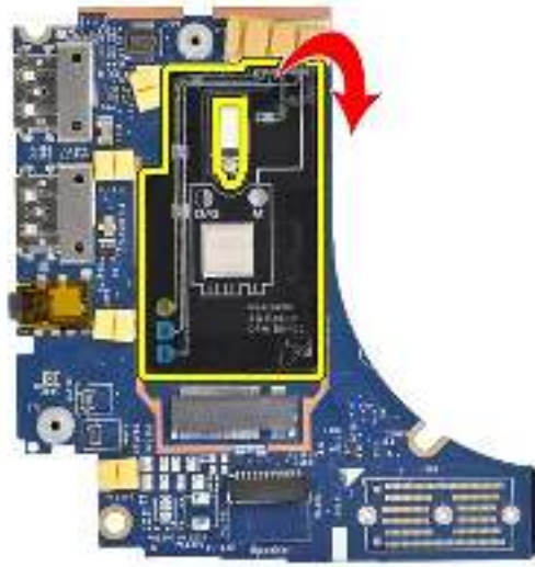
Abbildung 69. Latitude 7450 Clamshell in der 4G-WWAN-Konfiguration (Dichtungsaufkleber)
