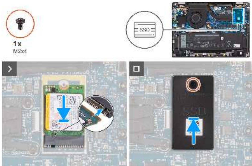
Abbildung 20. Installieren des M.2-2230-Solid-State-Laufwerks
