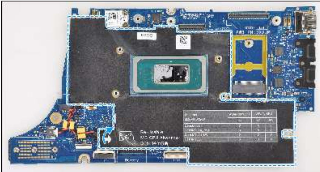
Abbildung 58. CPU-Absorber
