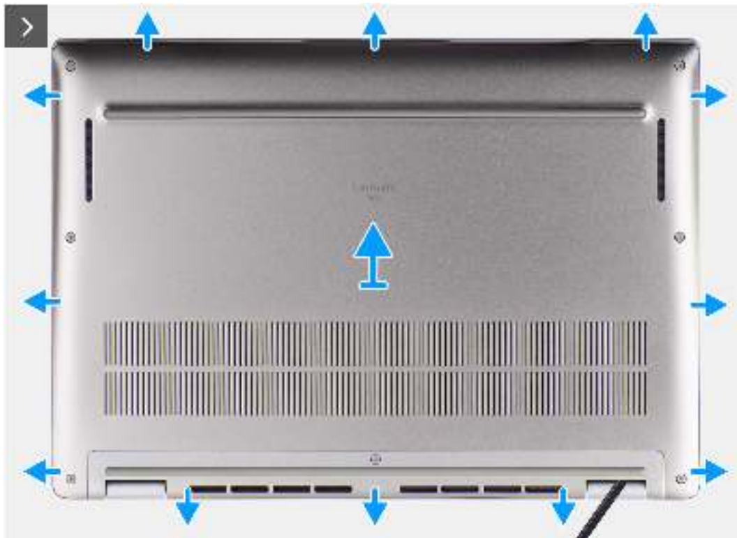
Abbildung 16. Entfernen der Bodenabdeckung
