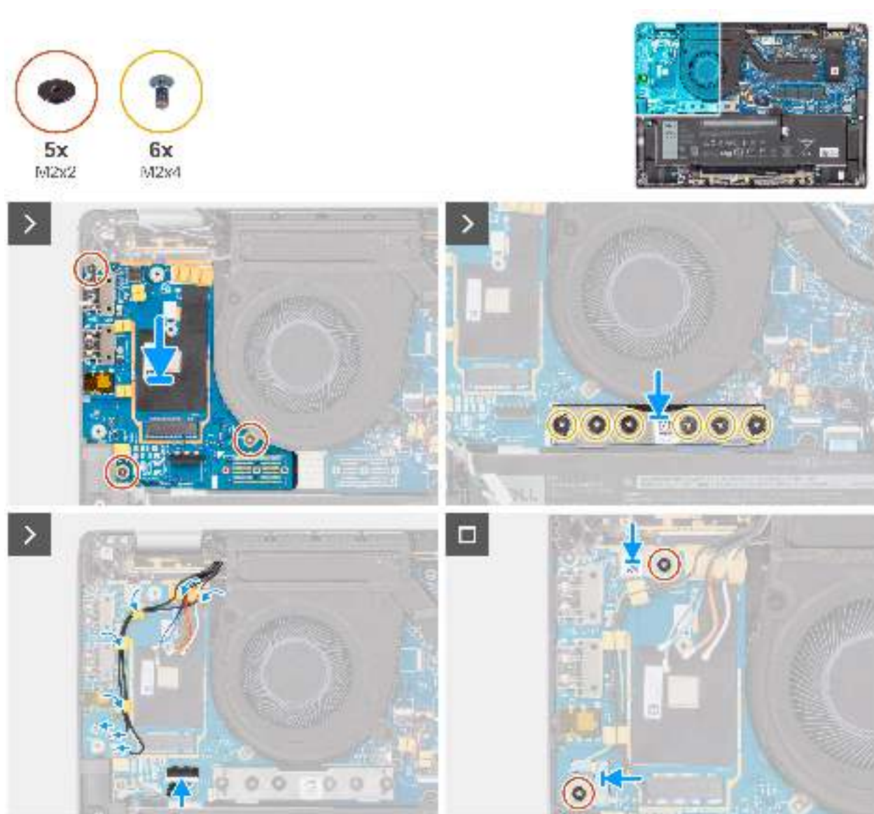
Abbildung 72. Installieren der I/O-Zusatzplatine
