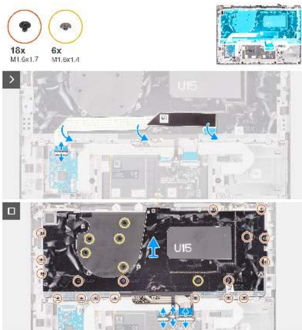
Abbildung 75. Entfernen der Tastatur
