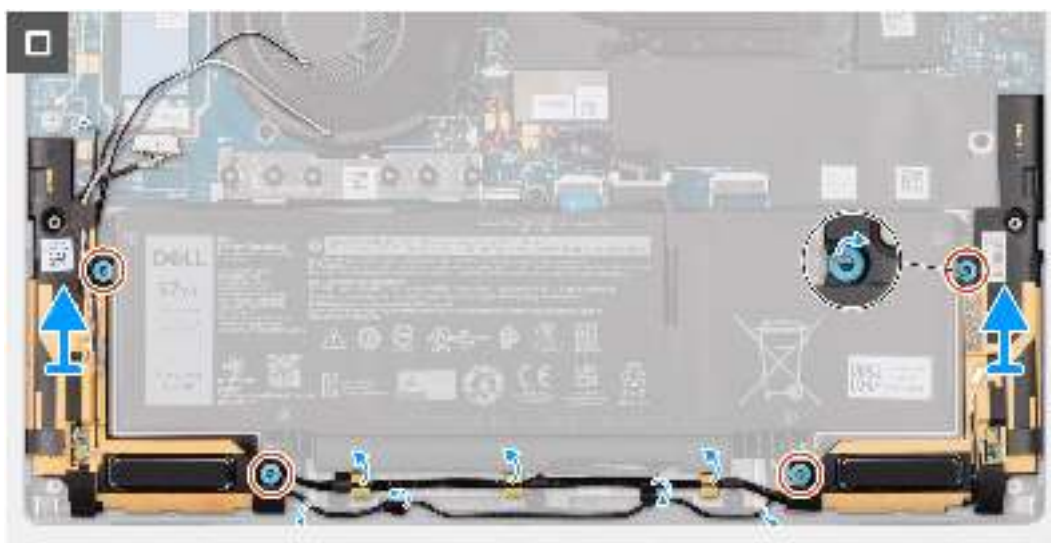
Abbildung 27. Entfernen der Lautsprecher (Ultralight)
