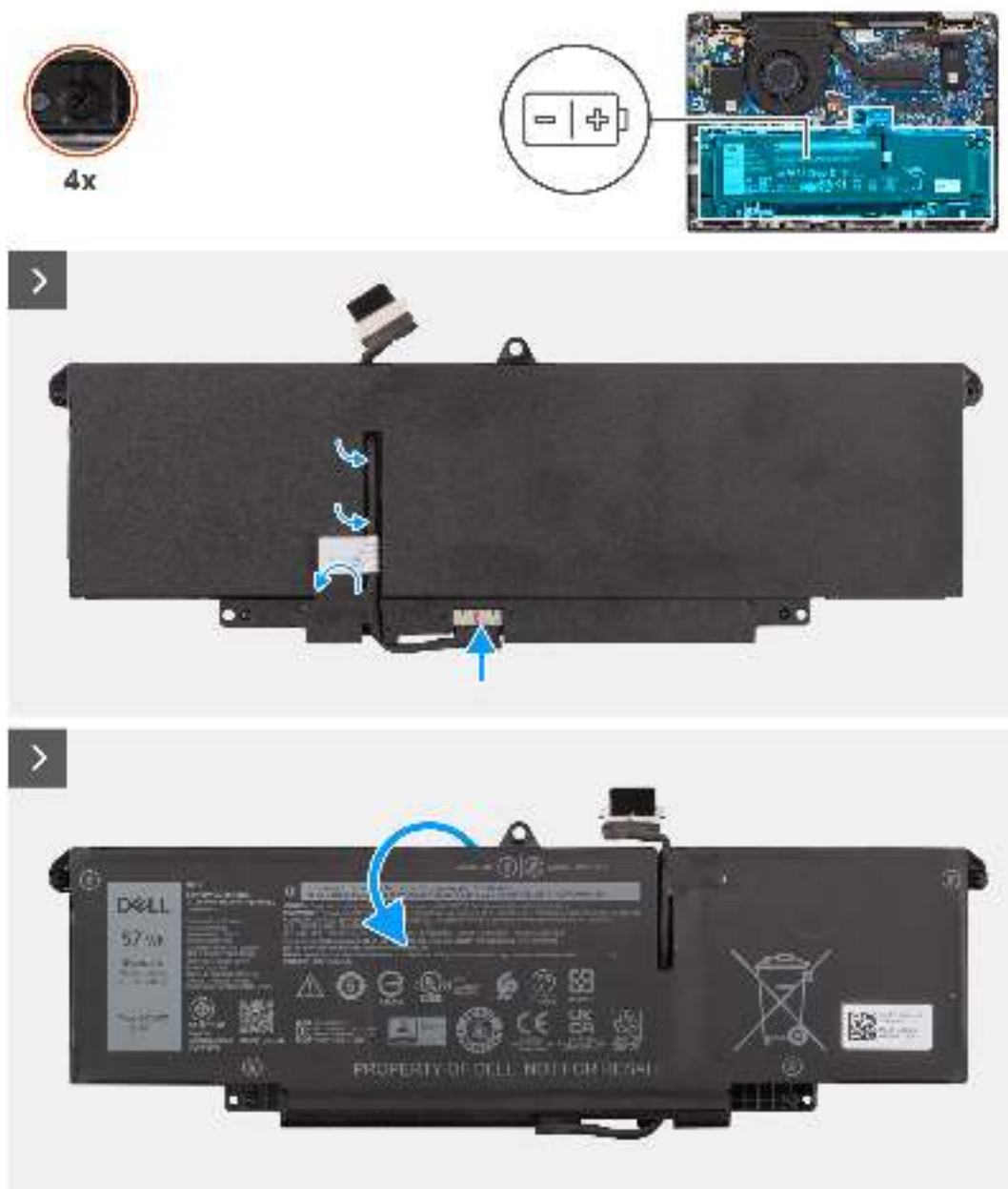
Abbildung 39. Installieren des 3-Zellen-Akkus
