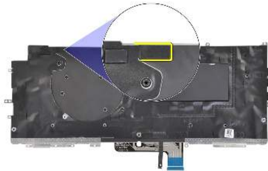
Abbildung 80. Anbringen der Tastaturfolie
