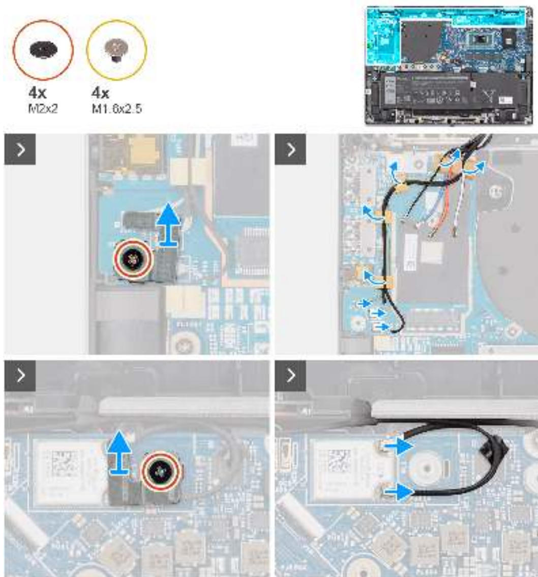
Abbildung 63. Entfernen des WLAN-Antennenmoduls
