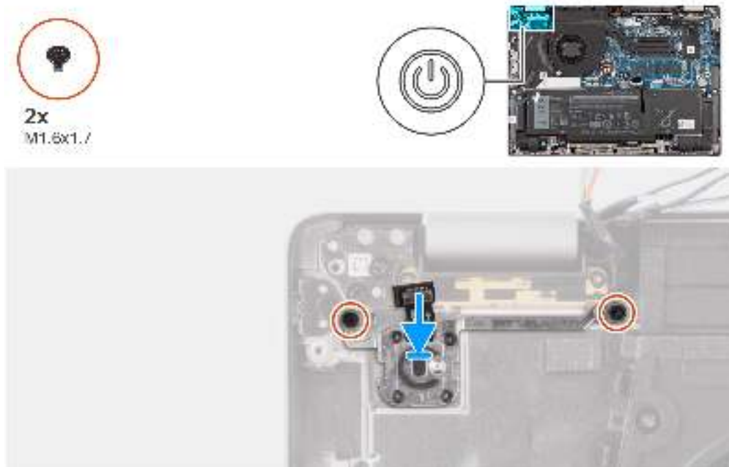
Abbildung 74. Installieren des Netzschalters mit optionalem Fingerabdruck-Lesegerät
