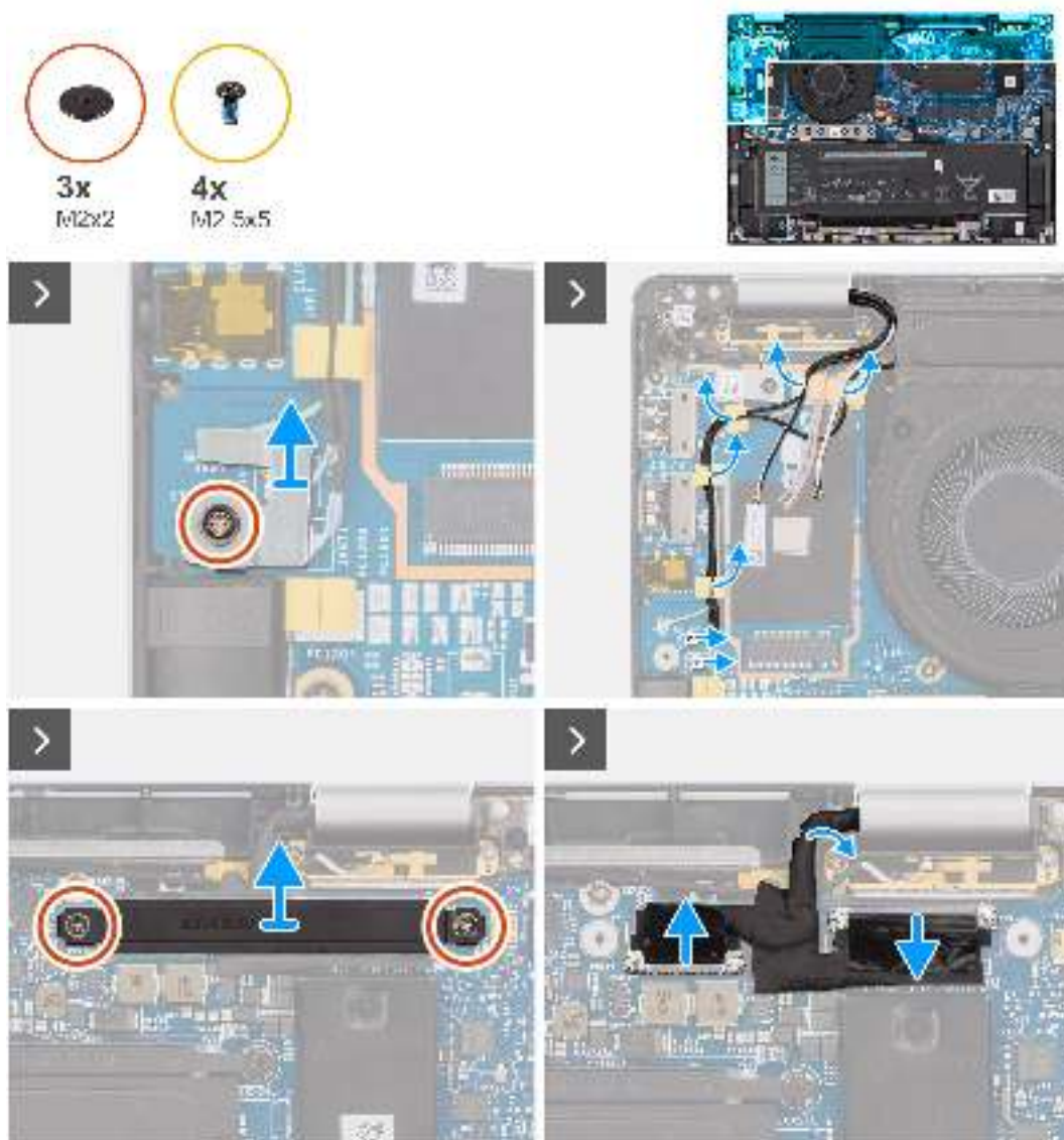
Abbildung 45. Entfernen der Displaybaugruppe
