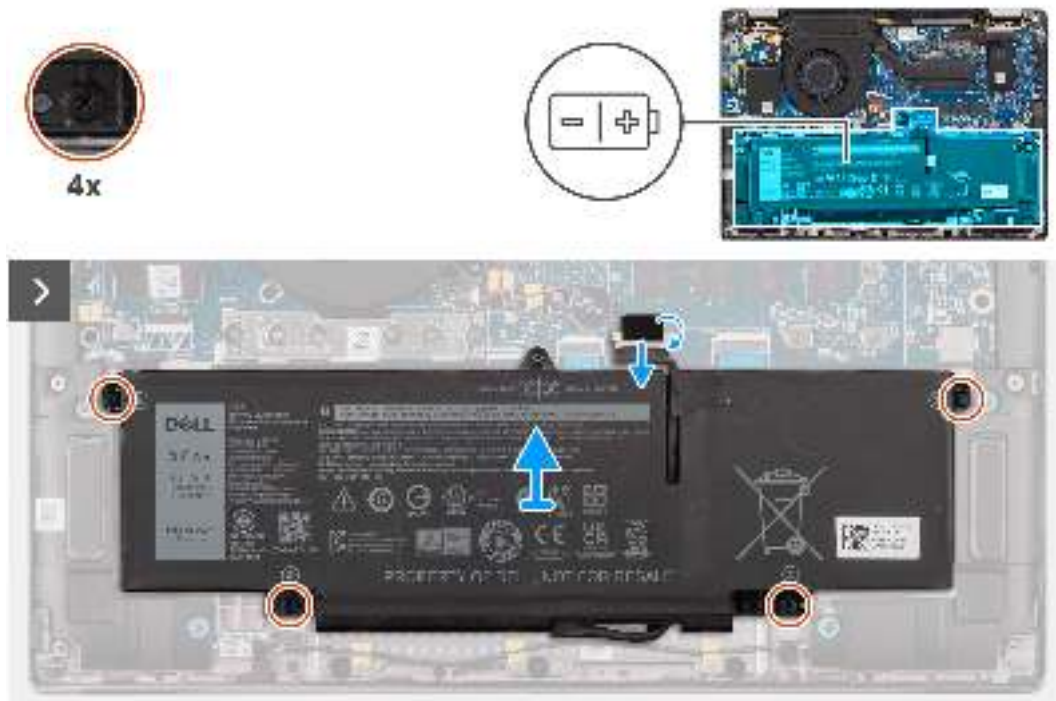
Abbildung 37. Entfernen des 3-Zellen-Akkus
