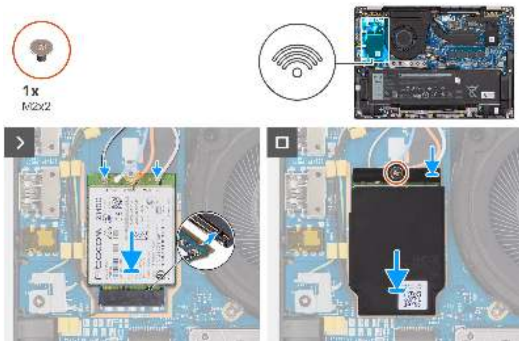
Abbildung 22. Installieren der 4G-WWAN-Karte
