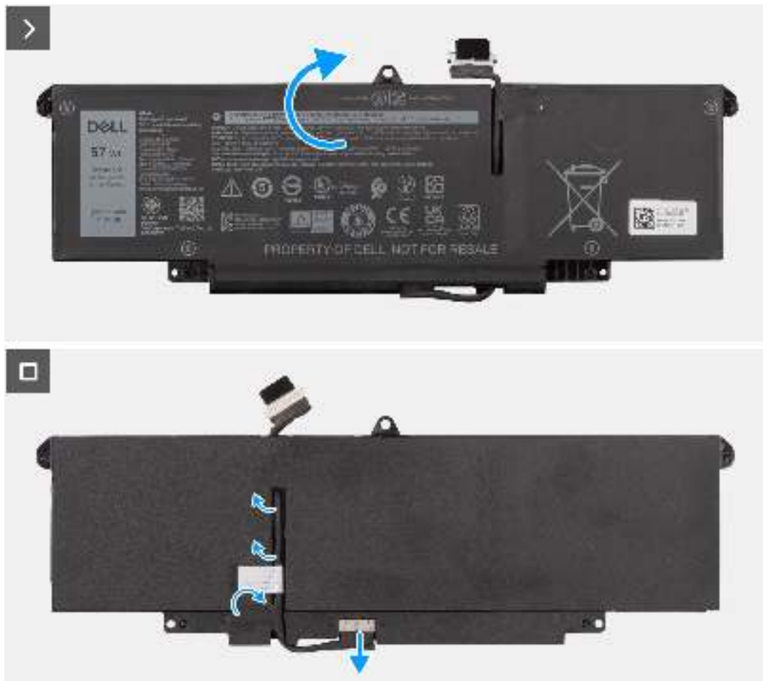
Abbildung 38. Entfernen des 3-Zellen-Akkus
