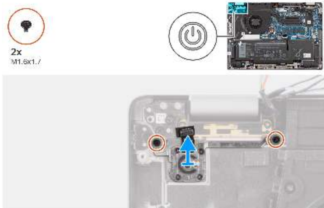
Abbildung 73. Entfernen des Netzschalters mit optionalem Fingerabdruck-Lesegerät
