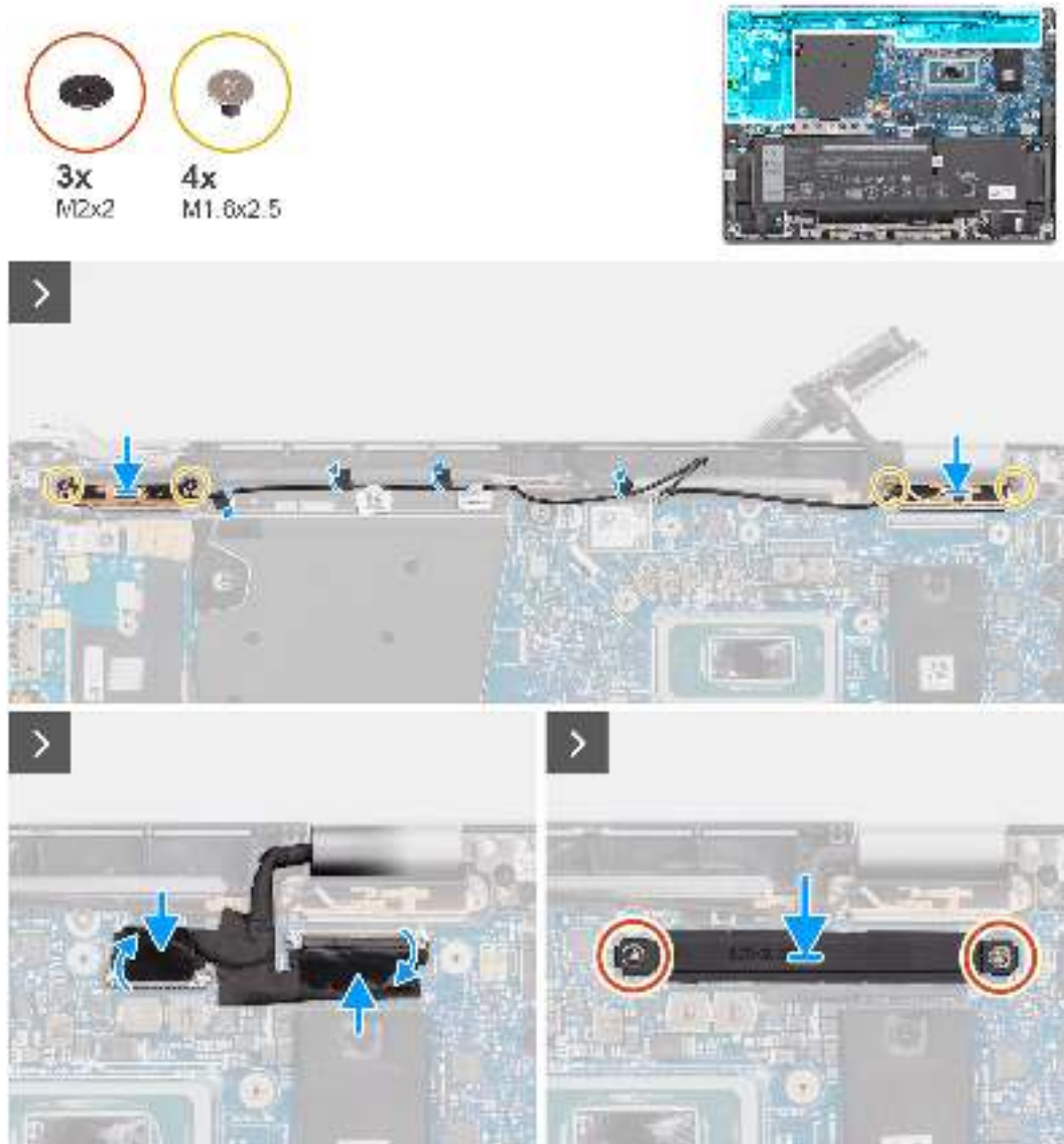
Abbildung 65. Installieren des WLAN-Antennenmoduls
