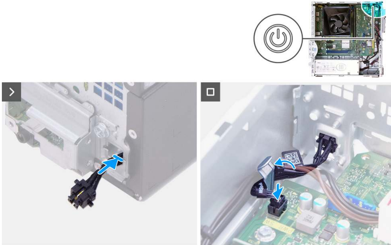
Abbildung 44. Installieren des Netzschalters
