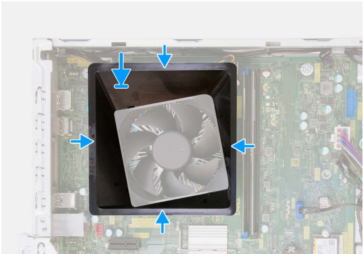
Abbildung 38. Installieren der Lüfterverkleidung
