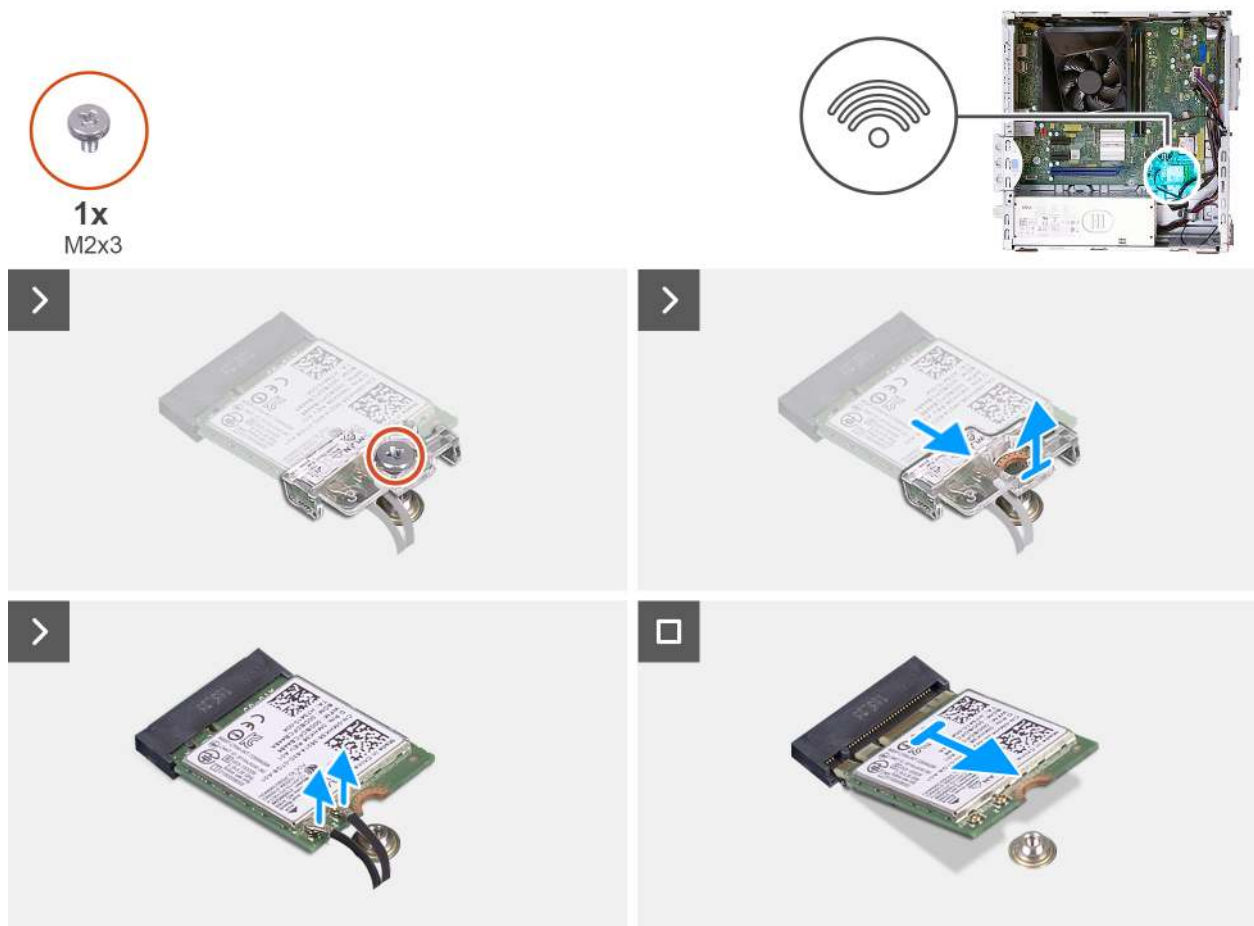
Abbildung 27. Entfernen der Wireless-Karte
