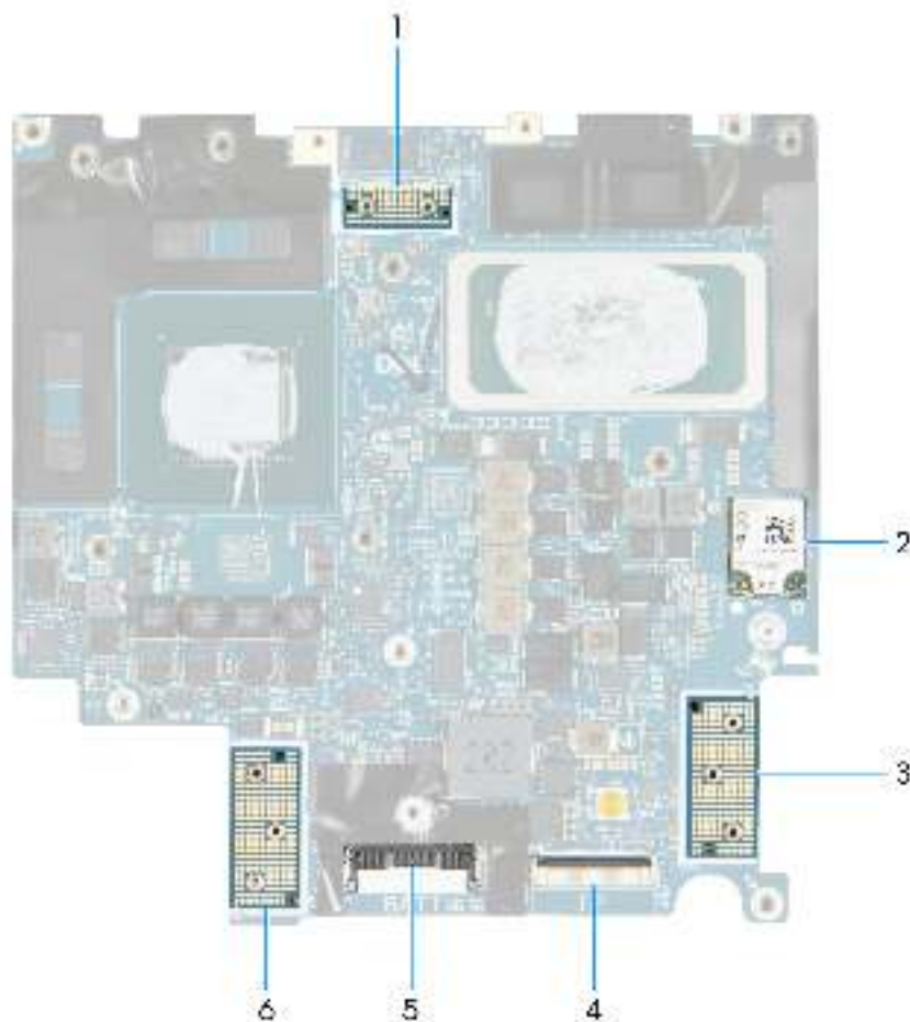
Abbildung 58. Anschlüsse auf der Hauptplatine
