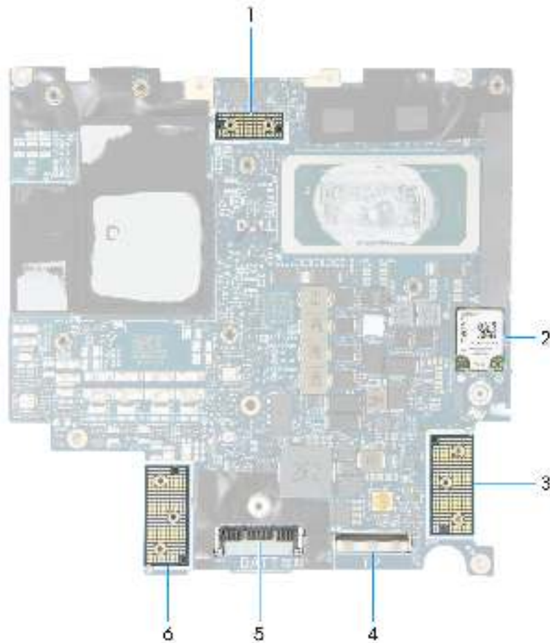
Abbildung 53. Anschlüsse auf der Hauptplatine
