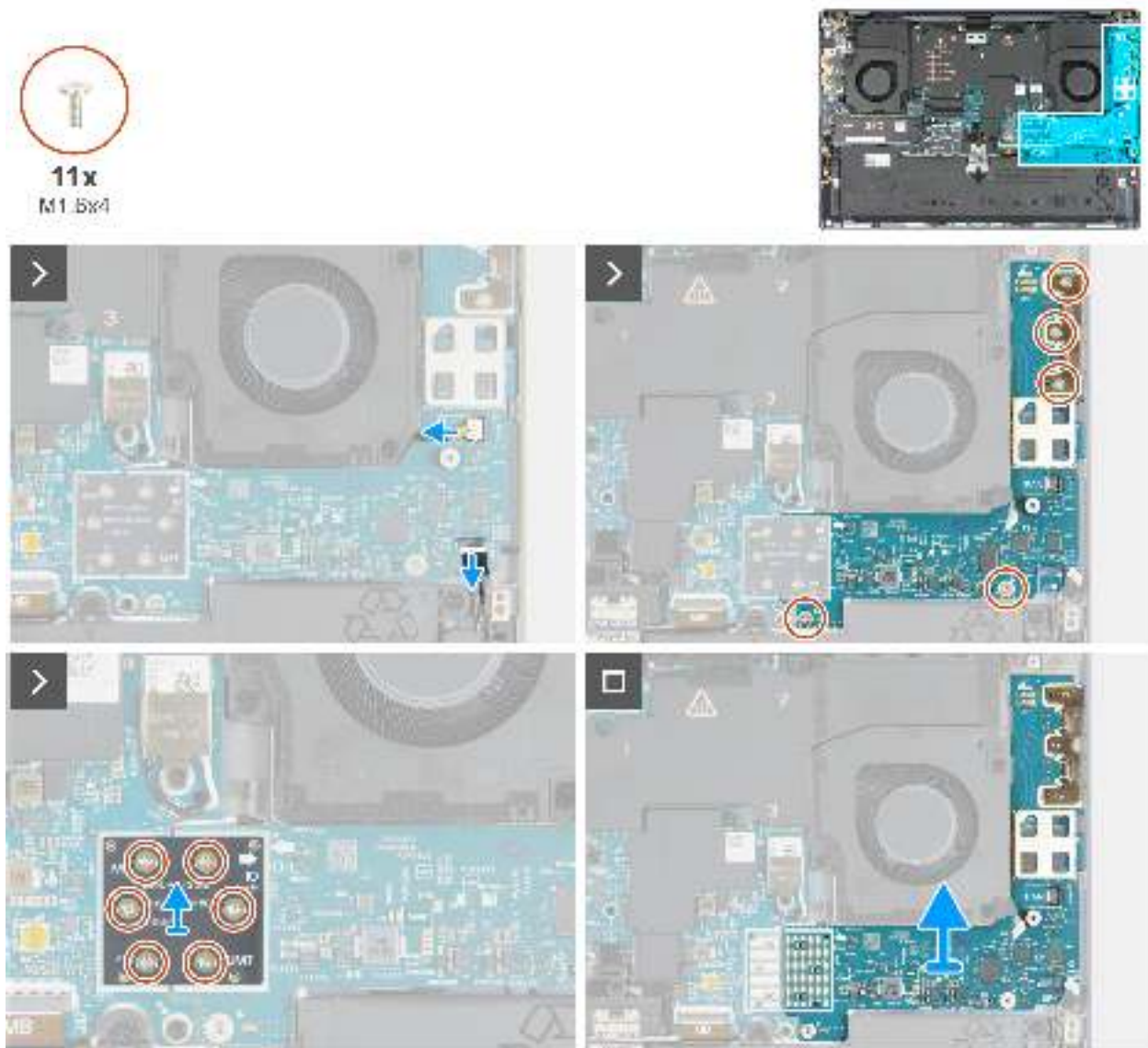
Abbildung 45. Entfernen der linken E/A-Platine
