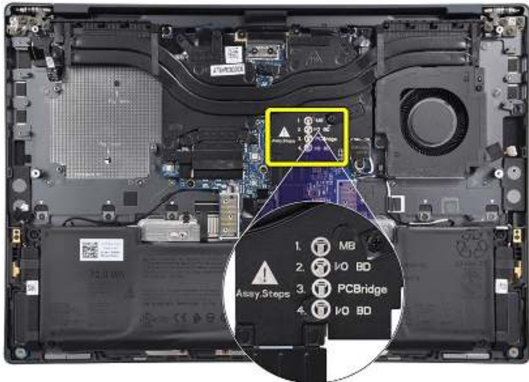
Abbildung 66. Auf dem Kühlkörper aufgedruckte Montageschritte
