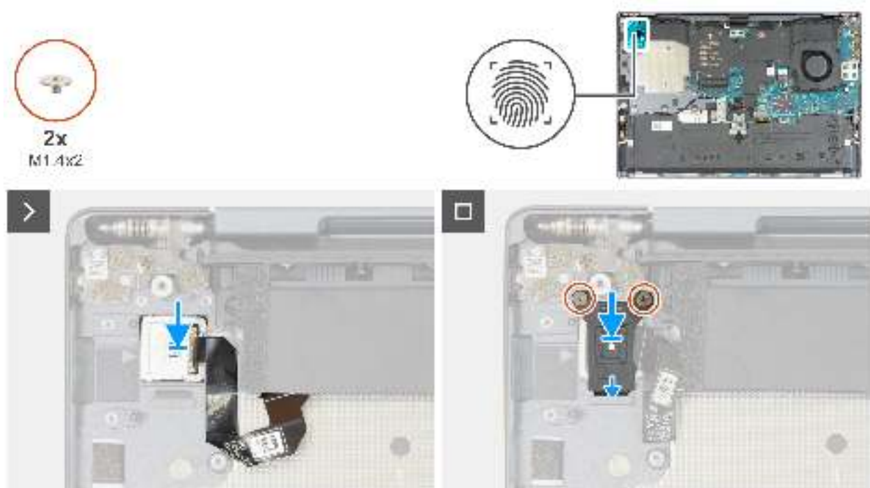
Abbildung 68. Einbauen des Netzschalters oder Fingerabdrucklesers
