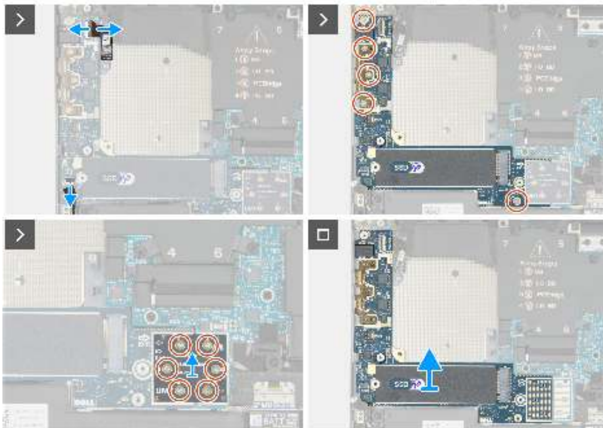
Abbildung 47. Entfernen der rechten E/A-Platine
