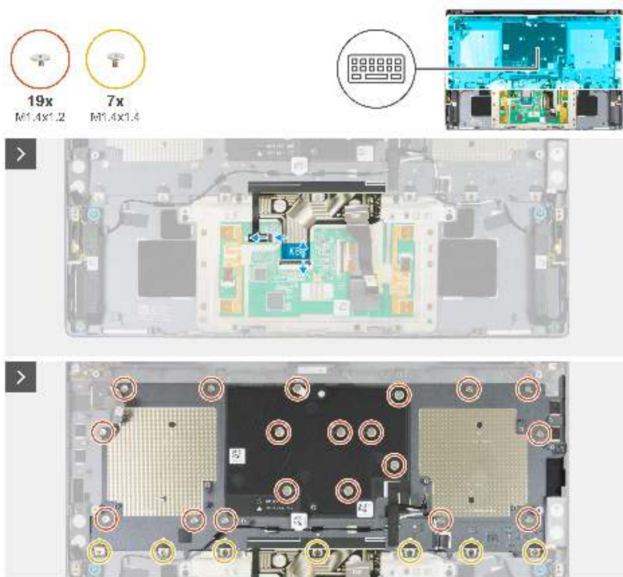
Abbildung 71. Entfernen der Tastatur
