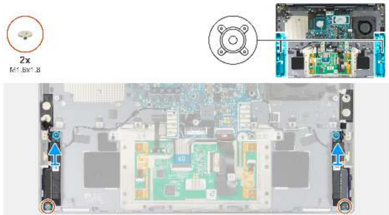
Abbildung 69. Entfernen der Lautsprecher
