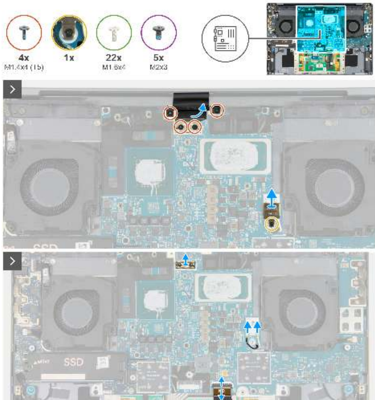
Abbildung 59. Entfernen der Hauptplatine (separate Grafikkarte)
