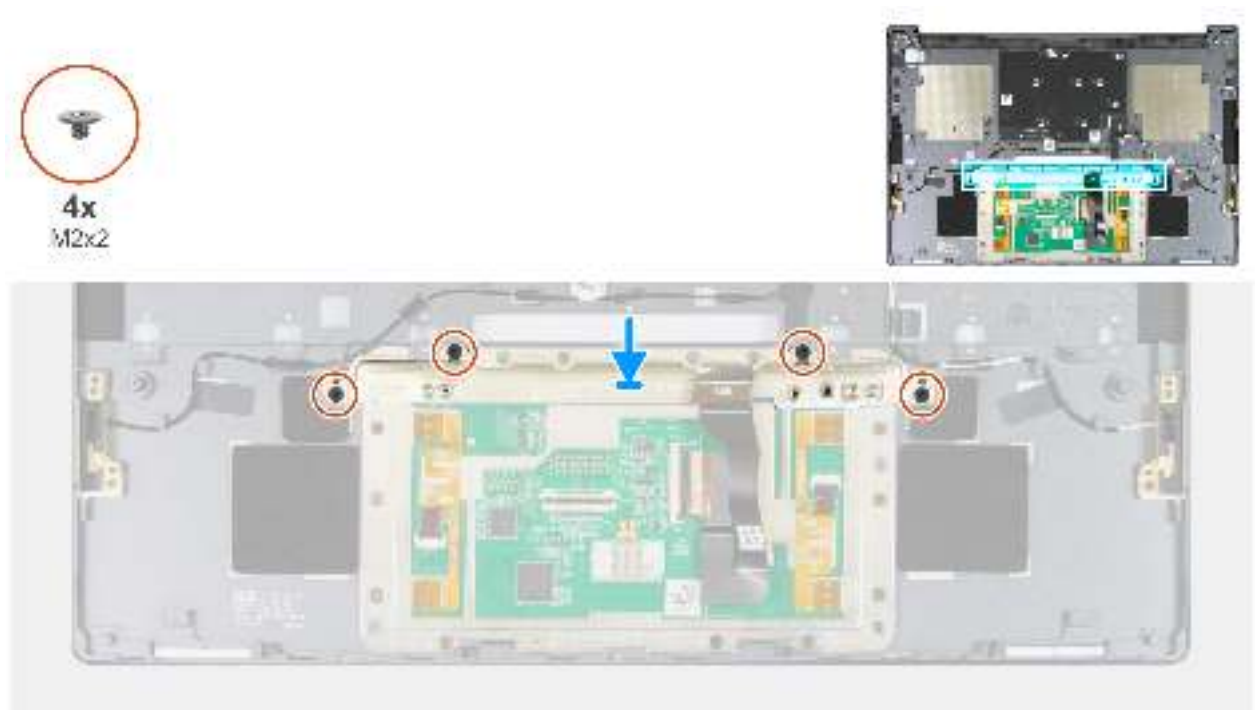
Abbildung 80. Wiedereinbauen der Touchpadhalterung
