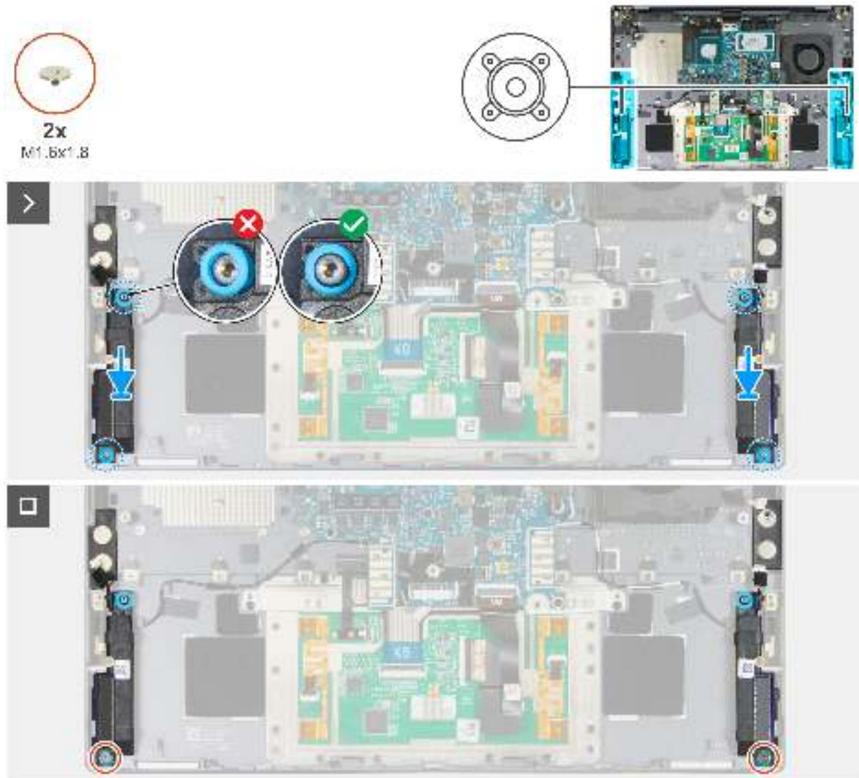
Abbildung 70. Installieren der Lautsprecher
