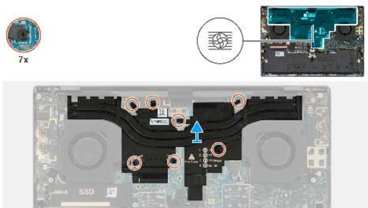
Abbildung 41. Kühlkörper entfernen
