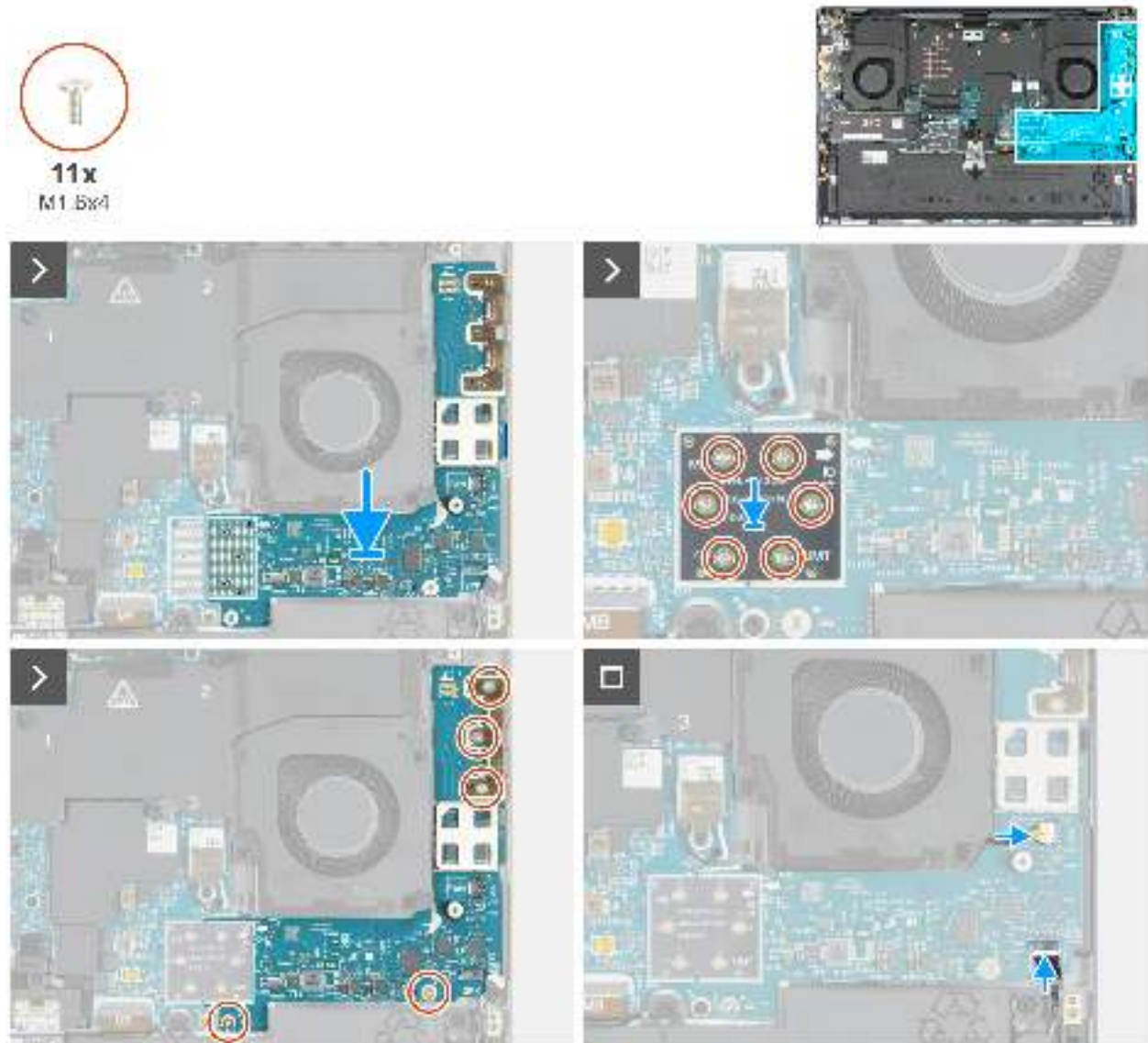
Abbildung 46. Installieren der linken E/A-Platine
