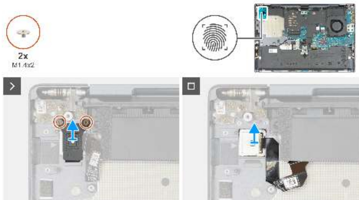
Abbildung 67. Entfernen des Netzschalters oder Fingerabdrucklesers
