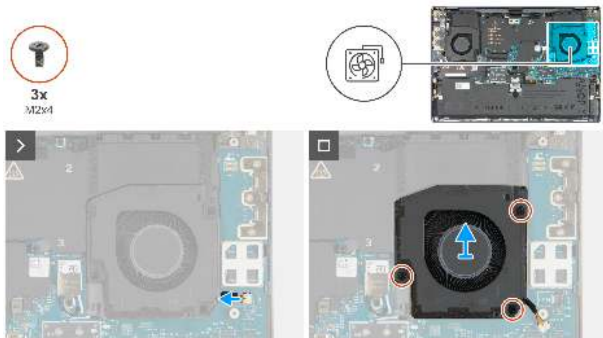
Abbildung 27. Entfernen des linken Lüfters
