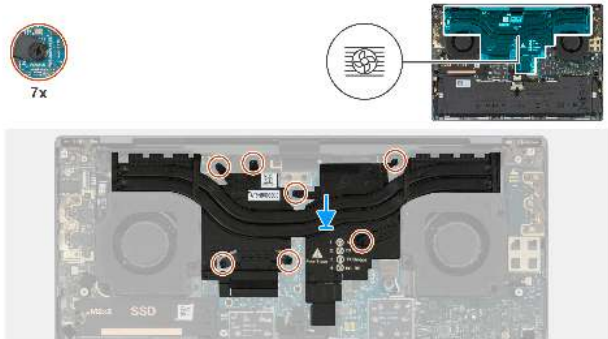
Abbildung 42. Einsetzen des Kühlkörpers
