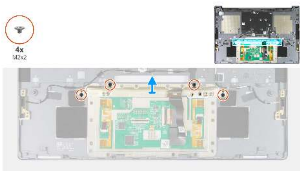
Abbildung 77. Entfernen der Touchpadhalterung
