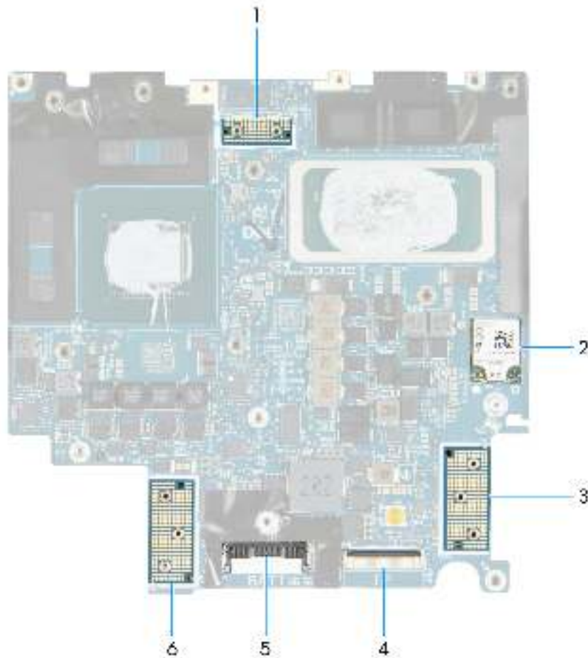
Abbildung 62. Anschlüsse auf der Hauptplatine
