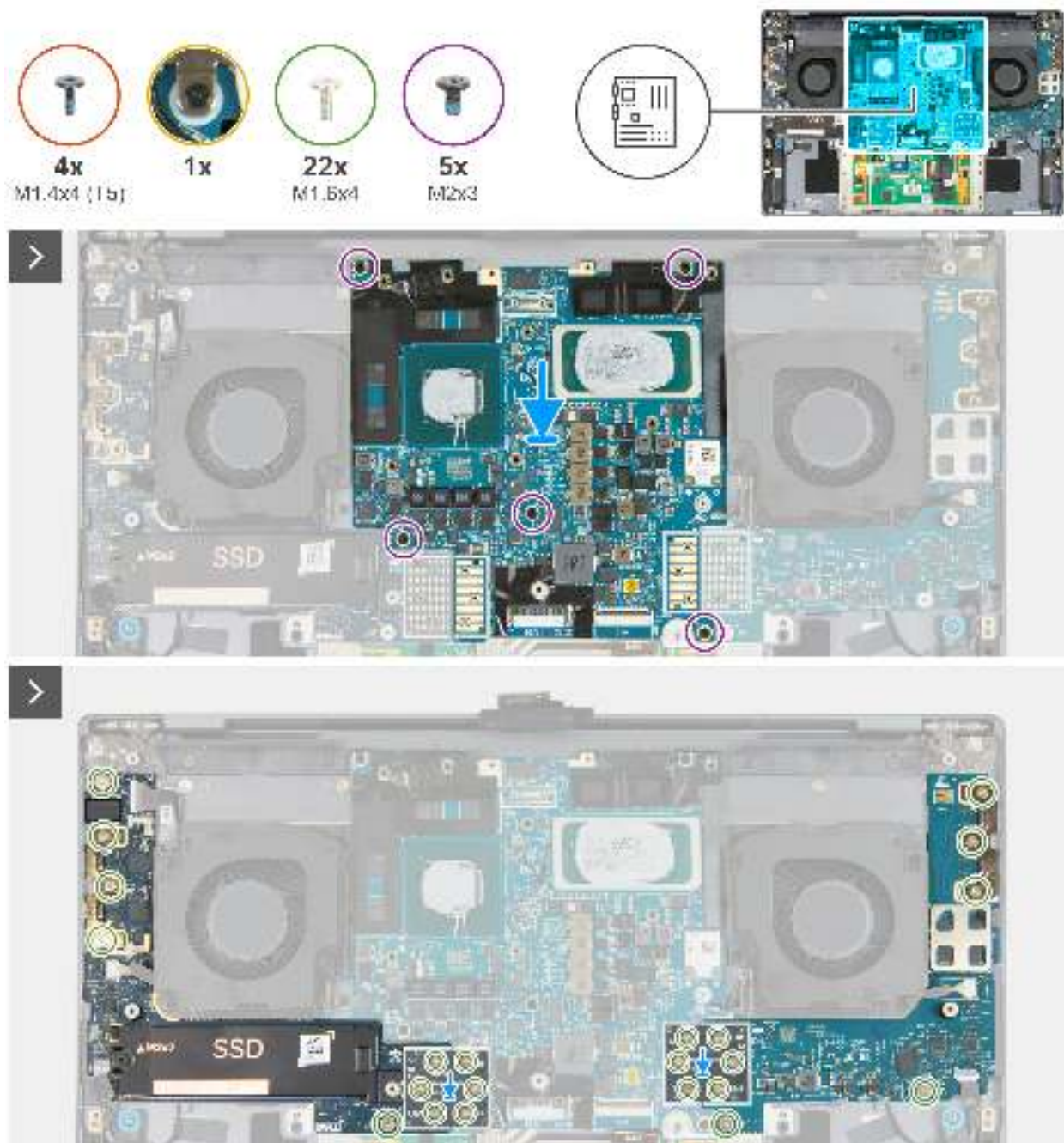
Abbildung 63. Einbauen der Hauptplatine (separate Grafikkarte)
