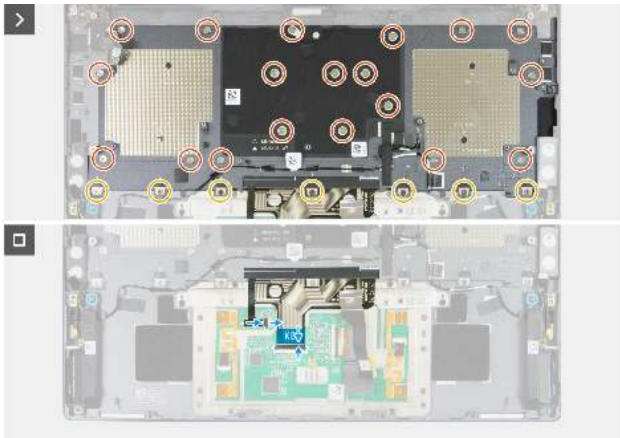
Abbildung 76. Einbauen der Tastatur
