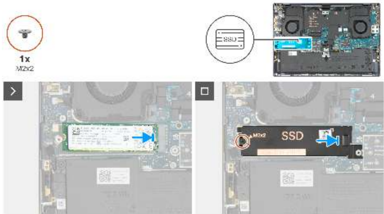
Abbildung 24. Installieren des M.2 2280-Solid-State-Laufwerks
