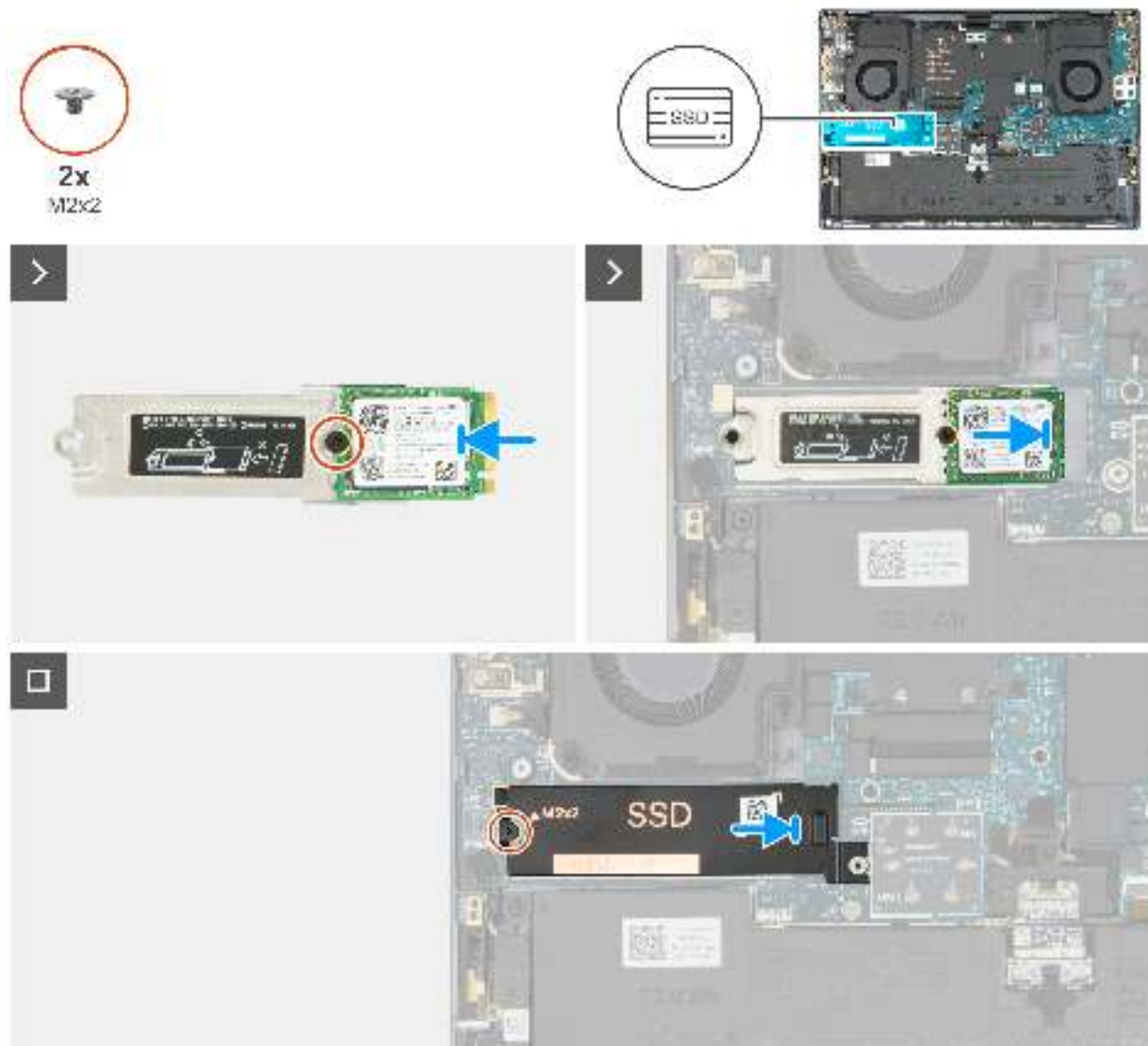
Abbildung 26. Installieren des M.2 2230-Solid-State-Laufwerks
