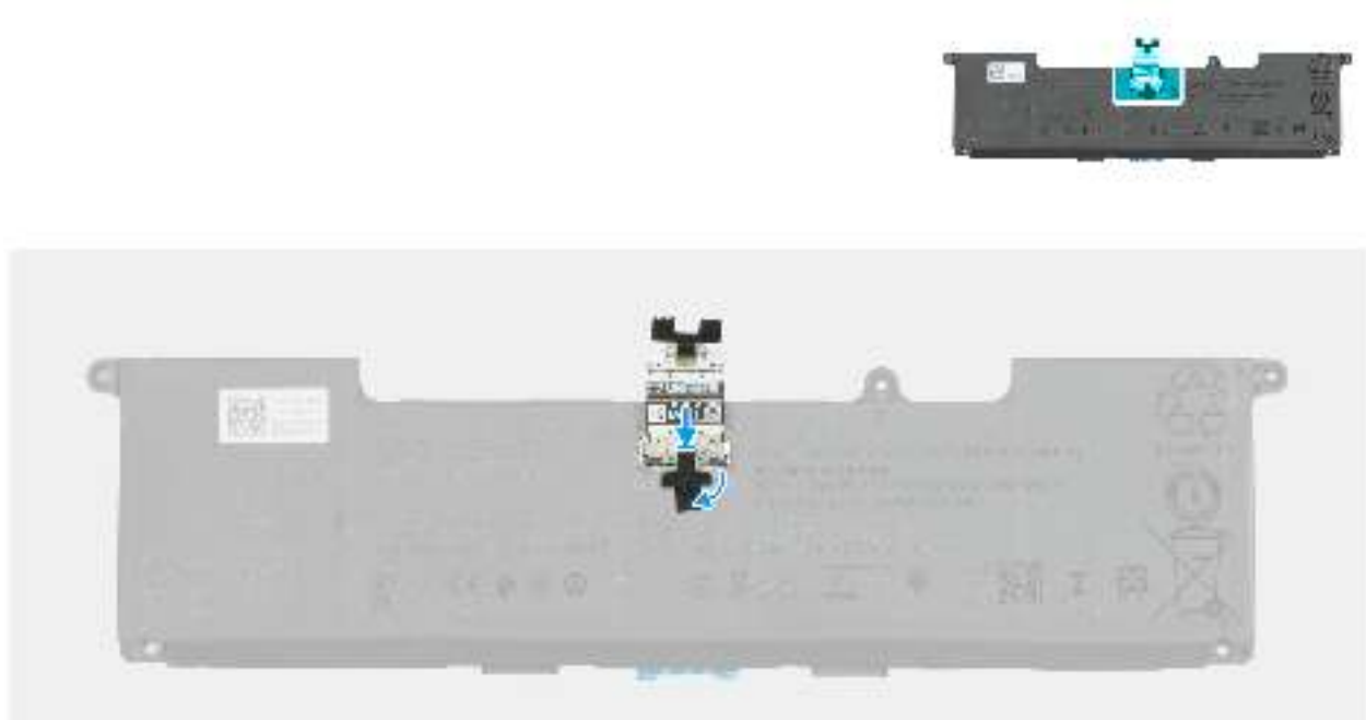
Abbildung 22. Austauschen des Akkukabels
