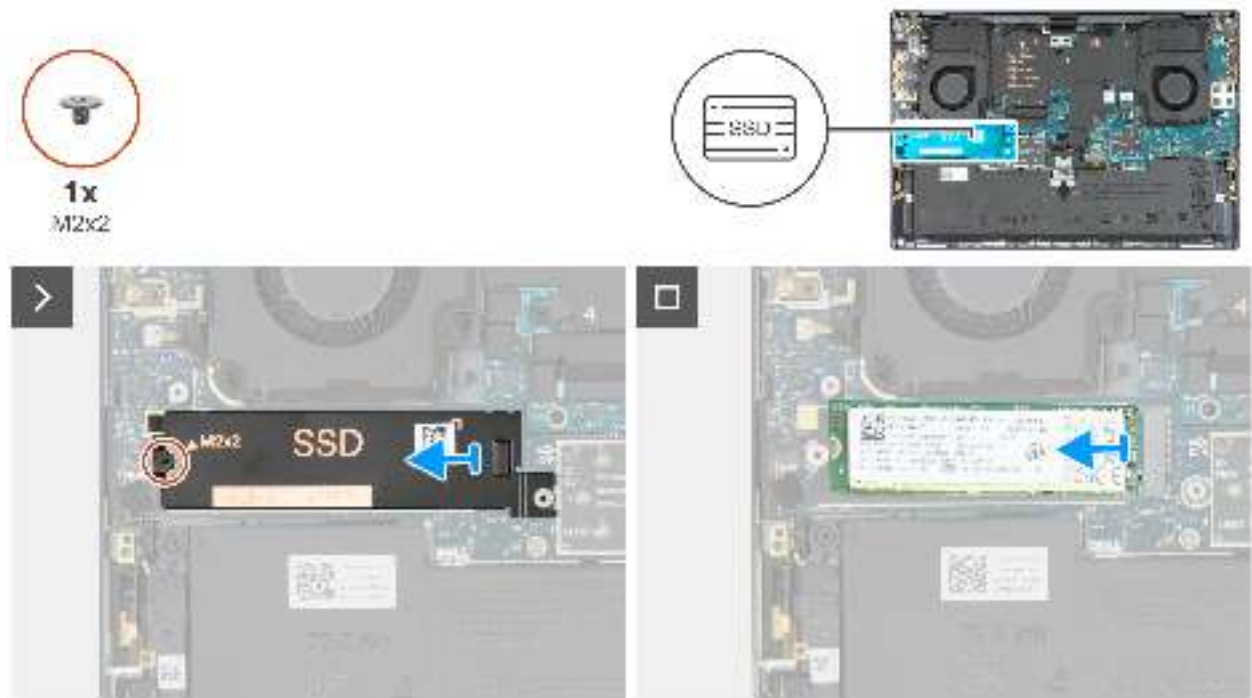
Abbildung 23. Entfernen des M.2-2280-Solid-State-Laufwerks
