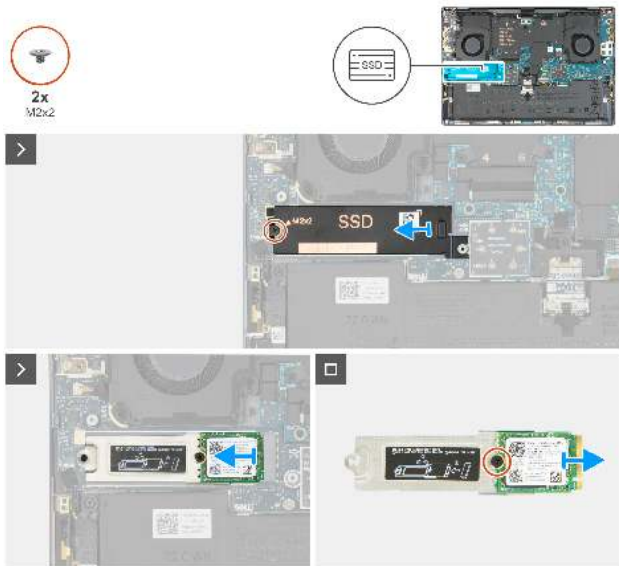
Abbildung 25. Entfernen des M.2-2230-Solid-State-Laufwerks
