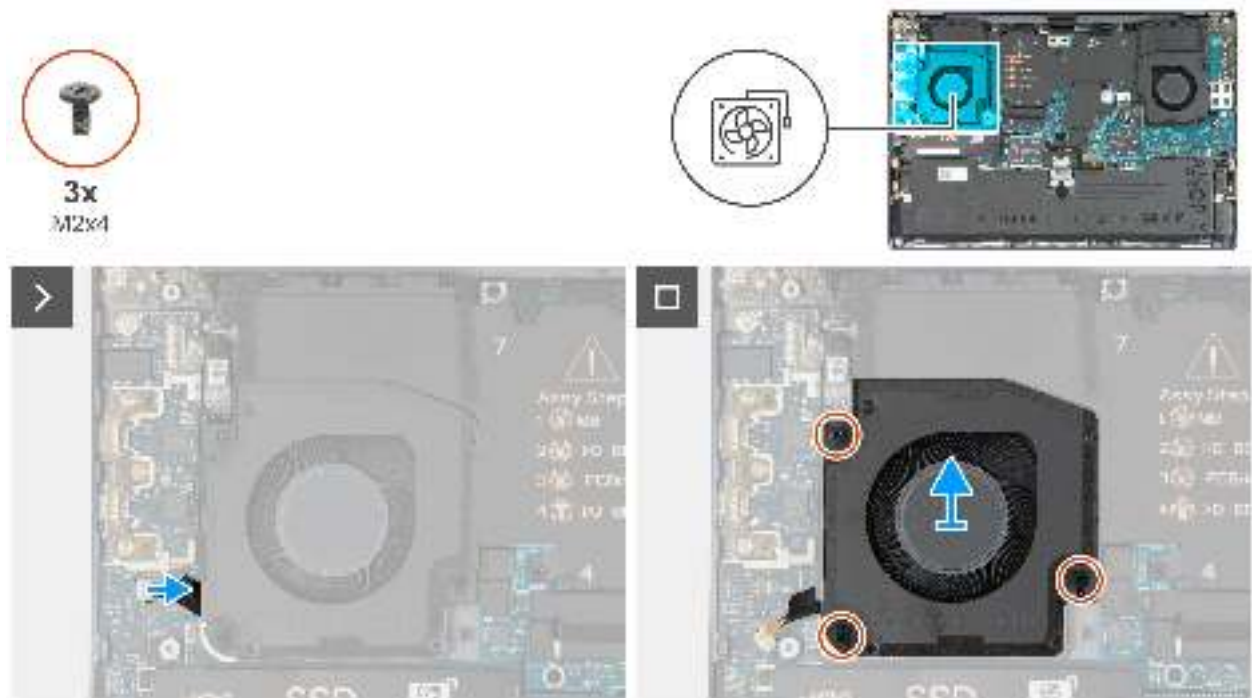
Abbildung 29. Entfernen des rechten Lüfters
