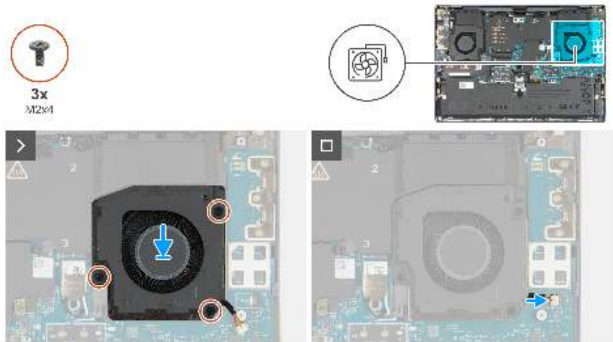
Abbildung 28. Installieren des linken Lüfters
