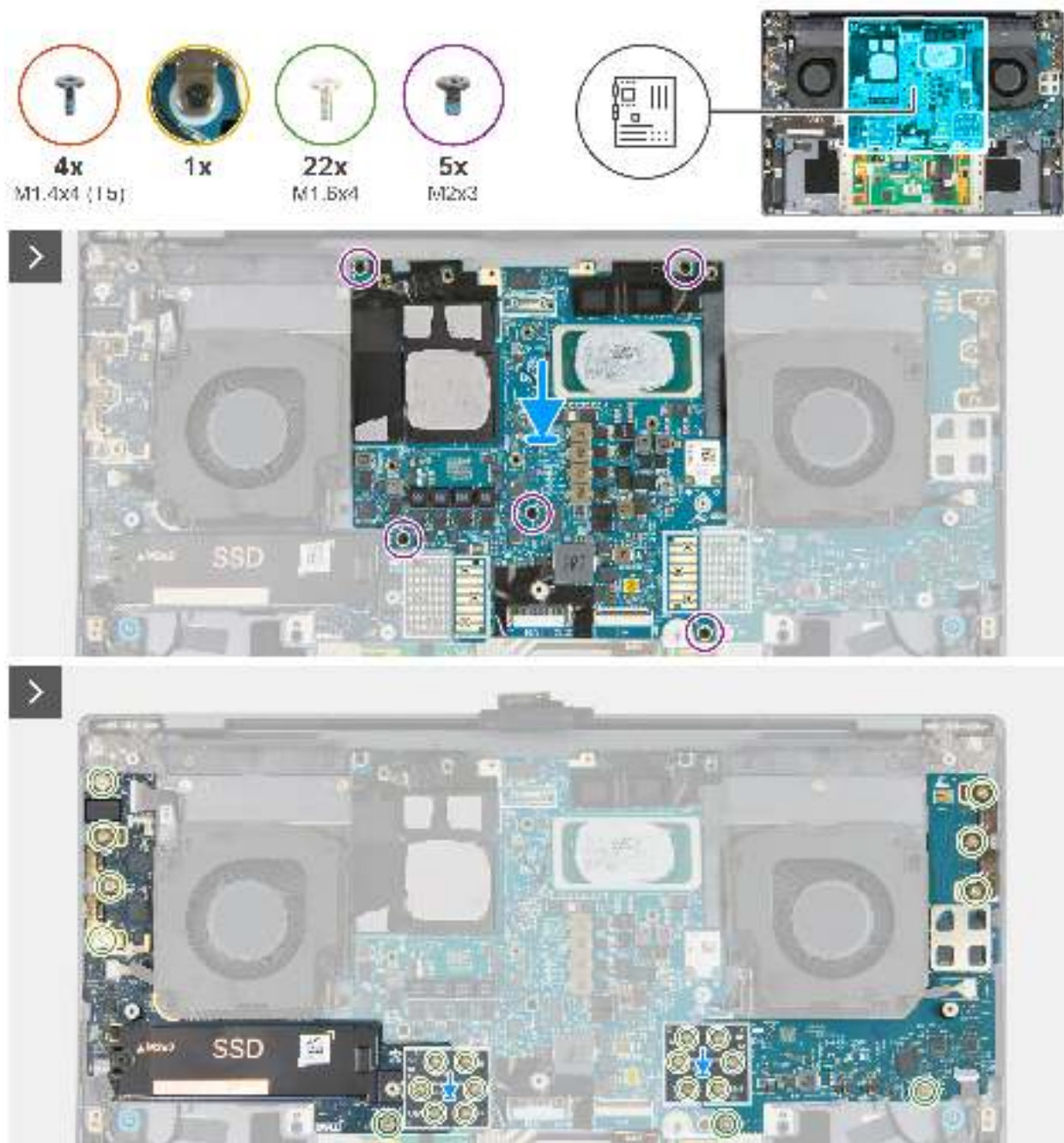
Abbildung 54. Einbauen der Hauptplatine (integrierte Grafikkarte)
