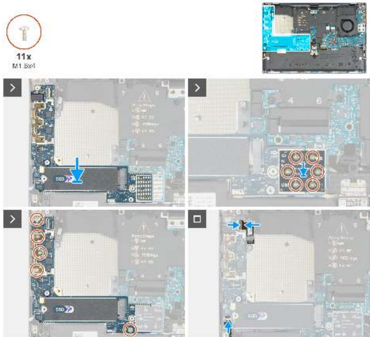
Abbildung 48. Installieren der rechten E/A-Platine
