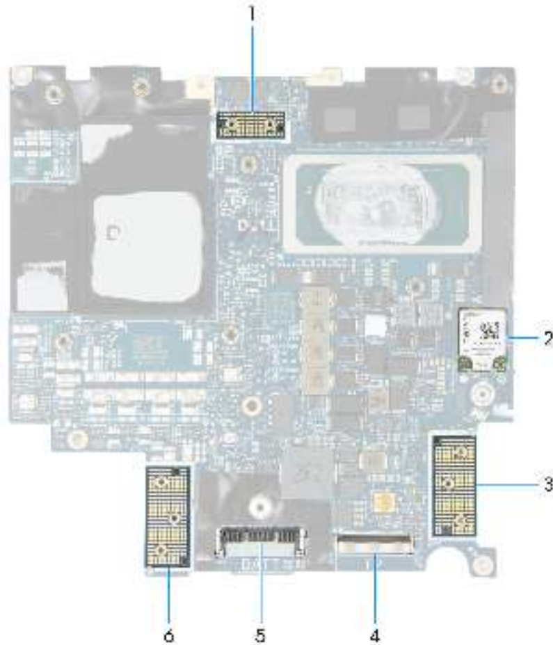
Abbildung 49. Anschlüsse auf der Hauptplatine
