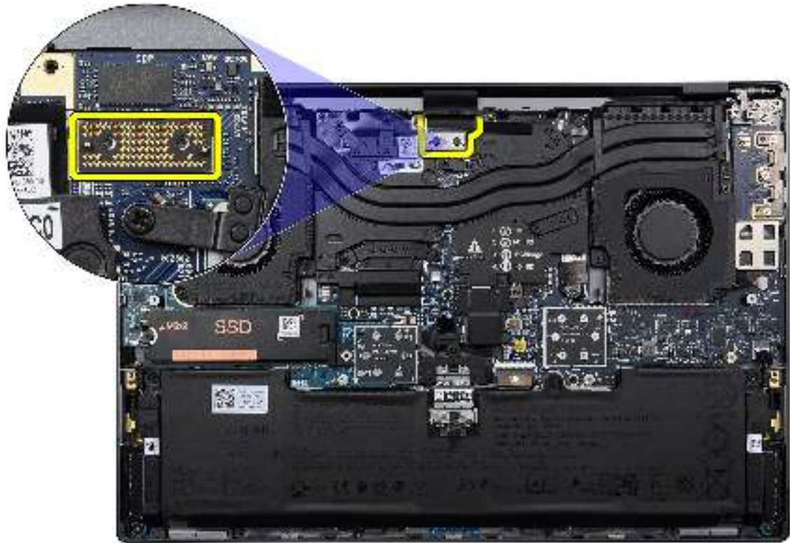
Abbildung 35. Kabelzwischenplatine der Bildschirmbaugruppe
