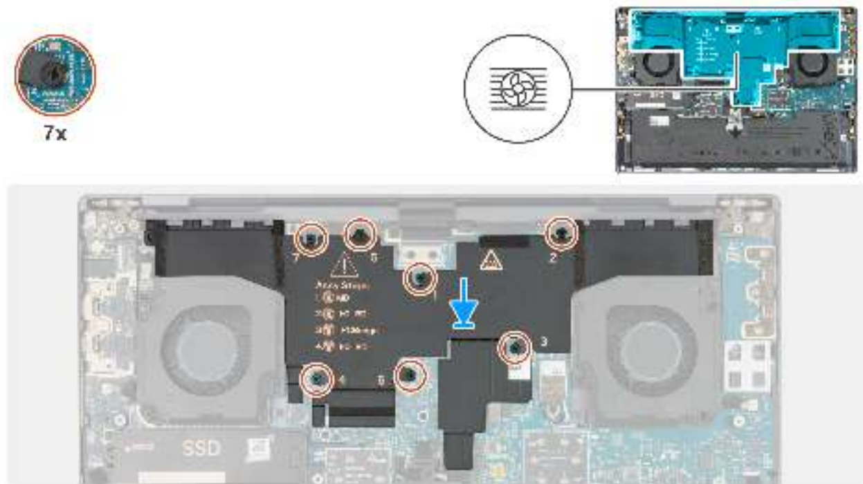
Abbildung 44. Einsetzen des Kühlkörpers
