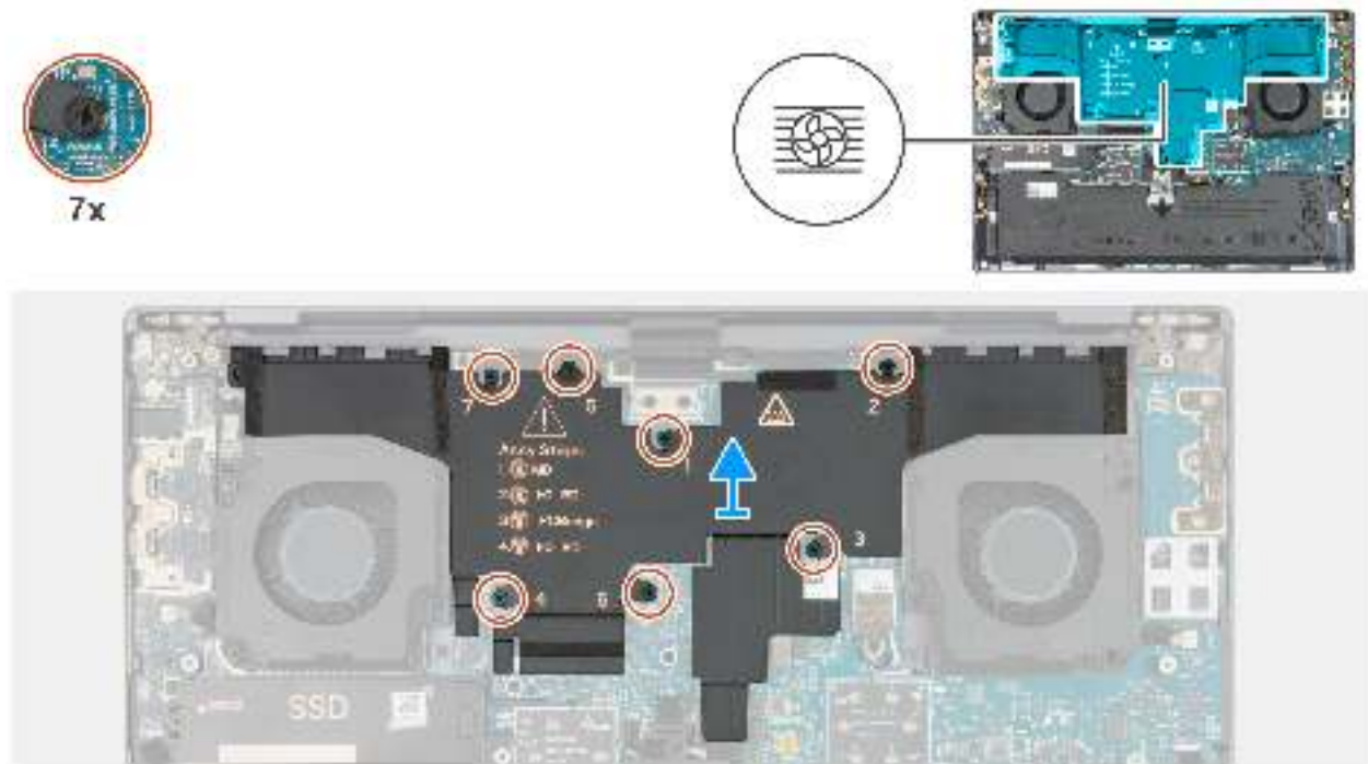
Abbildung 43. Kühlkörper entfernen
