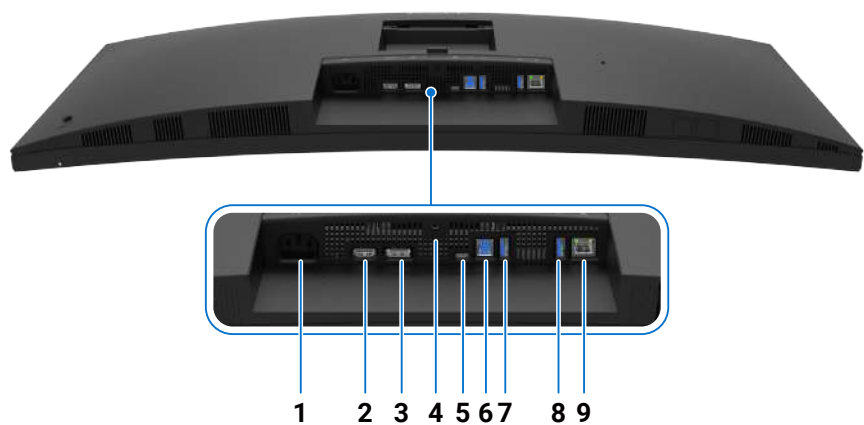
Abbildung 4. Unteransicht des Monitors
