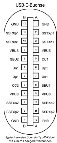
Abbildung 9. USB-C-Anschluss
