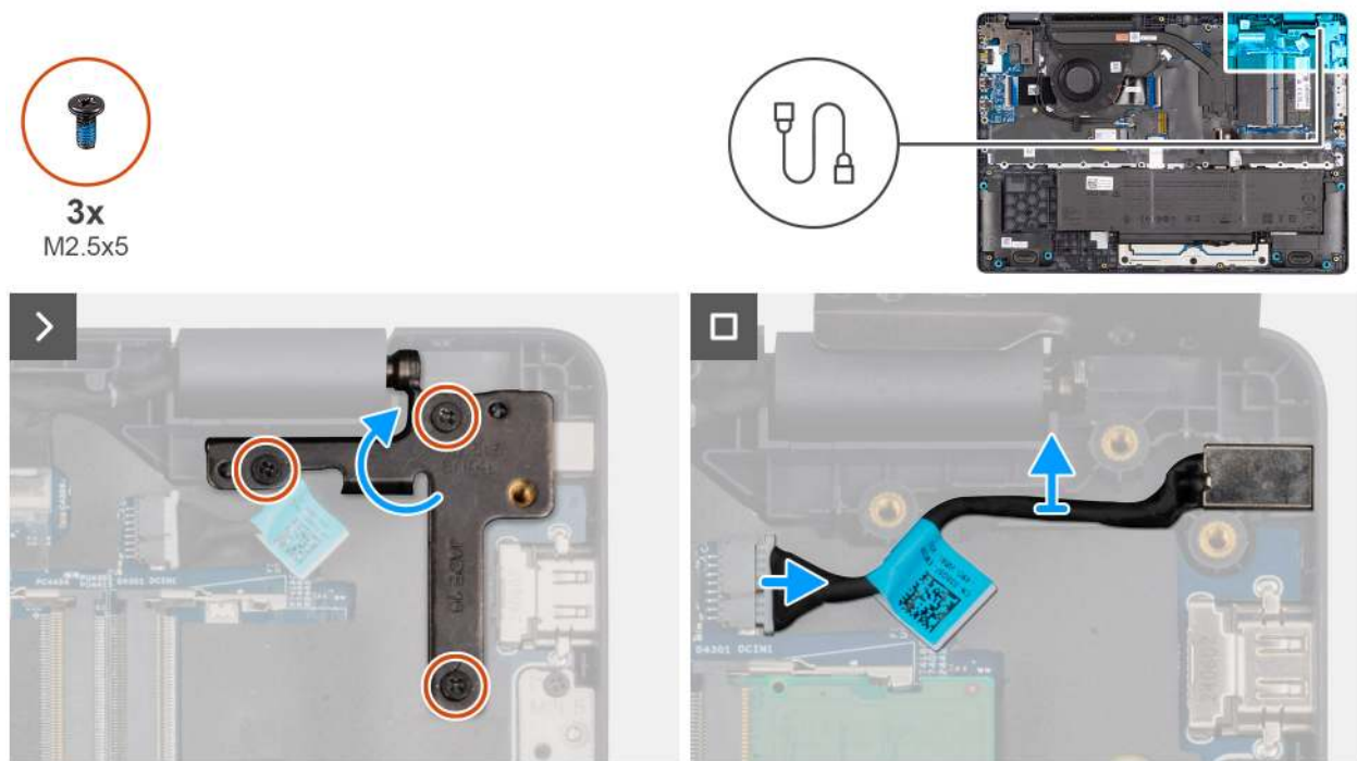
Abbildung 32. Entfernen des Netzadapteranschlusses
