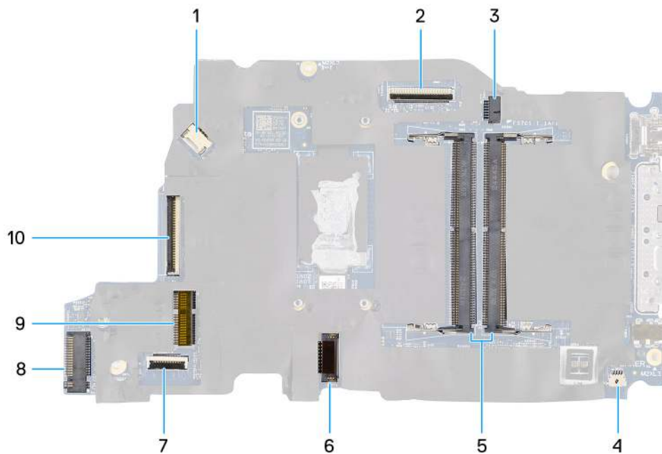
Abbildung 42. Hauptplatinenanschlüsse
