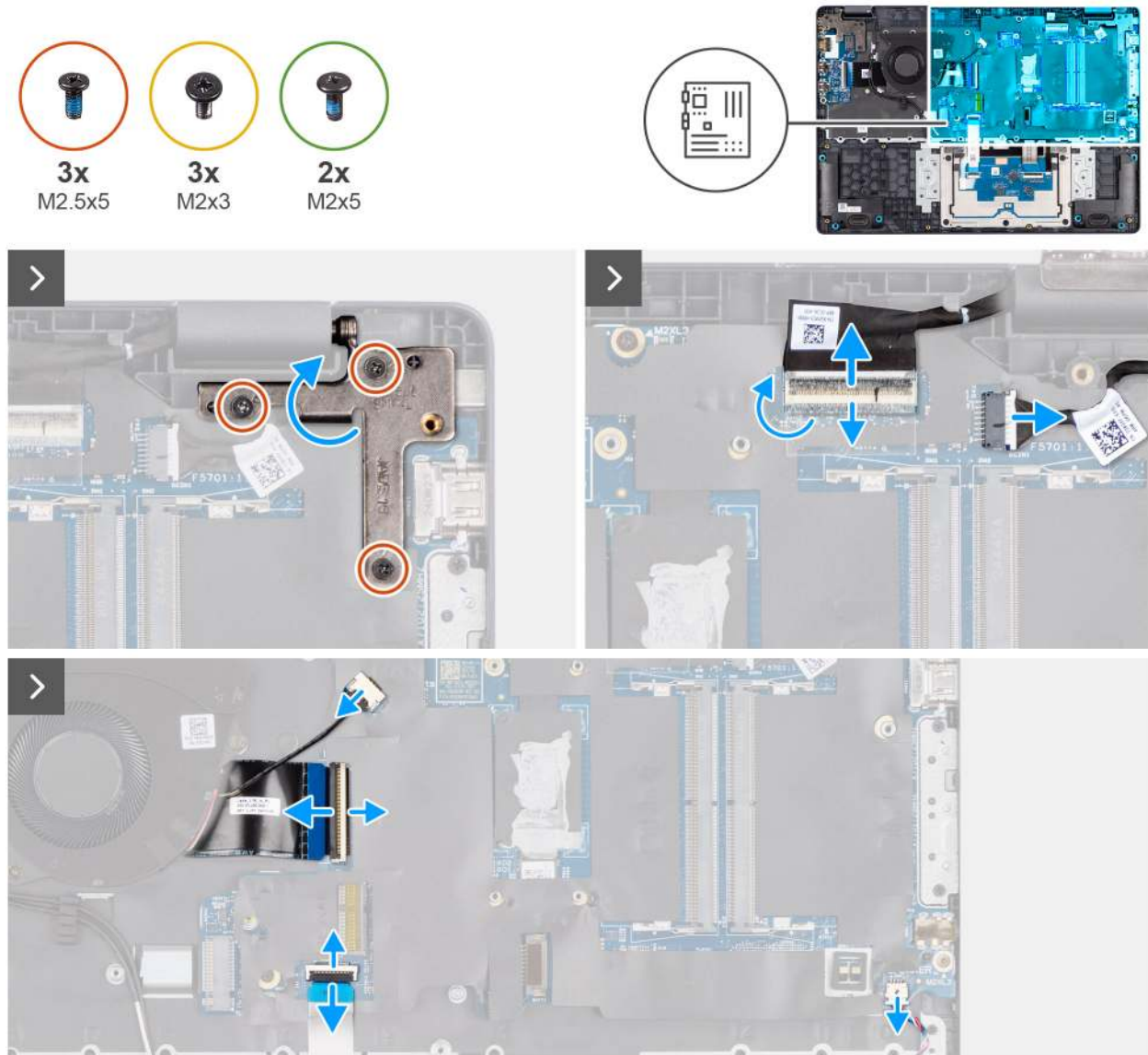
Abbildung 43. Entfernen der Systemplatine
