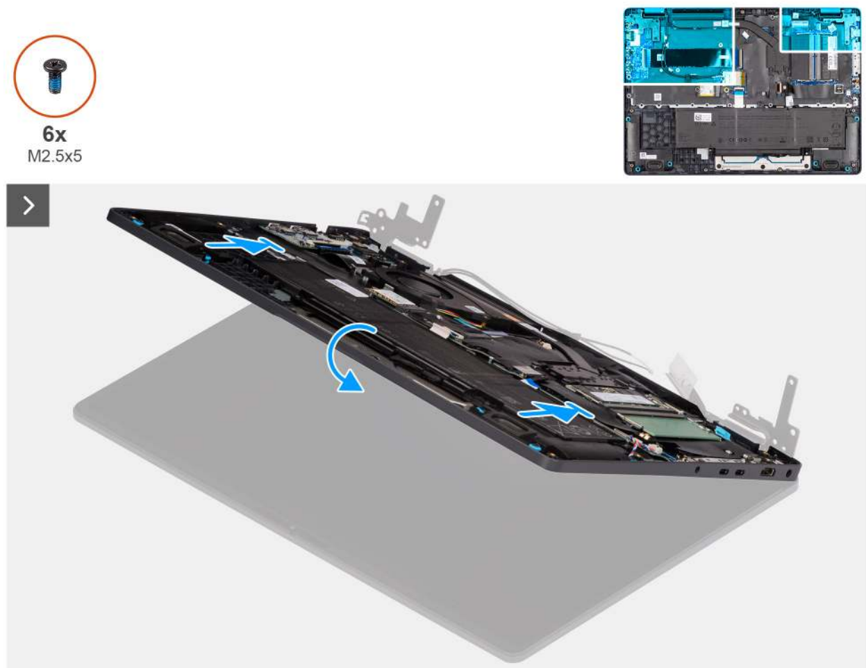
Abbildung 65. Einbauen der Displaybaugruppe
