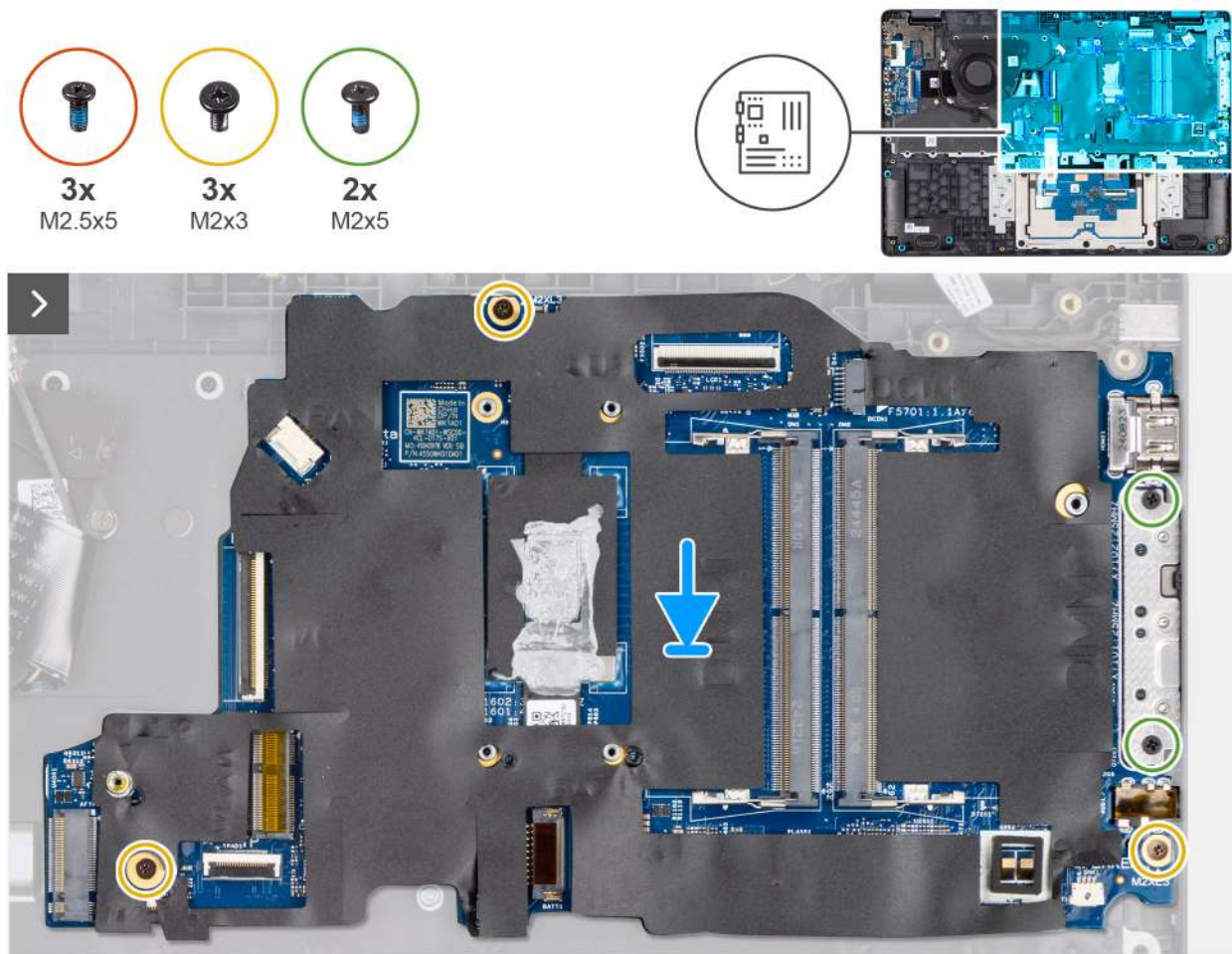
Abbildung 46. Einbauen der Systemplatine
