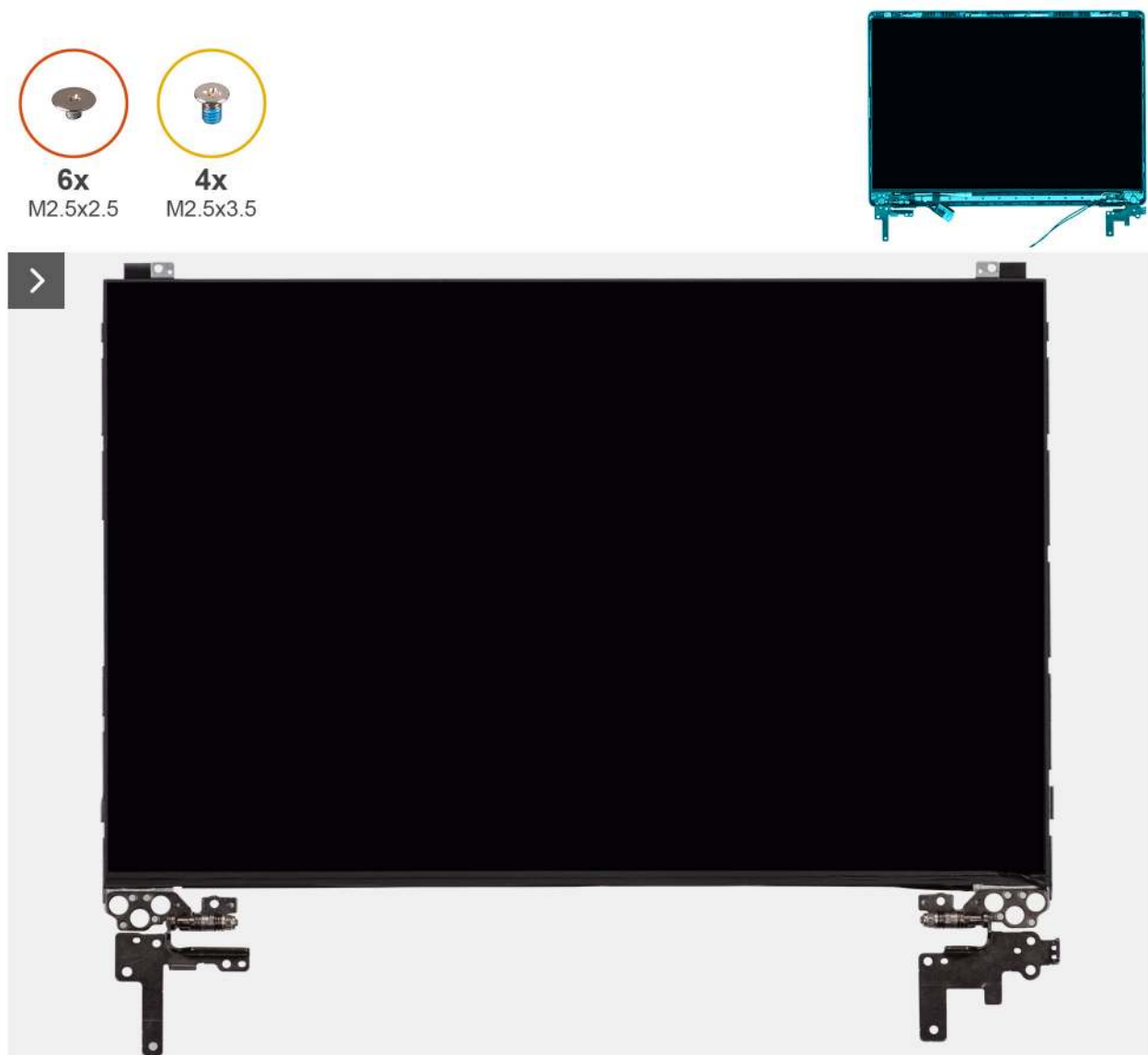
Abbildung 78. Installieren der Bildschirmbaugruppe
