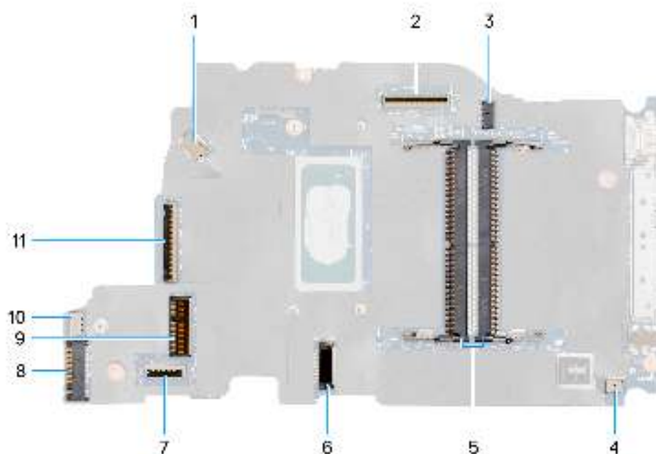
Abbildung 66. Hauptplatinenanschlüsse
