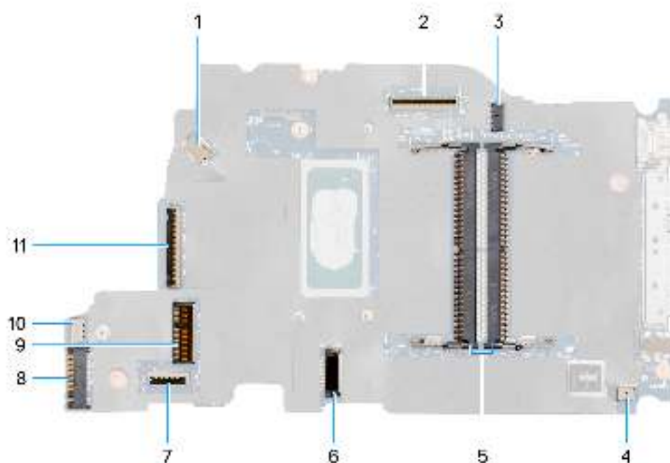
Abbildung 66. Hauptplatinenanschlüsse
