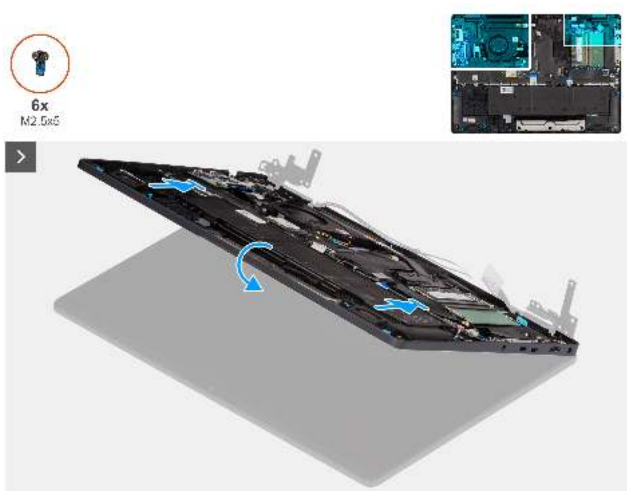
Abbildung 96. Einbauen der Displaybaugruppe
