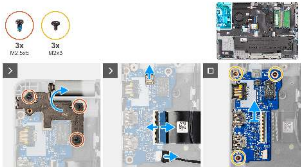
Abbildung 51. Entfernen der E/A-Platine
