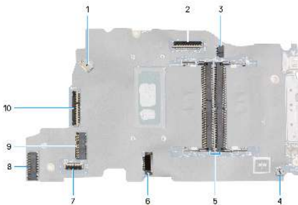
Abbildung 57. Hauptplattenanschlüsse
