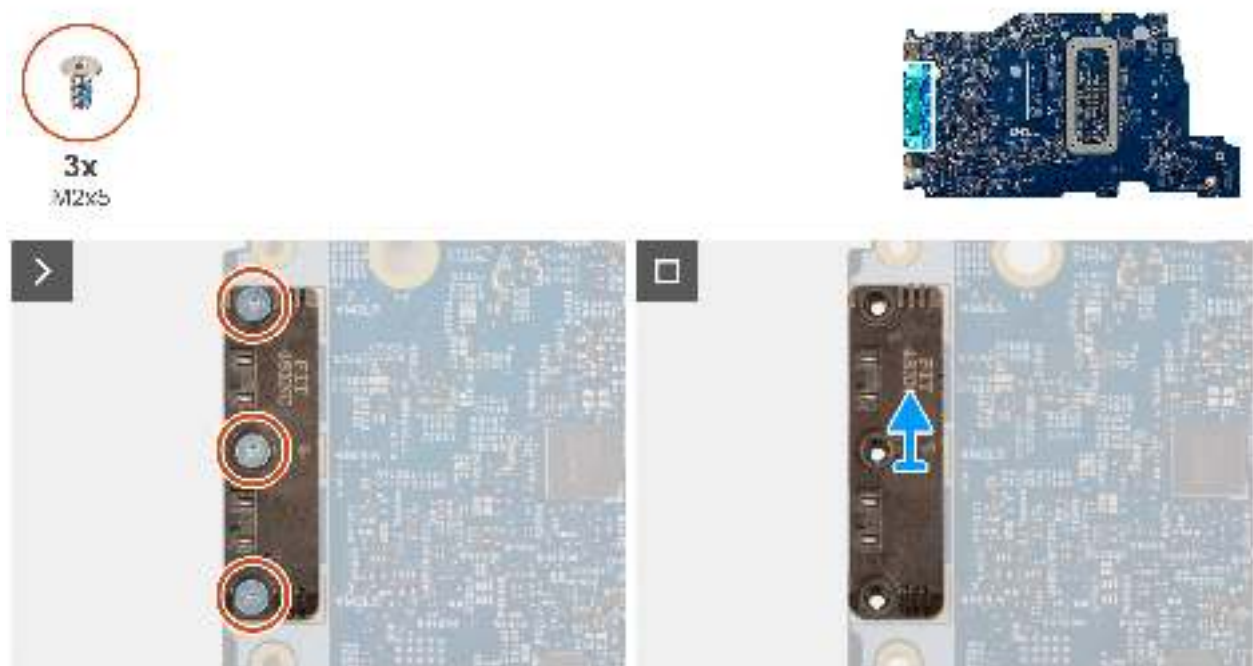
Abbildung 75. Entfernen des USB-Typ-C-Moduls
