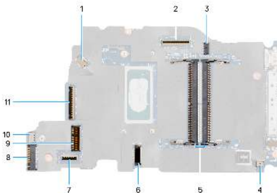
Abbildung 63. Hauptplattenanschlüsse
