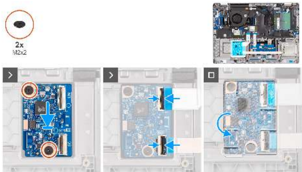
Abbildung 38. Einsetzen der USH-Platine
