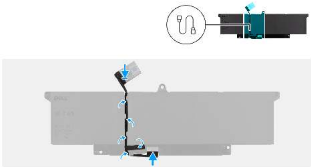
Abbildung 20. Einsetzen des Akkukabels
