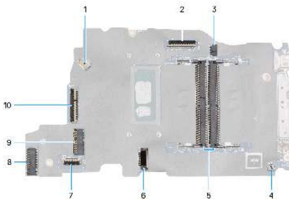
Abbildung 60. Hauptplatinenanschlüsse
