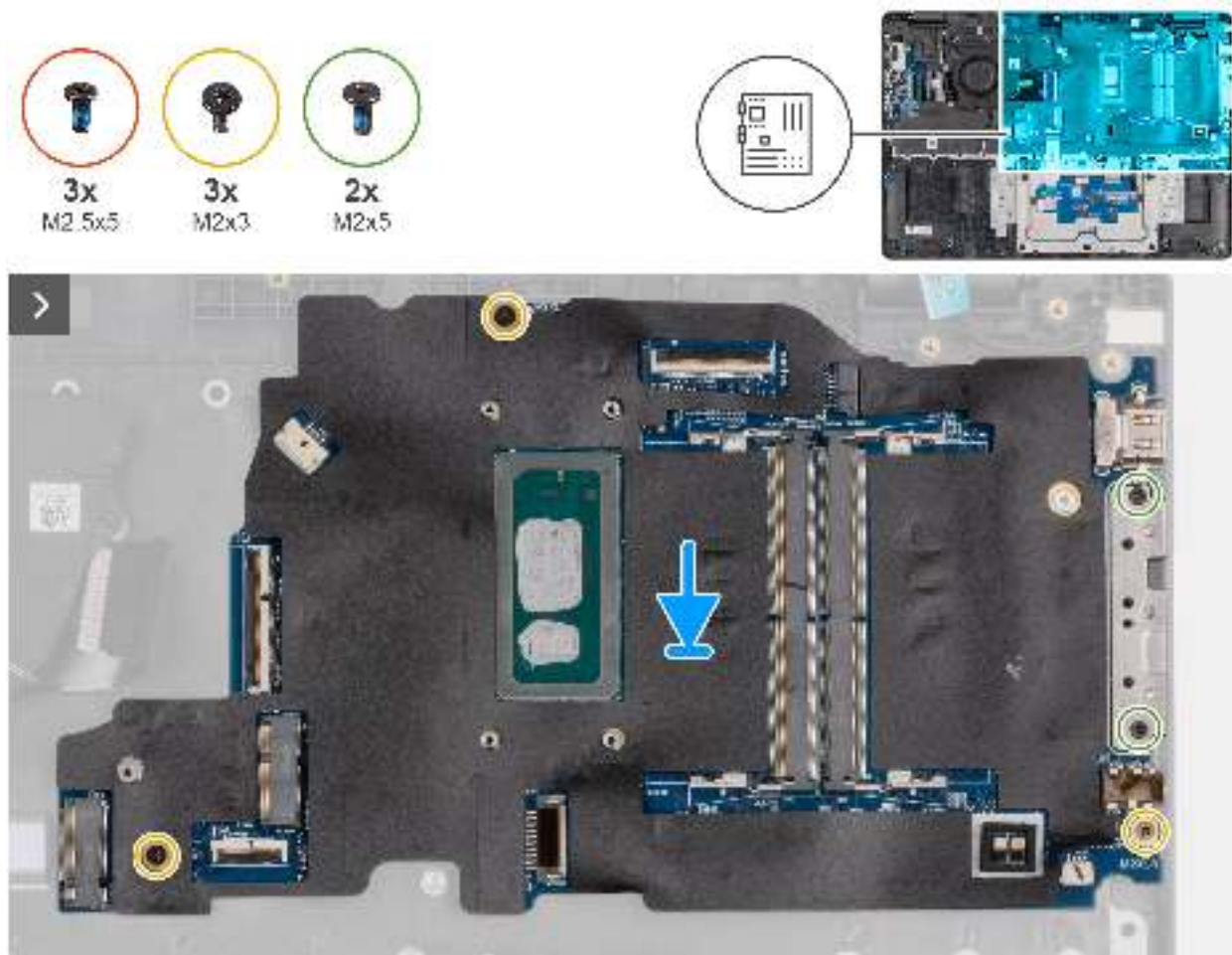
Abbildung 61. Einbauen der Systemplatine
