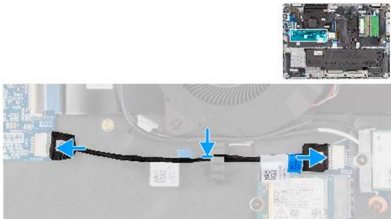
Abbildung 46. Einbauen des vPro-Kabels
