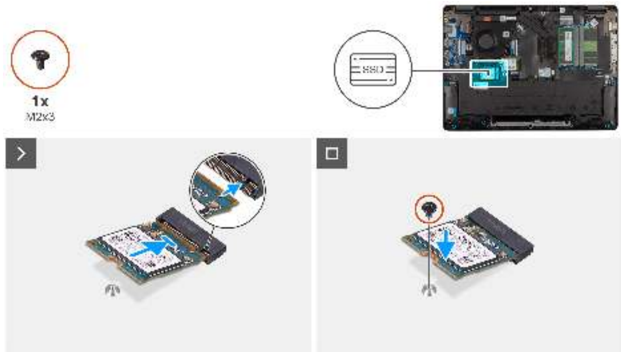
Abbildung 24. Einbauen der SSD-Karte
