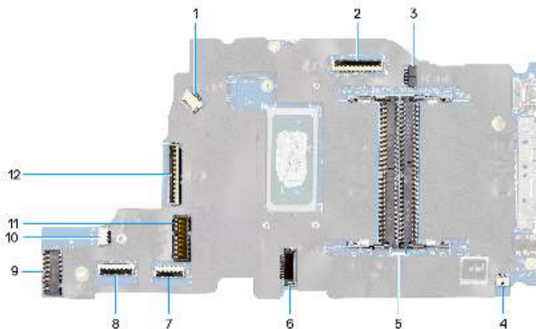
Abbildung 69. Hauptplattenanschlüsse
