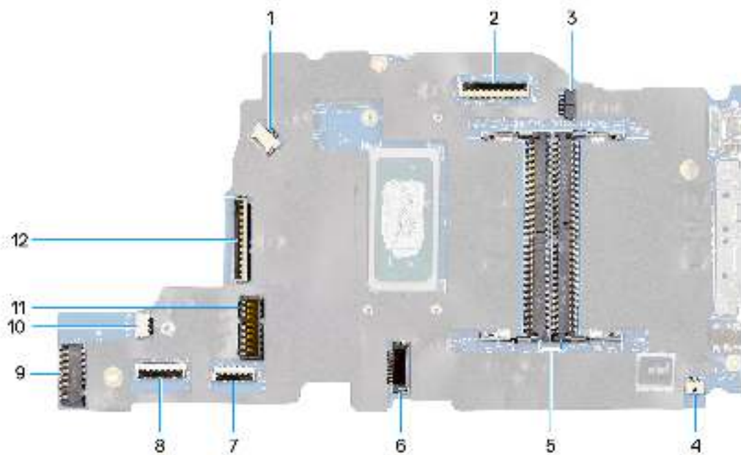
Abbildung 72. Hauptplatinenanschlüsse
