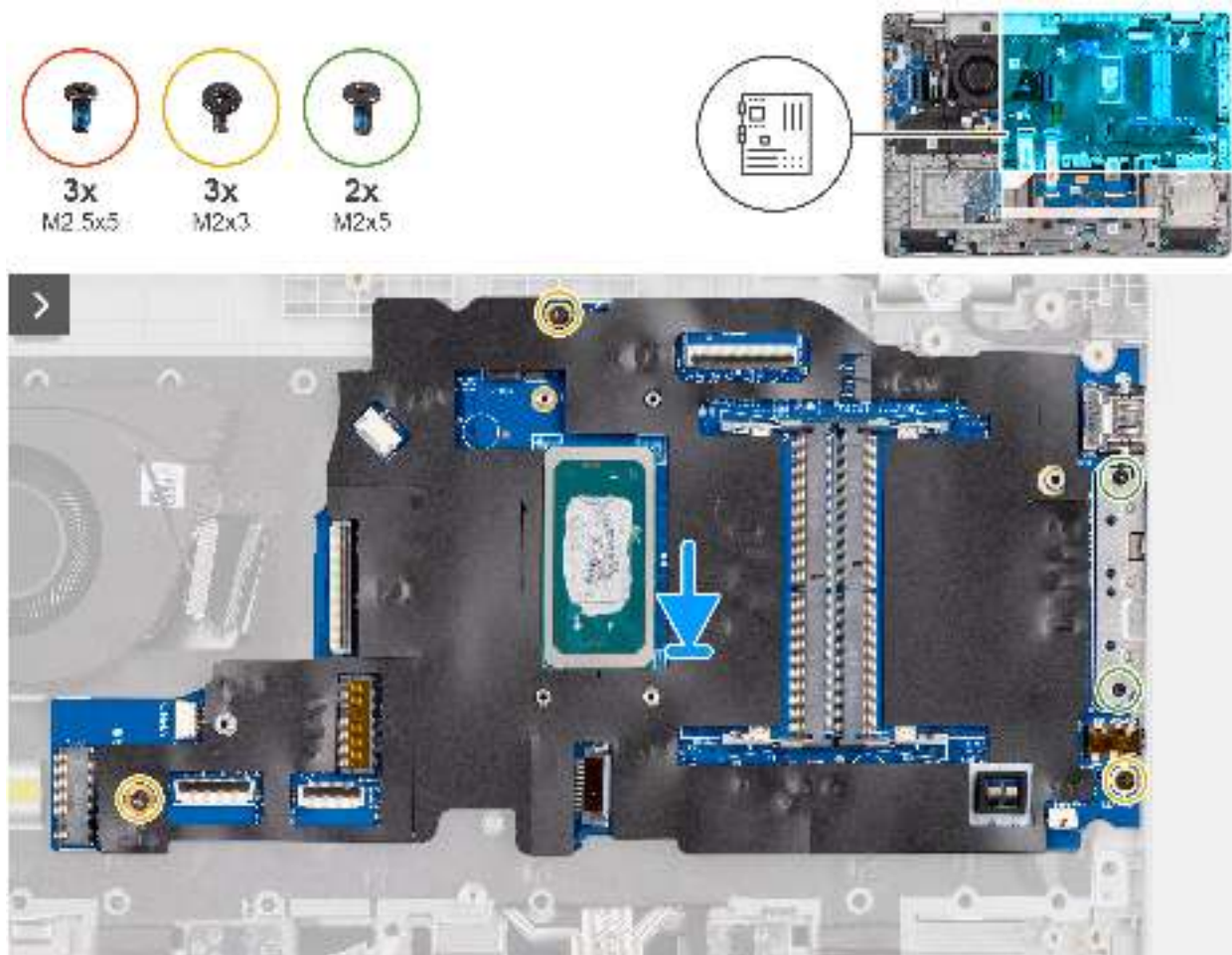
Abbildung 73. Einbauen der Systemplatine
