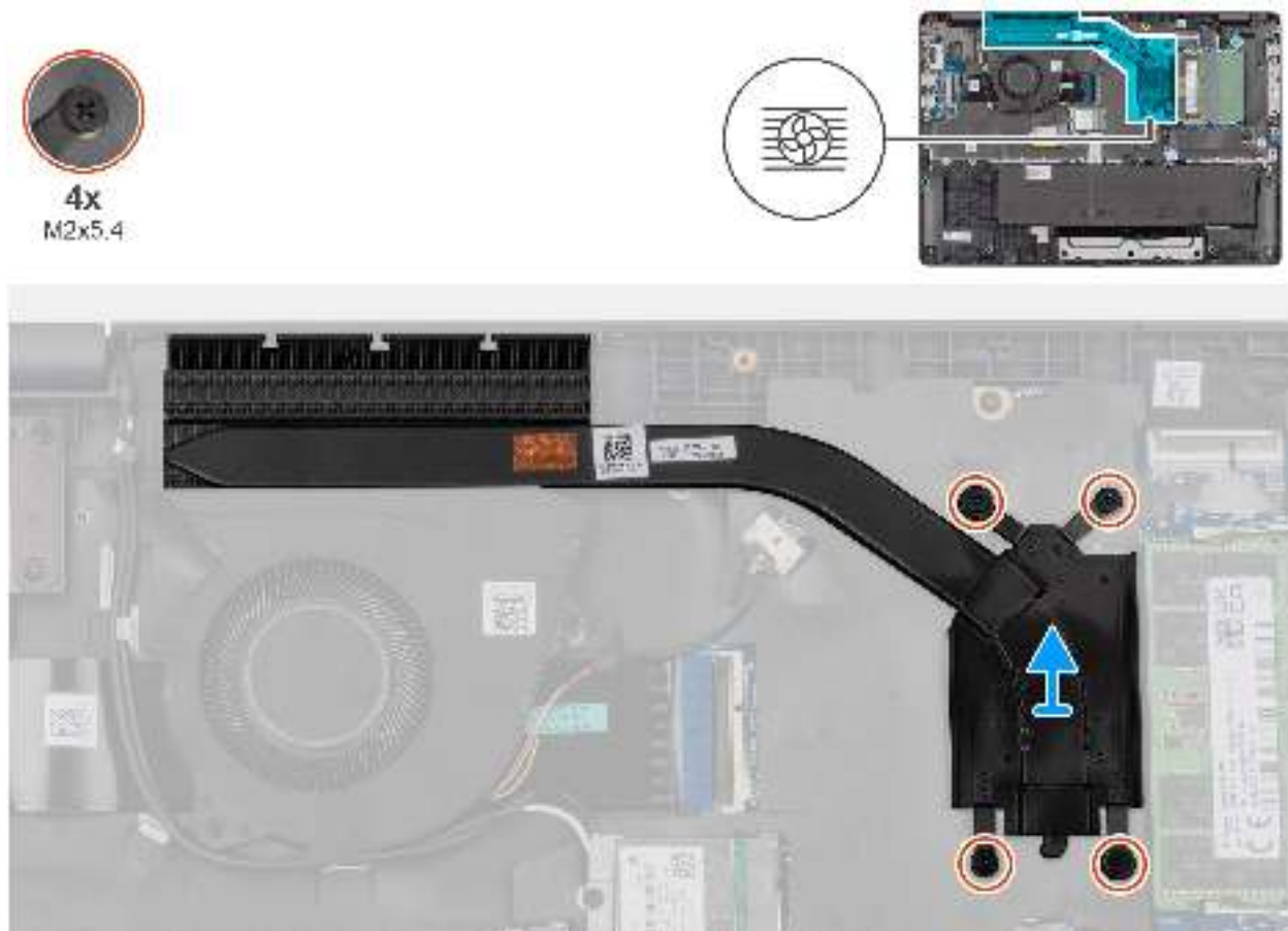
Abbildung 43. Kühlkörper entfernen
