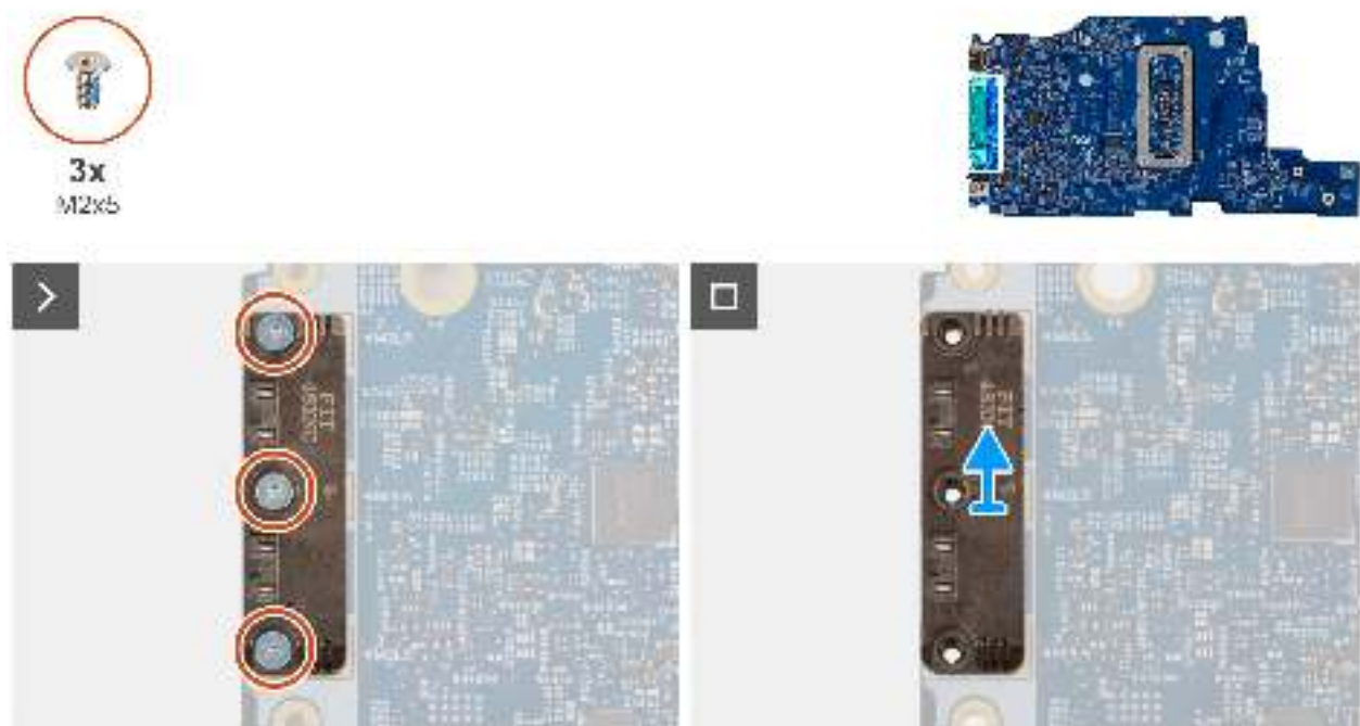
Abbildung 77. Entfernen des USB-Typ-C-Moduls
