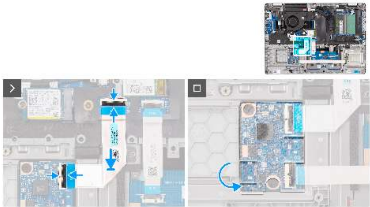
Abbildung 36. Einbauen des USH-Platinen-FPC
