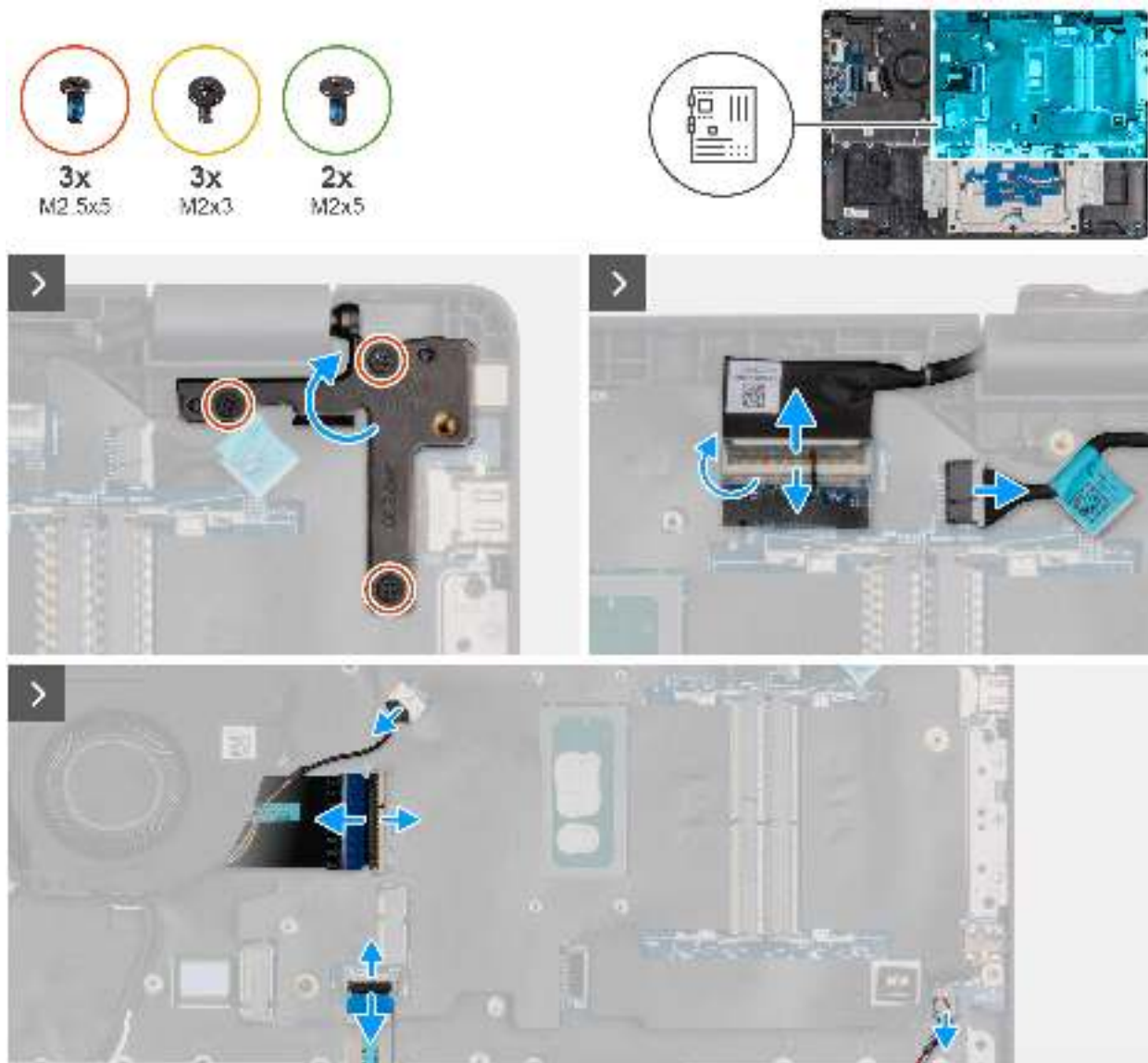
Abbildung 58. Entfernen der Systemplatine
