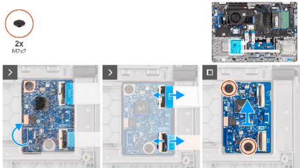
Abbildung 37. Entfernen der USH-Platine
