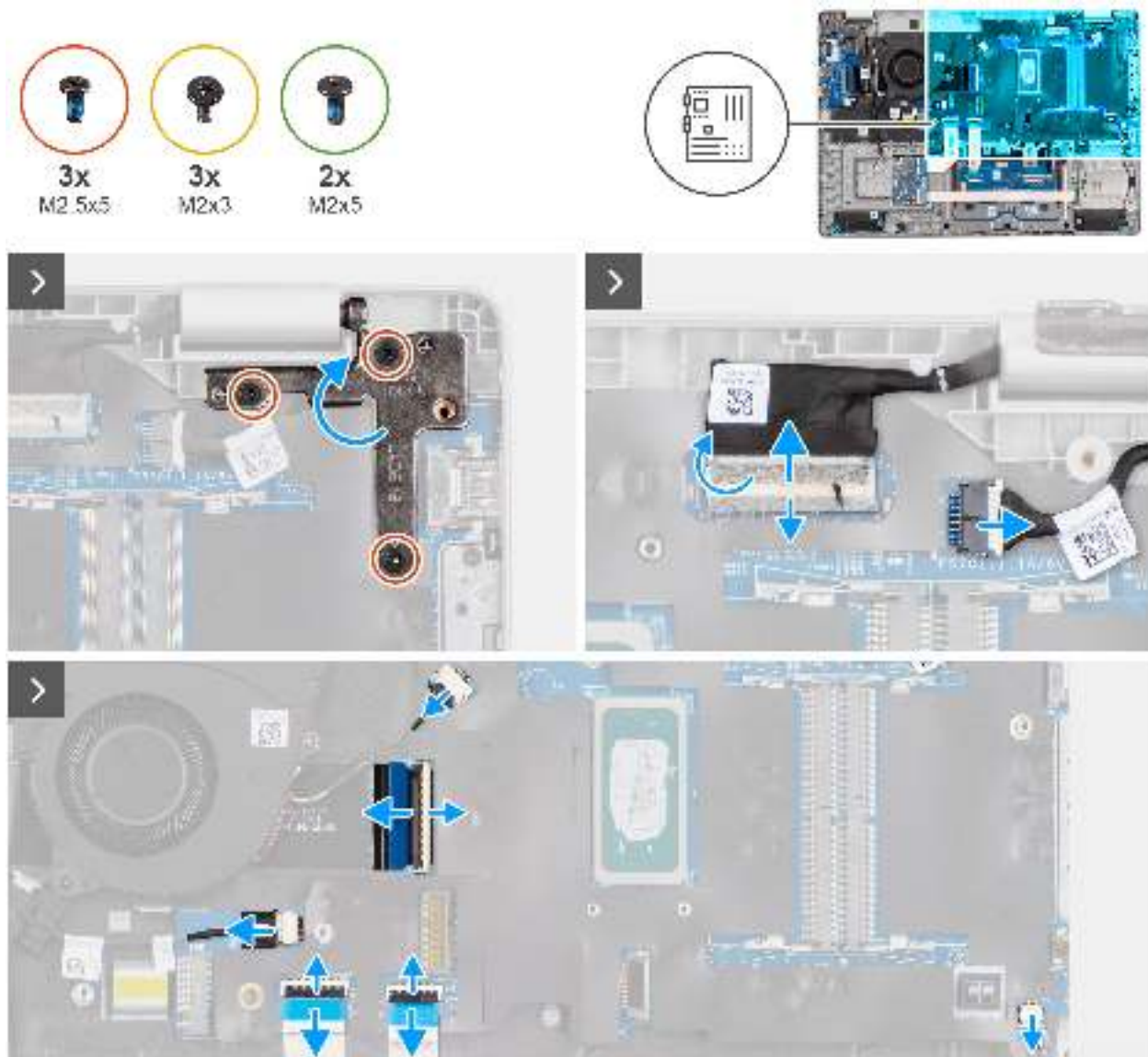
Abbildung 70. Entfernen der Systemplatte
