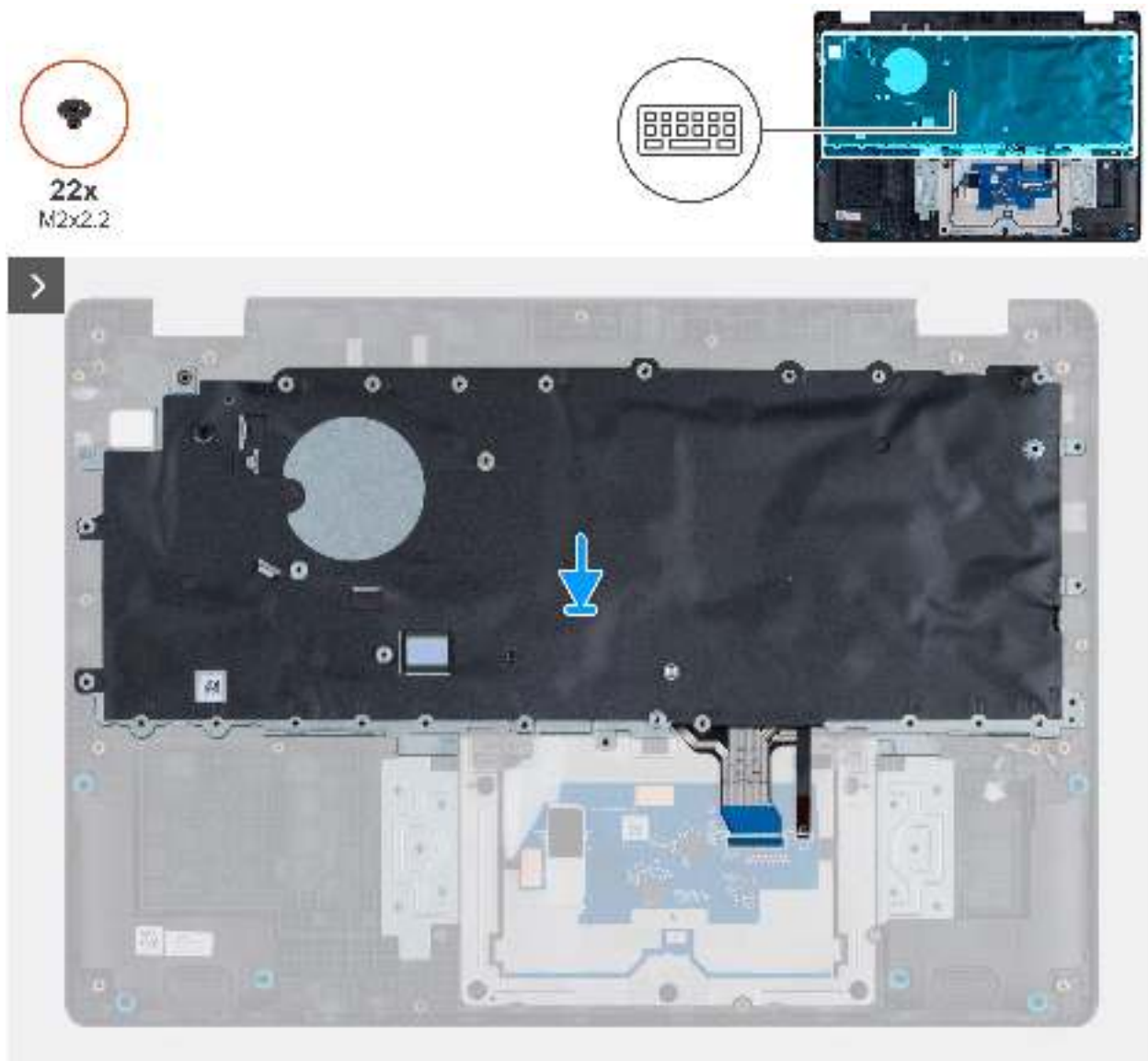
Abbildung 83. Einbauen der Tastatur
