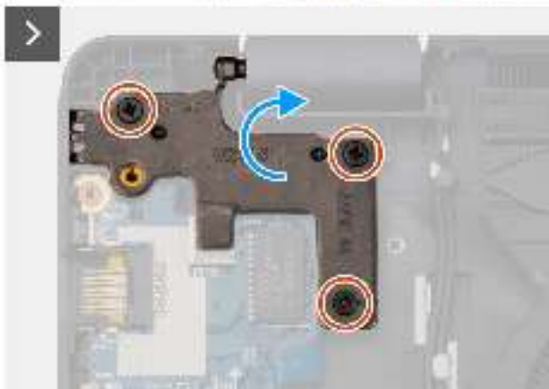
Abbildung 93. Entfernen der Bildschirmbaugruppe
