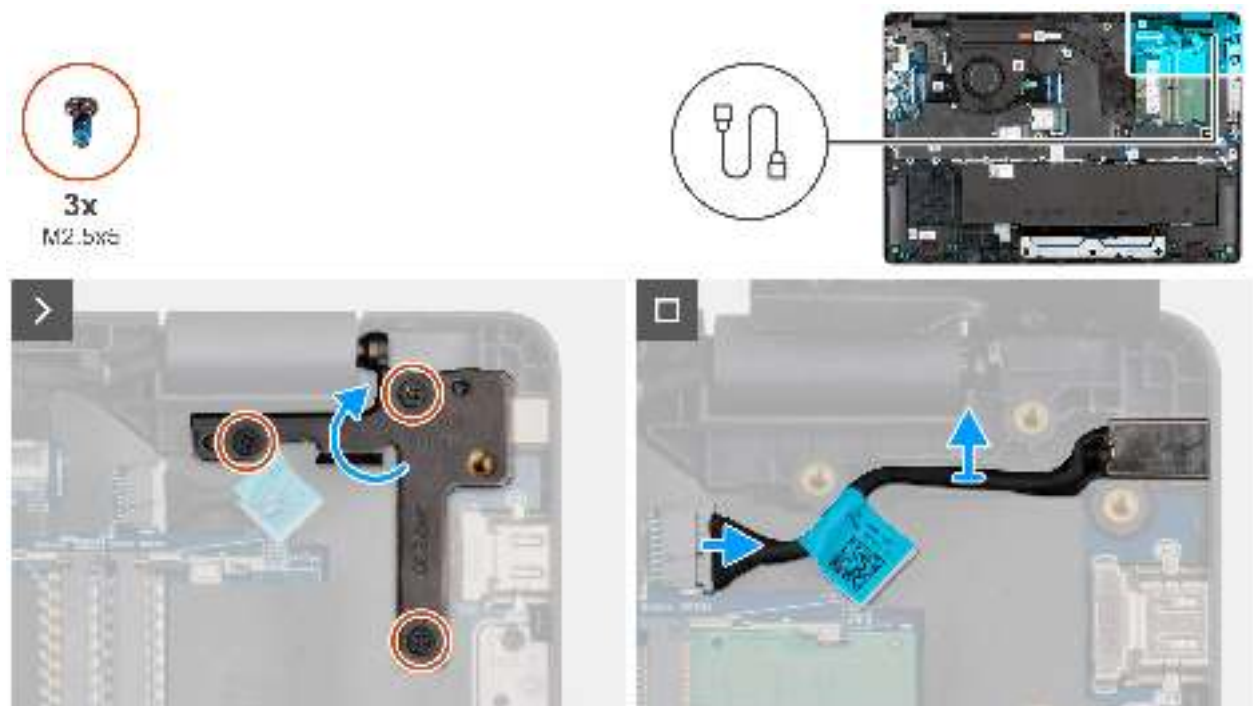
Abbildung 41. Entfernen des Netzadapteranschlusses
