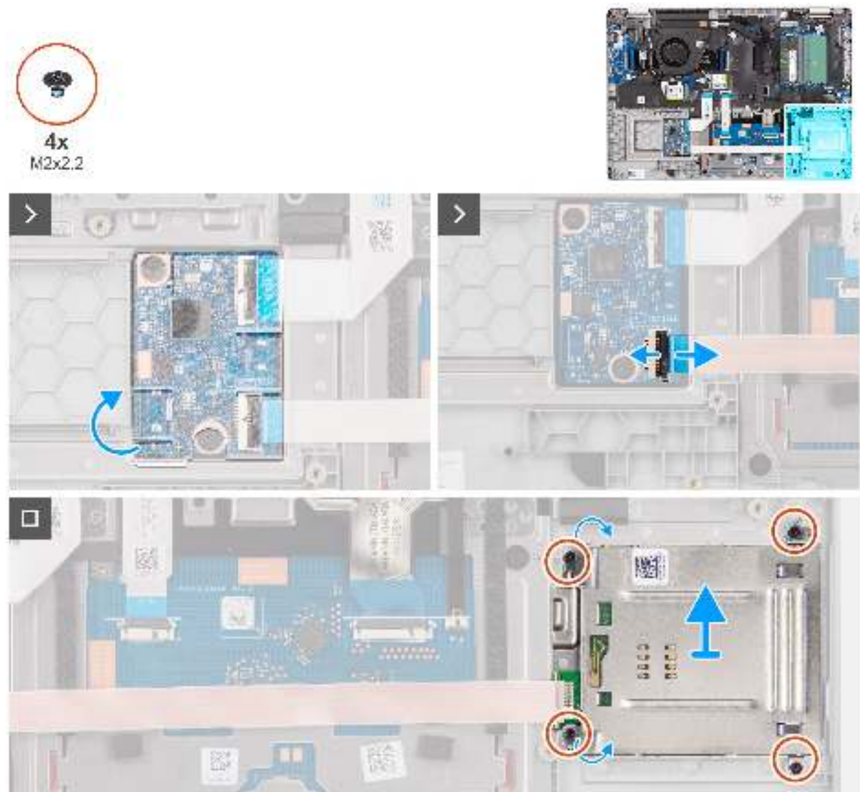
Abbildung 39. Entfernen des Smartcardlesegeräts
