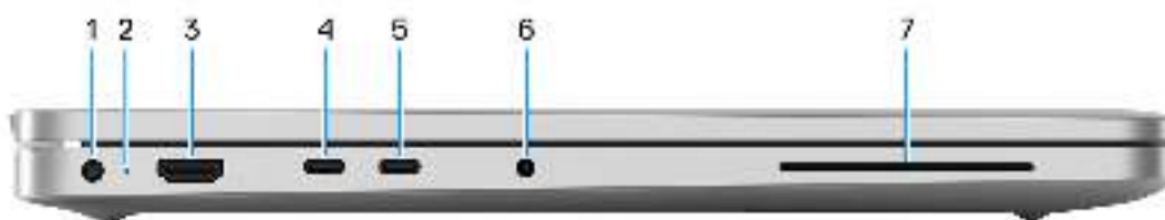
Abbildung 2. Linke Seitenansicht
