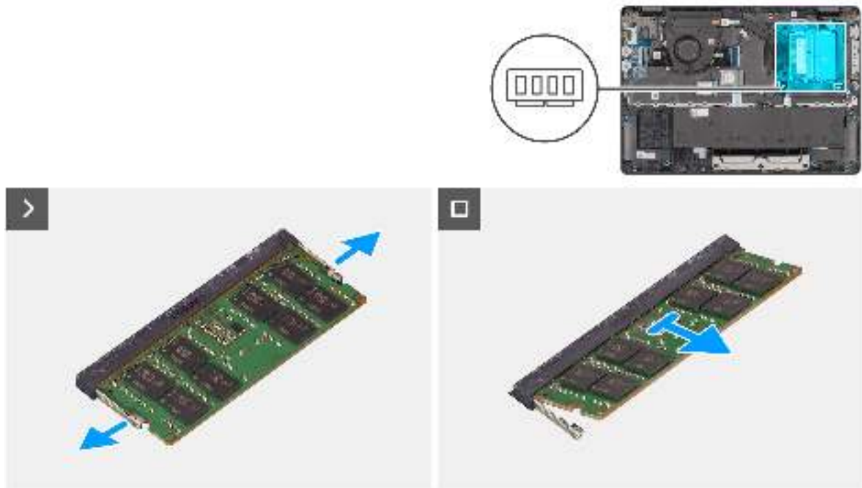
Abbildung 21. Entfernen des Arbeitsspeichersmoduls
