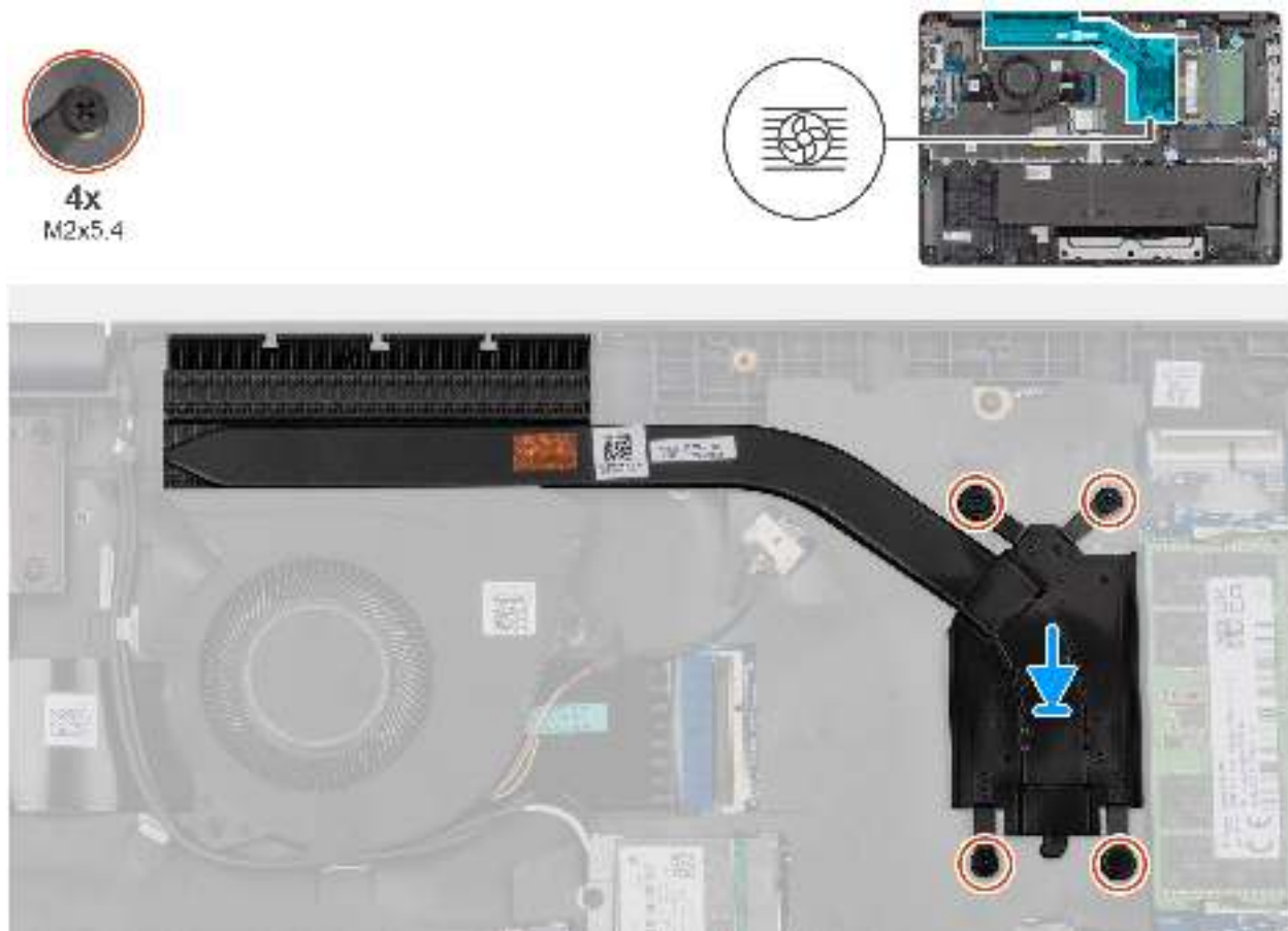
Abbildung 44. Einsetzen des Kühlkörpers
