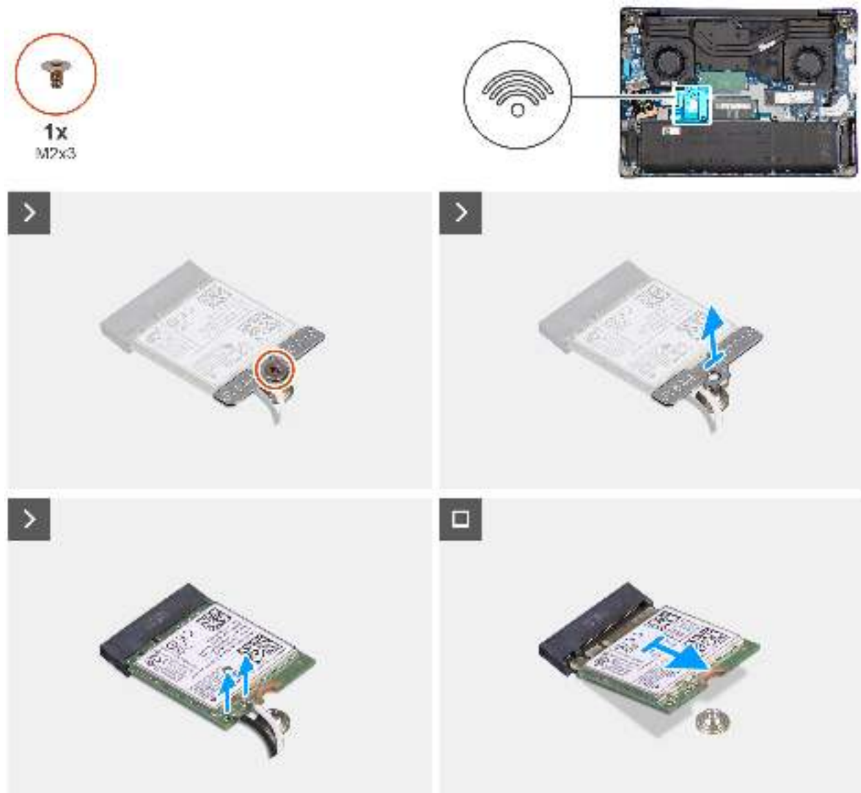
Abbildung 27. Entfernen der Wireless-Karte
