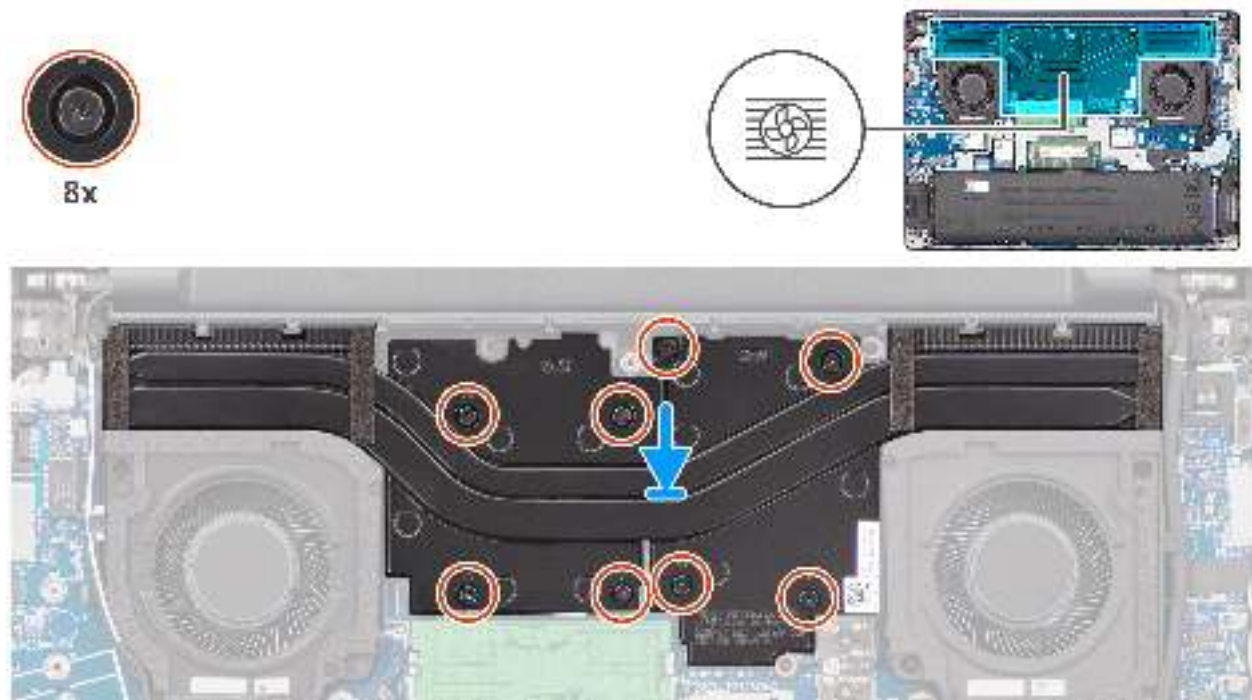
Abbildung 43. Einsetzen des Kühlkörpers
