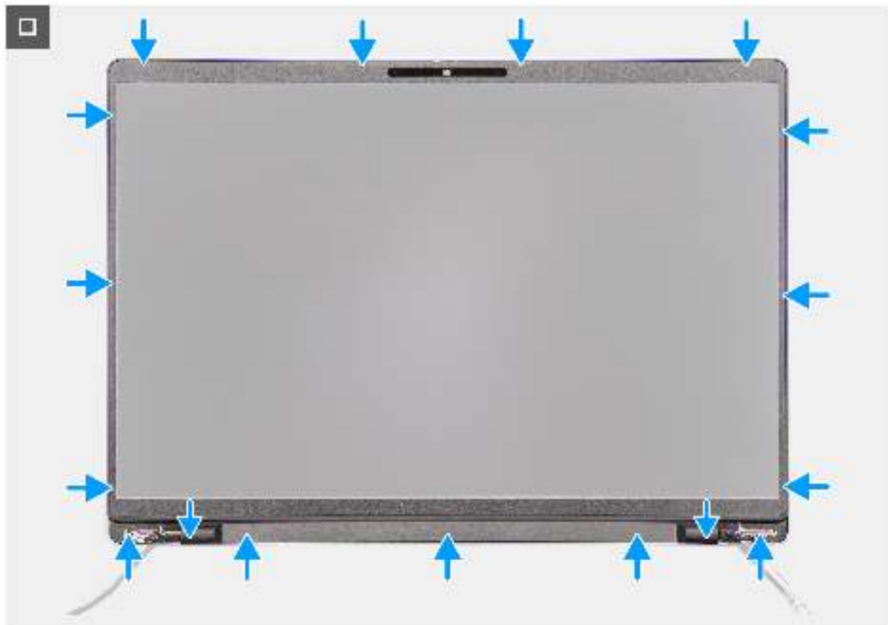
Abbildung 67. Einbauen der Bildschirmblende
