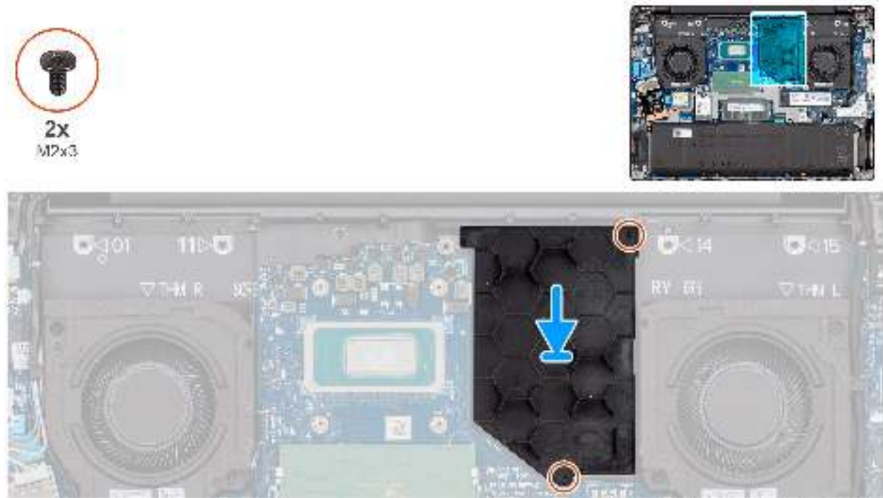
Abbildung 45. Installieren des GPU-Kartenplatzhalters
