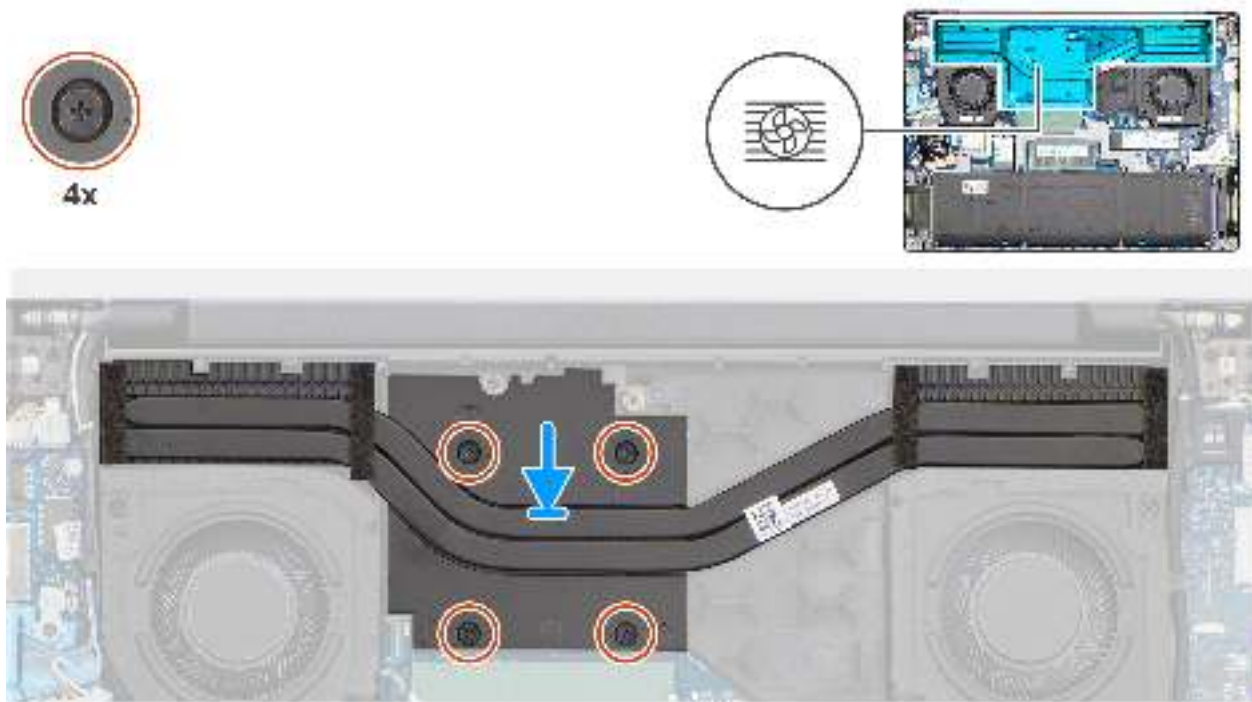
Abbildung 41. Einsetzen des Kühlkörpers
