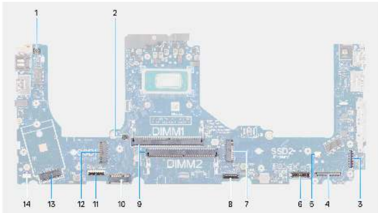
Abbildung 85. Anschlüsse auf der Hauptplatine
