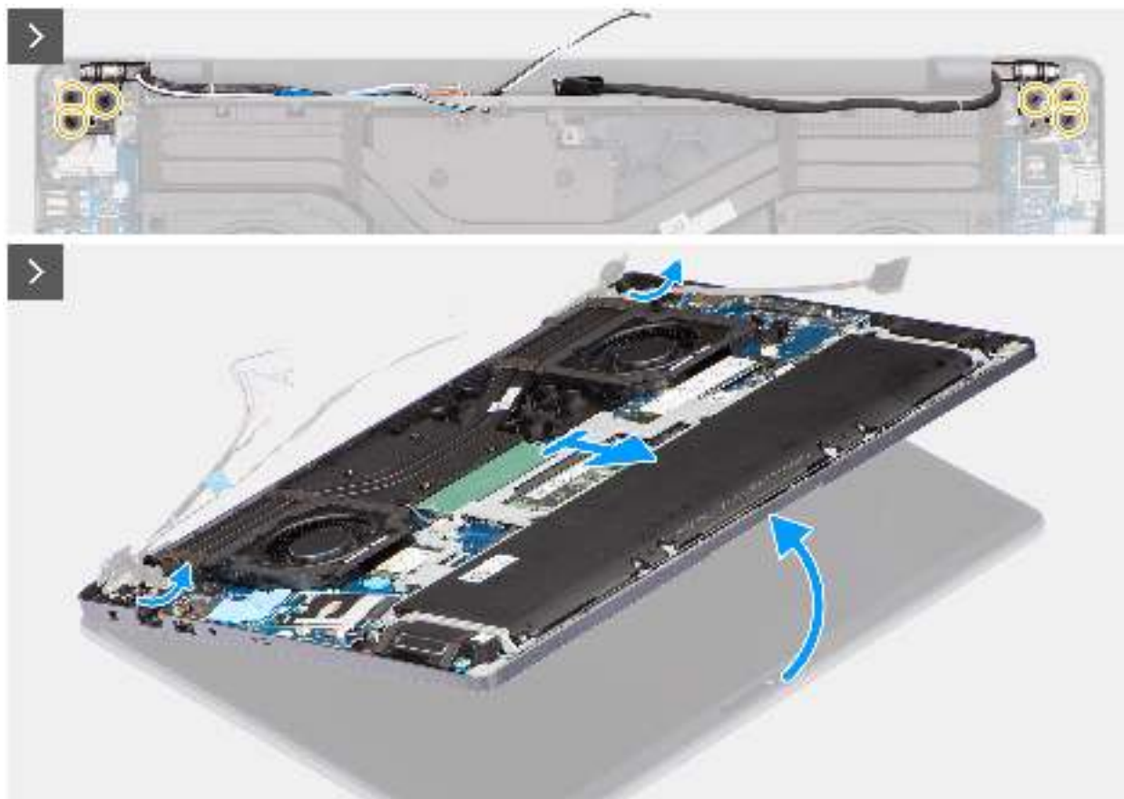
Abbildung 55. Entfernen der Bildschirmbaugruppe
