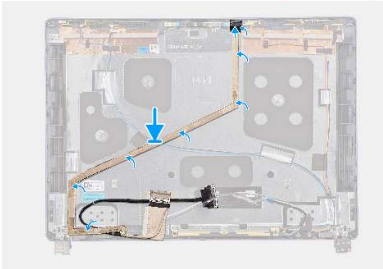
Abbildung 77. Einbauen des Bildschirmkabels
