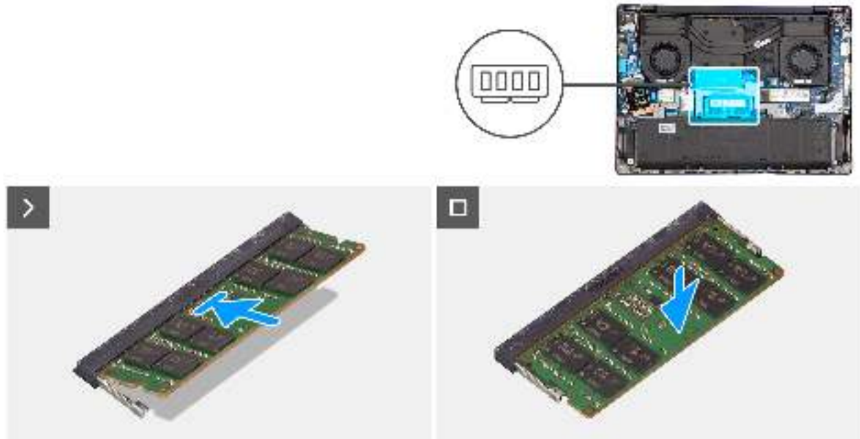
Abbildung 22. Einsetzen des Speichermoduls
