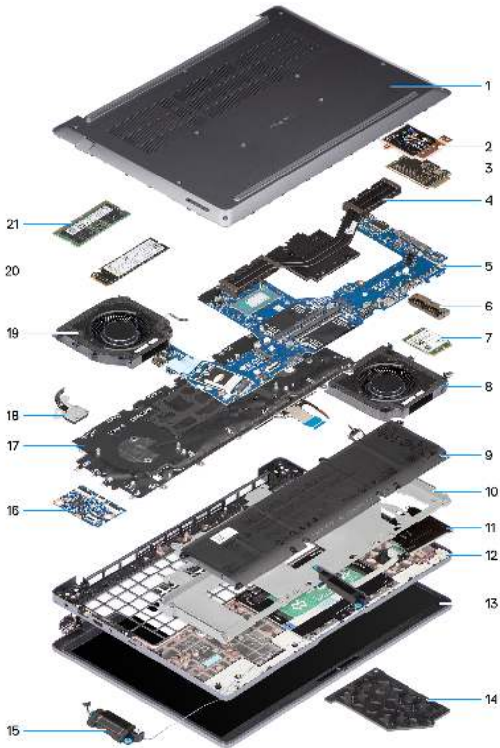
Abbildung 11. Hauptkomponenten des Dell Pro Max 16 MC16250
