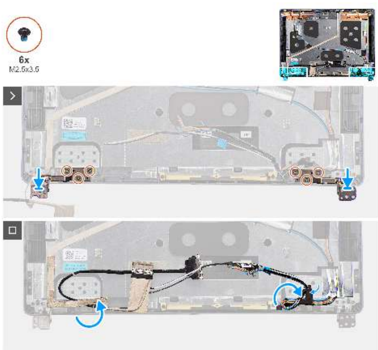
Abbildung 75. Einbauen der Bildschirmscharniere
