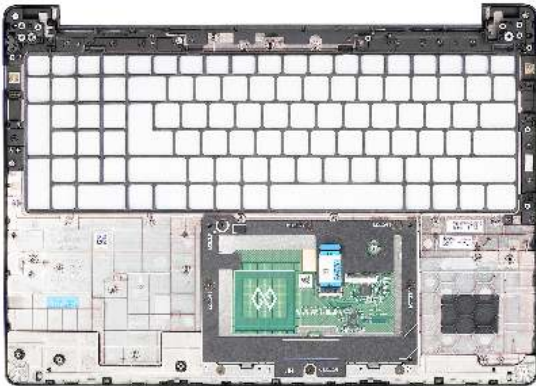
Abbildung 103. Handauflagenbaugruppe
