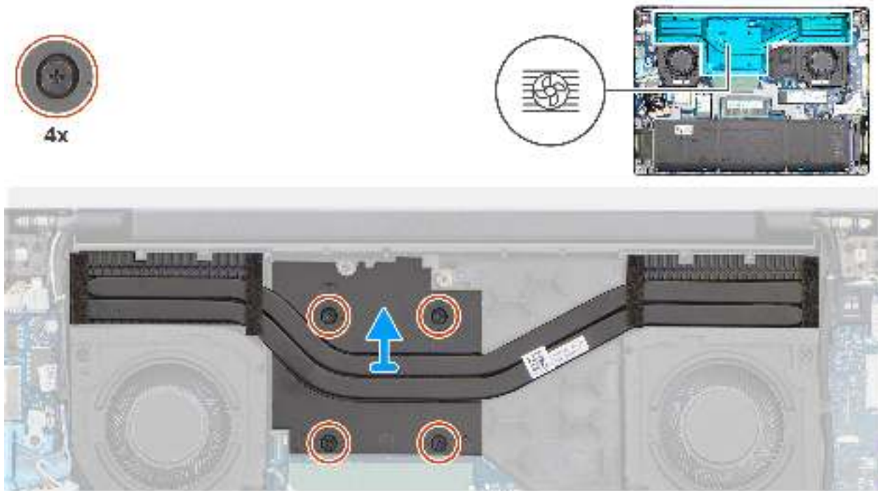
Abbildung 40. Kühlkörper entfernen
