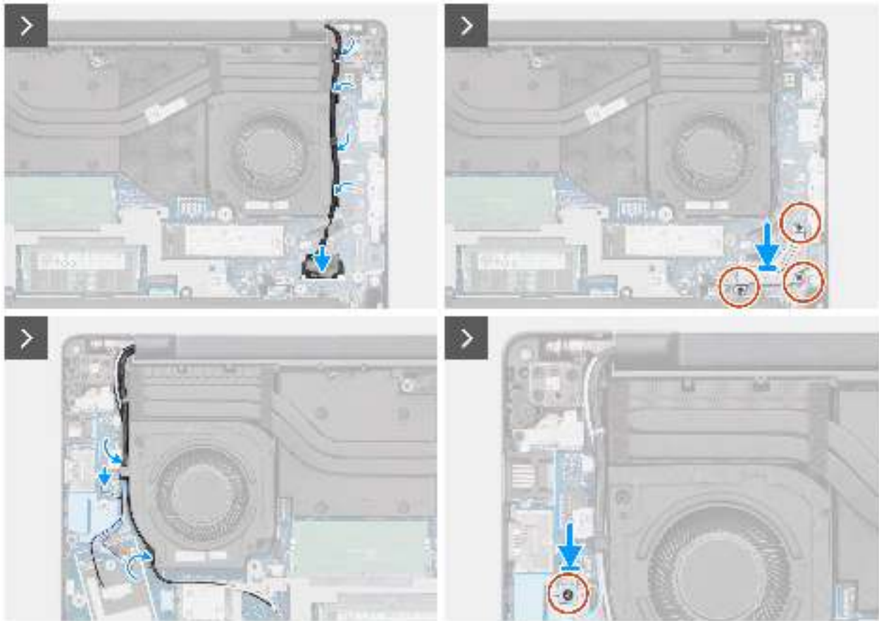
Abbildung 59. Einbauen der Bildschirmbaugruppe
