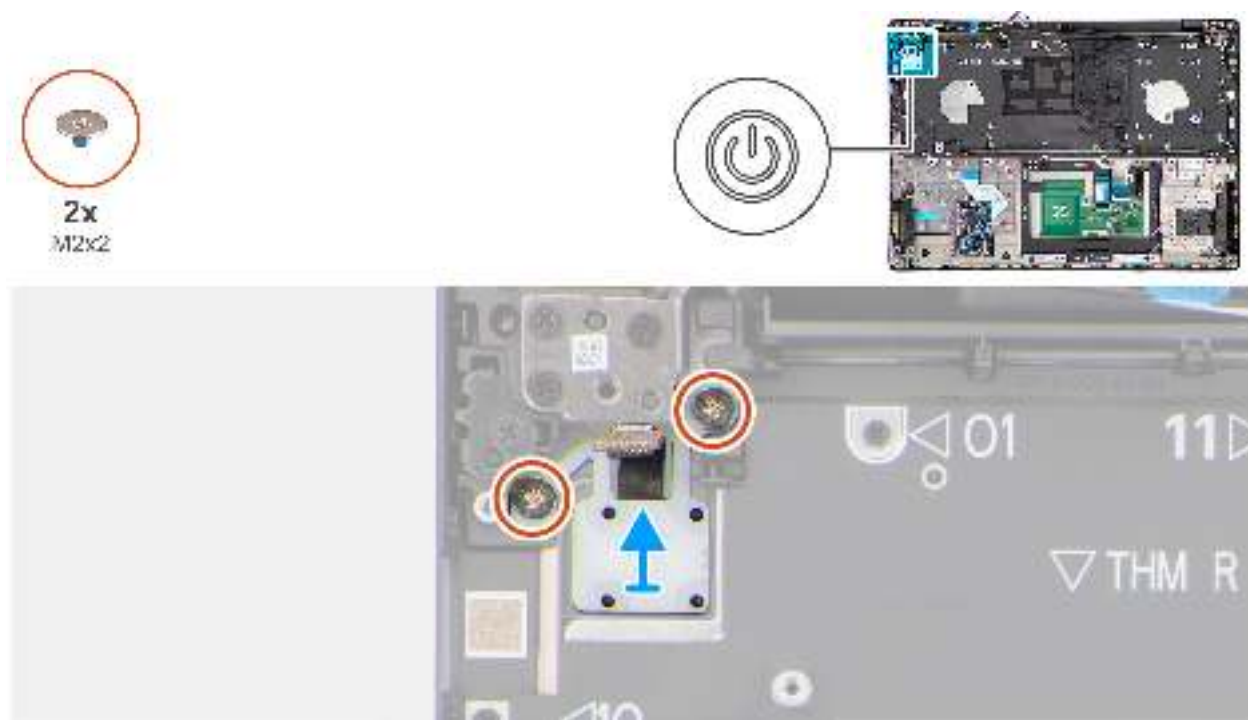
Abbildung 96. Entfernen des Netzschalters
