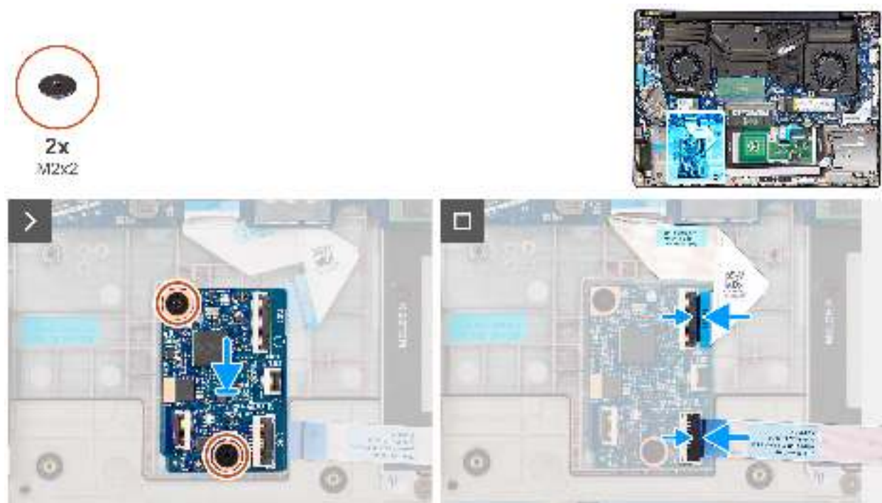
Abbildung 51. Einsetzen der USH-Platine
