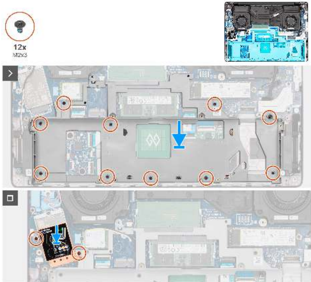
Abbildung 49. Einsetzen des Akkurahmens
