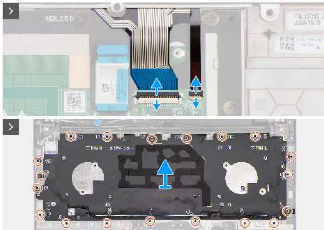
Abbildung 98. Entfernen der Tastatur
