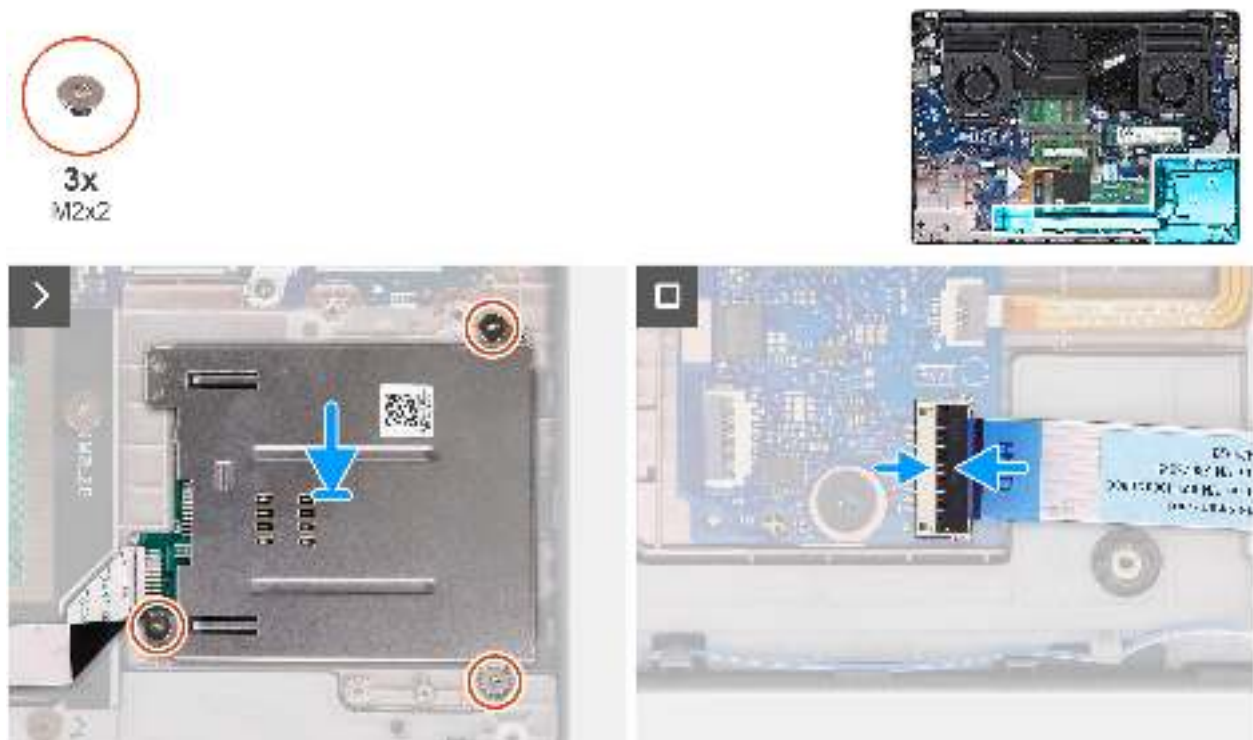
Abbildung 53. Installieren des Smartcardlesegeräts
