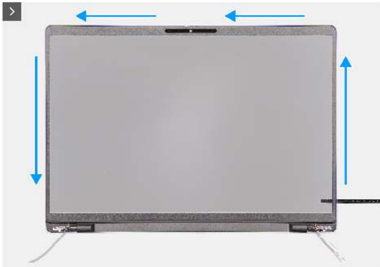
Abbildung 62. Entfernen der Bildschirmblende
