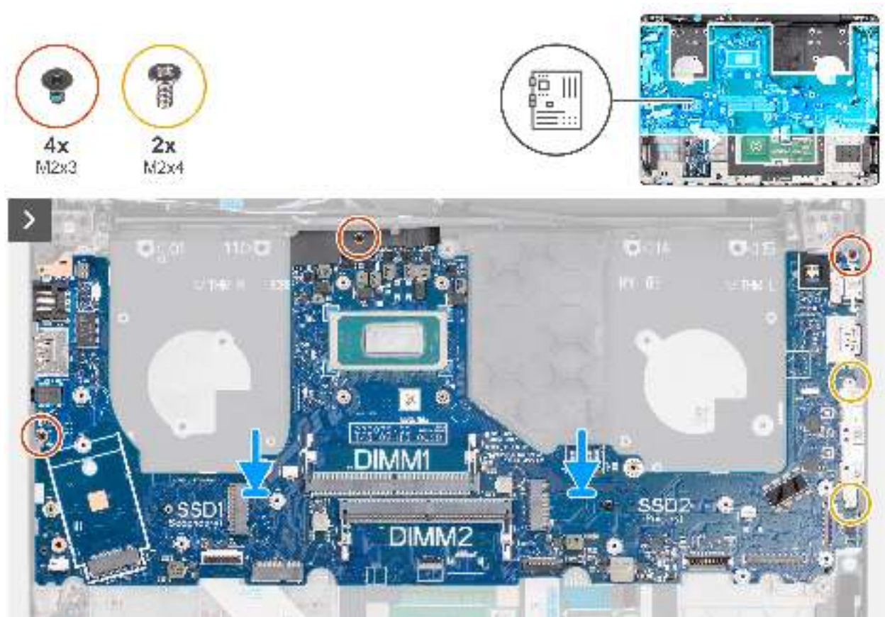
Abbildung 86. Einbauen der Systemplatine
