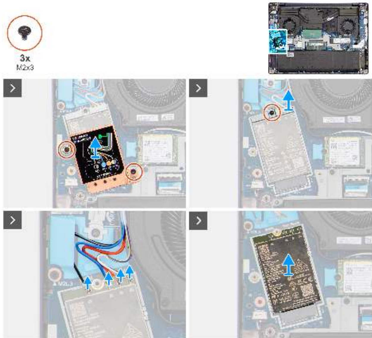
Abbildung 29. Entfernen des WWAN-Moduls
