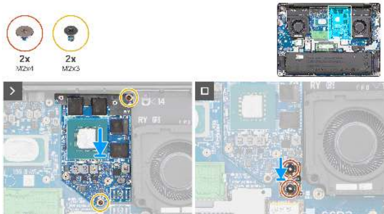
Abbildung 47. Einsetzen der GPU
