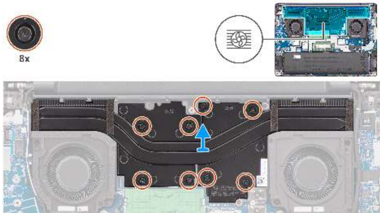
Abbildung 42. Kühlkörper entfernen
