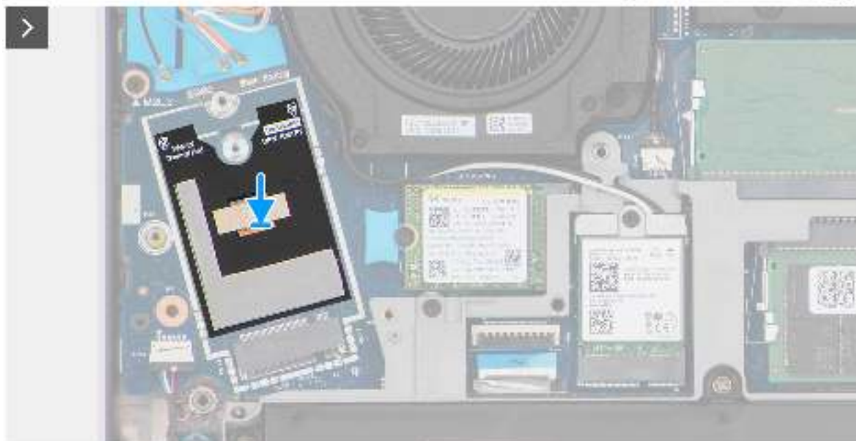
Abbildung 31. Installieren des WWAN-Moduls
