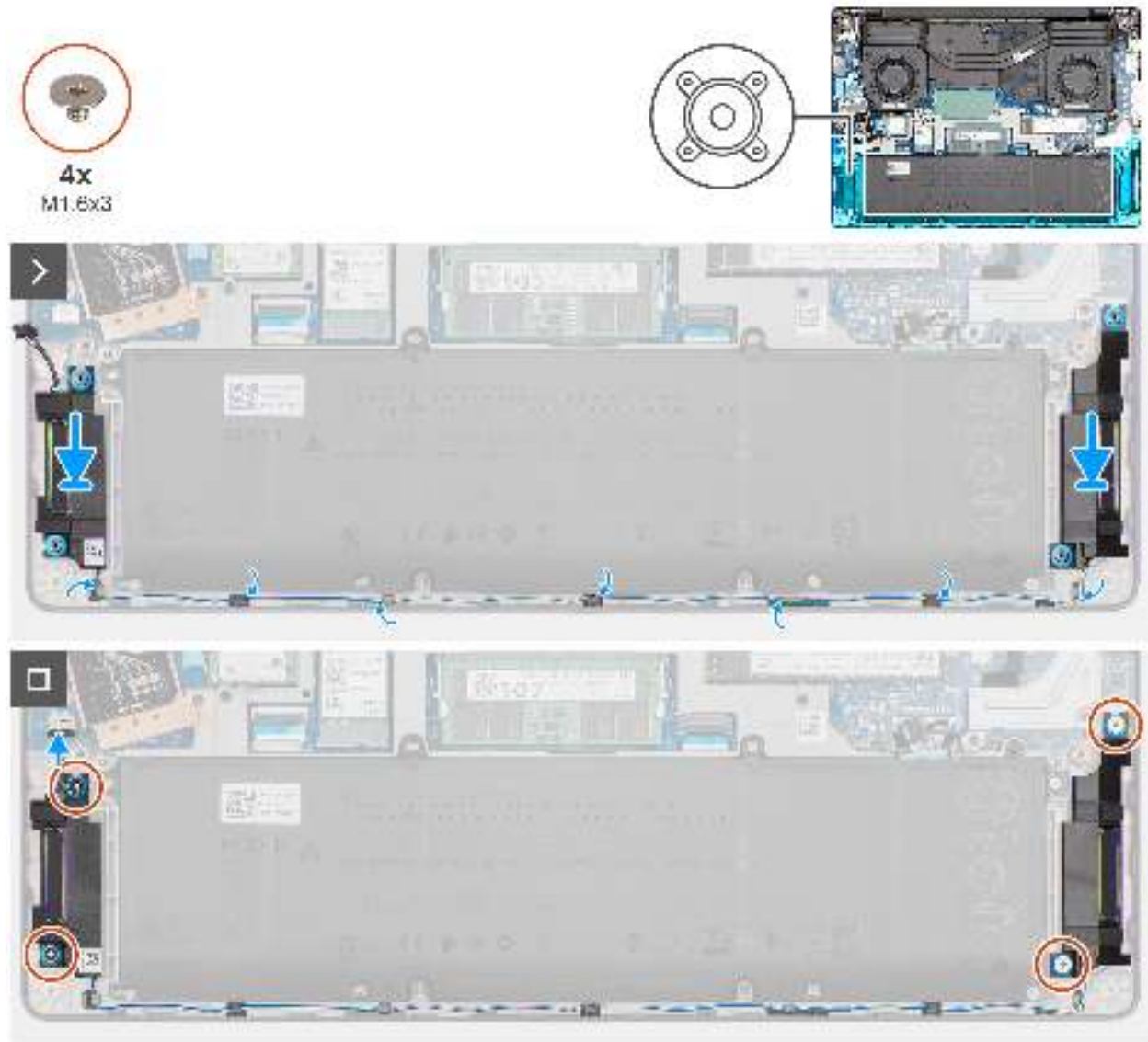
Abbildung 34. Installieren der Lautsprecher
