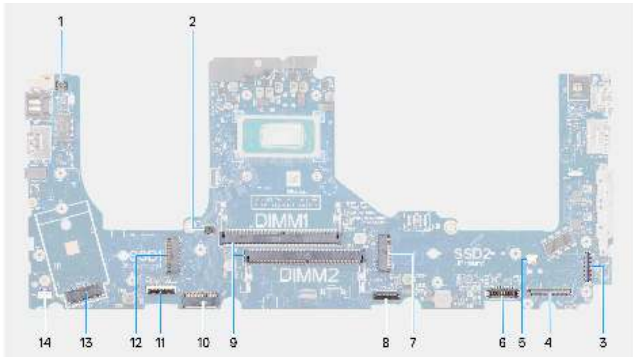
Abbildung 82. Anschlüsse auf der Hauptplatine
