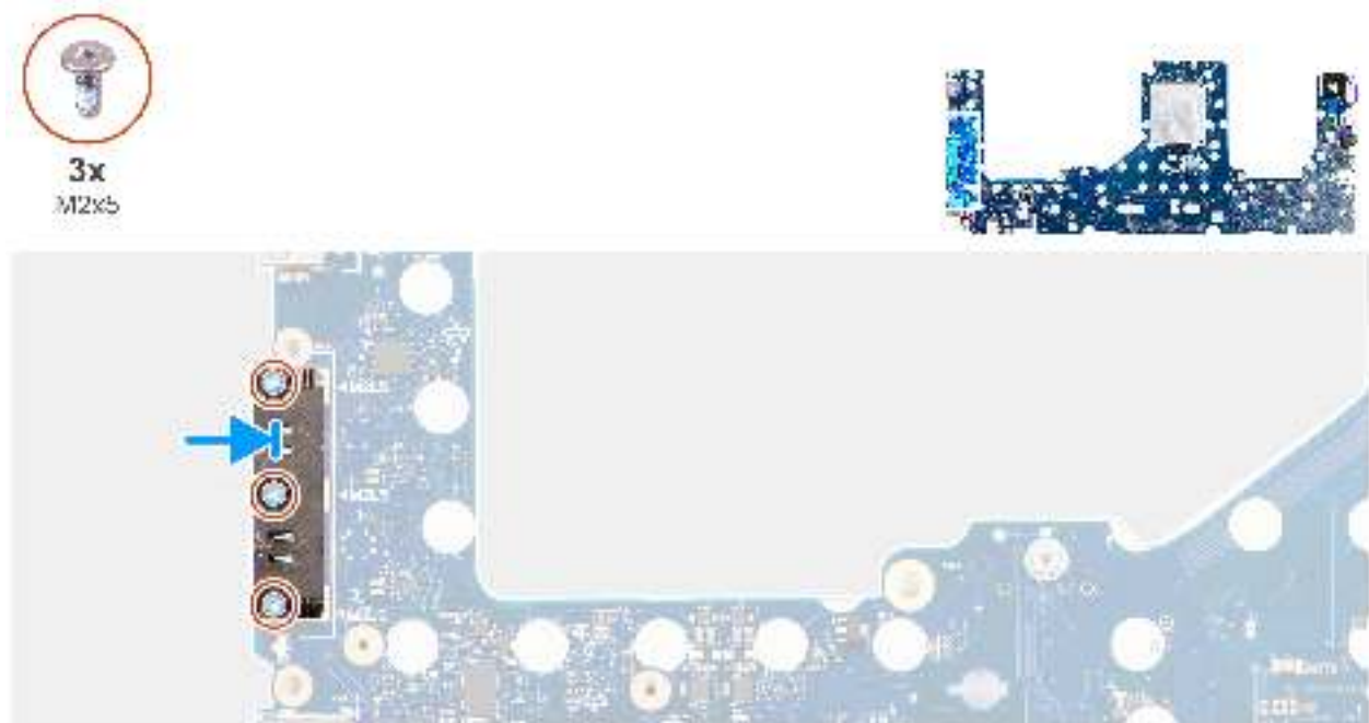
Abbildung 95. Installieren des USB-Typ-C-Moduls
