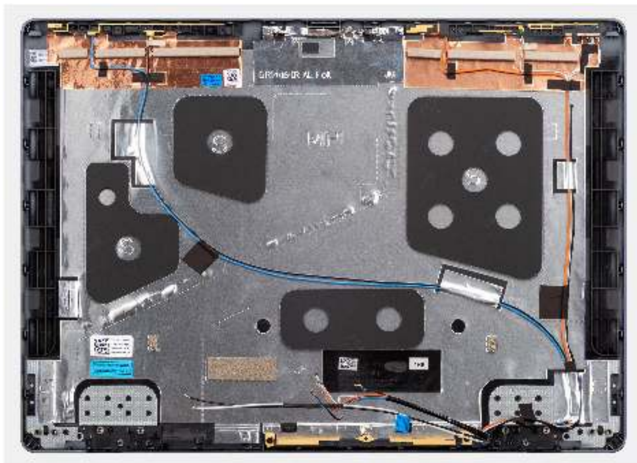
Abbildung 81. Bildschirmrückwand-Antennen-Baugruppe
