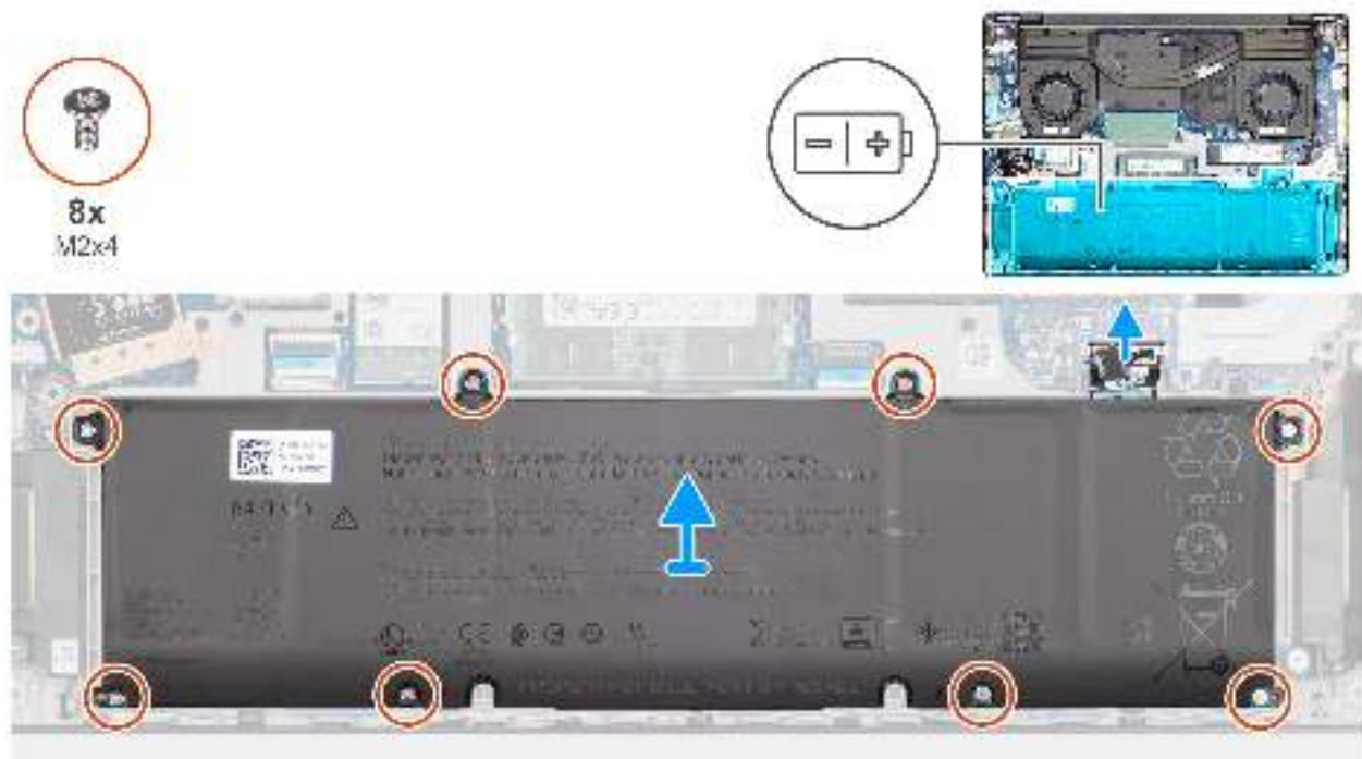
Abbildung 17. Entfernen des Akkus
