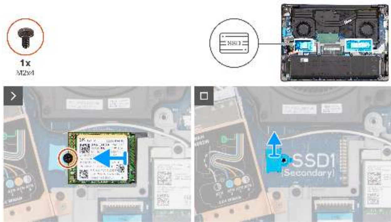
Abbildung 23. Entfernen des M.2-2230-Solid-State-Laufwerks
