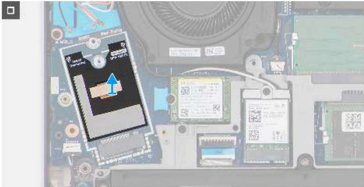
Abbildung 30. Entfernen des WWAN-Moduls
