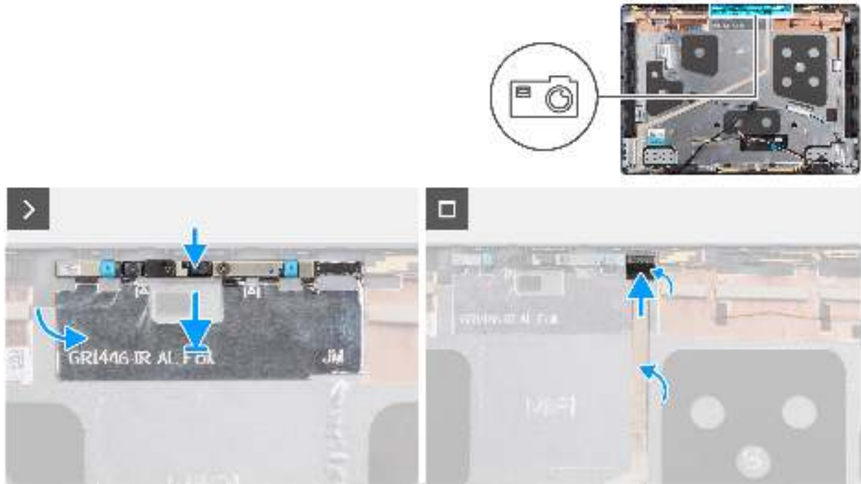
Abbildung 79. Installieren der Kamera
