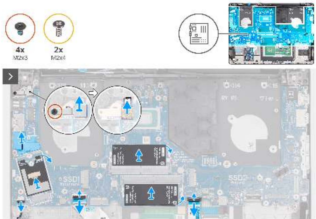
Abbildung 83. Entfernen der Systemplatine
