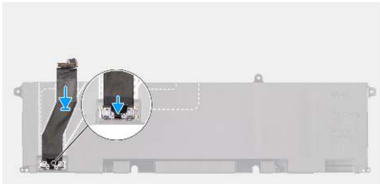
Abbildung 20. Verbinden des Akkukabels
