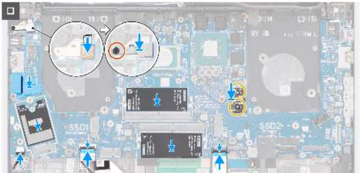
Abbildung 93. Einbauen der Systemplatine
