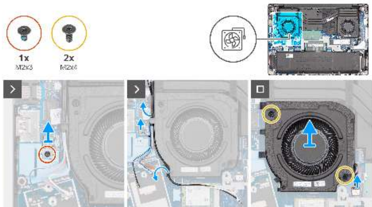
Abbildung 36. Entfernen des rechten/Prozessorlüfters
