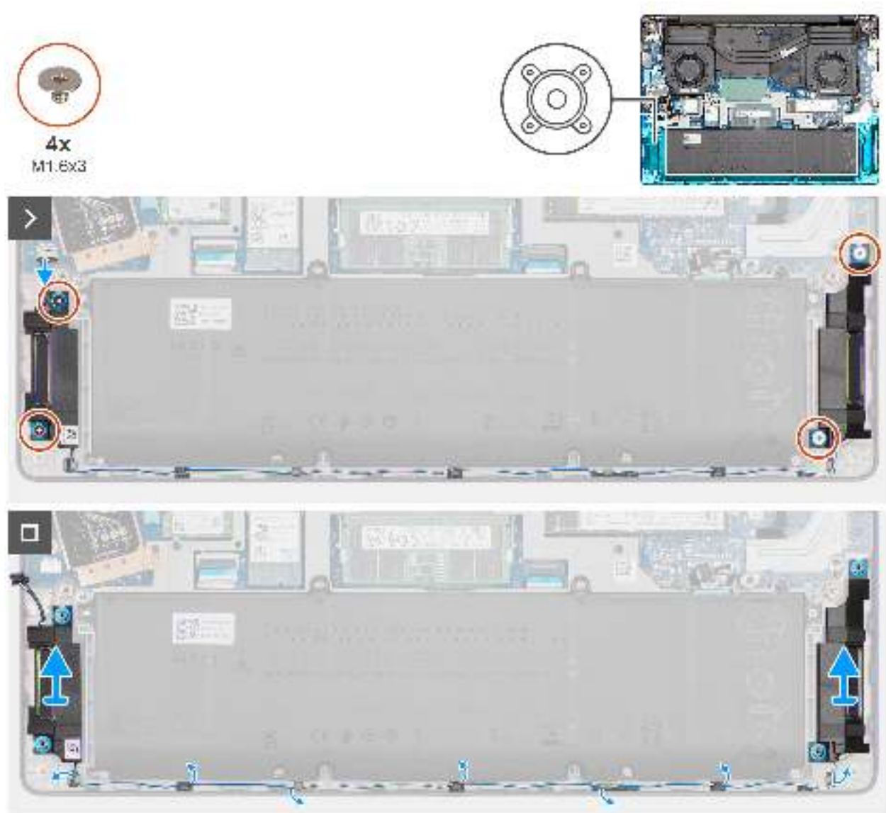
Abbildung 33. Entfernen der Lautsprecher
