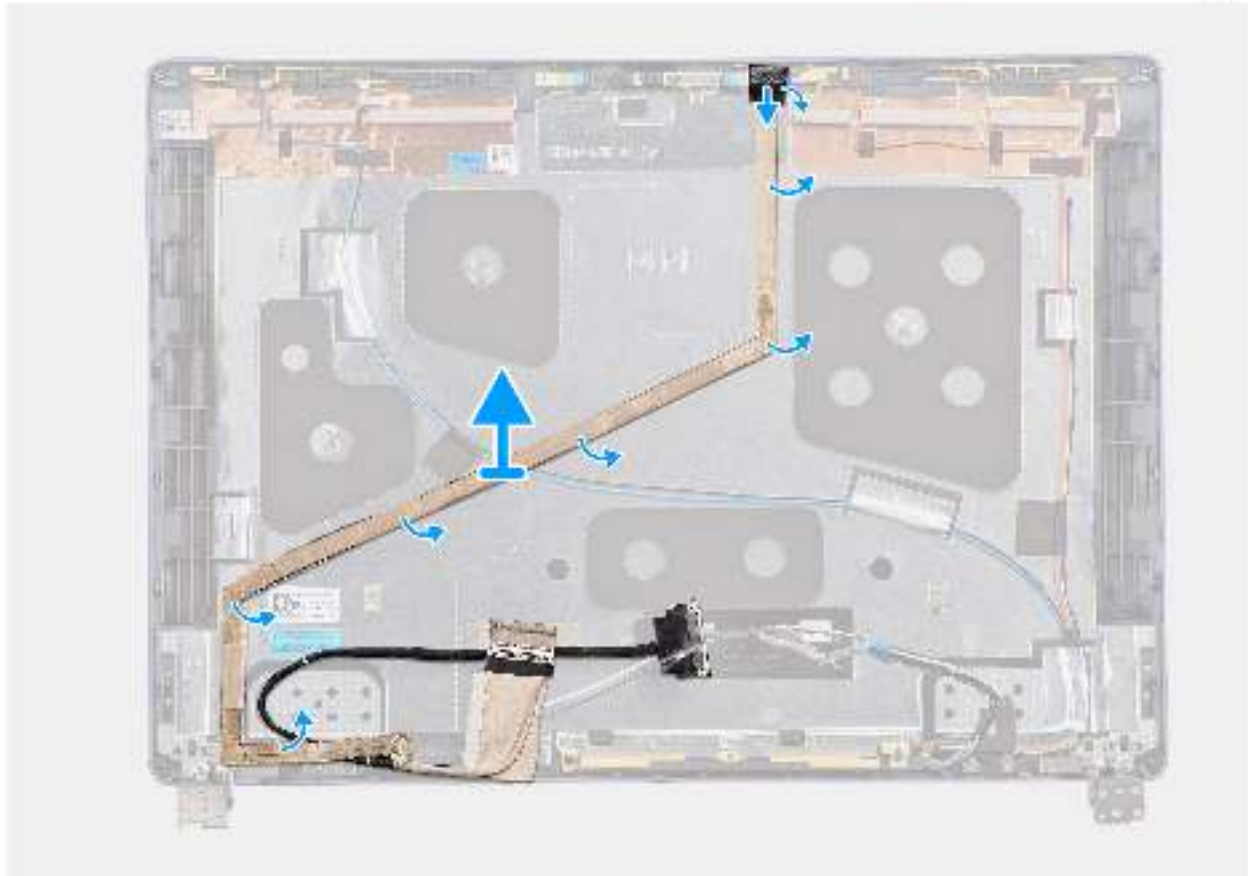
Abbildung 76. Entfernen des Bildschirmkabels
