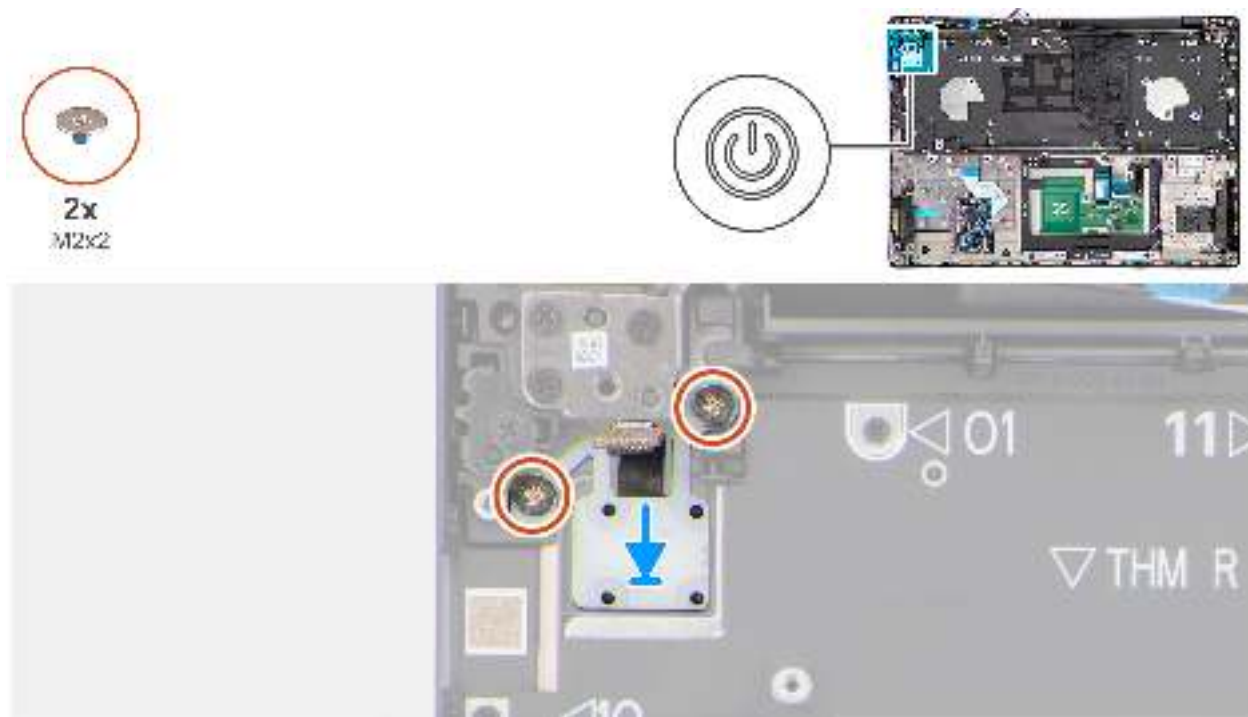
Abbildung 97. Installieren des Netzschalters
