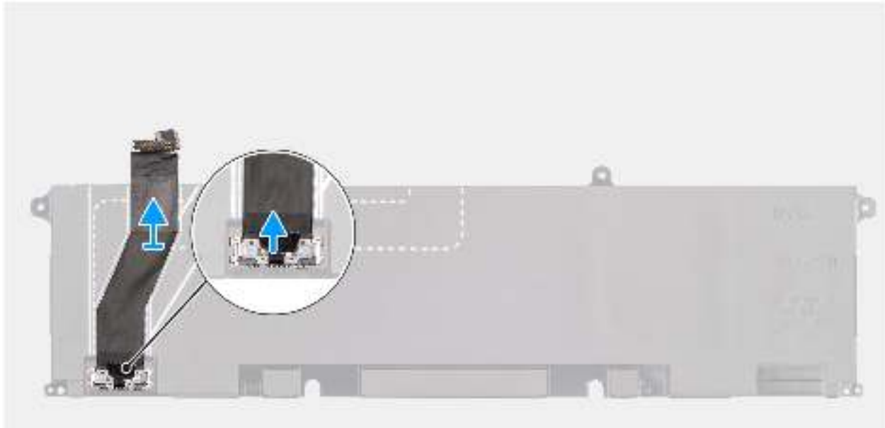
Abbildung 19. Trennen des Batteriekabels.
