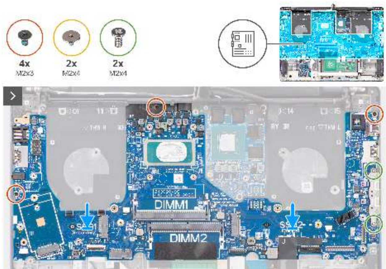
Abbildung 92. Einbauen der Systemplatine
