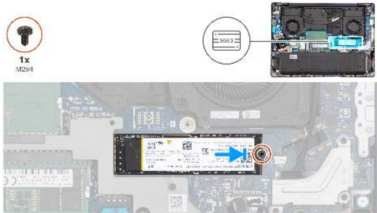
Abbildung 26. Installieren des M.2 2280-Solid-State-Laufwerks
