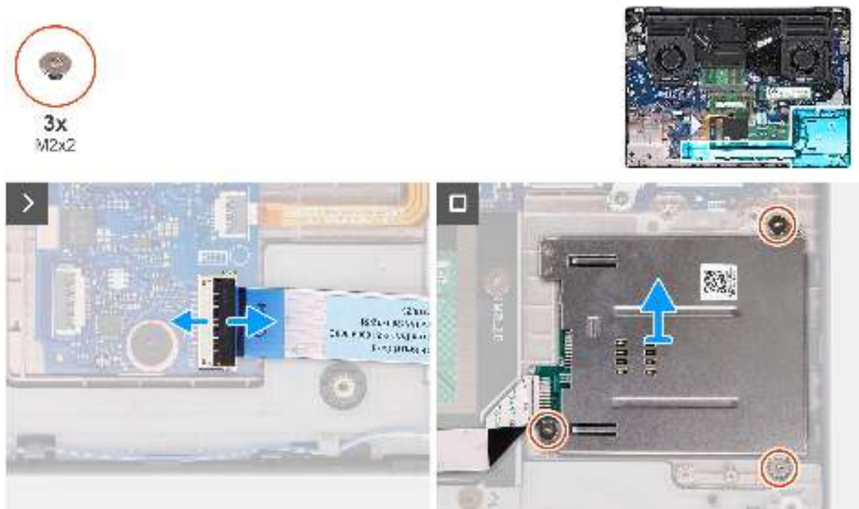
Abbildung 52. Entfernen des Smartcardlesegeräts
