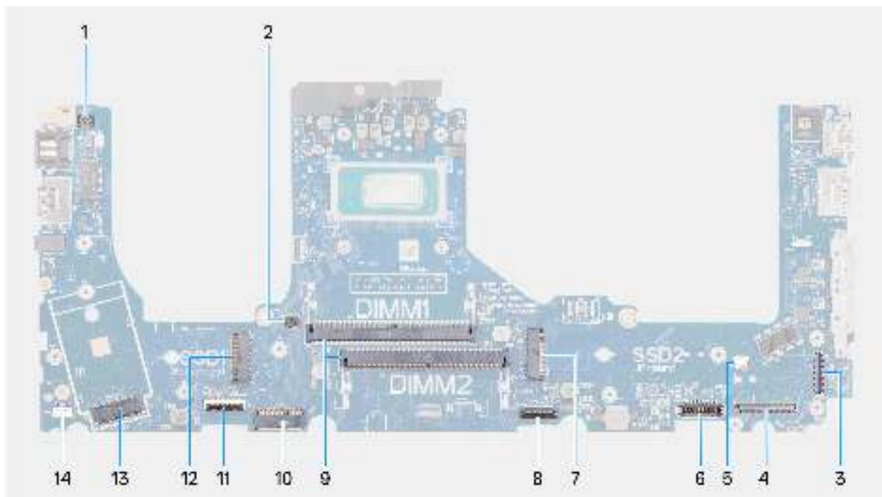
Abbildung 88. Anschlüsse auf der Hauptplatine
