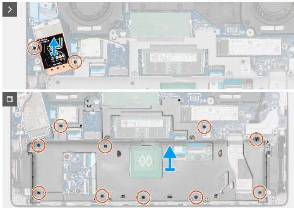
Abbildung 48. Entfernen des Akkurahmens
