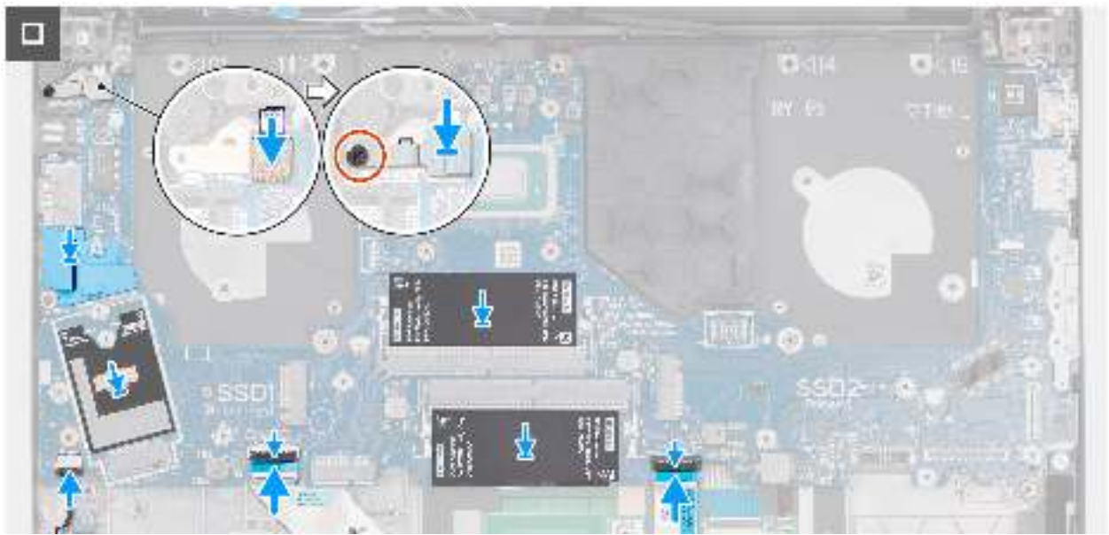
Abbildung 87. Einbauen der Systemplatine
