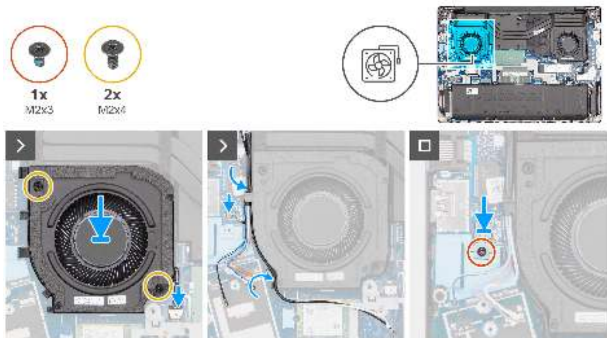
Abbildung 37. Installieren des rechten/Prozessorlüfters
