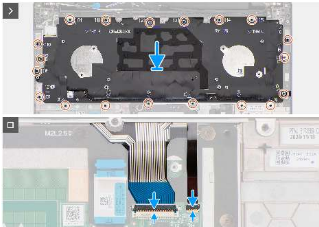
Abbildung 101. Einbauen der Tastatur
