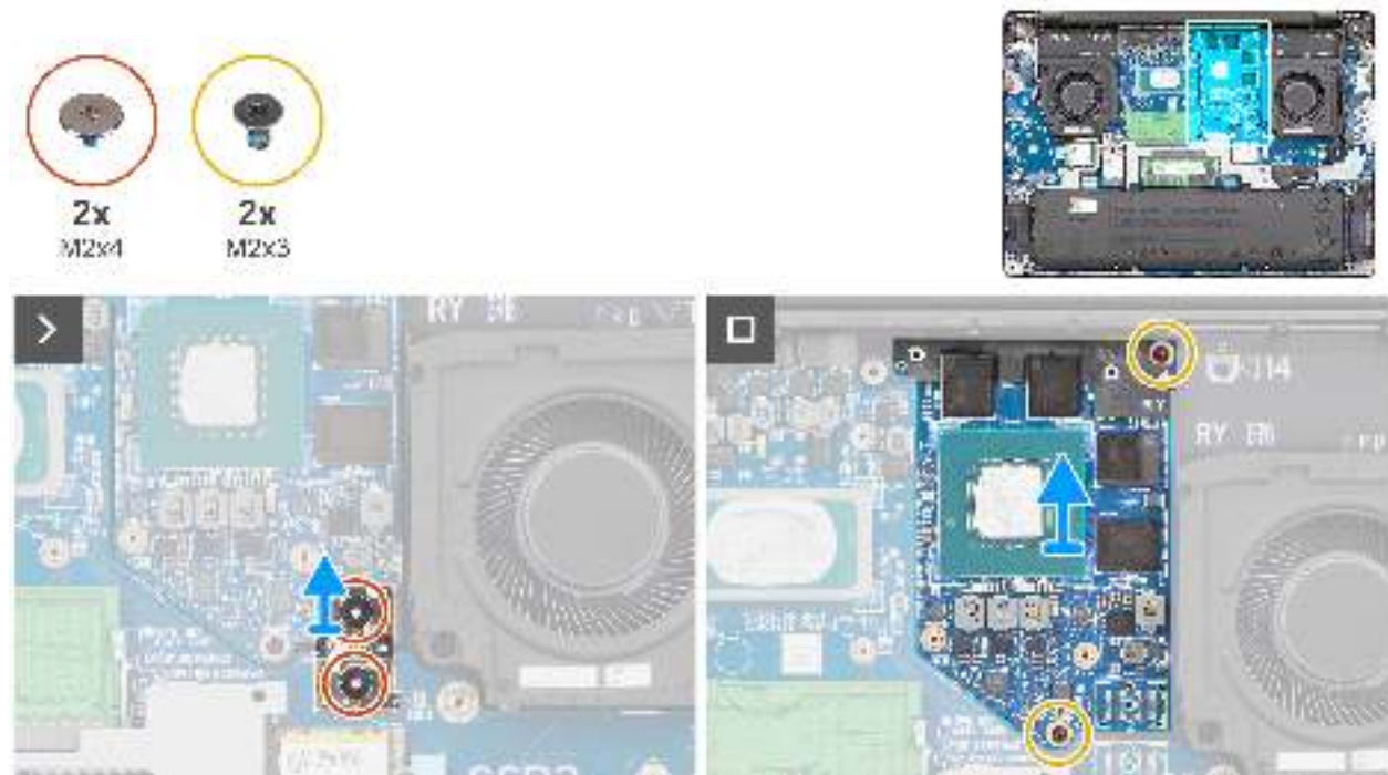
Abbildung 46. Entfernen der GPU
