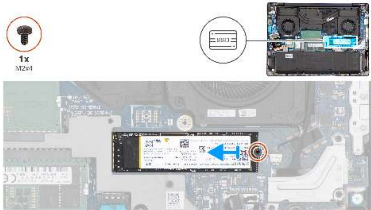
Abbildung 25. Entfernen des M.2-2280-Solid-State-Laufwerks
