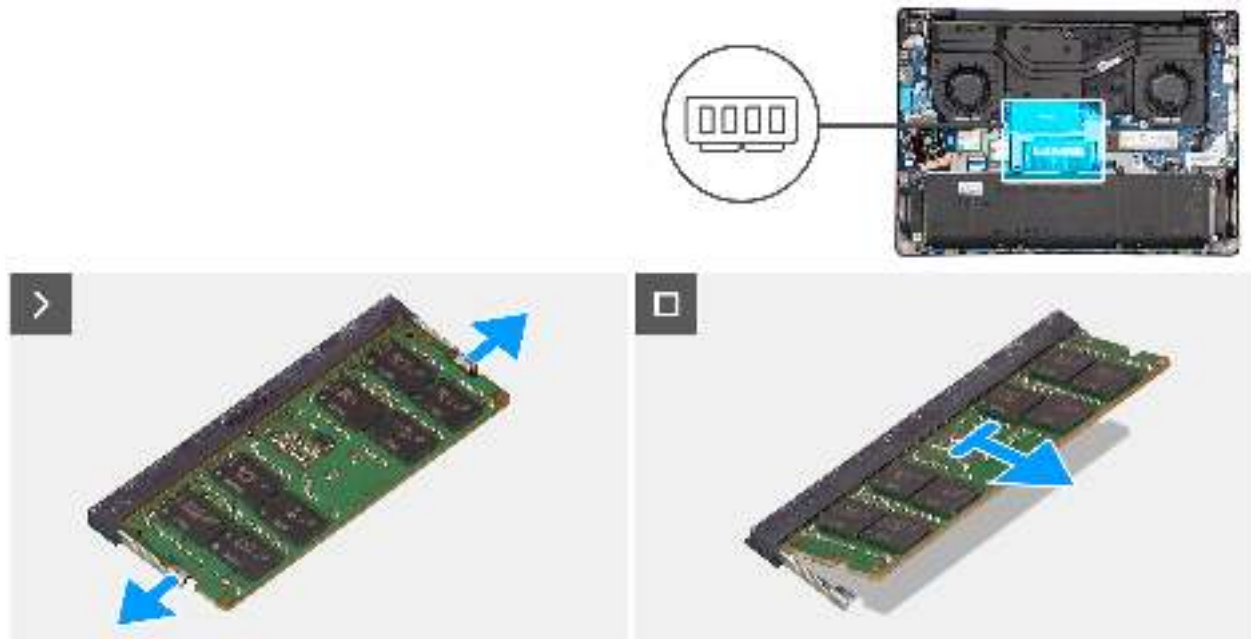
Abbildung 21. Entfernen des Arbeitsspeichersmoduls
