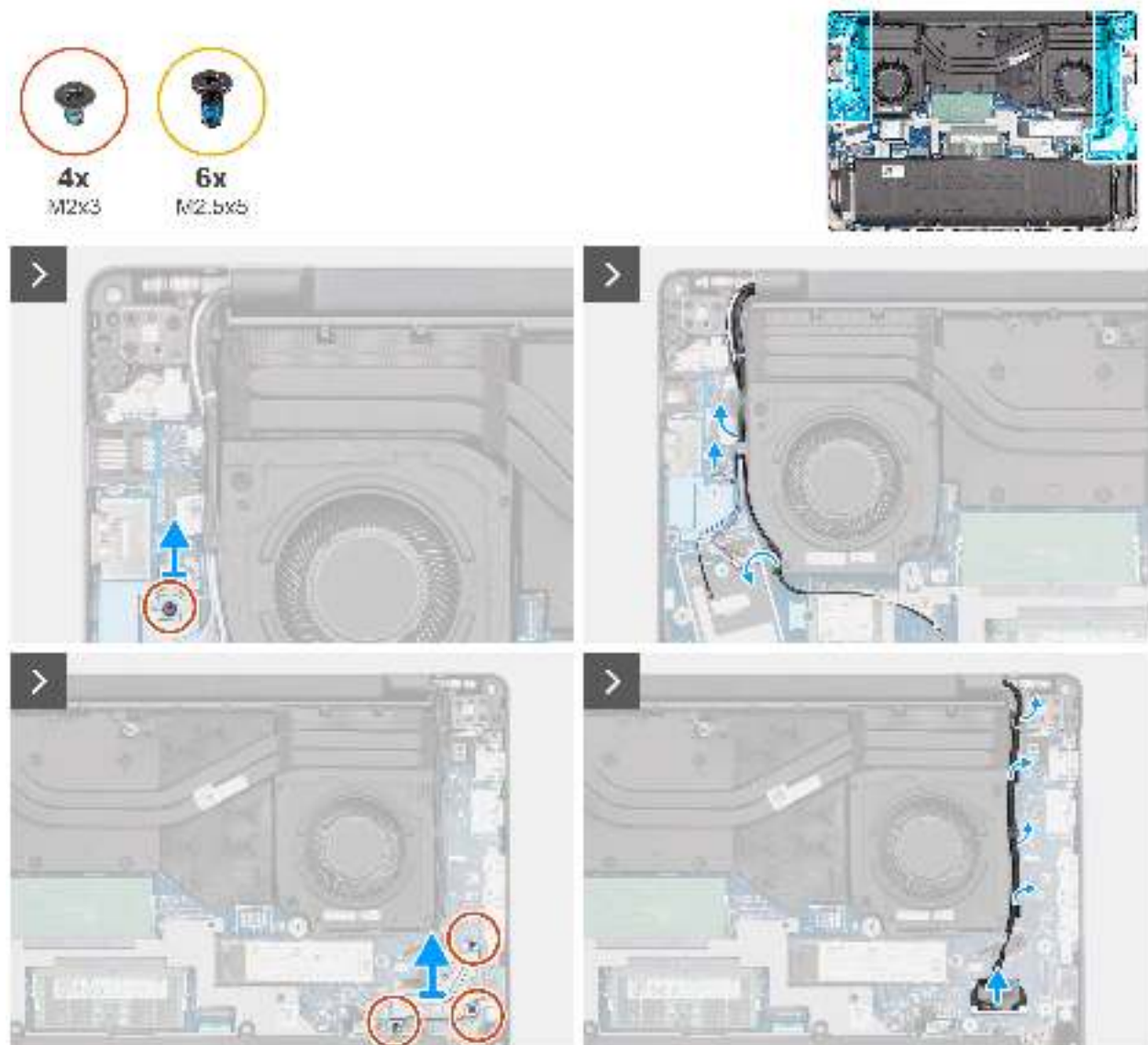
Abbildung 54. Entfernen der Bildschirmbaugruppe
