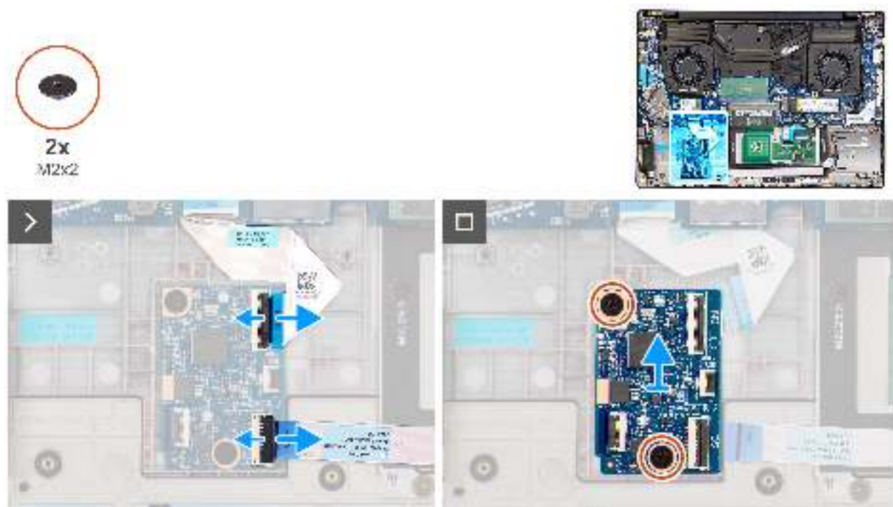
Abbildung 50. Entfernen der USH-Platine
