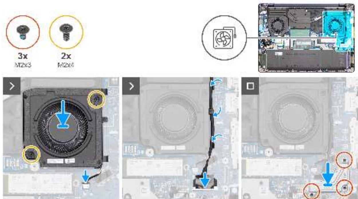
Abbildung 39. Einbauen des linken/Videolüfters
