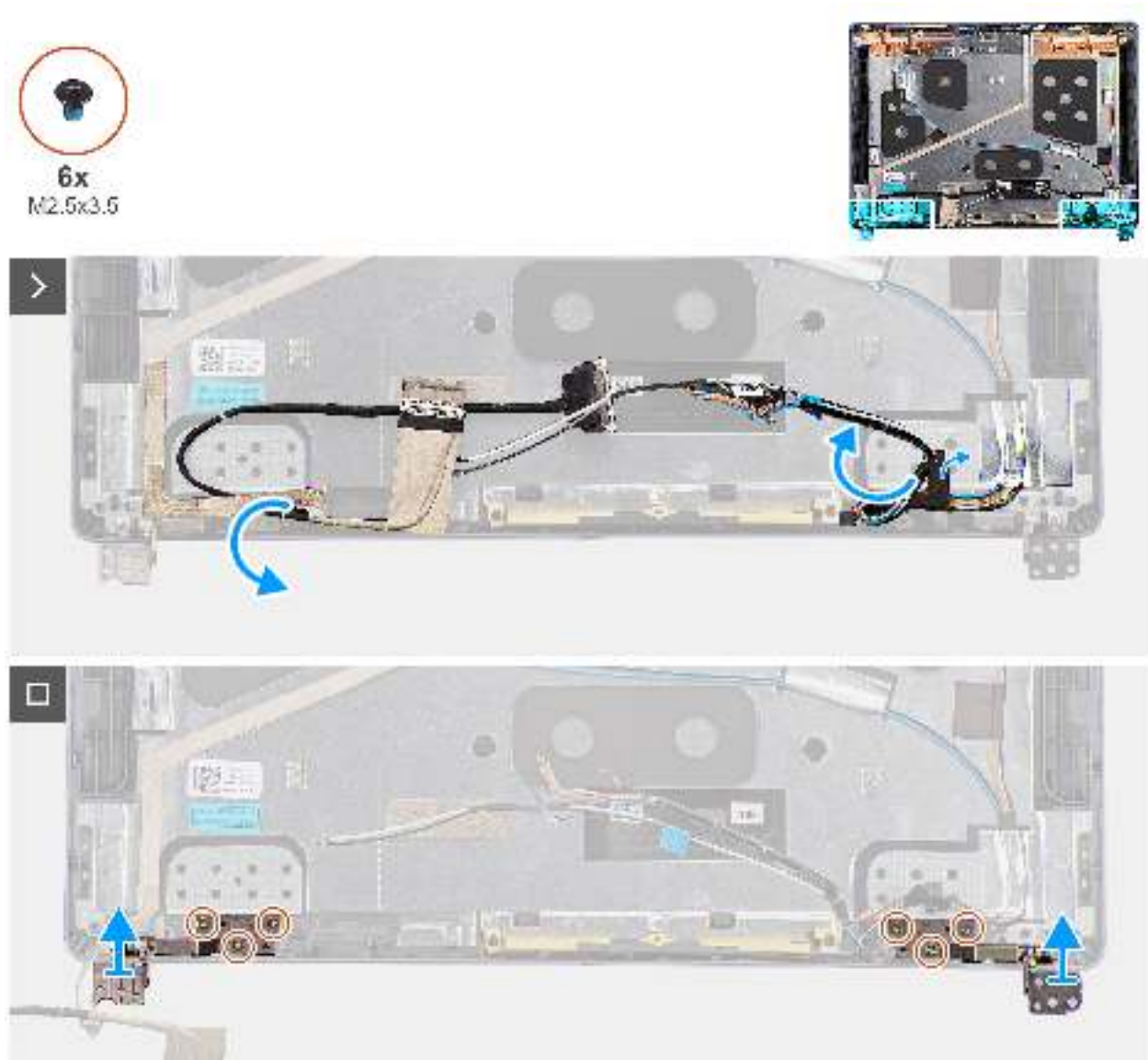
Abbildung 74. Entfernen der Bildschirmscharniere
