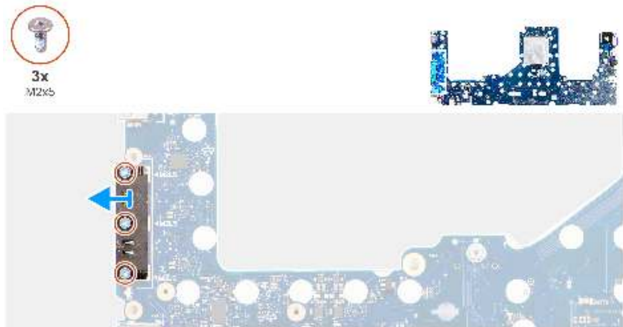
Abbildung 94. Entfernen des USB-Typ-C-Moduls
