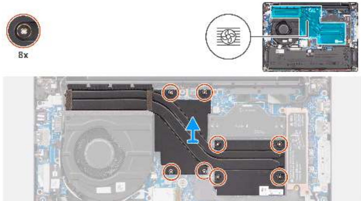
Abbildung 41. Kühlkörper entfernen
