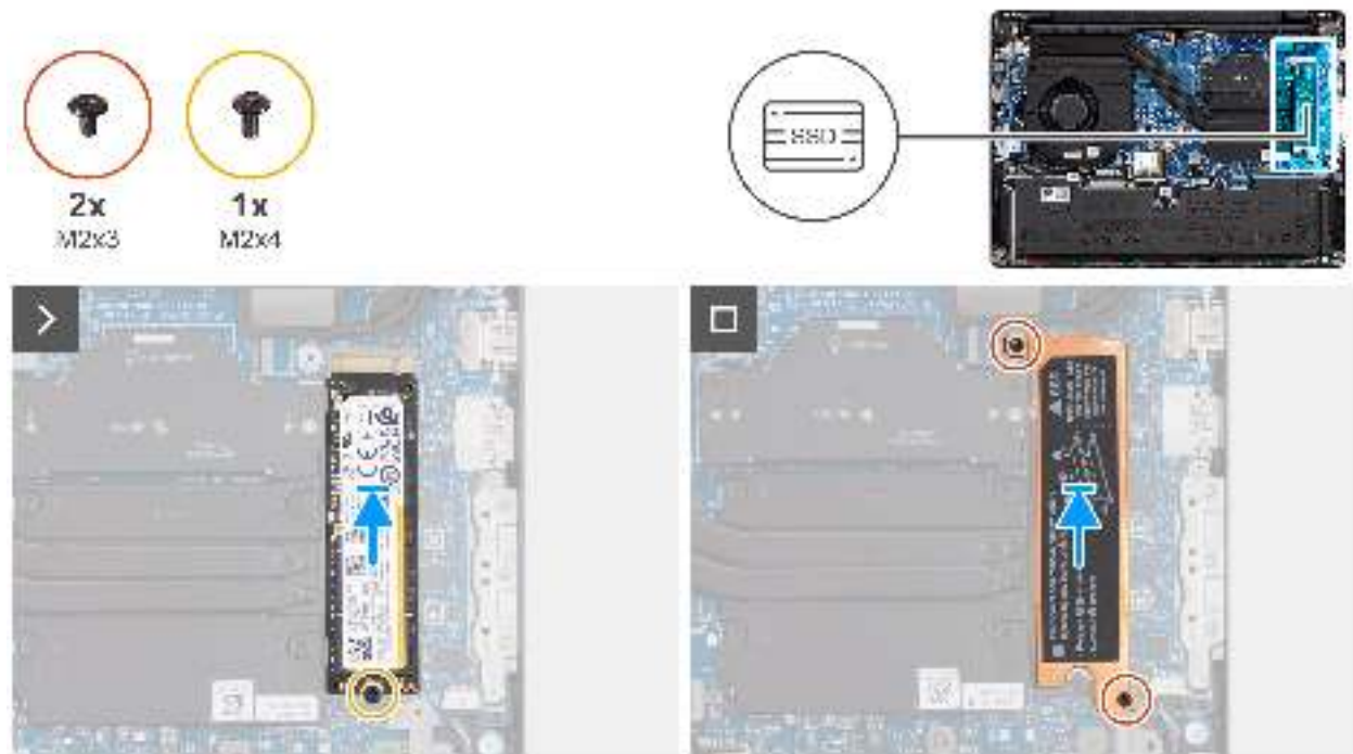
Abbildung 25. Installieren des M.2 2280-Solid-State-Laufwerks
