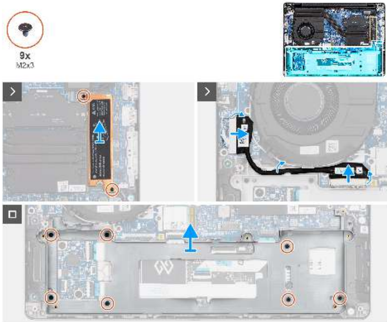
Abbildung 33. Entfernen des Akkurahmens
