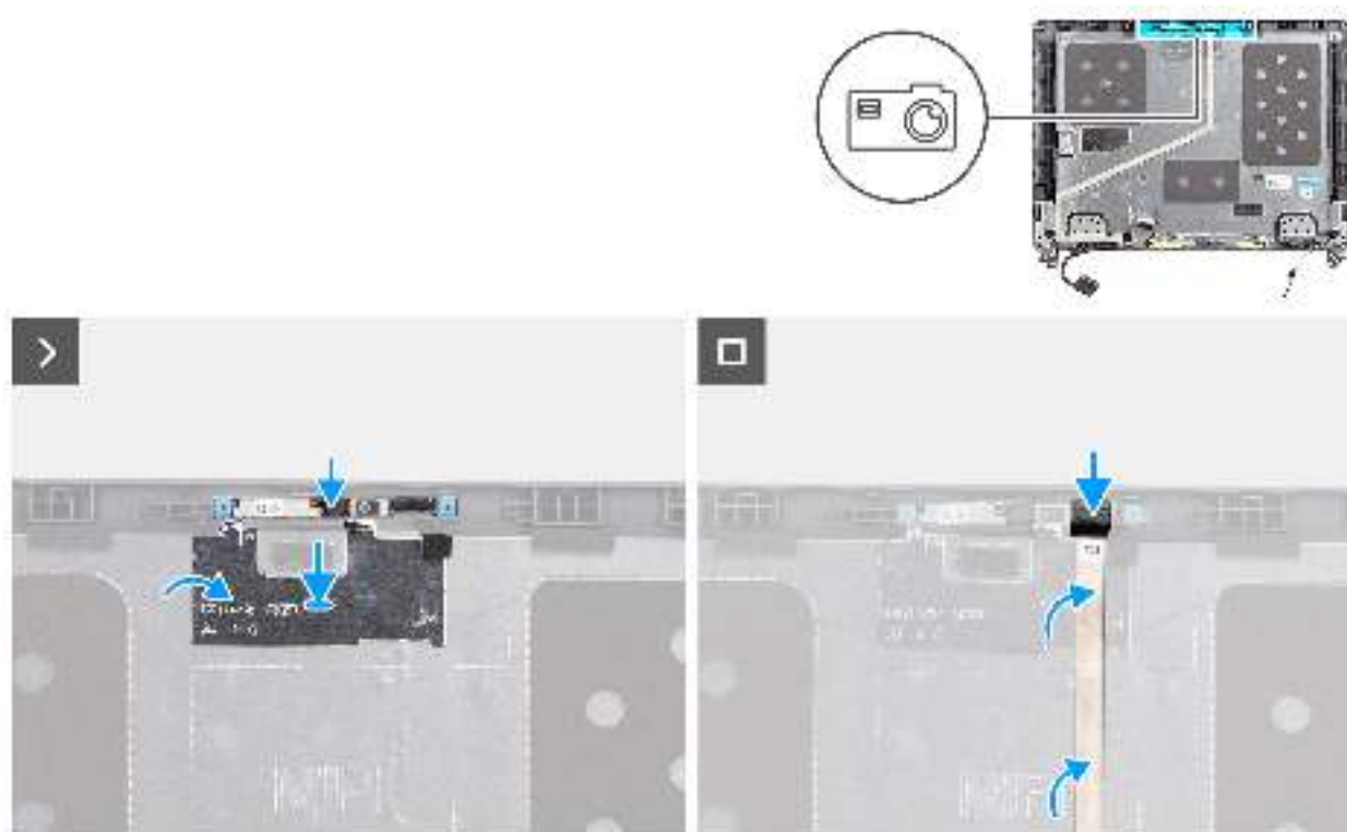
Abbildung 71. Installieren der Kamera
