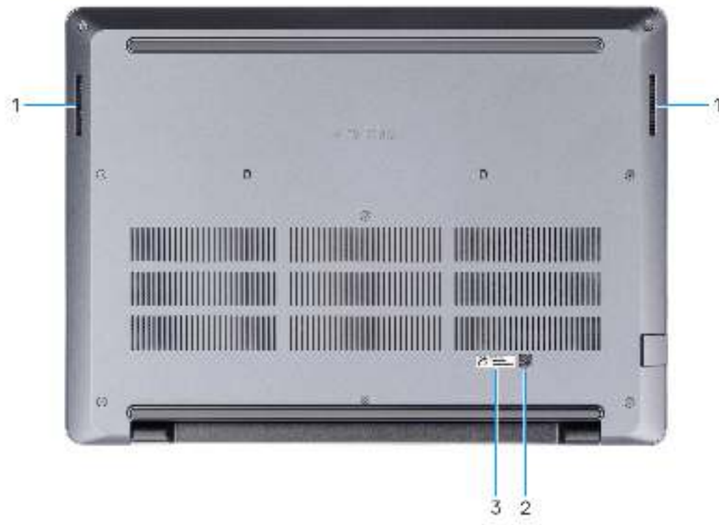
Abbildung 6. Untere Ansicht
