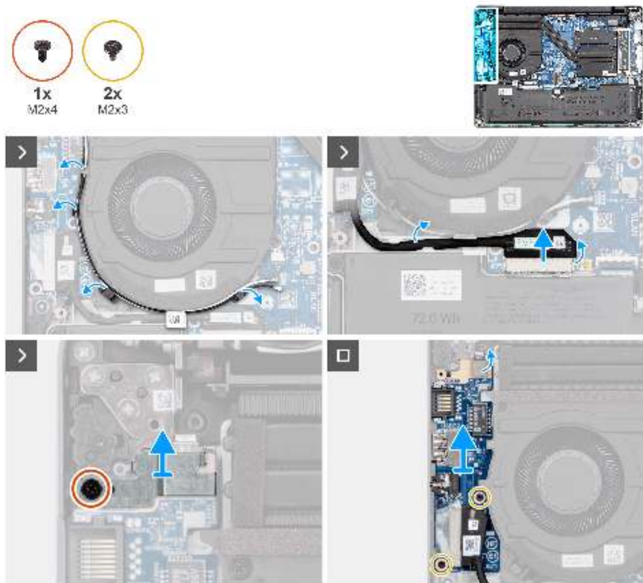
Abbildung 43. Entfernen der E/A-Platine
