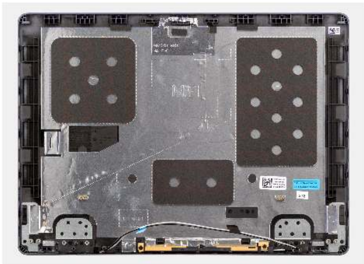
Abbildung 72. Bildschirmrückwand-Antennen-Baugruppe
