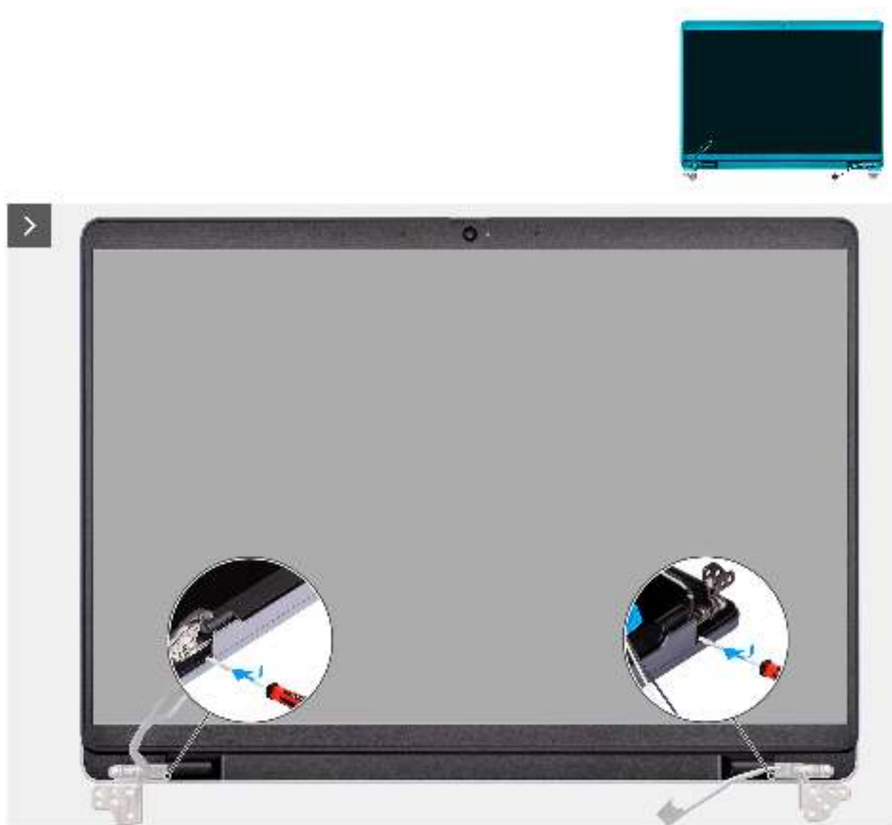
Abbildung 52. Removing the display bezel
