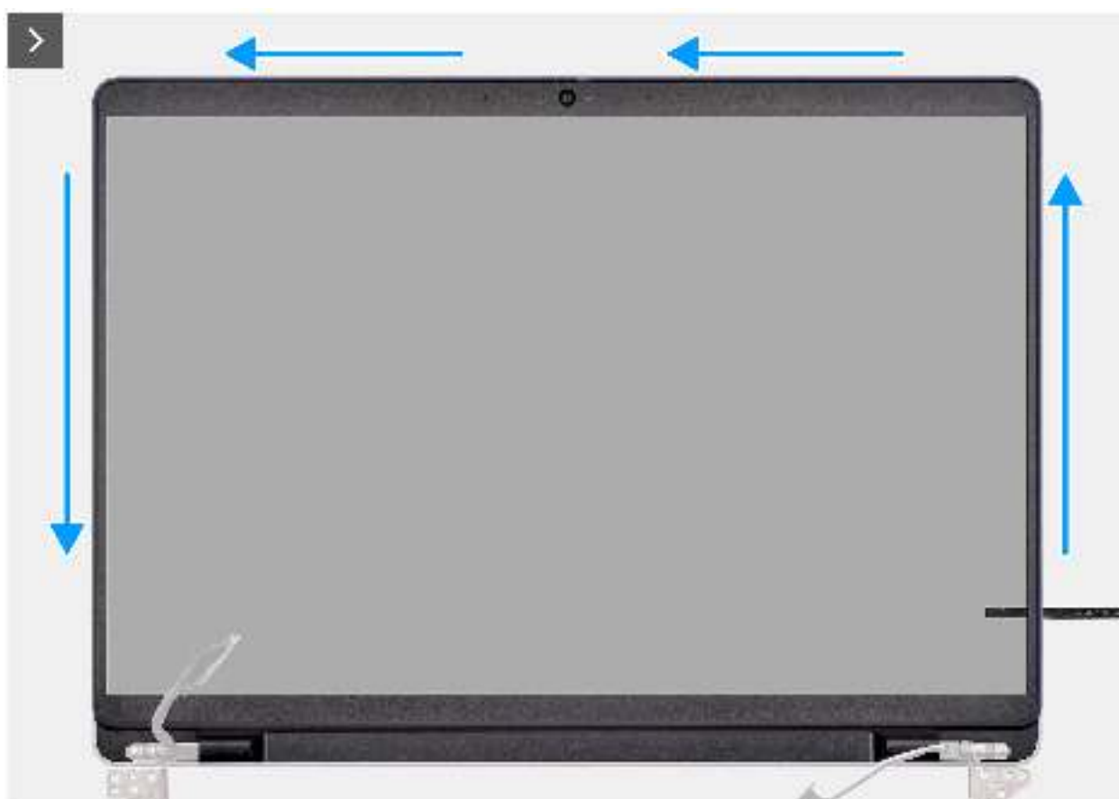
Abbildung 54. Removing the display bezel
