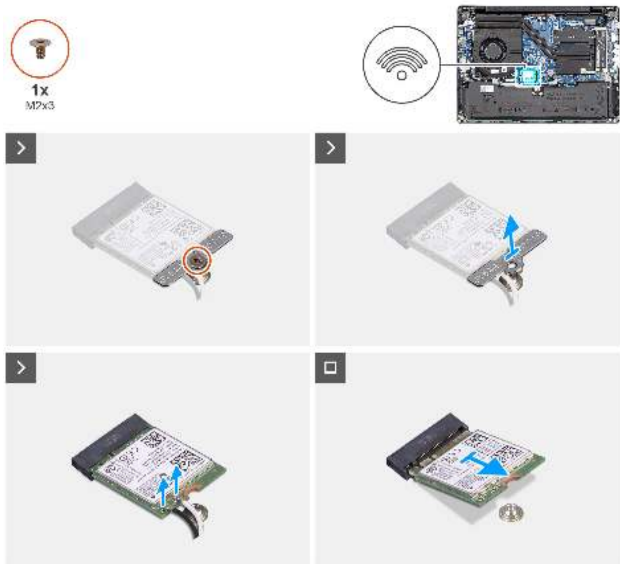
Abbildung 26. Entfernen der Wireless-Karte
