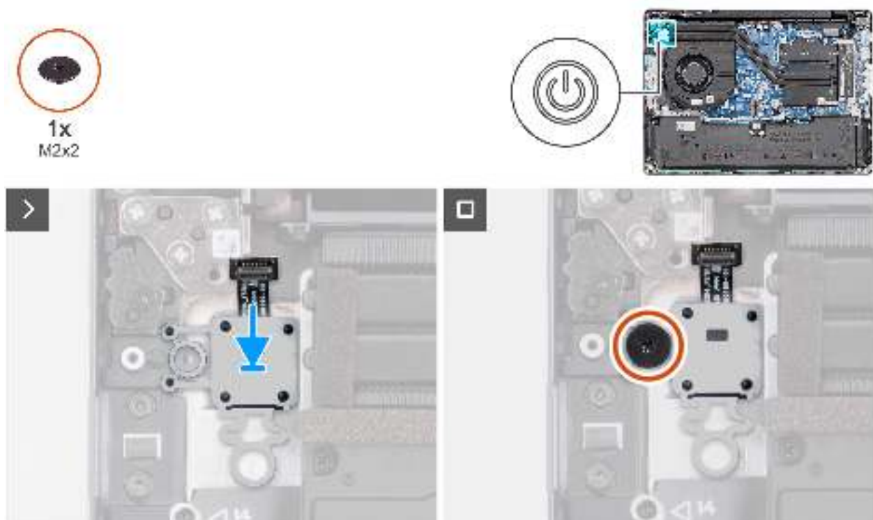
Abbildung 46. Installieren des Netzschalters
