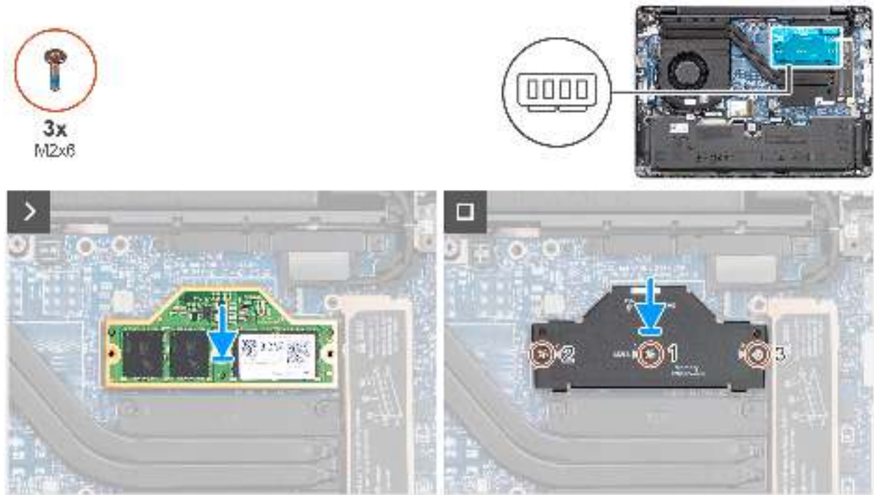
Abbildung 21. Einsetzen des Speichermoduls
