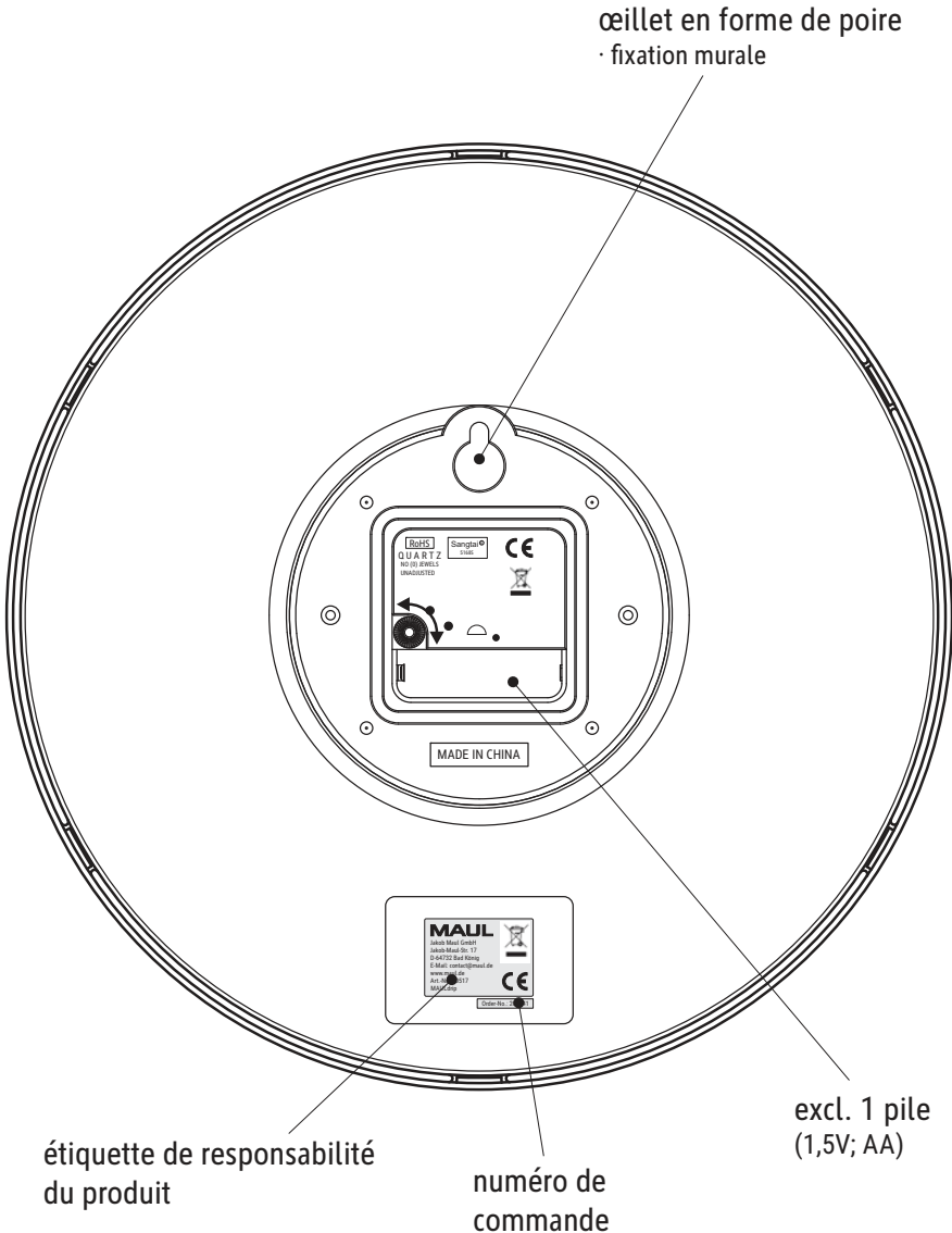
Face arrière
