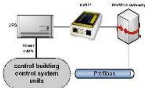
Abbildung 122: CS121 PROFIBUS Installation
