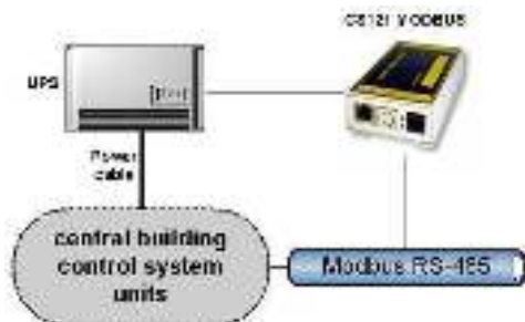
Abbildung 121: CS121MODBUS Installation
