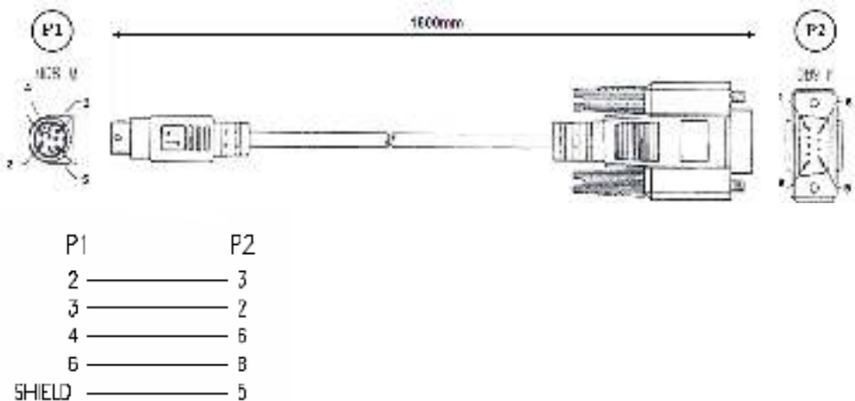
Abbildung 137: Cable configuration HW121/HW131 COM2
