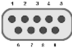
Abbildung 138: External D-SUB 9-polig male
