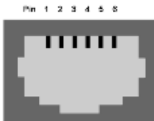
Abbildung 146: AUX Port Assignment
