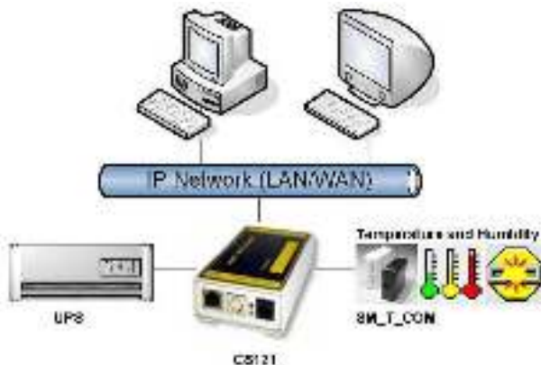
Abbildung 98: CS121-Installation mit Temperaturfühler SM_T_COM
