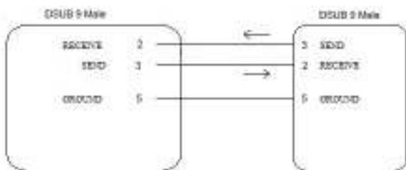
Abbildung 114: PIN-Belegung Adapter-Stecker GSM_A
