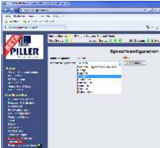
Abbildung 29: Sprachkonfiguration
