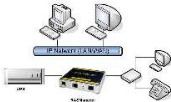
Abbildung 113: RASMANAGER – Netzwerkintegration
