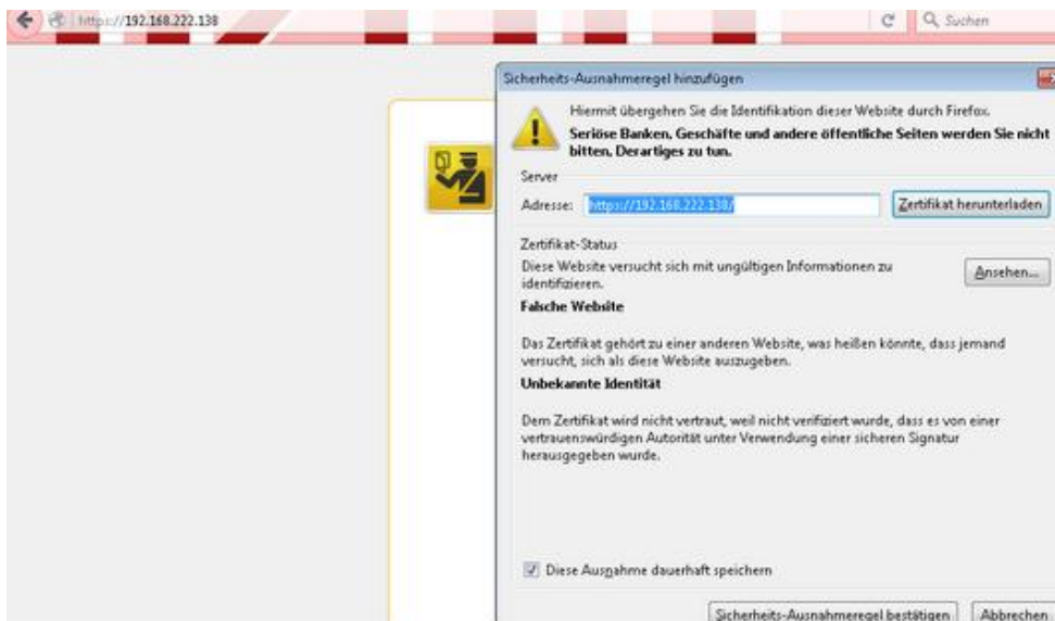
Abbildung 136: Sicherheits-Ausnahmeregel hinzufügen
