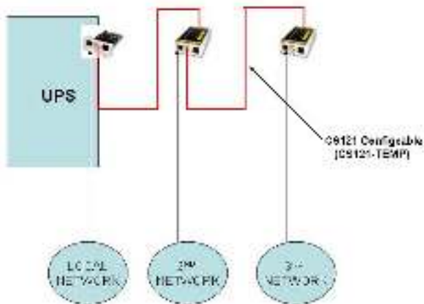
Abbildung 44: Pipe Thru Installation
