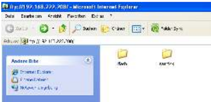
Abbildung 78: CS121-FTP-Ordner
