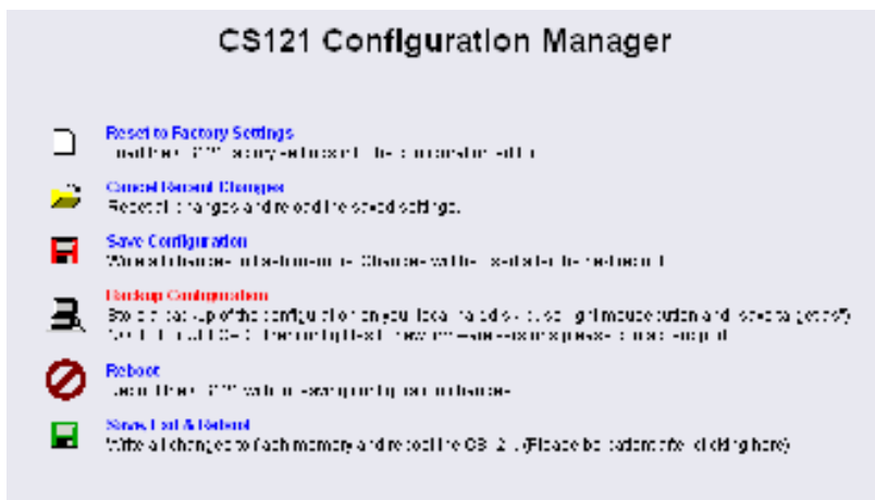
Abbildung 75: CS121-Configuration Manager
