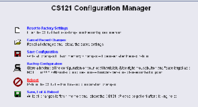
Abbildung 81: CS121-Reboot
