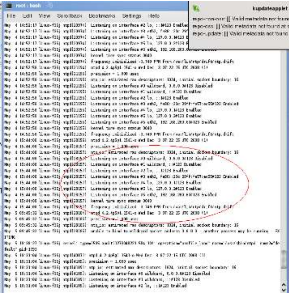
Abbildung 130: Log Messages
