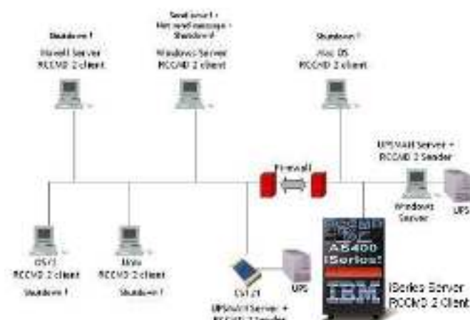
Abbildung 82: RCCMD - Überblick
