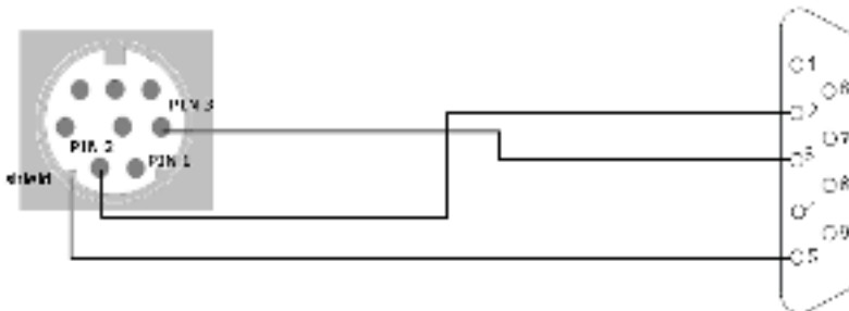
Abbildung 115: Mini8-DSUB9 Kabel Querschnitt
