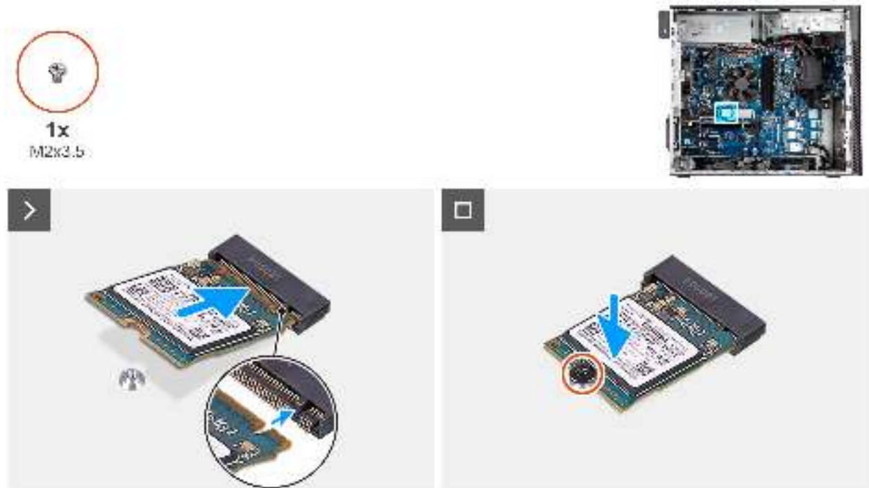
Abbildung 32. Einbauen des M.2 2230-PCIe-SSD-Laufwerks
