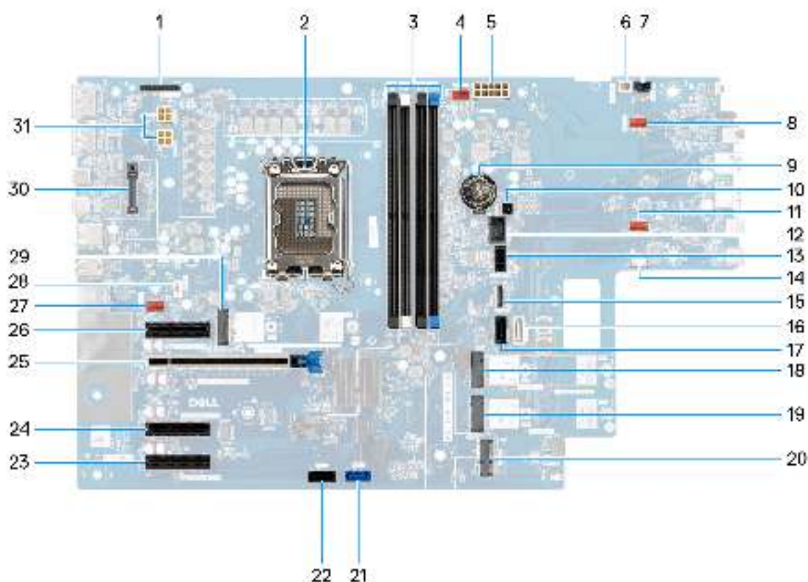
Abbildung 93. Systemplatinenbeschriftung
