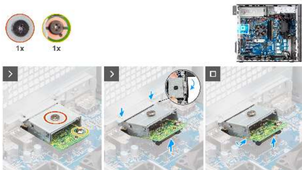
Abbildung 67. Entfernen des optionalen DisplayPort-Moduls
