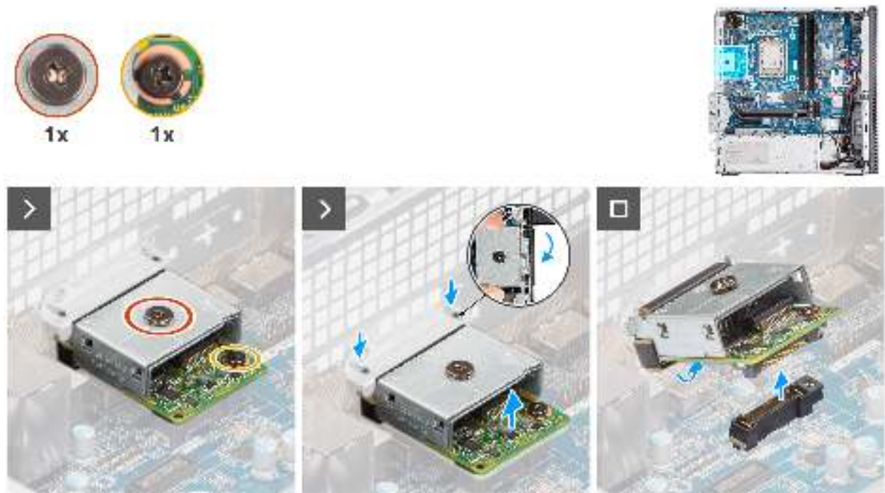
Abbildung 70. Entfernen des optionalen LAN-Moduls
