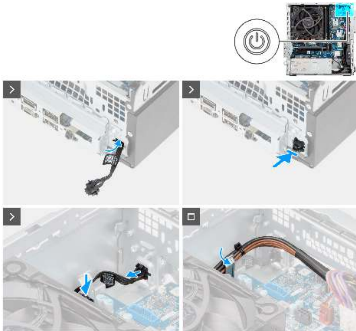
Abbildung 46. Installieren des Netzschalters
