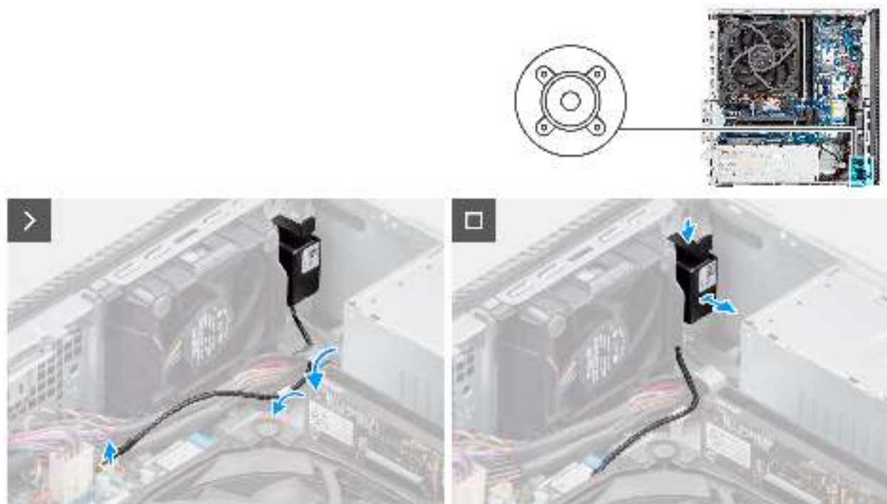
Abbildung 25. Entfernen des internen Lautsprechers
