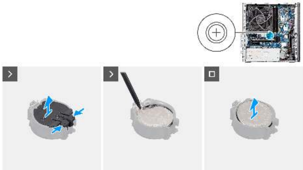
Abbildung 13. Entfernen der Knopfzellenbatterie
