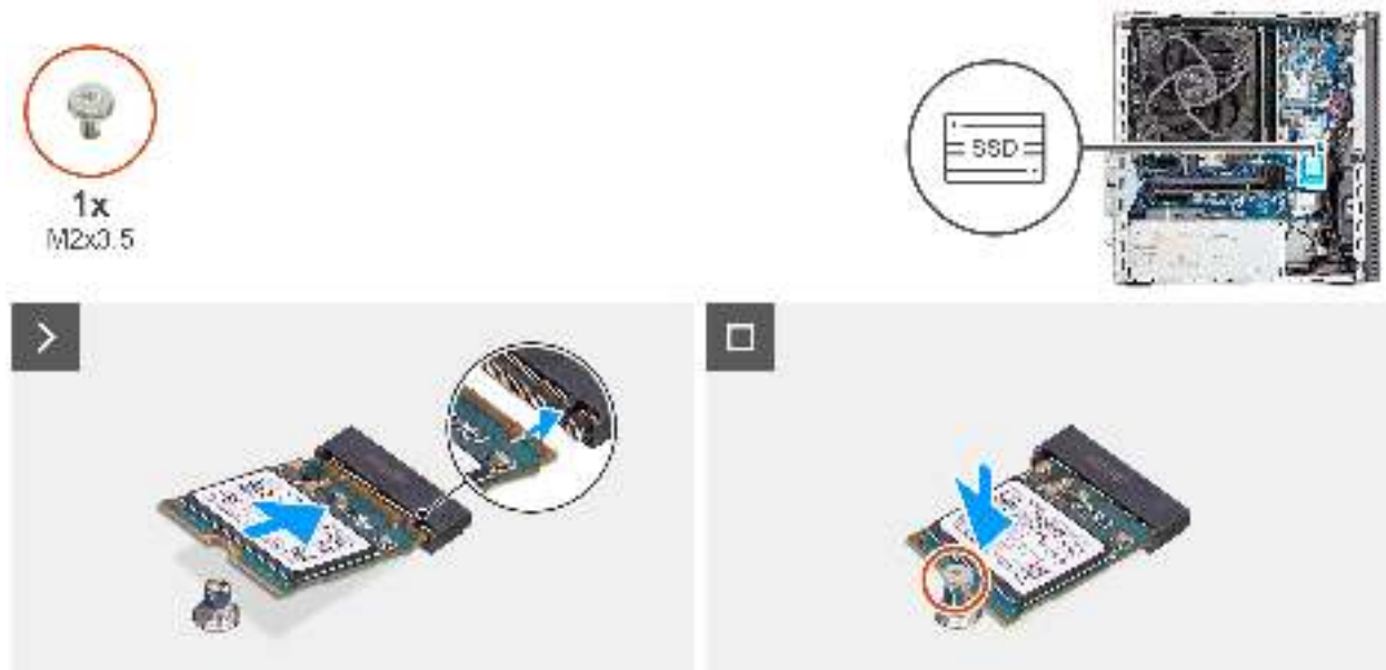
Abbildung 32. Installieren des M.2 2230-SSD-Laufwerks in Steckplatz 0
