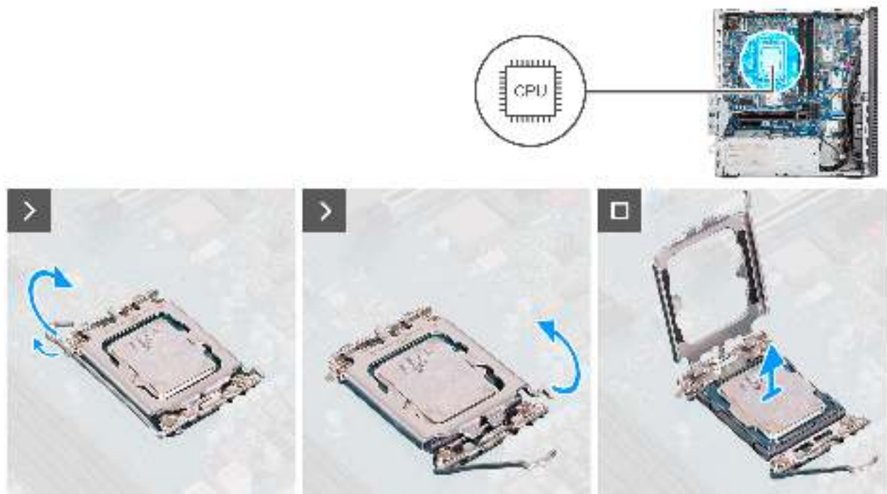
Abbildung 55. Entfernen des Prozessors
