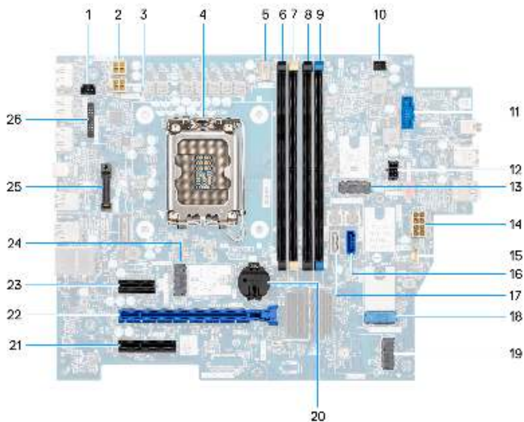
Abbildung 82. Übersicht über die Systemplatine
