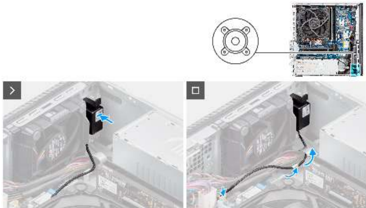
Abbildung 26. Einbauen des internen Lautsprechers
