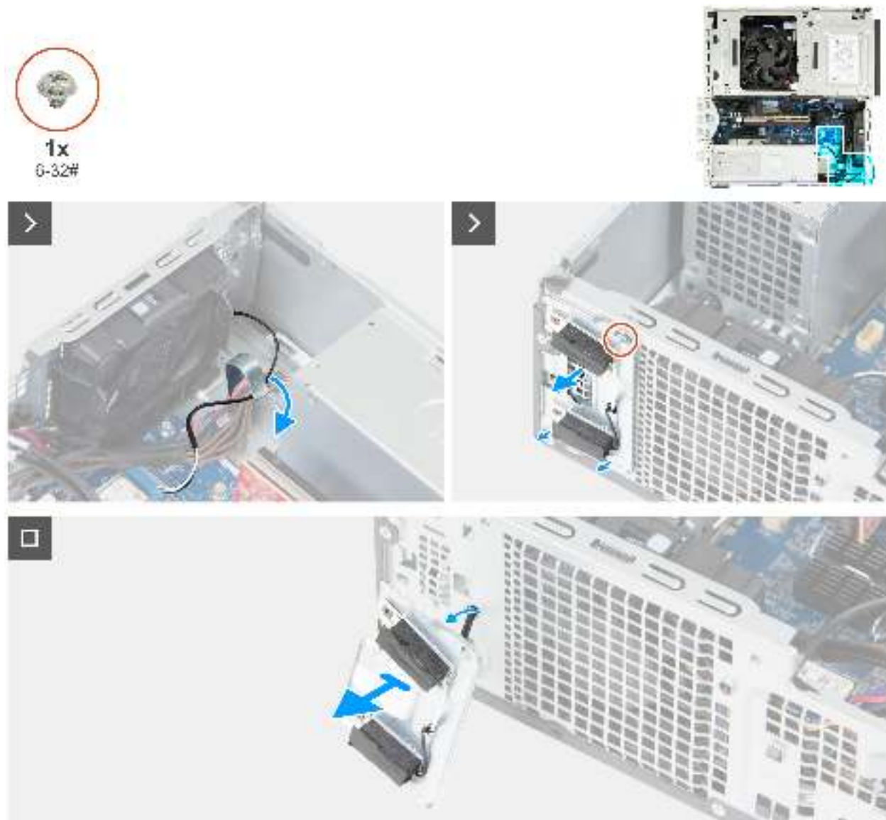
Abbildung 49. Entfernen des Antennenmoduls
