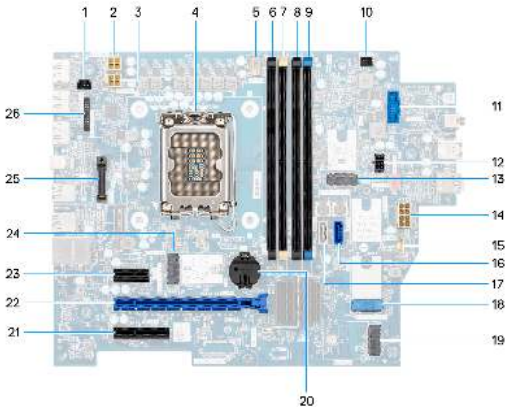
Abbildung 87. Übersicht über die Systemplatine
