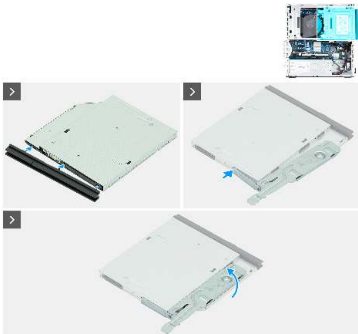
Abbildung 19. Installieren des optischen Laufwerks
