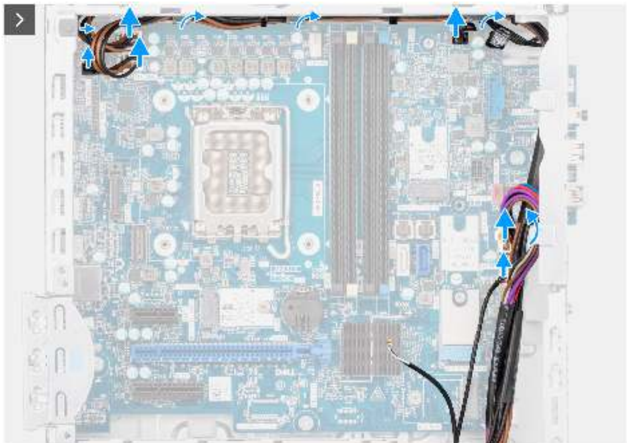
Abbildung 84. Entfernen der Systemplatine
