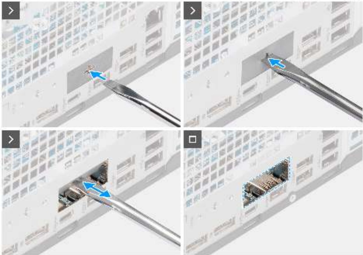
Abbildung 68. Installieren des optionalen Thunderbolt-Moduls
