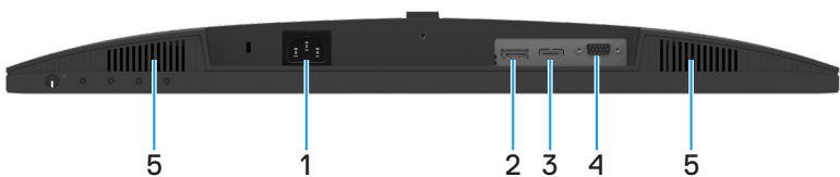
Abbildung 4. Unteransicht
