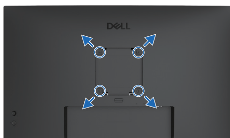
Abbildung 29. VESA-Wandmontage
