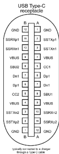
Abbildung 8. Thunderbolt 4-/USB-C-Anschluss
