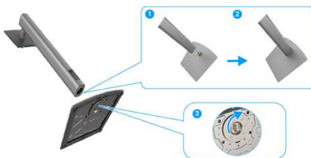
Abbildung 18. Ständer anschließen
