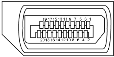
Abbildung 5. DisplayPort (Eingang)
