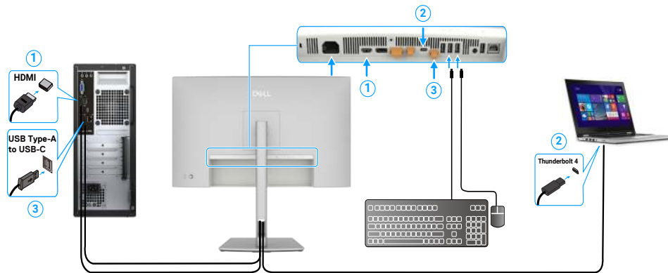
Abbildung 92. KVM 2-Anschluss
