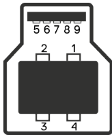
Abbildung 6. USB-Type-B-Upstream-Port.
