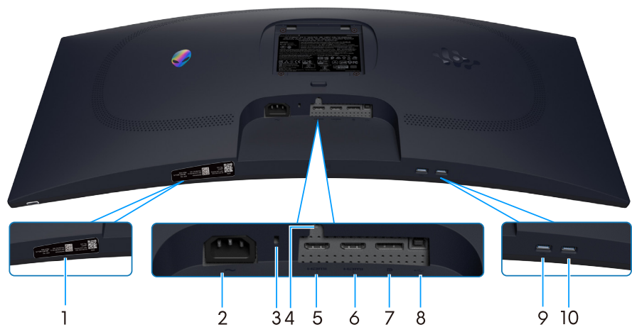
Abbildung 3. Ansicht des Monitors von unten
