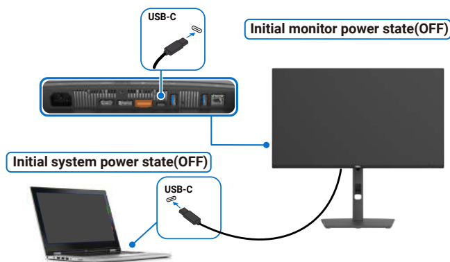
Abbildung 40. Erstmaliges Verbinden des Monitors für DPBS
