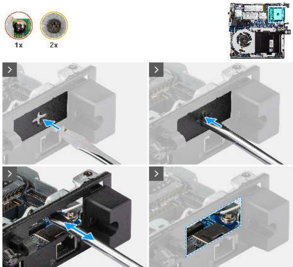
Abbildung 60. Installieren des Glasfasermoduls
