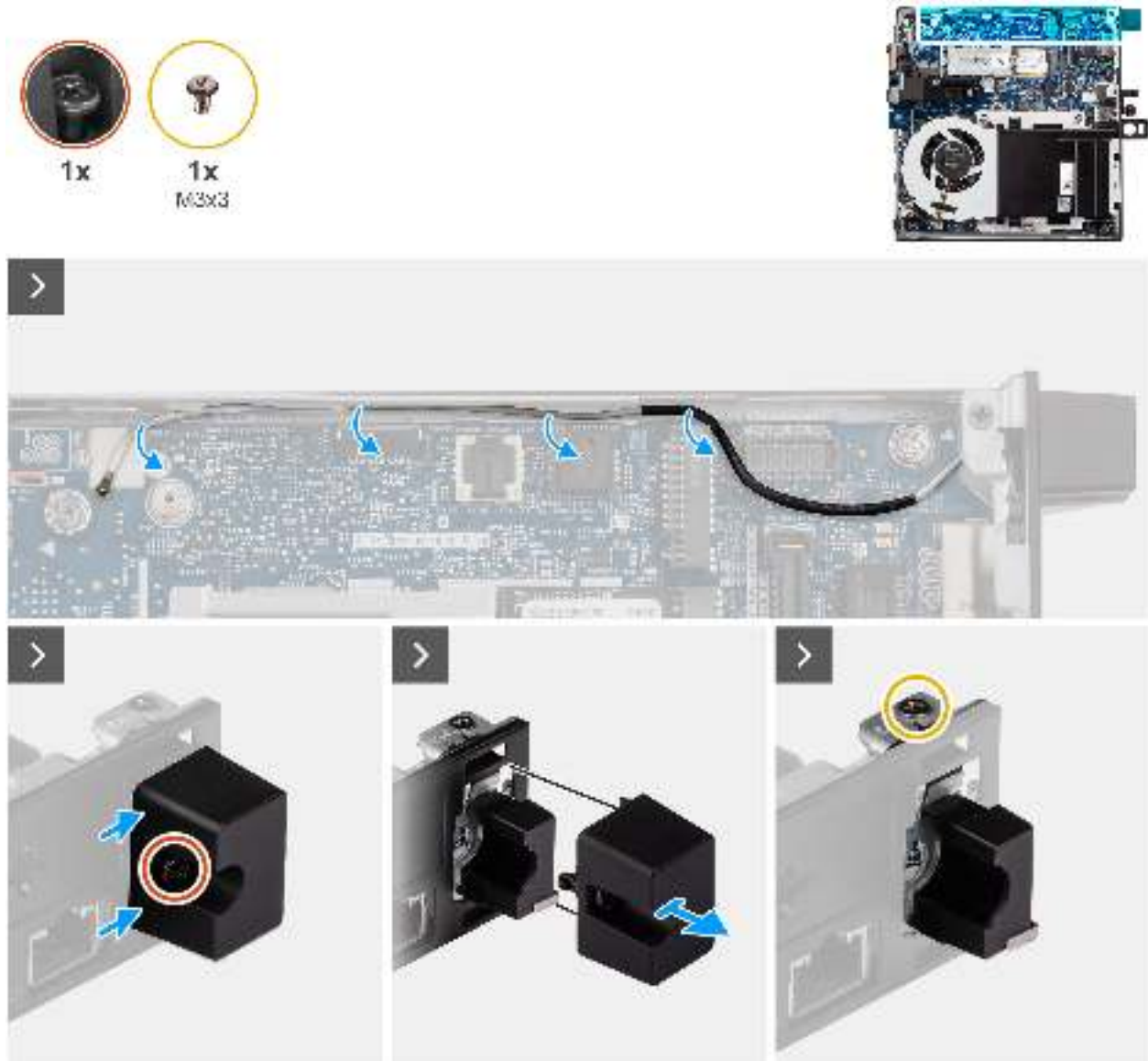
Abbildung 66. Entfernen des Antennenmoduls (weißes Kabel)
