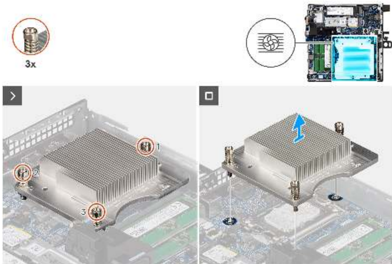
Abbildung 62. Kühlkörper entfernen
