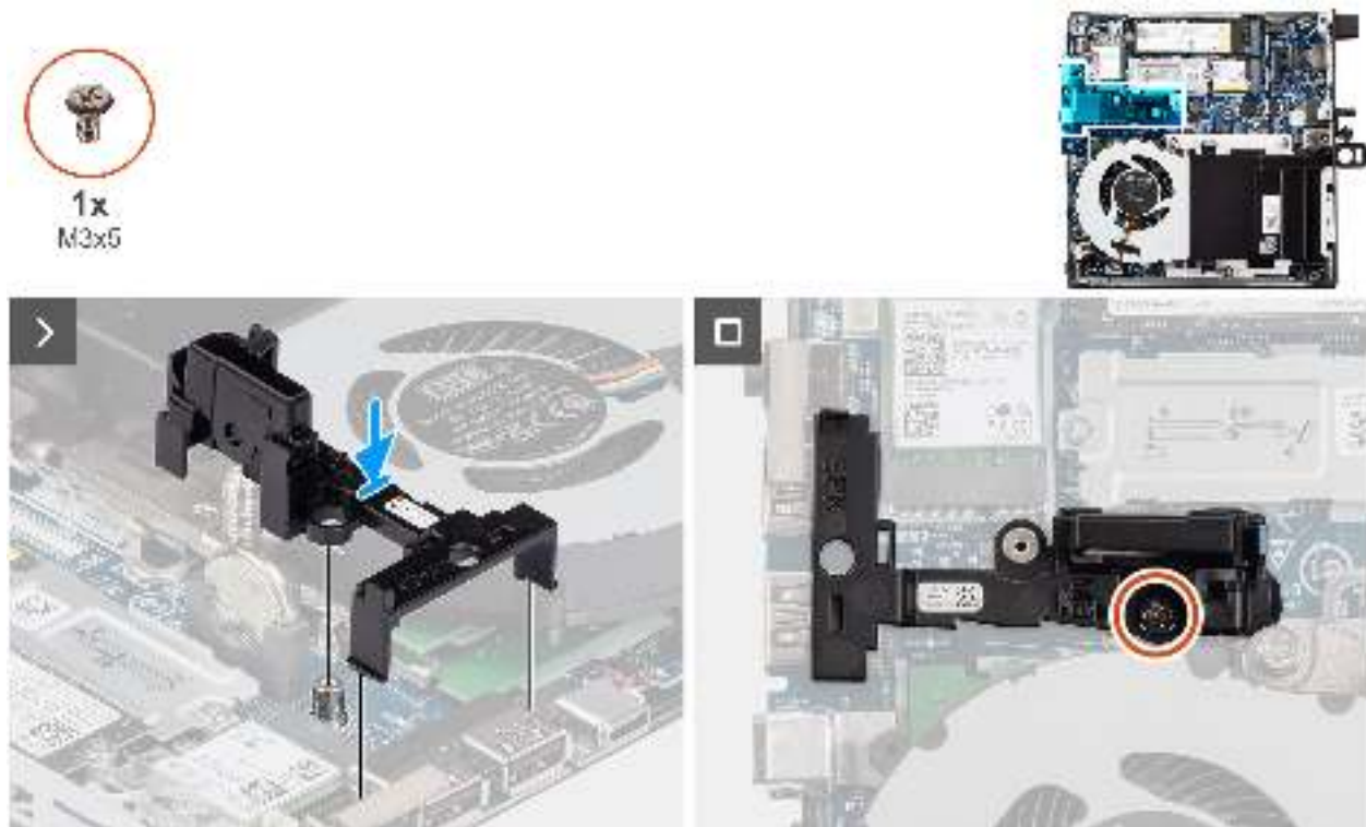
Abbildung 73. Installieren der Lautsprecherhalterung
