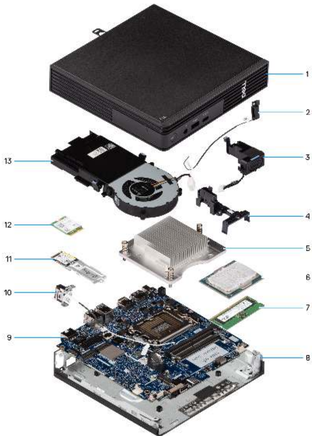
Abbildung 9. Hauptkomponenten des Dell Pro Micro, QCM1250
