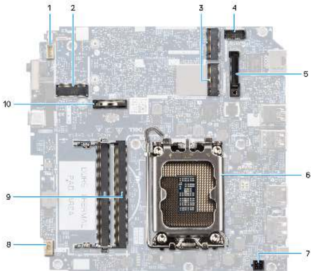
Abbildung 74. Anschlüsse auf der Hauptplatine
