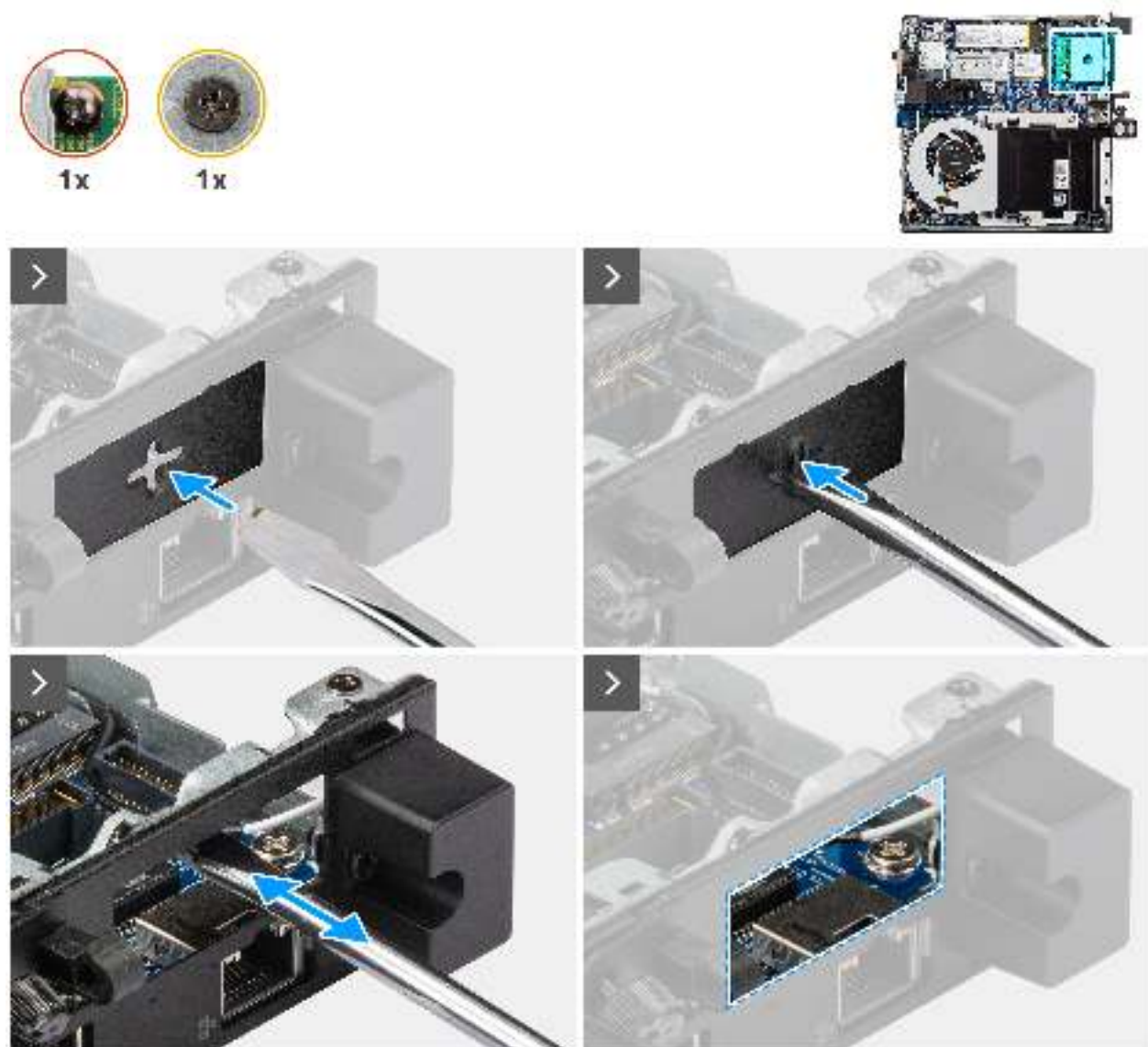
Abbildung 39. Installieren des dualen USB-3.2-Gen2-Anschlussmoduls
