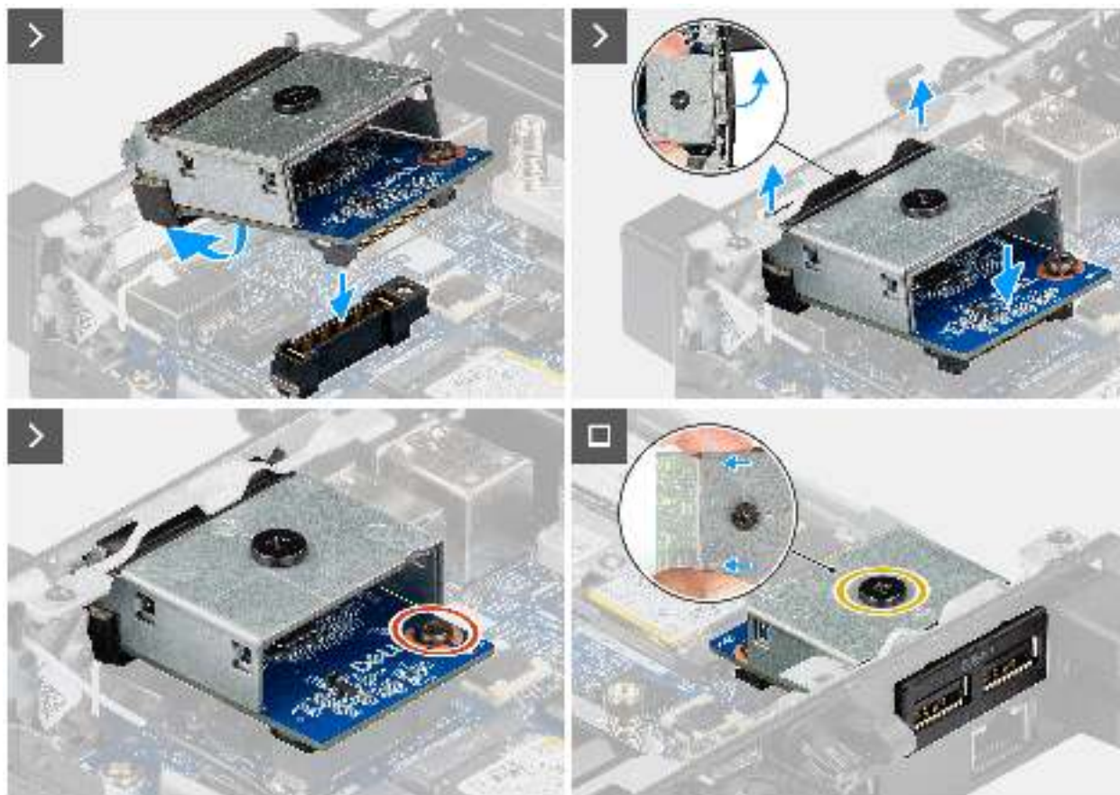
Abbildung 40. Installieren des dualen USB-3.2-Gen2-Anschlussmoduls
