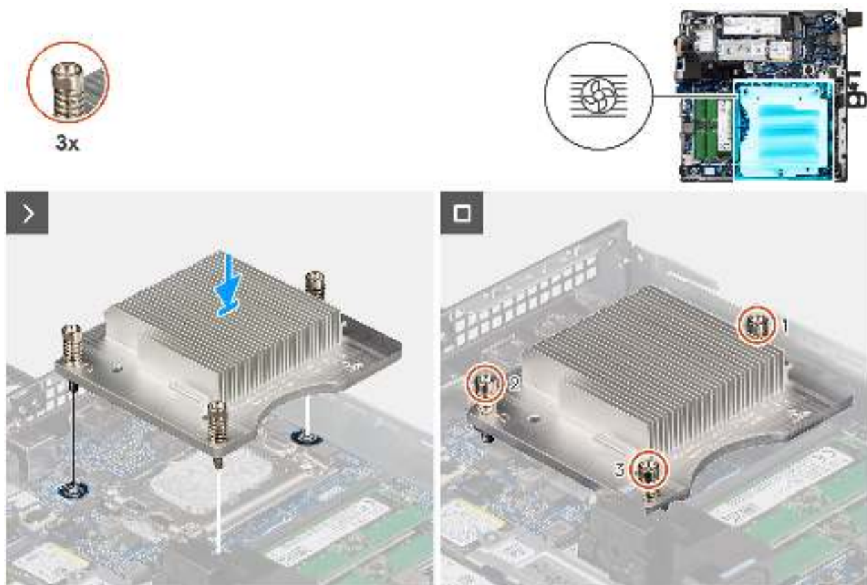
Abbildung 63. Einsetzen des Kühlkörpers
