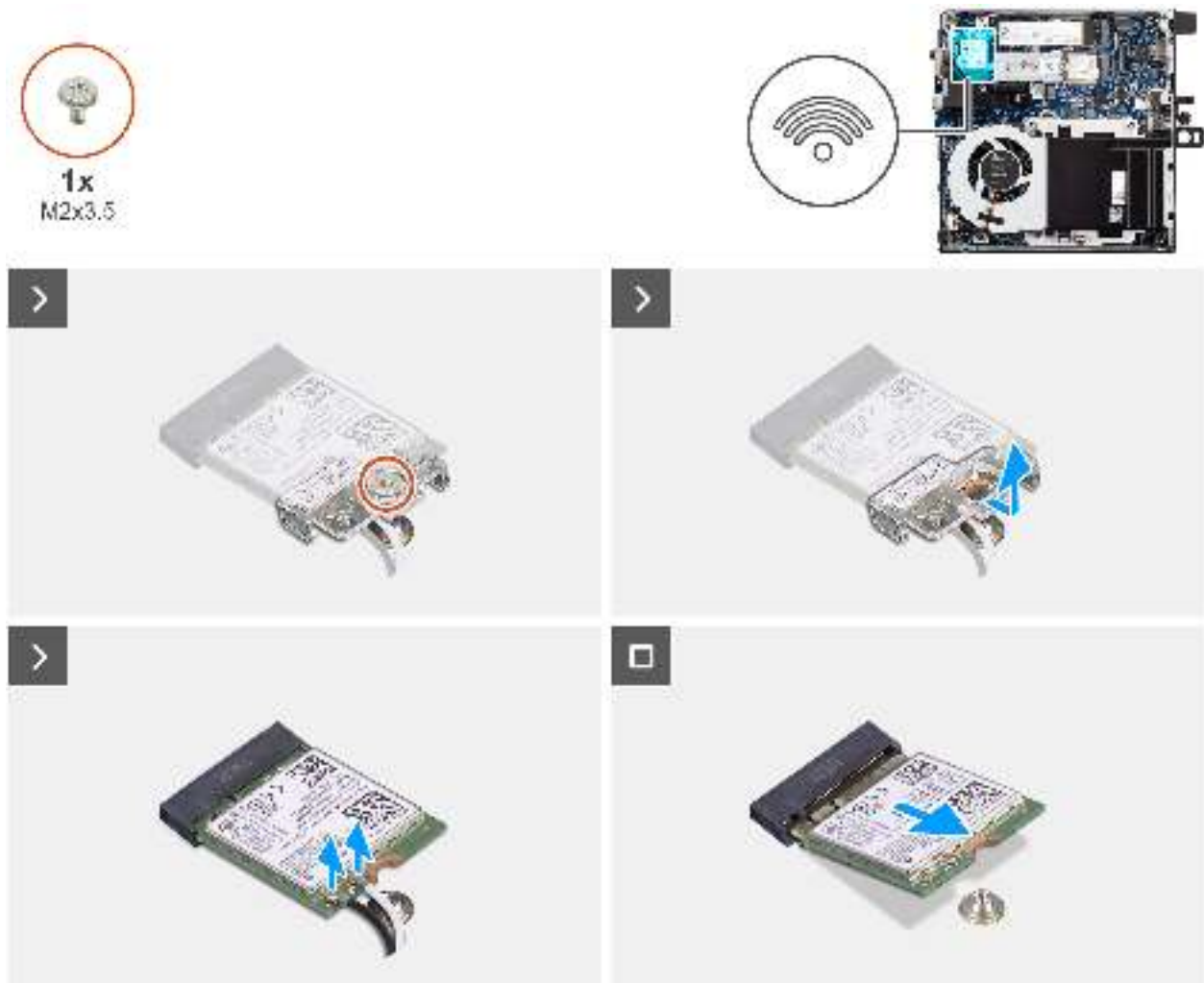
Abbildung 26. Entfernen der Wireless-Karte
