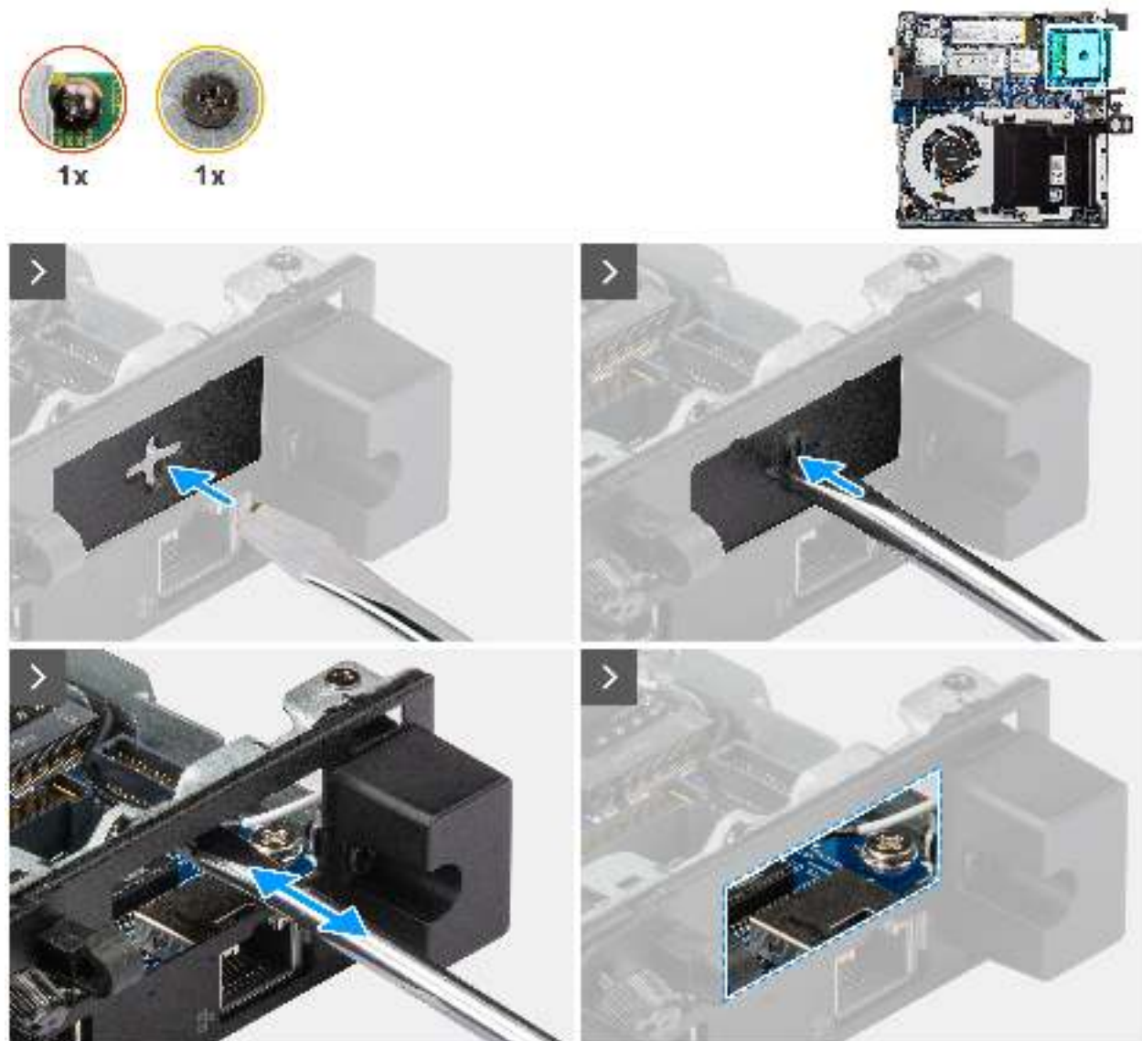
Abbildung 45. Einbauen des DisplayPort-Moduls
