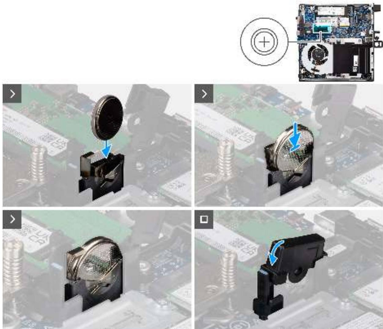
Abbildung 13. Einsetzen der Knopfzellenbatterie
