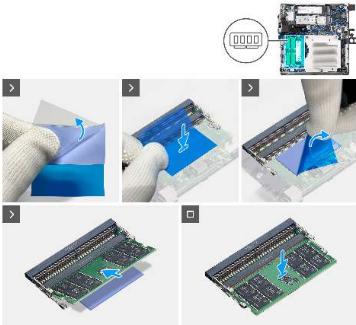
Abbildung 33. Einsetzen des Speichermoduls
