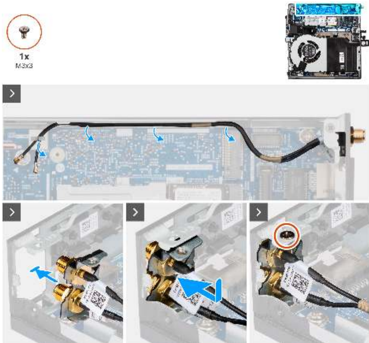
Abbildung 37. Installieren des SMA-Antennenmoduls
