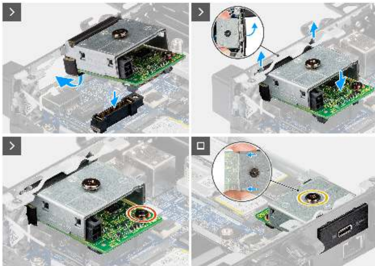
Abbildung 43. Installieren des USB-Typ-C-Anschlussmoduls
