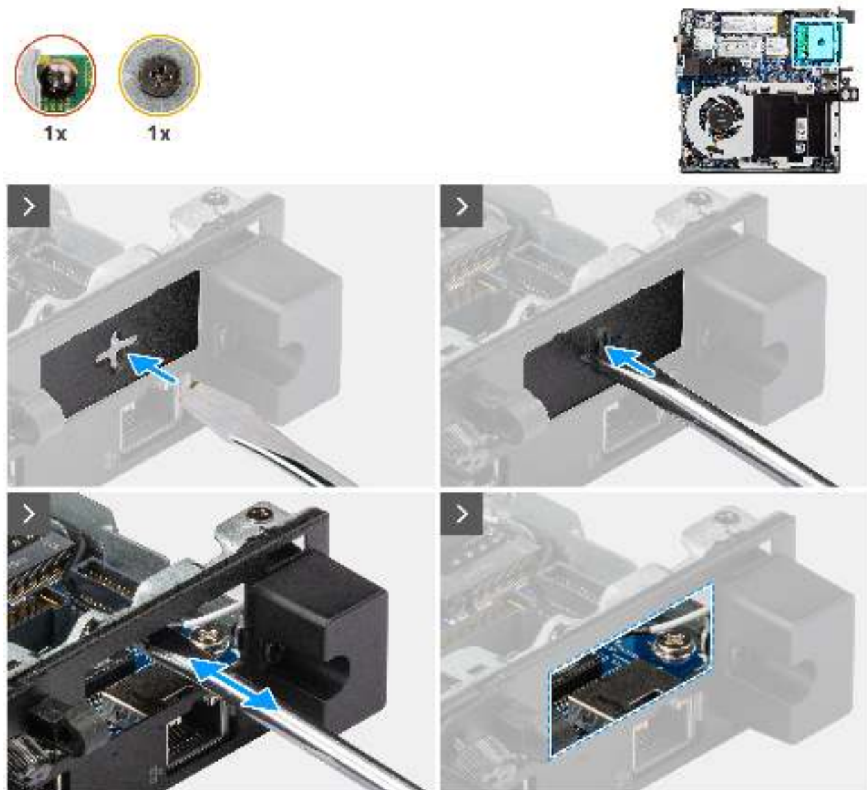
Abbildung 42. Installieren des USB-Typ-C-Anschlussmoduls
