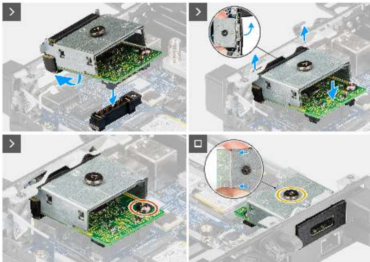
Abbildung 46. Einbauen des DisplayPort-Moduls
