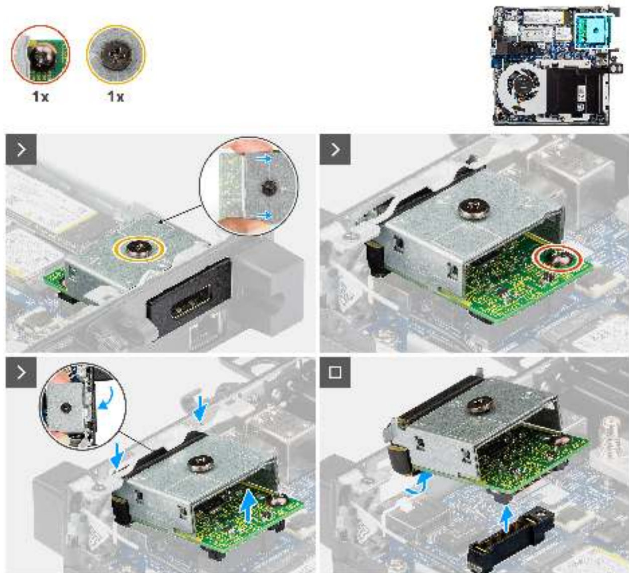
Abbildung 44. Entfernen des DisplayPort-Moduls
