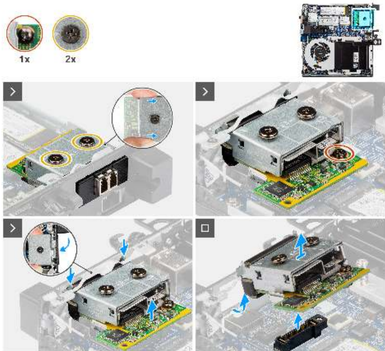
Abbildung 59. Entfernen des Glasfasermoduls
