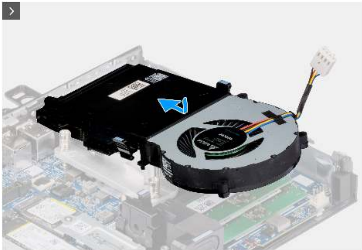
Abbildung 31. Einbauen des Lüfters
