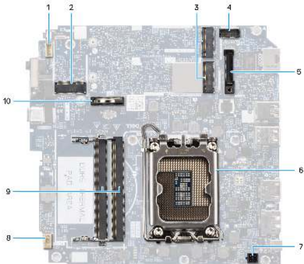
Abbildung 77. Anschlüsse auf der Hauptplatine
