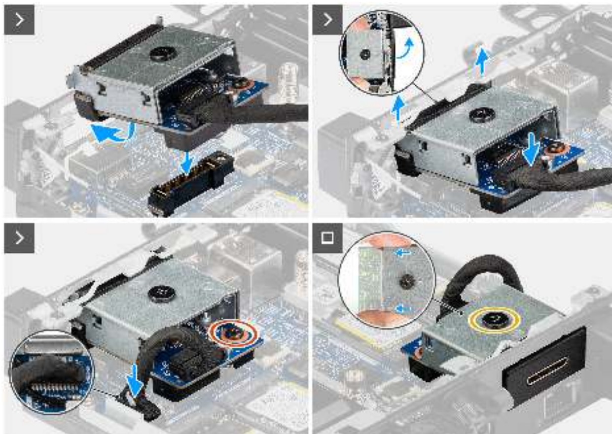
Abbildung 55. Einbauen des PS2-Anschlussmoduls
