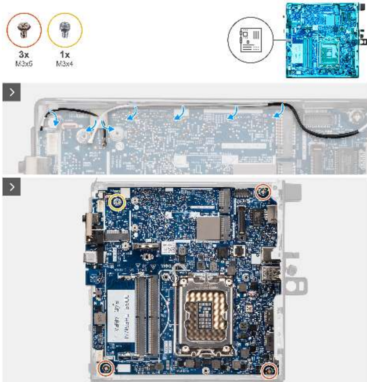
Abbildung 75. Entfernen der Systemplatine
