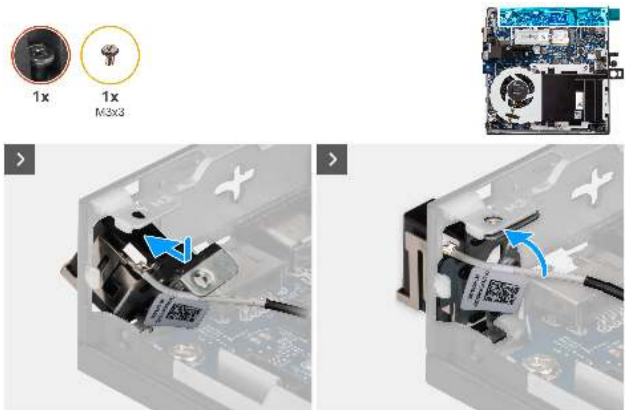
Abbildung 68. Einbauen des Antennenmoduls (weißes Kabel)
