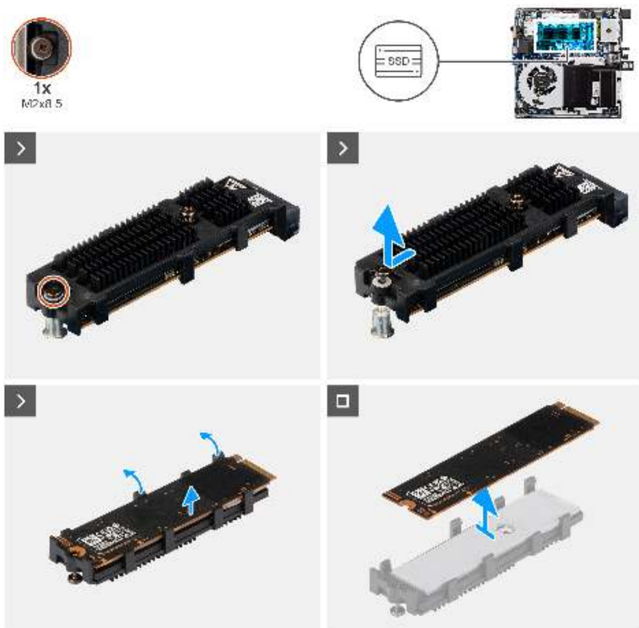
Abbildung 24. Entfernen des M.2 2280-PCIe-SSD-Laufwerks
