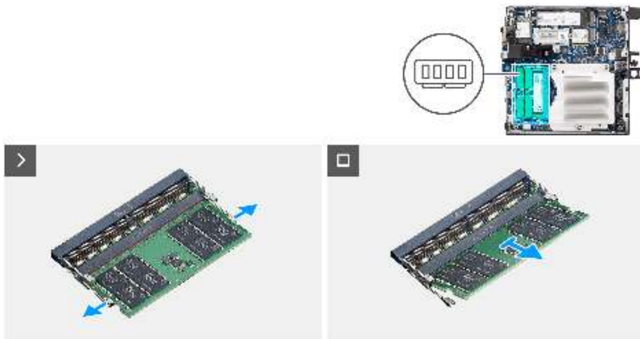
Abbildung 32. Entfernen des Arbeitsspeichers
