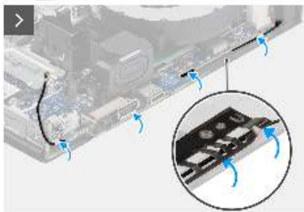
Abbildung 65. Einbauen des Antennenmoduls (schwarzes Kabel)
