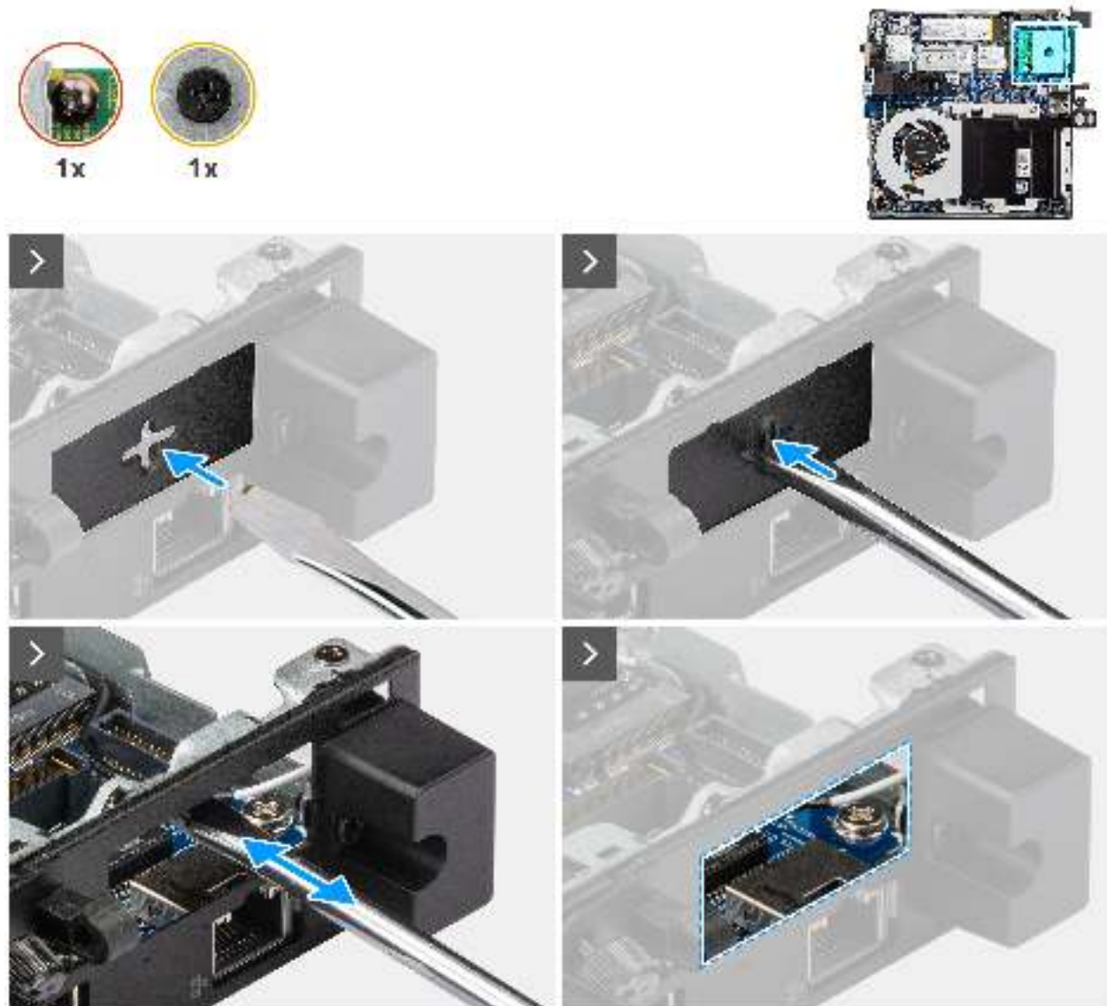
Abbildung 48. Einbauen des HDMI-Anschlussmoduls
