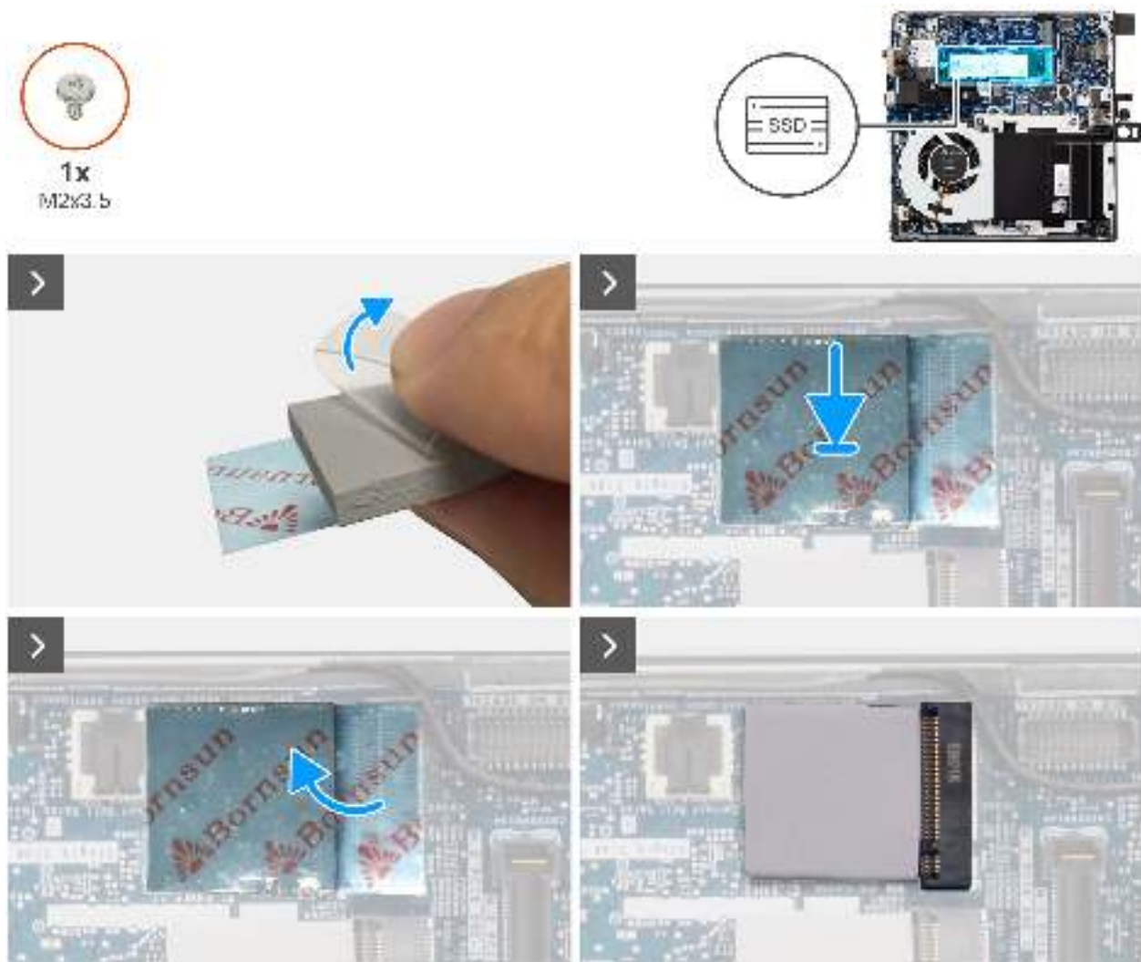
Abbildung 20. Einbauen des M.2-2280-Solid-State-Laufwerks
