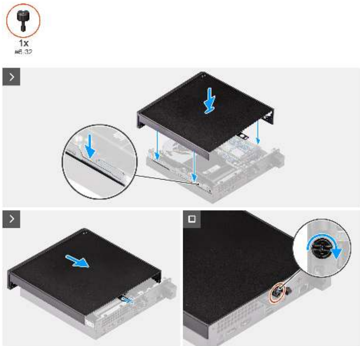
Abbildung 11. Anbringen der Seitenabdeckung
