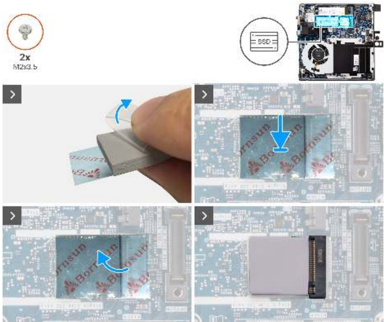
Abbildung 17. Einbauen des 2230-Solid-State-Laufwerks
