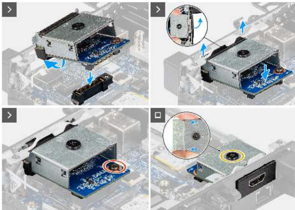
Abbildung 49. Einbauen des HDMI-Anschlussmoduls
