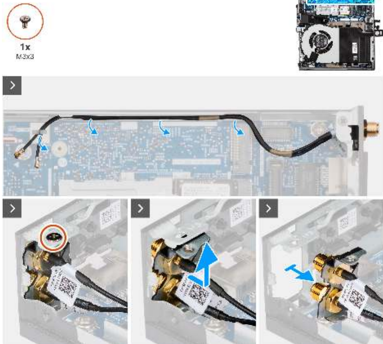
Abbildung 36. Entfernen der SMA-Antenne
