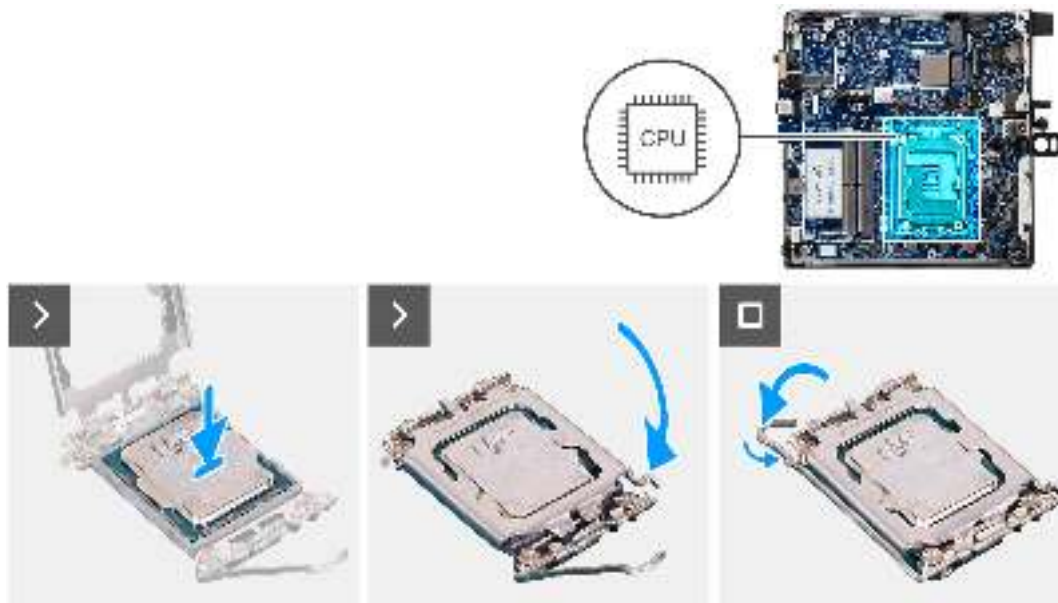
Abbildung 71. Einbauen des Prozessors
