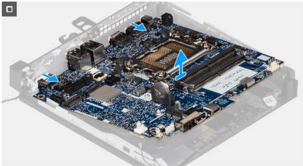
Abbildung 76. Entfernen der Systemplatine
