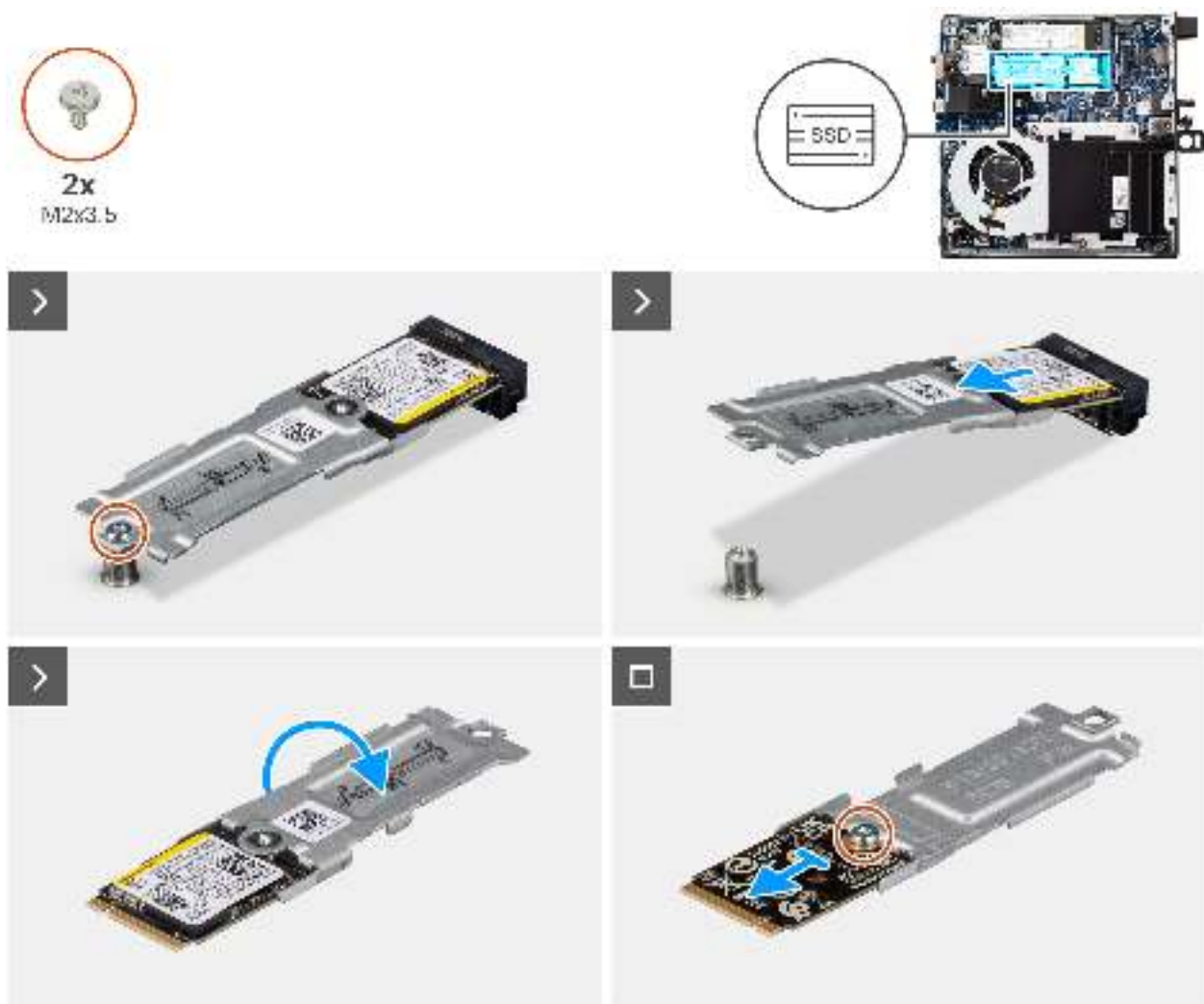
Abbildung 16. Entfernen des 2230-Solid-State-Laufwerks
