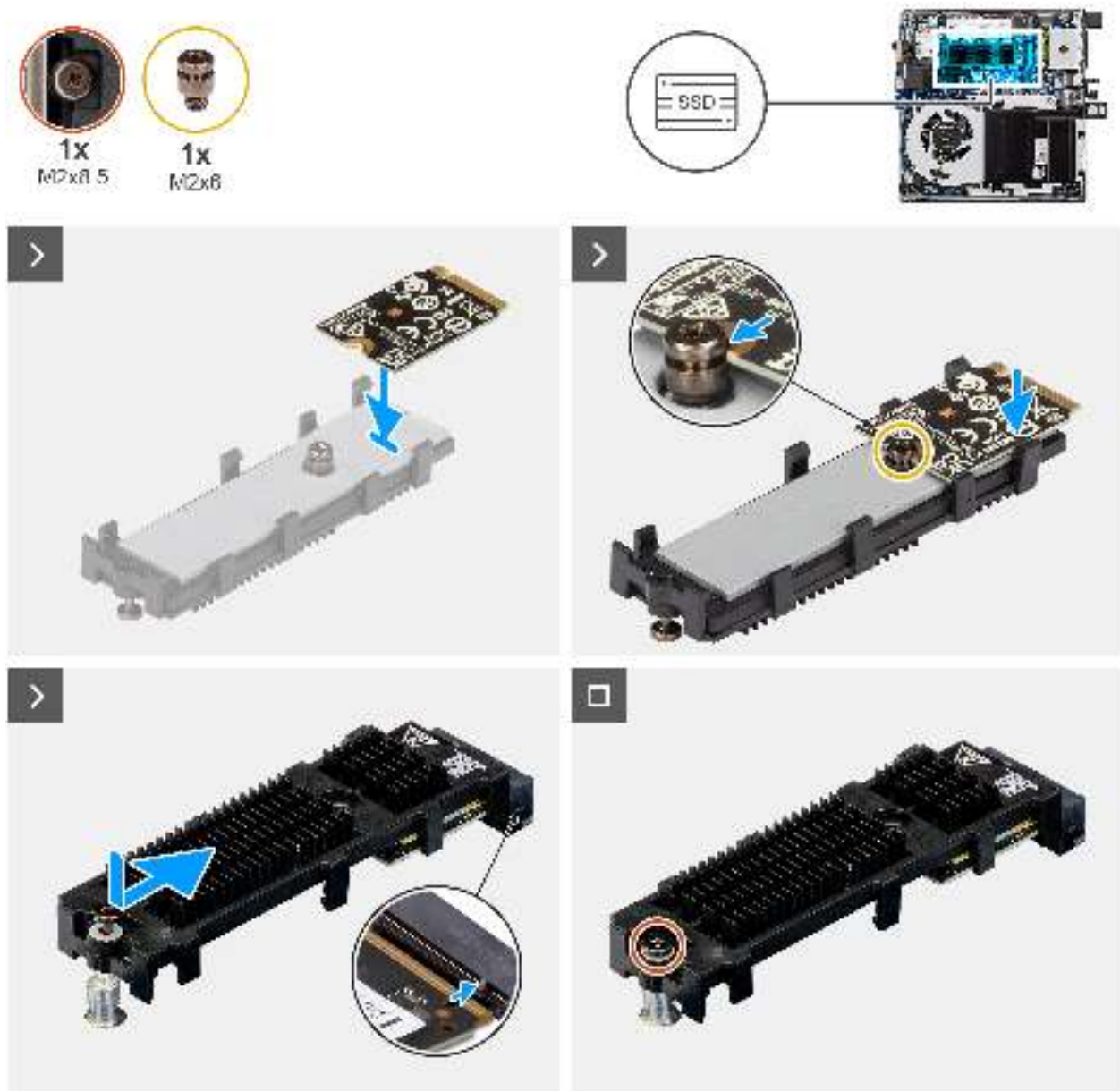
Abbildung 23. Einbauen des M.2 2230-PCIe-SSD-Laufwerks
