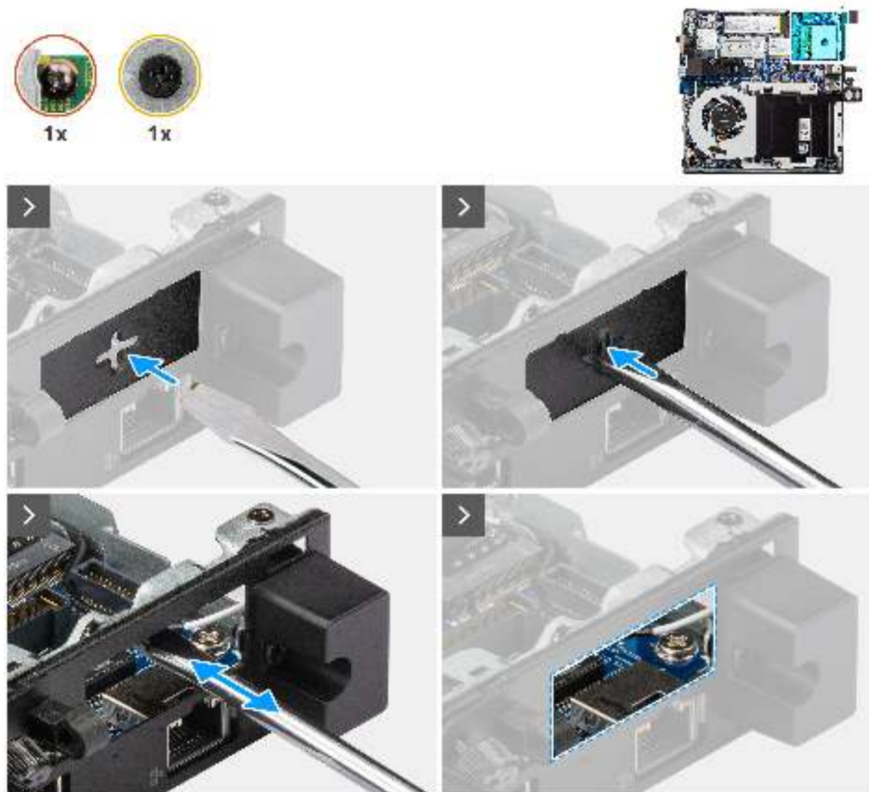
Abbildung 51. Installieren des VGA-Anschlussmoduls
