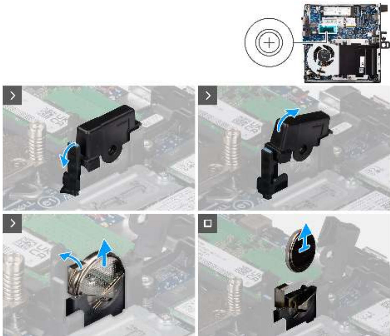
Abbildung 12. Entfernen der Knopfzellenbatterie
