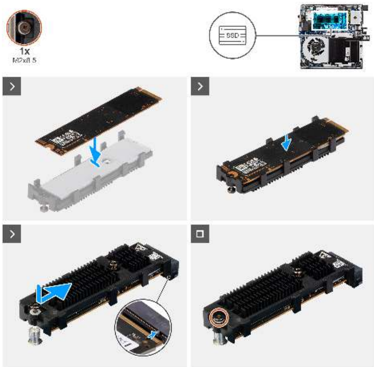
Abbildung 25. Einbauen des M.2 2280-PCIe-SSD-Laufwerks
