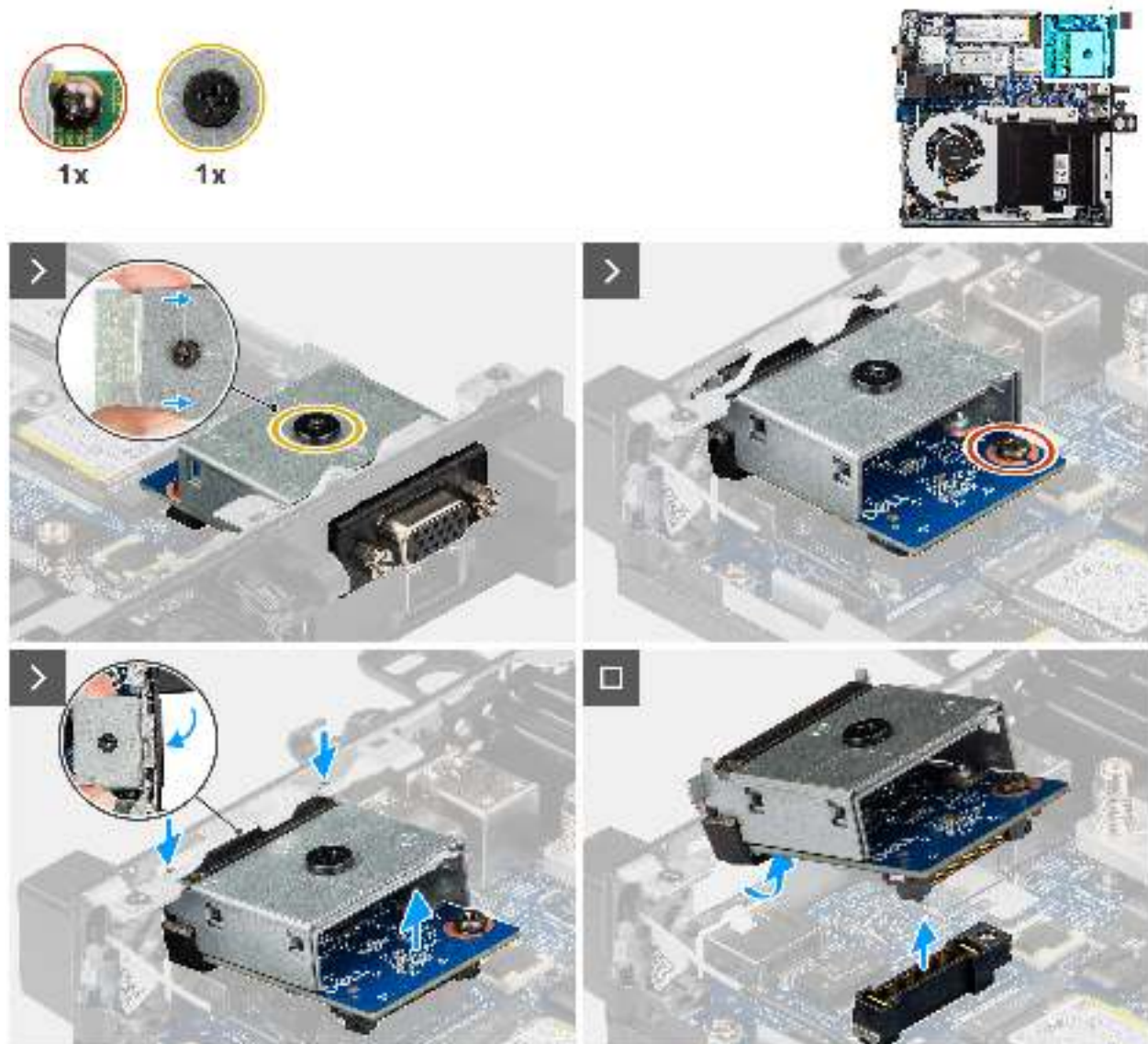
Abbildung 50. Entfernen des VGA-Anschlussmoduls
