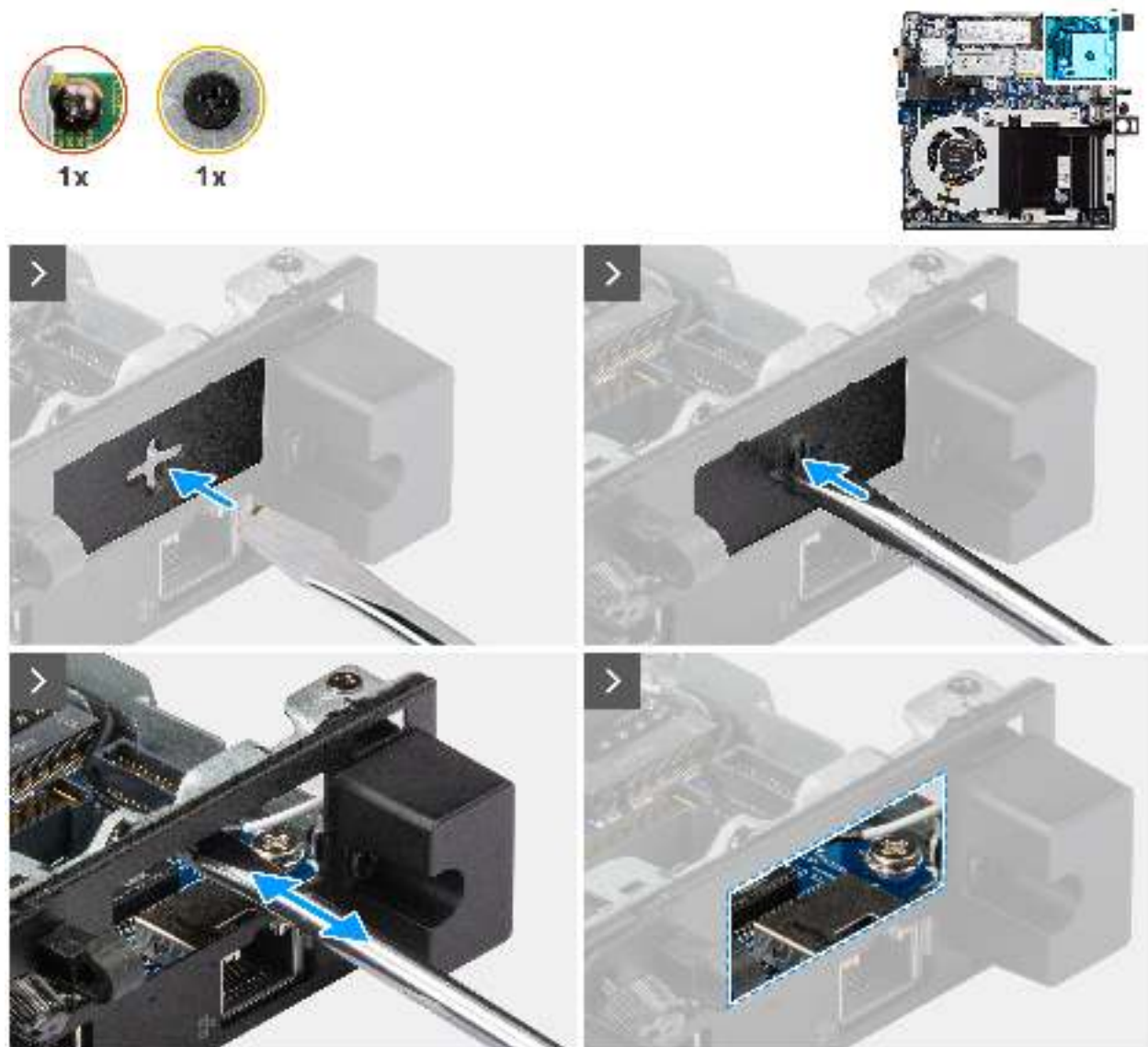
Abbildung 54. Einbauen des PS2-Anschlussmoduls
