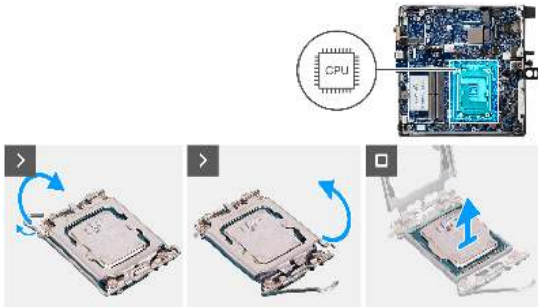
Abbildung 70. Entfernen des Prozessors
